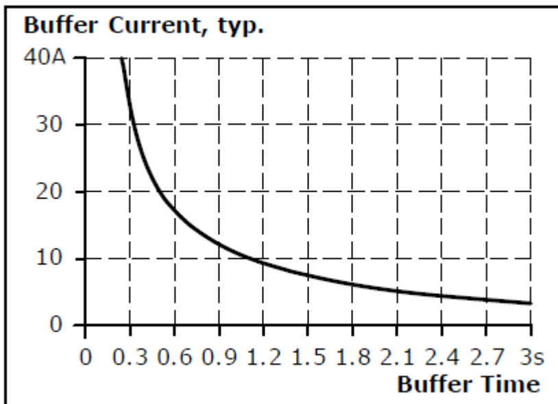
Abb. 9: Pufferzeit, typ.
