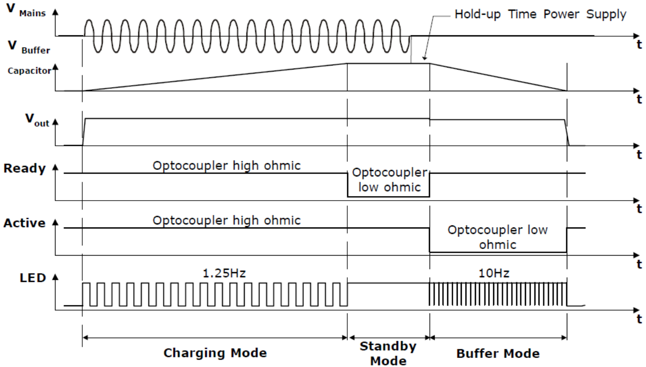
Abb. 12: Betriebsdiagramm
