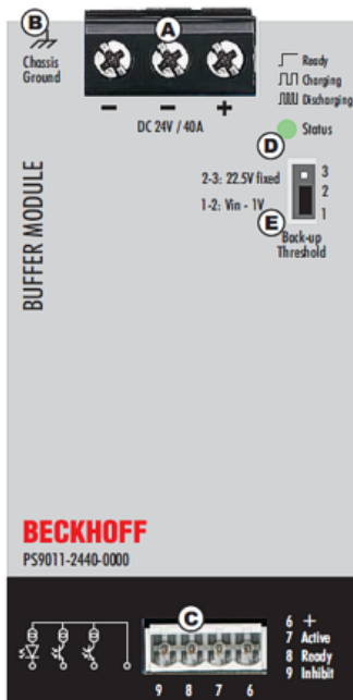
Abb. 17: Vorderseite PS9011-2440-0000
