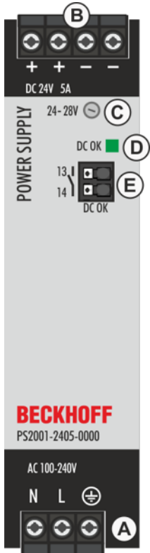
Abb. 14: Vorderseite PS2001-2405-0000
