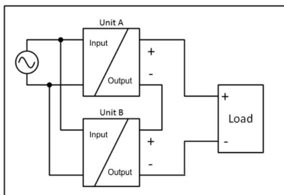
Abb. 21: Serienschaltung
