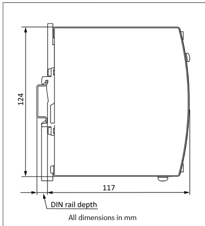
Abb. 16: Vorder-/Seitenansicht PS9731-2410-0000, alle Angaben in mm
