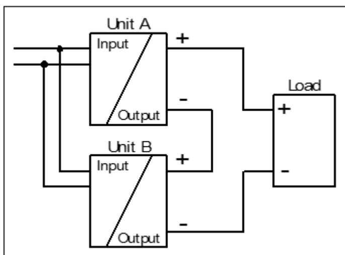
Abb. 19: Serienbetrieb
