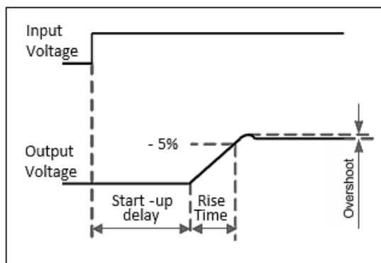
Abb. 1: Eingangsspannungsbereich, Einschaltverhalten, Definitionen
