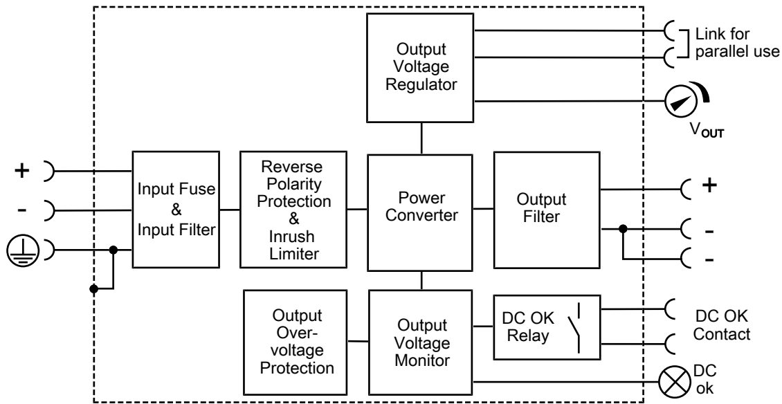
Abb. 12: Funktionsschaltbild
