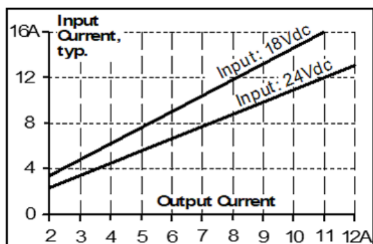
Abb. 2: Eingangsstrom vs. Ausgangslast
