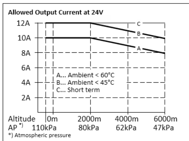
Abb. 14: Ausgangsstrom zu Umgebungstemperatur; Ausgangsstrom zu Höhe
