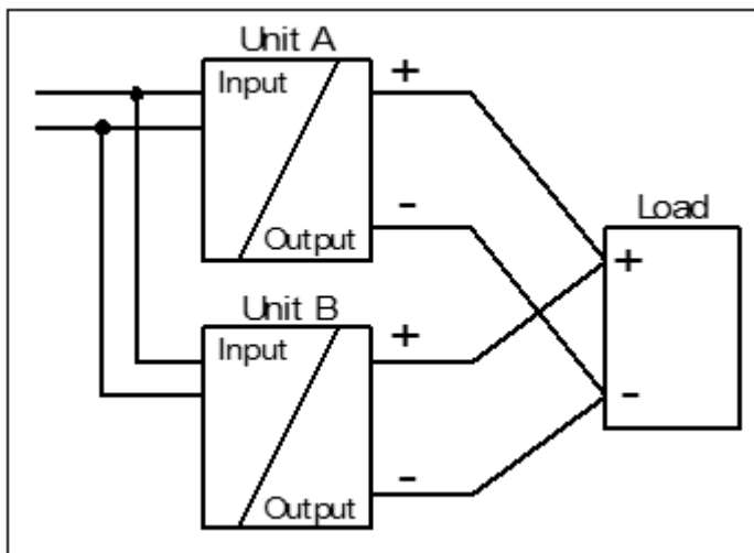
Abb. 20: Parallelschaltung
