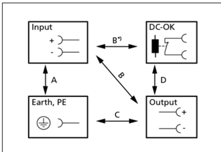
Abb. 15: Spannungsfestigkeit
