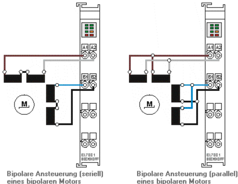
Abb. 32: Bipolaren Motoren
