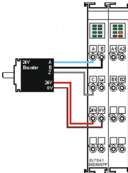
Abb. 45: Anschluss eines Encoders (24 V)
