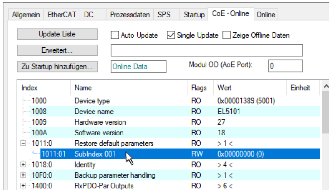
Abb. 216: Auswahl des PDO Restore default parameters
