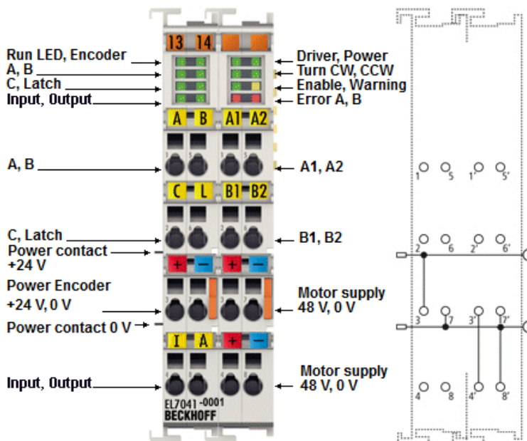
Abb. 6: EL7041-0001
