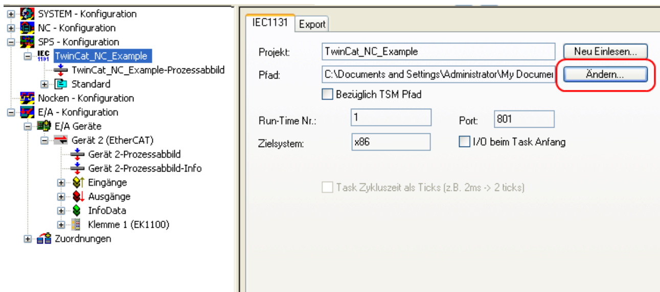
Abb. 196: Ändern des SPS-Pfades
