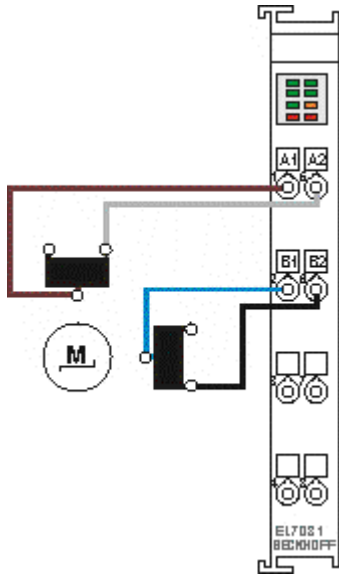
Abb. 33: Biopolare Ansteuerung eines unipolaren Motors, nur eine Hälfte jeder Wicklung wird angesteuert.
