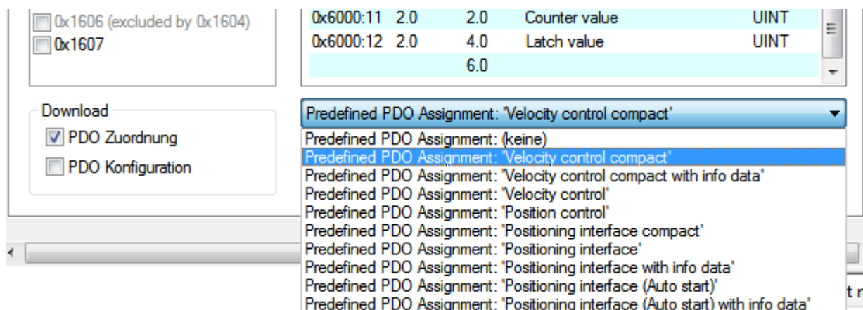
Abb. 193: Karteireiter Prozessdaten Predefined PDO Assignment, EL70xx
