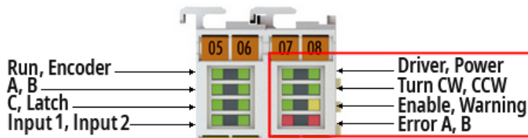
Abb. 35: EL7041-0000 LEDs (rechtes Prisma)
