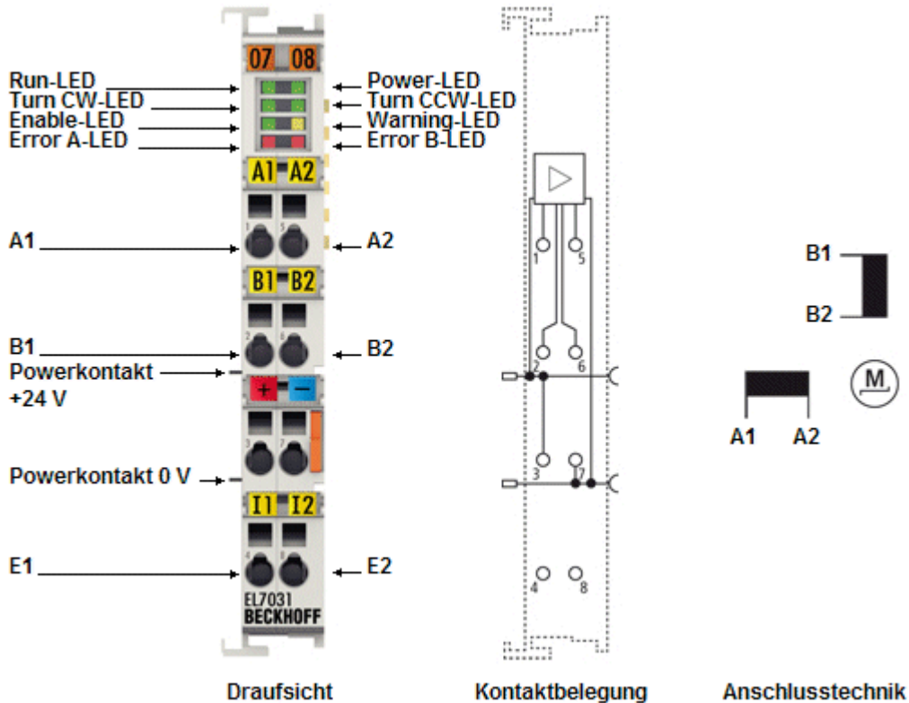
Abb. 4: EL7031
