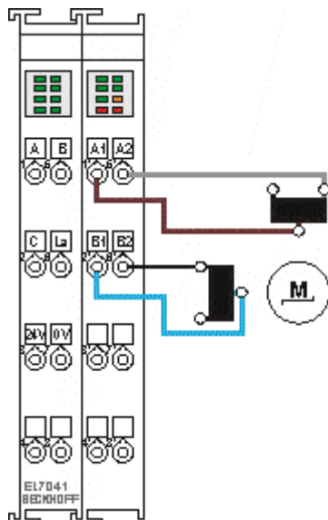
Abb. 44: Biopolare Ansteuerung eines unipolaren Motors
