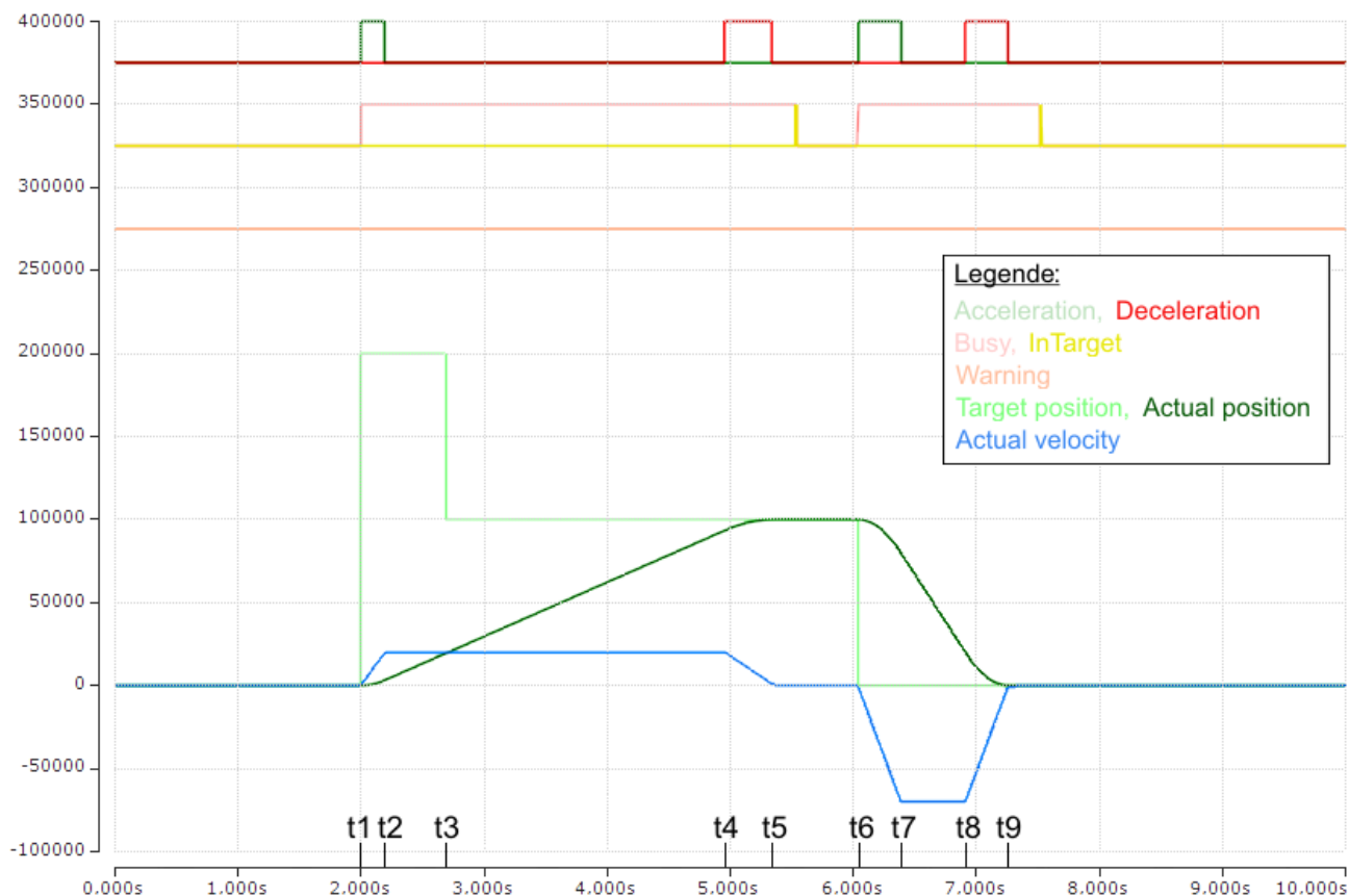
Abb. 189: Scope-Aufnahme ohne Überfahren der Zielposition
