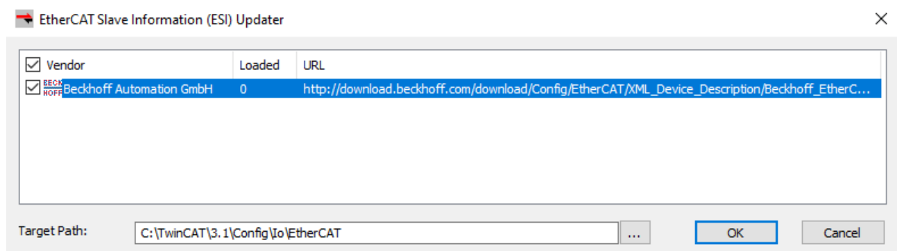
Abb. 104: (ESI) Updater
