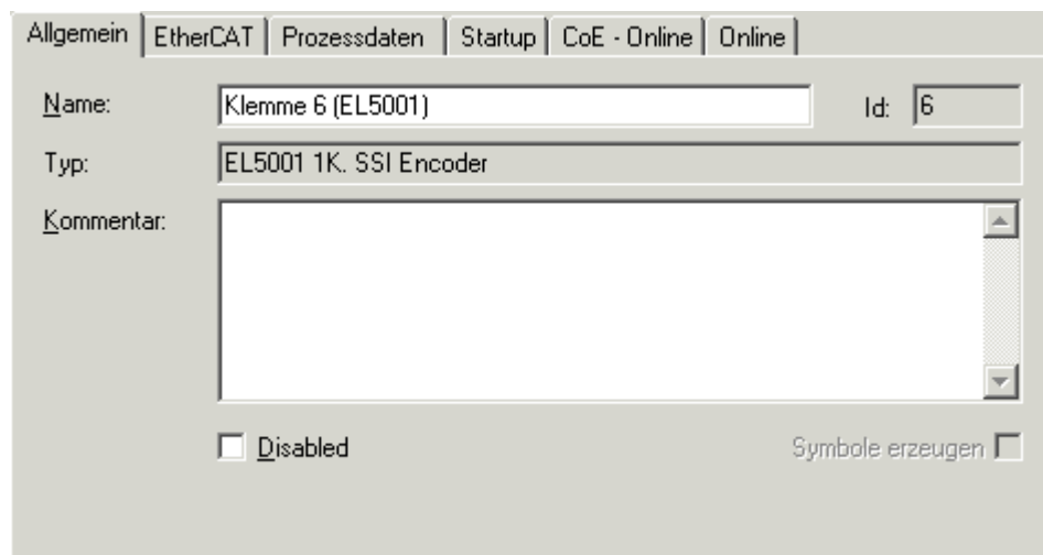
Abb. 138: Karteireiter „Allgemein“
