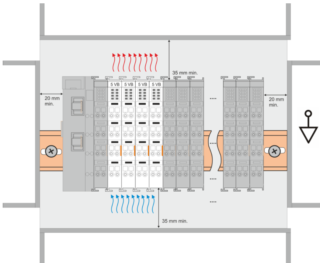
Abb. 26: Empfohlene Abstände Einbaulage bei Betrieb ohne Lüfter
