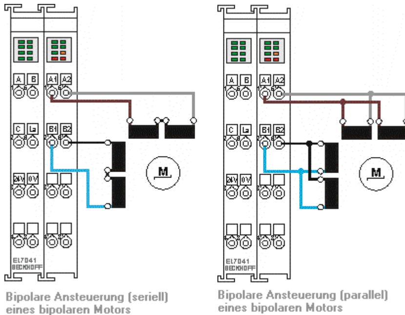
Abb. 43: Bipolaren Motoren
