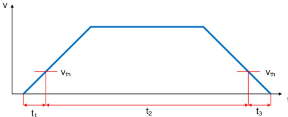
Abb. 174: Geschwindigkeitsrampe mit Grenzwerten des K v -Faktors
