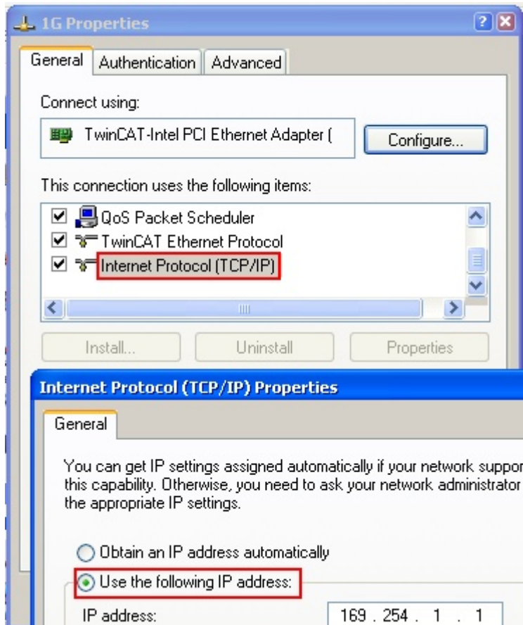
Abb. 96: TCP/IP-Einstellung des Ethernet Ports
