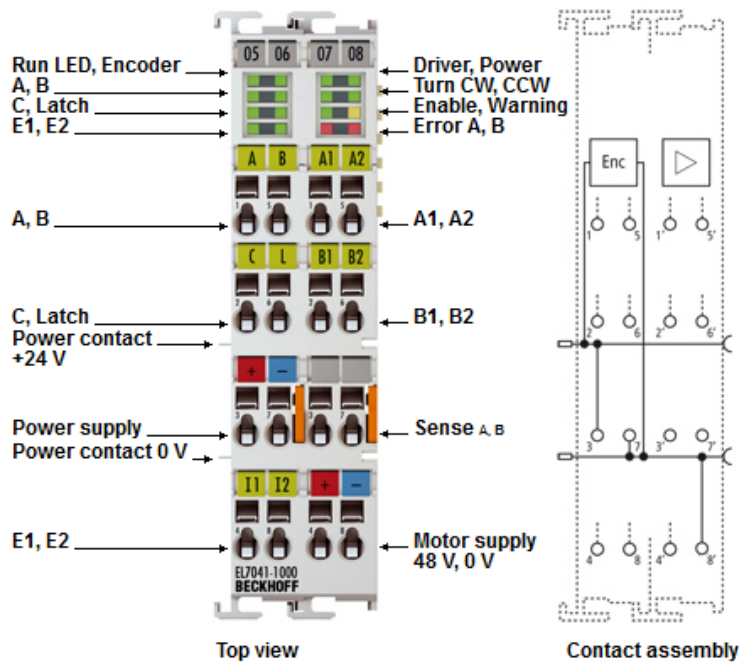
Abb. 42: EL7041-1000 - Anschlussbelegung
