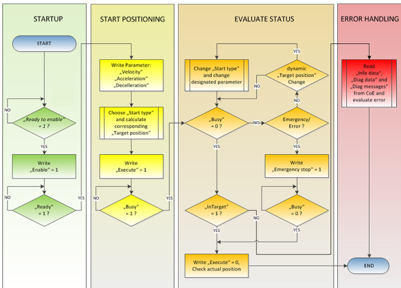
Abb. 181: Ablauf-Diagramm eines Fahrauftrages
