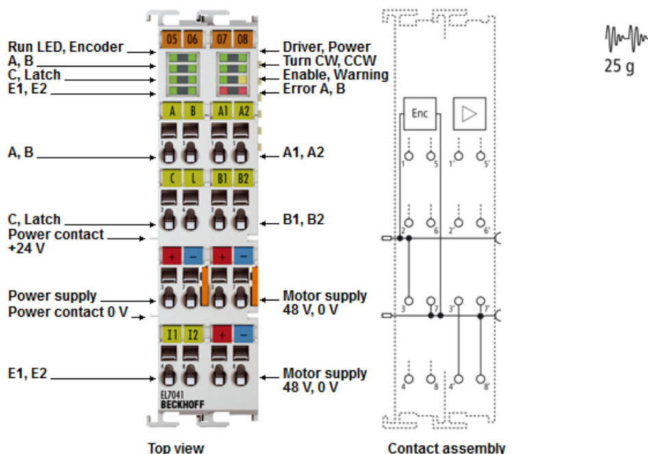
Abb. 36: EL7041-0000 Anschlussbelegung
