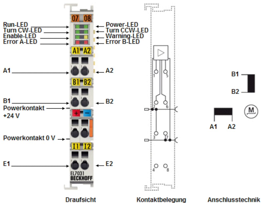
Abb. 31: Anschlussbelegung EL7031
