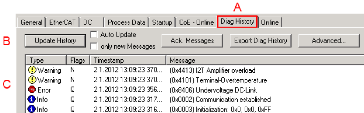
Abb. 203: Implementierung DiagMessage-System im TwinCAT System Manager
