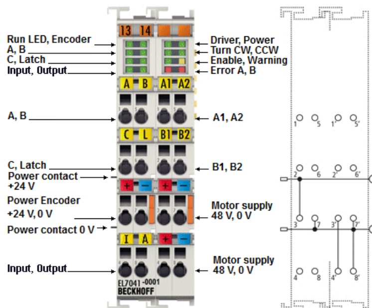
Abb. 39: EL7041-0001 Anschlussbelegung
