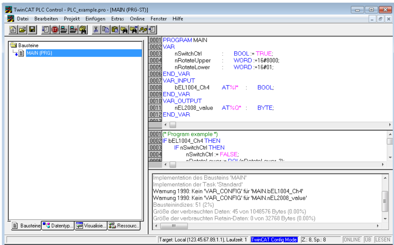
Abb. 56: Beispielprogramm mit Variablen nach einem Kompiliervorgang (ohne Variablenanbindung)
