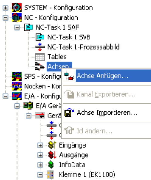
Abb. 158: Auswahl einer neuen Achse
