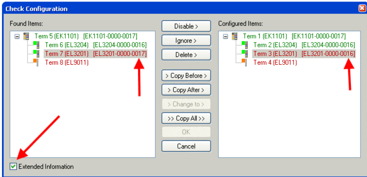
Abb. 207: Änderungsdialog
