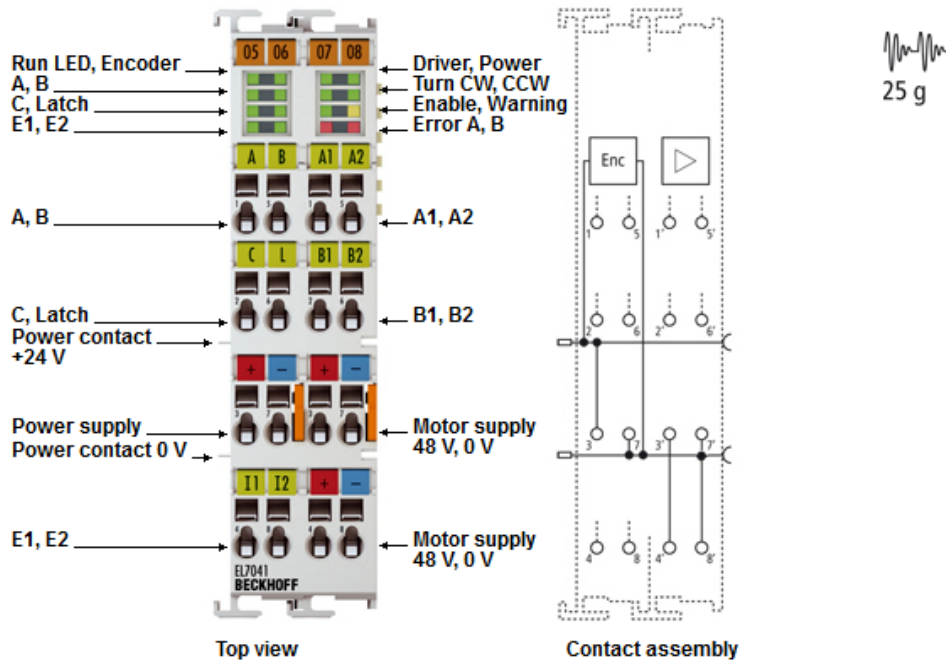
Abb. 5: EL7041-0000
