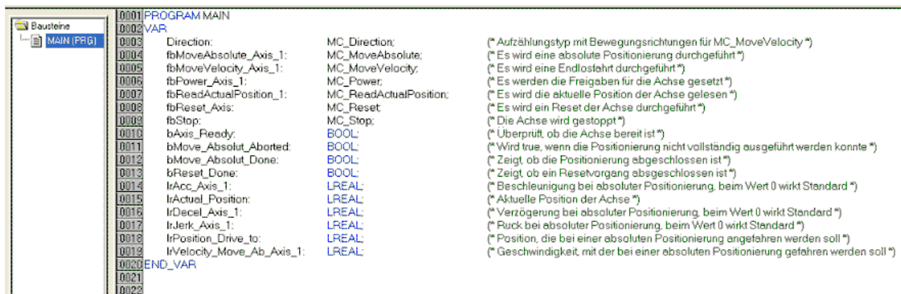
Abb. 199: Lokale Variablen
