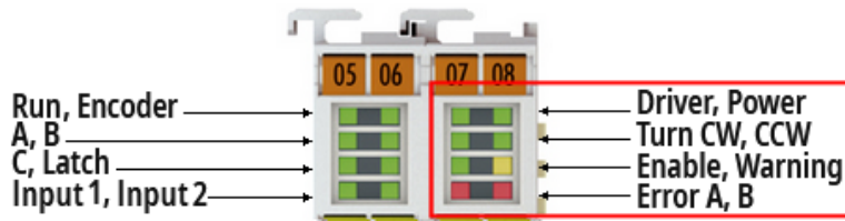
Abb. 41: EL7041-1000 LEDs (rechtes Prisma)
