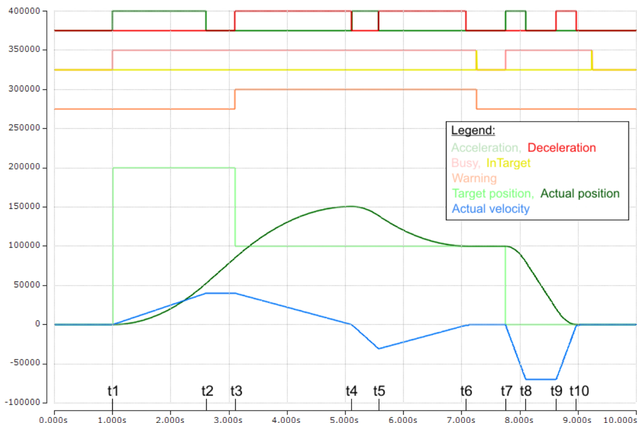
Abb. 176: Scope-Aufnahme mit Überfahren der endgültigen Zielposition
