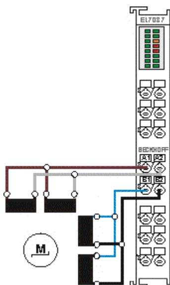
Abb. 30: Bipolare Ansteuerung (parallel) eines bipolaren Motors
