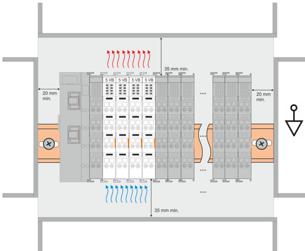
Abb. 23: Empfohlene Abstände Einbaulage bei Betrieb ohne Lüfter
