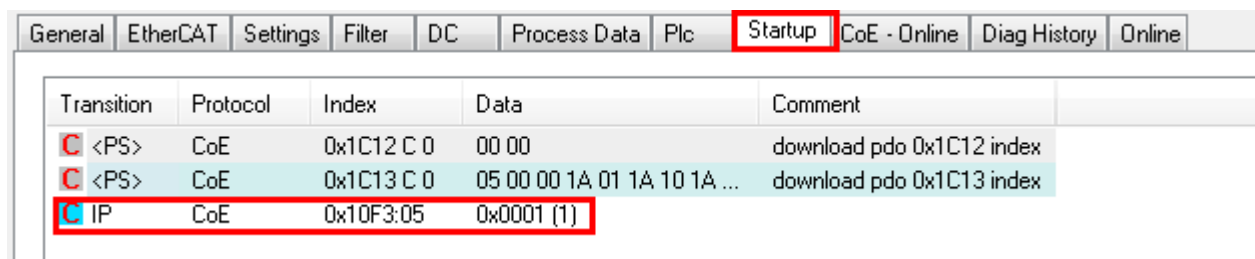
Abb. 199: StartUp-Liste
