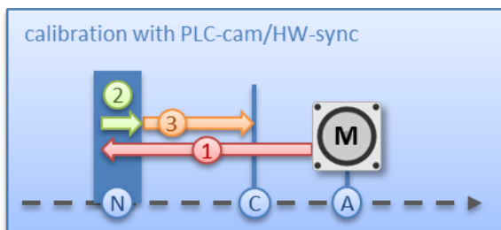
Abb. 173: Kalibrierung mit Nocke und C-Spur
