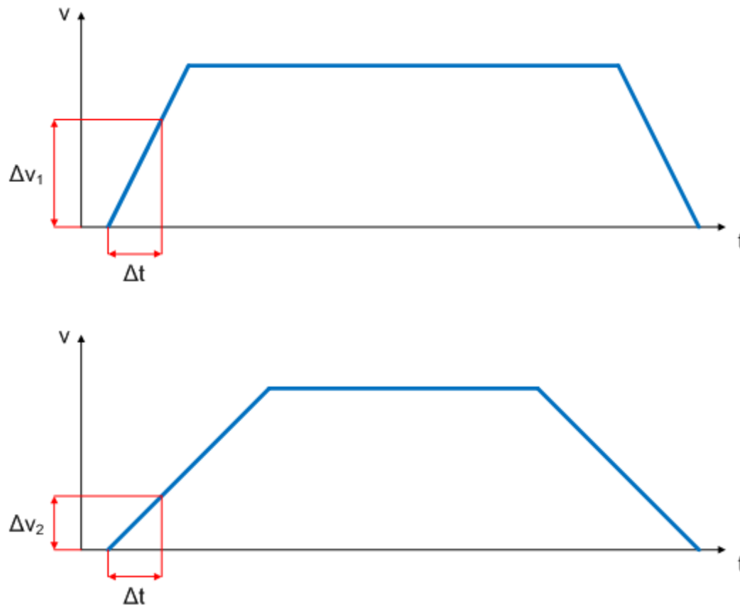
Abb. 154: Geschwindigkeitsrampen
