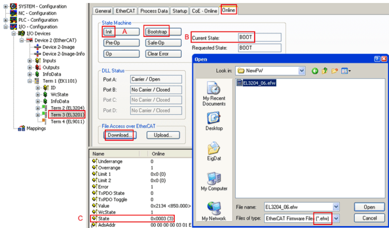
Abb. 207: Firmware Update
