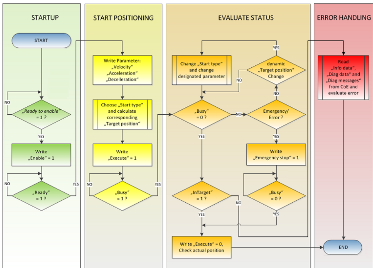
Abb. 167: Ablauf-Diagramm eines Fahrauftrages
