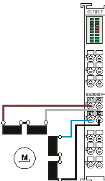
Abb. 29: Bipolare Ansteuerung (seriell) eines bipolaren Motors
