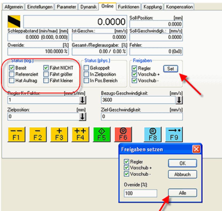
Abb. 149: Achse freigeben
