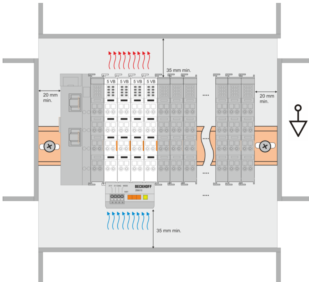
Abb. 24: Empfohlene Abstände bei Betrieb mit Lüfter
