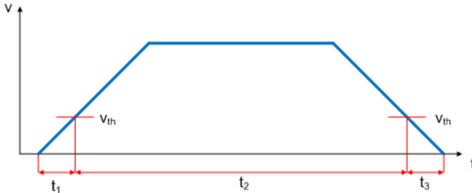
Abb. 160: Geschwindigkeitsrampe mit Grenzwerten des K v -Faktors
