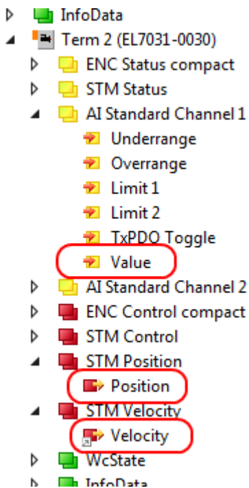
Abb. 183: notwendige PDOs
