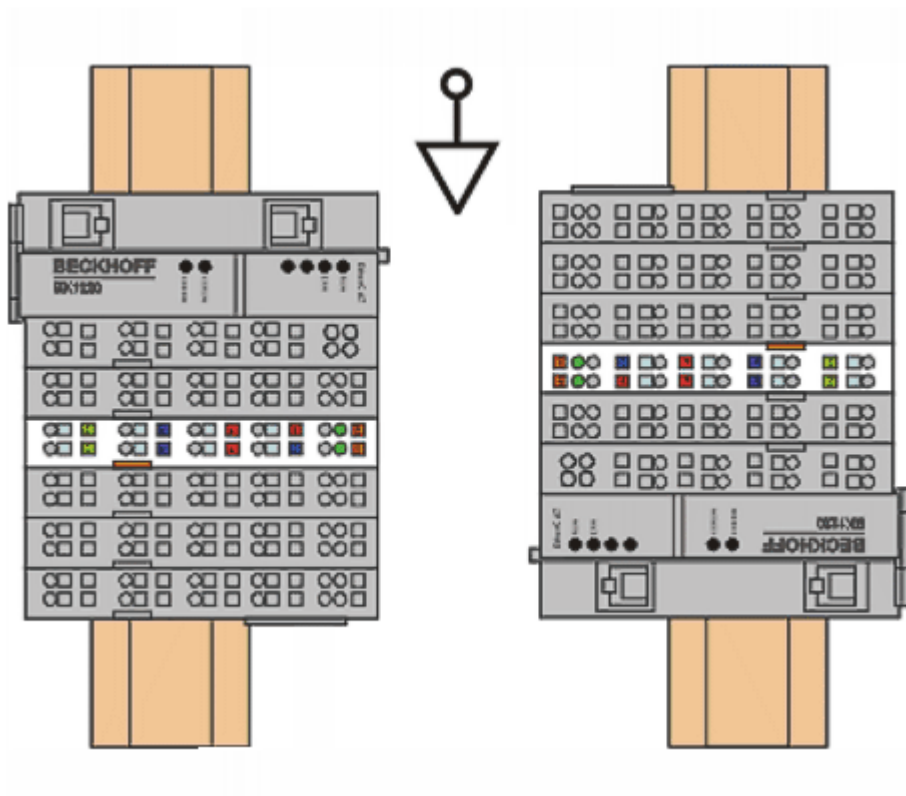
Abb. 25: Weitere Einbaulagen, Beispiel 1
