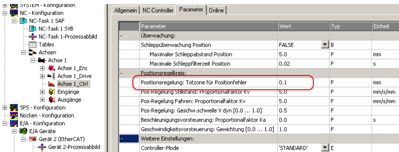
Abb. 162: Totzone für Positionsfehler
