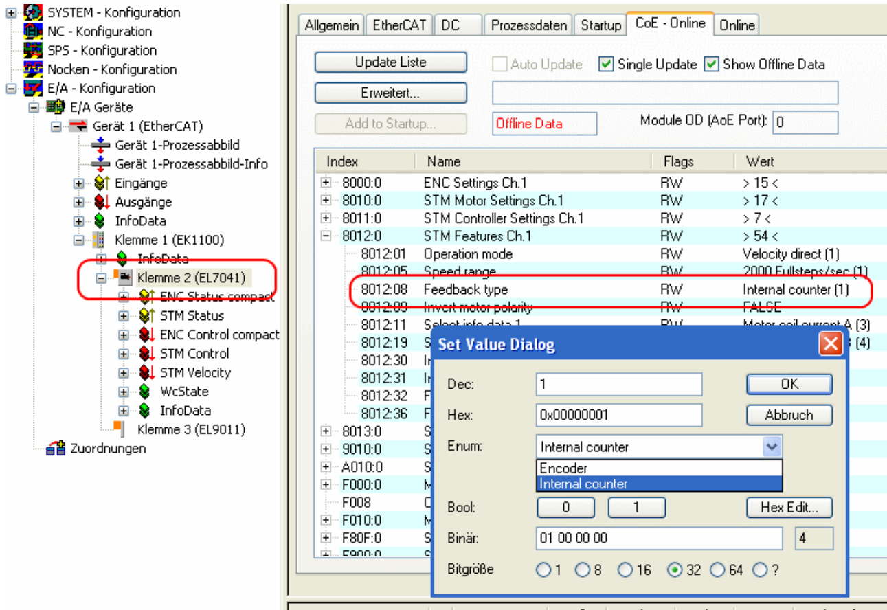
Abb. 153: Feedbacksystem auswählen
