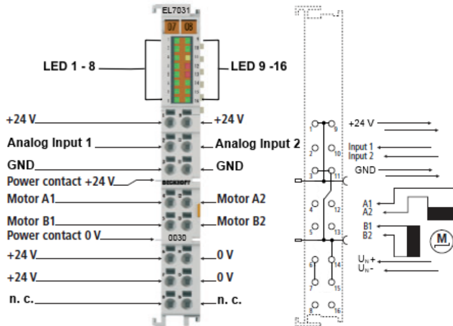
Abb. 27: LEDs und Anschluss EL7031-0030
