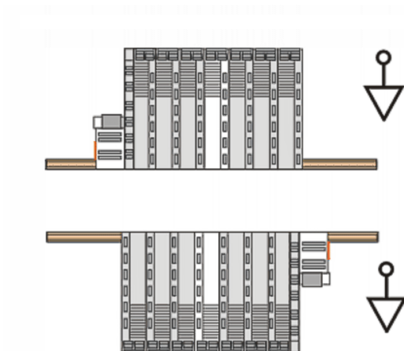
Abb. 25: Weitere Einbaulagen, Beispiel 1
