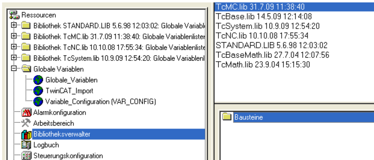
Abb. 192: Erforderliche Bibliotheken
