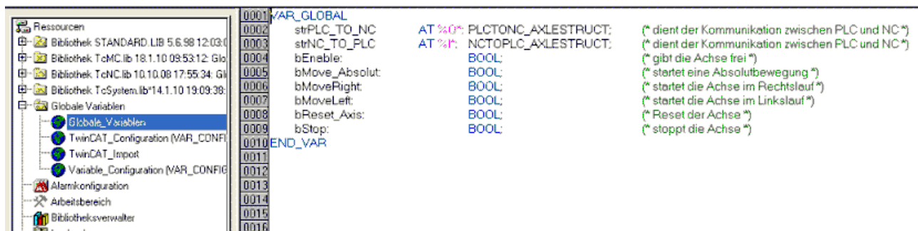
Abb. 193: Globale Variablen
