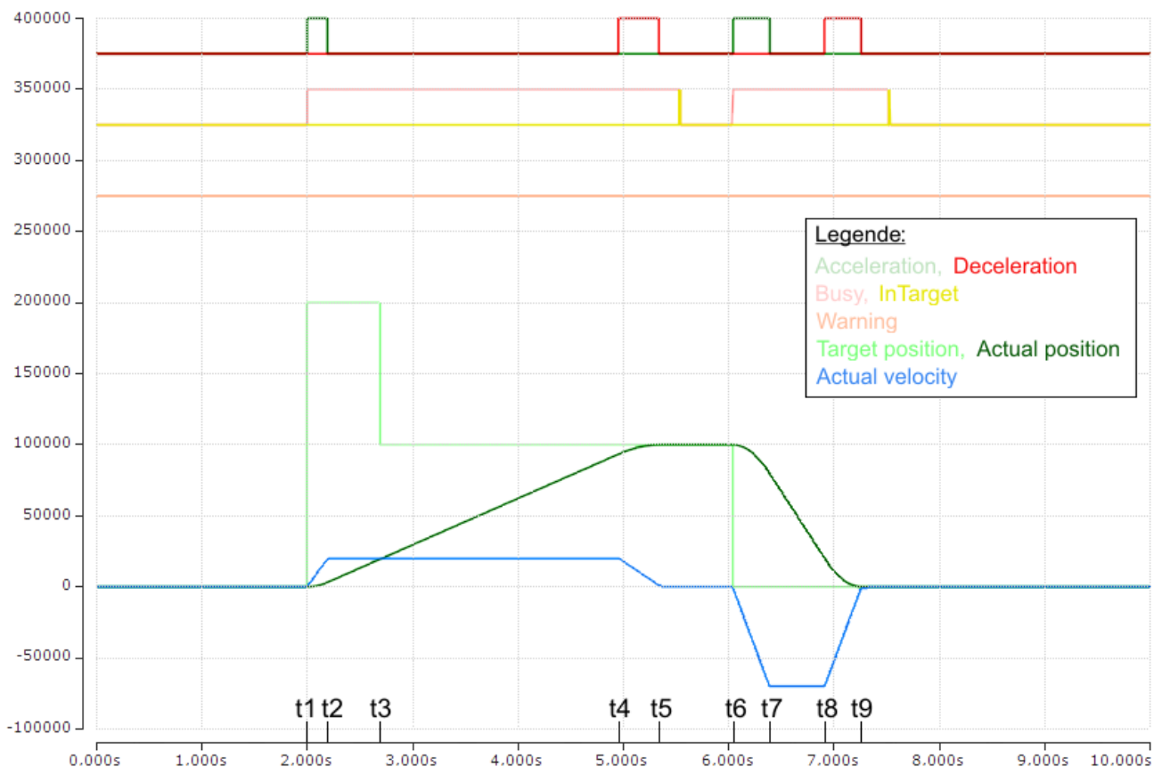
Abb. 175: Scope-Aufnahme ohne Überfahren der Zielposition
