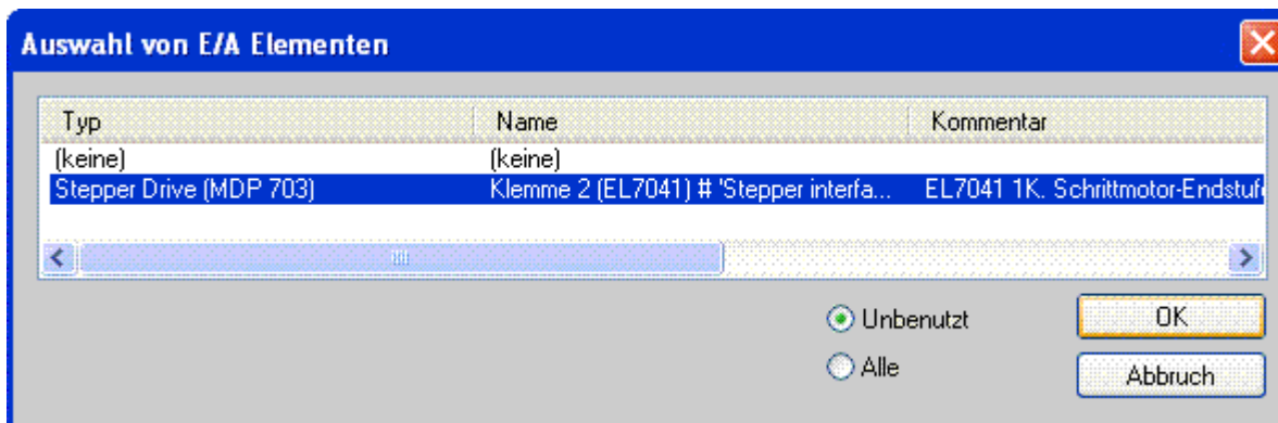
Abb. 147: Auswahl der richtigen Klemme
