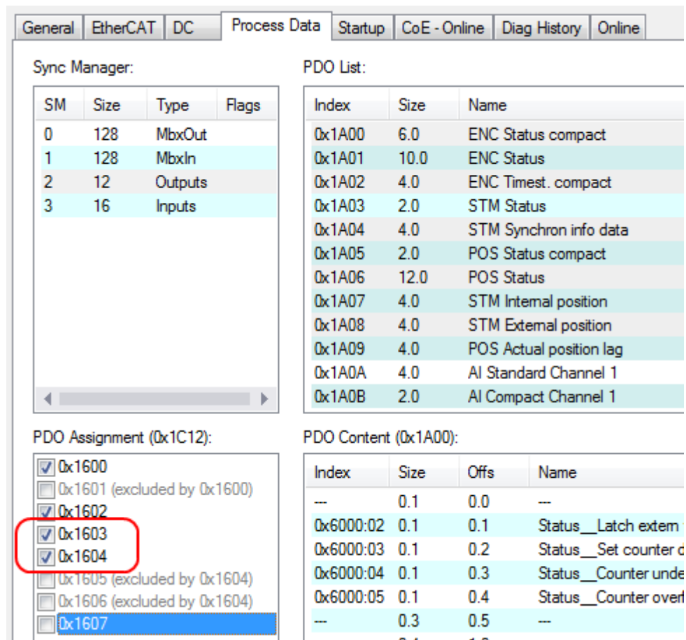
Abb. 182: PDOs aktivieren
