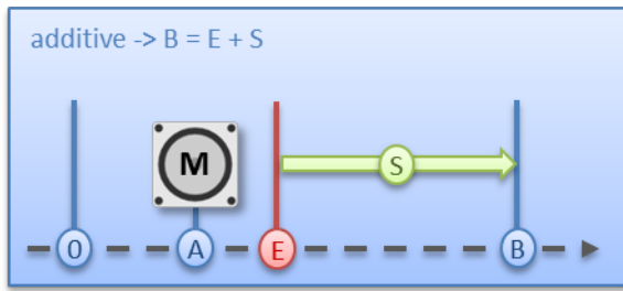
Abb. 171: Additive Positionierung
