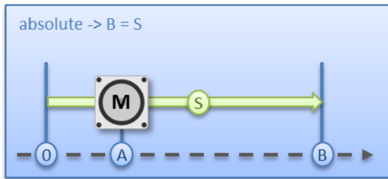
Abb. 168: Absolute Positionierung
