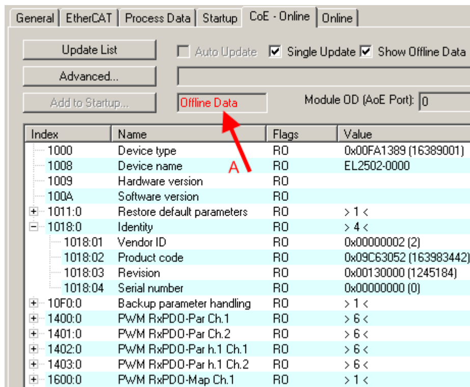
Abb. 10: Offline-Verzeichnis
