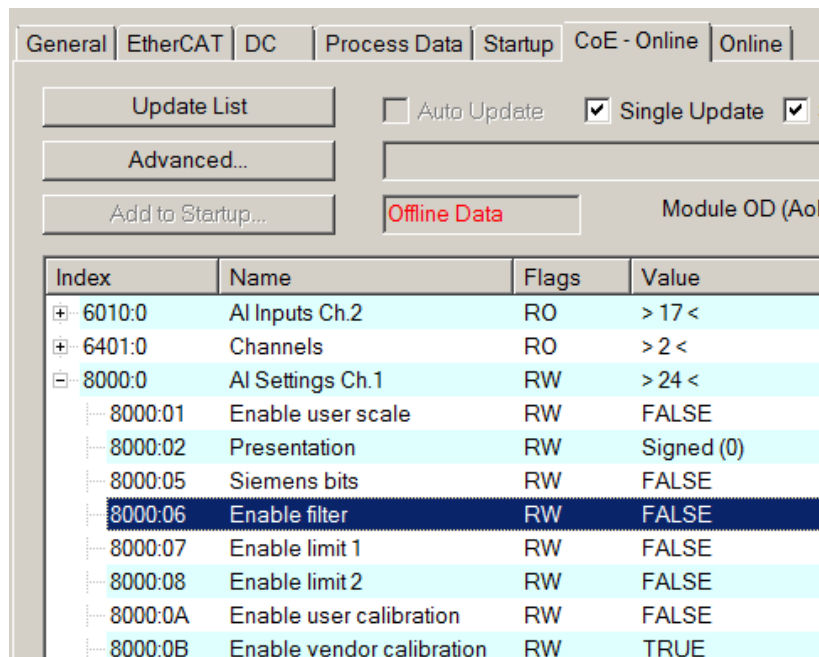
Abb. 136: EL3102, CoE-Verzeichnis
