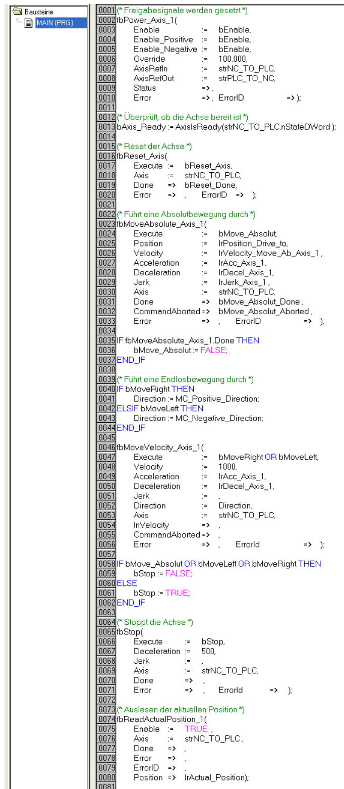
Abb. 195: Programmcode
