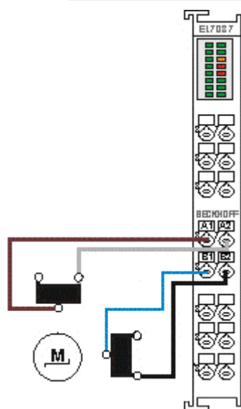
Abb. 31: Bipolare Ansteuerung eines unipolaren Motors
