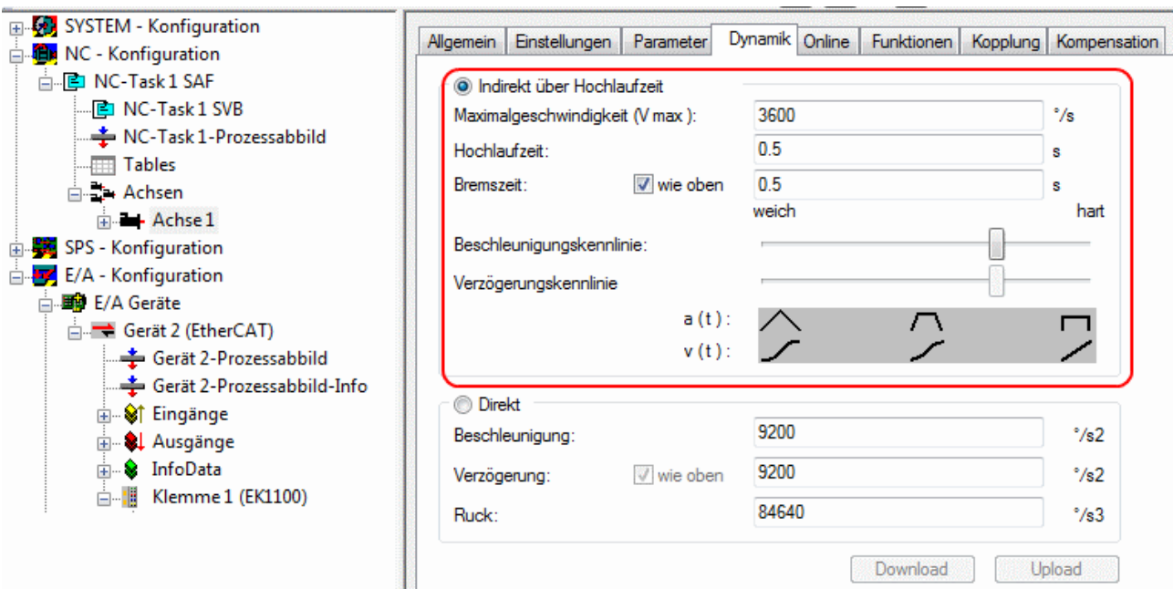
Abb. 163: Einstellung der Hochlaufzeit im Reiter „Dynamik“
