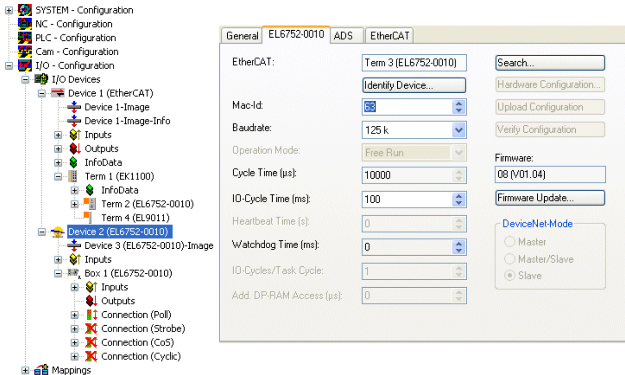
Fig. 33: "EL6752-0010" tab
