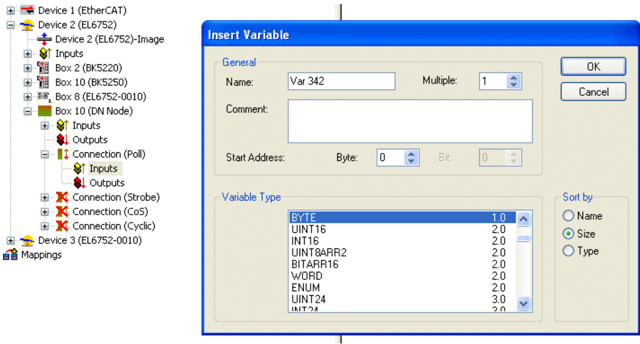
Fig. 51: Add Variables
