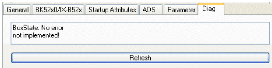
Fig. 59: "Diag" tab
