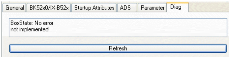
Fig. 45: "Diag" tab
