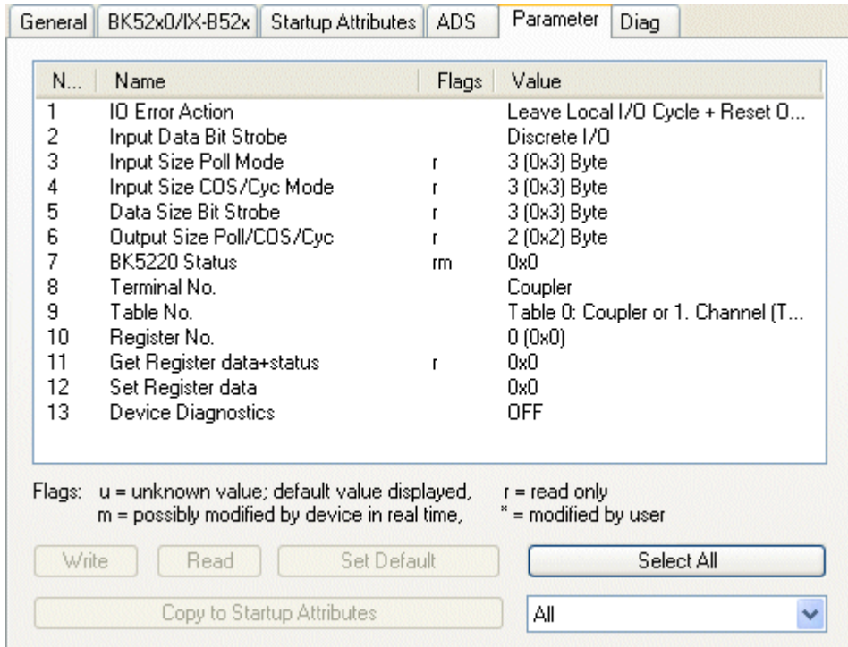
Fig. 44: “Parameter” tab
