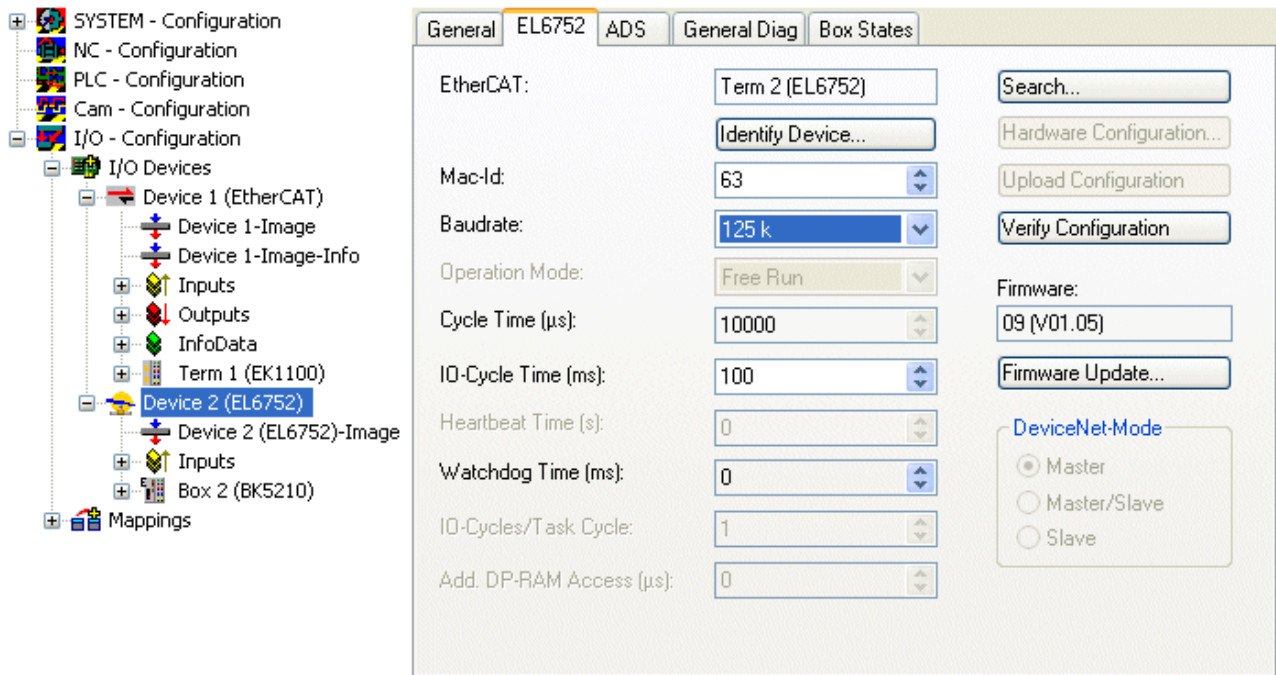
Fig. 28: "EL6752" tab
