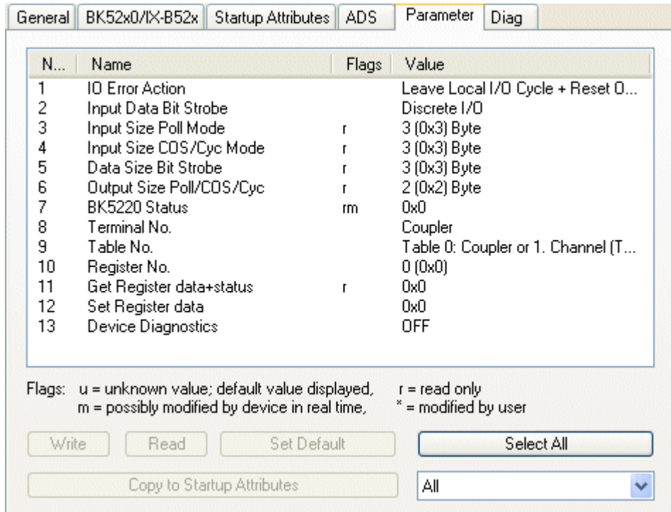
Fig. 58: “Parameter” tab
