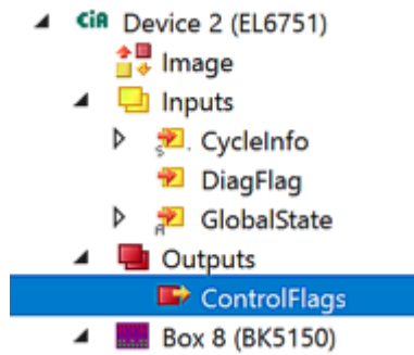
Fig. 127: Variable ControlFlags
