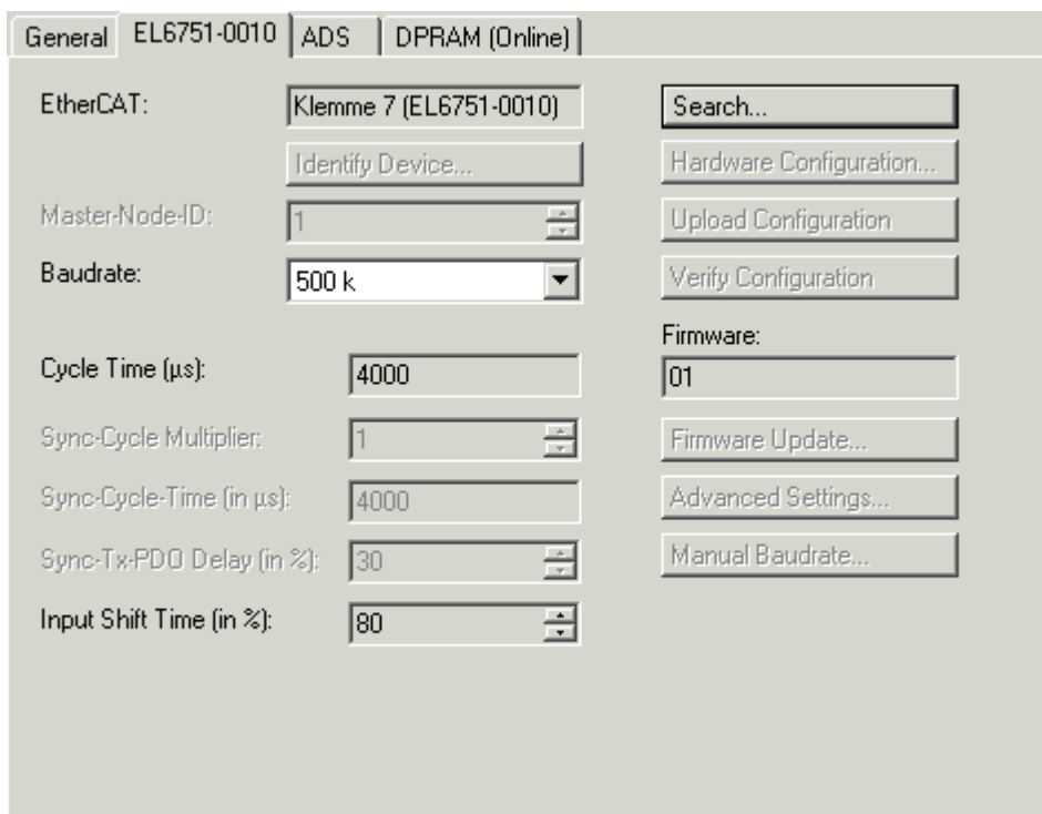
Fig. 94: "EL6751-0010" tab
