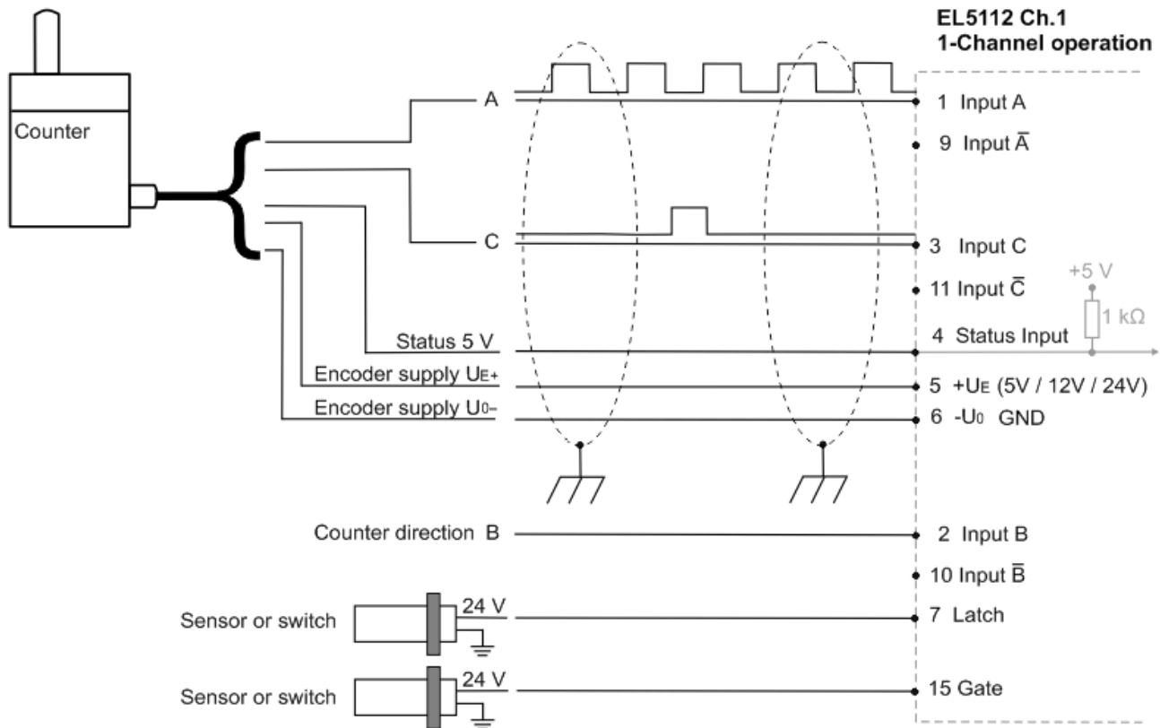
Abb. 31: Anschluss Zähler / Impulsgeber TTL - Mode mit Nullimpuls im 1-Kanal-Betrieb
