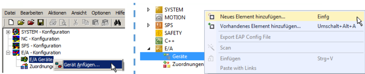
Abb. 101: Anfügen eines EtherCAT Device: links TwinCAT 2; rechts TwinCAT 3
