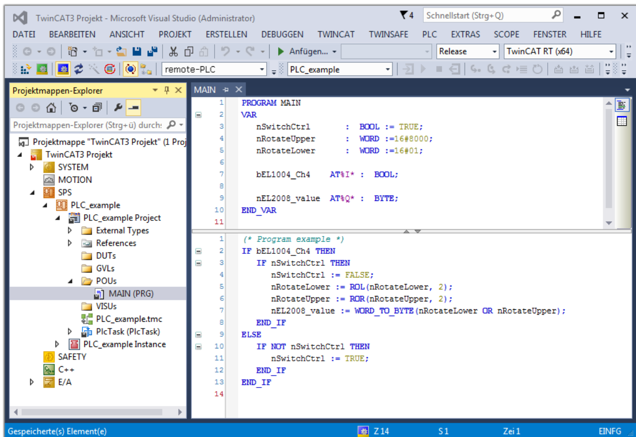
Abb. 73: Beispielprogramm mit Variablen nach einem Kompiliervorgang (ohne Variablenanbindung)
