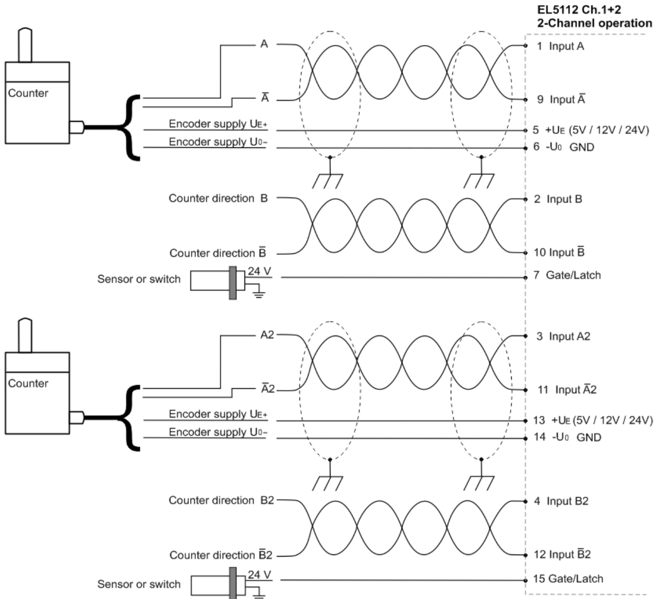
Abb. 35: Anschluss Zähler / Impulsgeber RS422 - Mode ohne Nullimpuls im 2-Kanal-Betrieb
