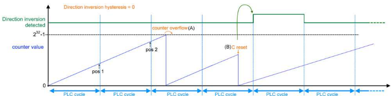
Abb. 164: Detektion der Zählrichtung
