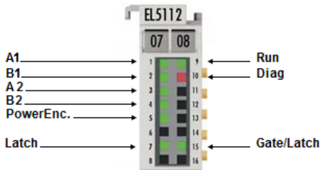
Abb. 41: EL5112 - LEDs im 2-Kanal-Betrieb
