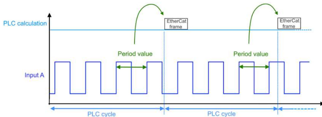
Abb. 169: Periodendauermessung
