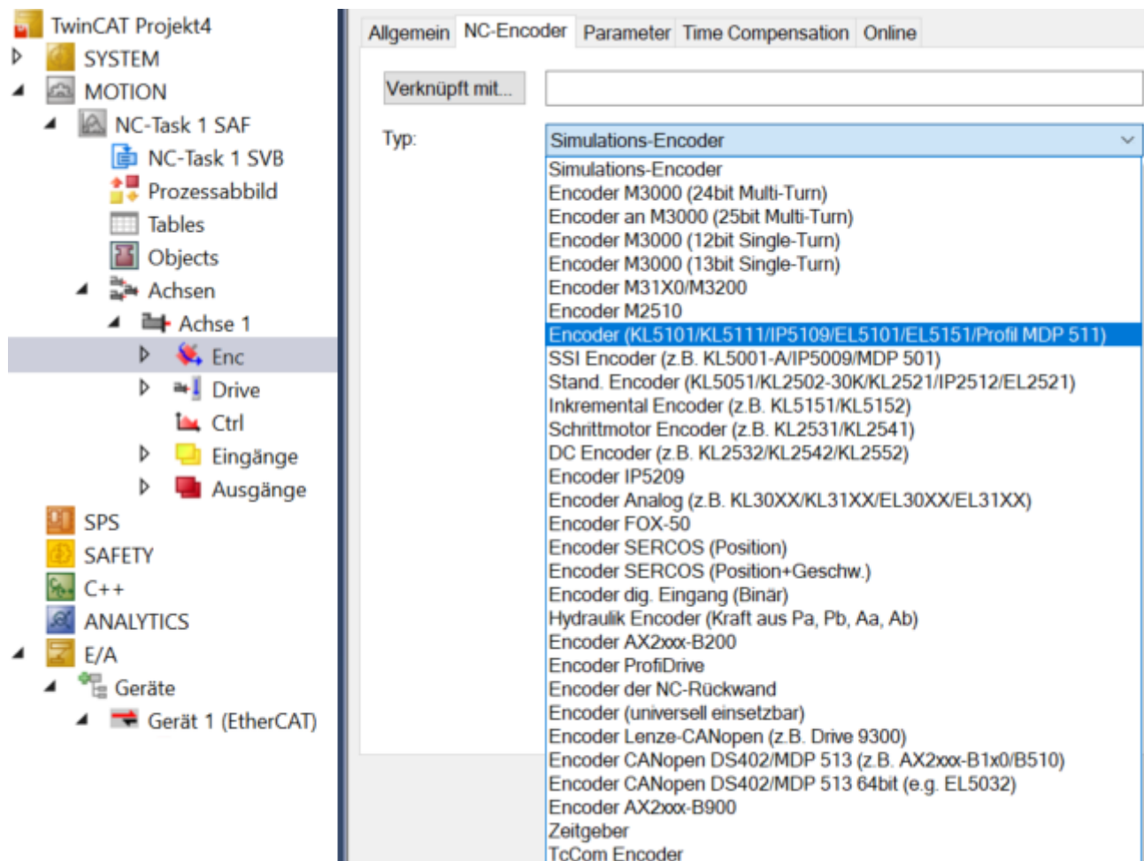
Abb. 146: Auswahl des Encoders
