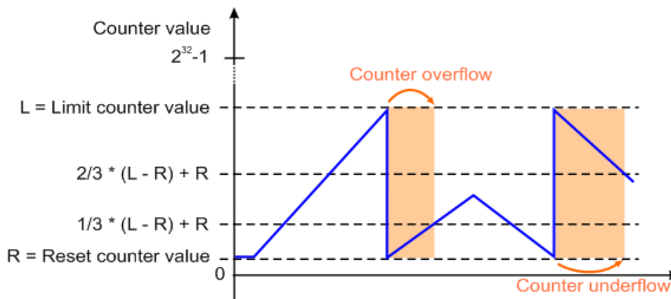
Abb. 161: Über- und Unterschreiten der Zählergrenzen mit festgelegtem Wertebereich
