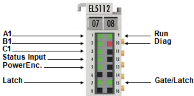
Abb. 40: EL5112 - LEDs im 1-Kanal-Betrieb
