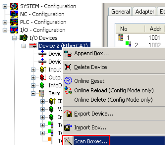
Abb. 187: Rechtsklick auf das EtherCAT-Gerät bewirkt das Scannen des unterlagerten Feldes
