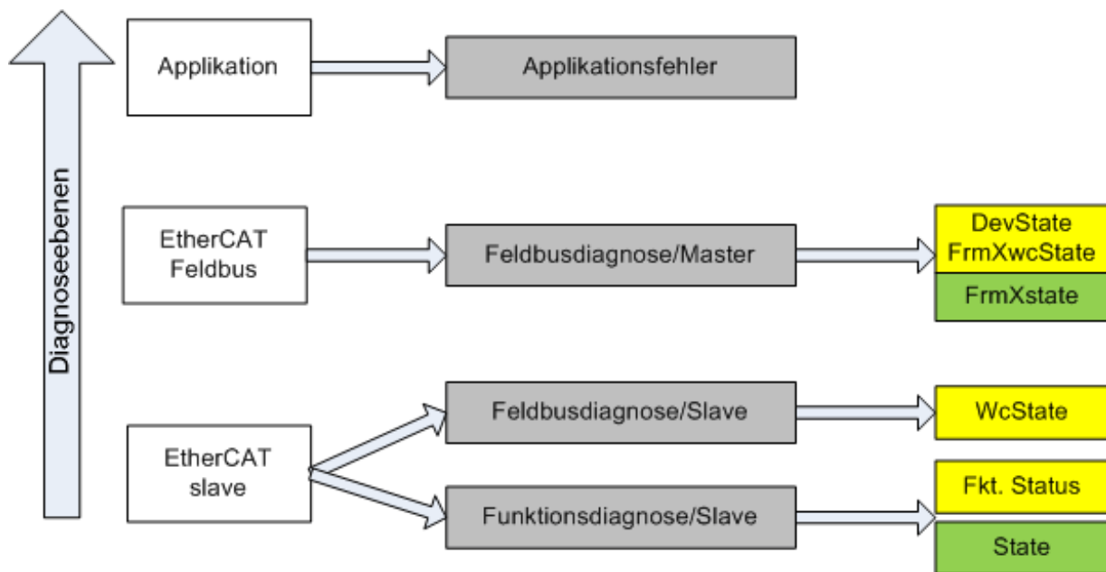
Abb. 149: Auswahl an Diagnoseinformationen eines EtherCAT-Slaves
