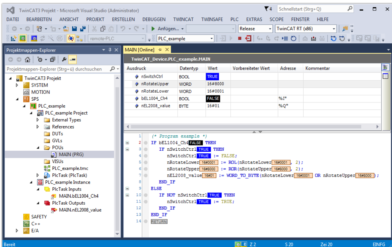
Abb. 83: TwinCAT 3 Entwicklungsumgebung (VS Shell): Logged-in, nach erfolgten Programmstart
