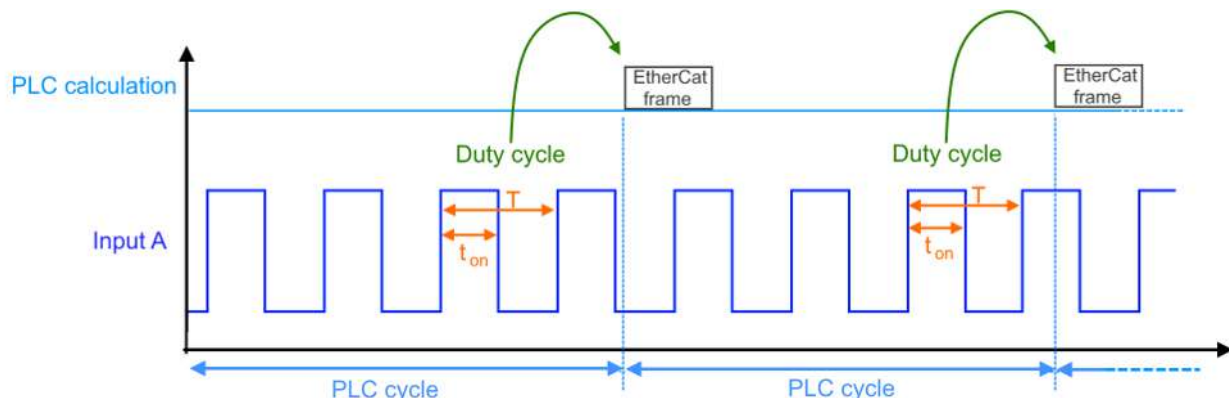
Abb. 171: Duty Cycle Messung
