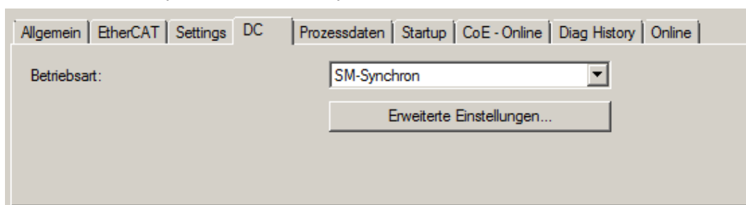
Abb. 141: Karteireiter „DC“ (Distributed Clocks)
