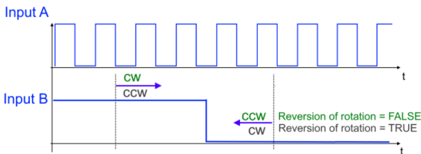
Abb. 178: Zählrichtungsumkehr (Index 0x80n0:0E „Reversion of rotation“) bei einem Zähler/Impulsgeber
