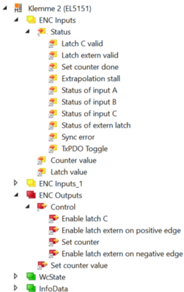
Abb. 148: Verknüpfte Ein- und Ausgänge der EL5112 mit der NC-Task
