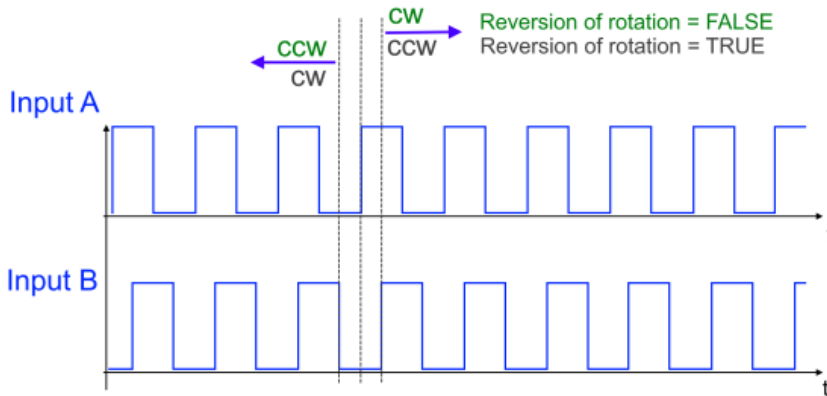
Abb. 177: Zählrichtungsumkehr (Index 0x80n0:0E „Reversion of rotation“) bei einem Encoder
