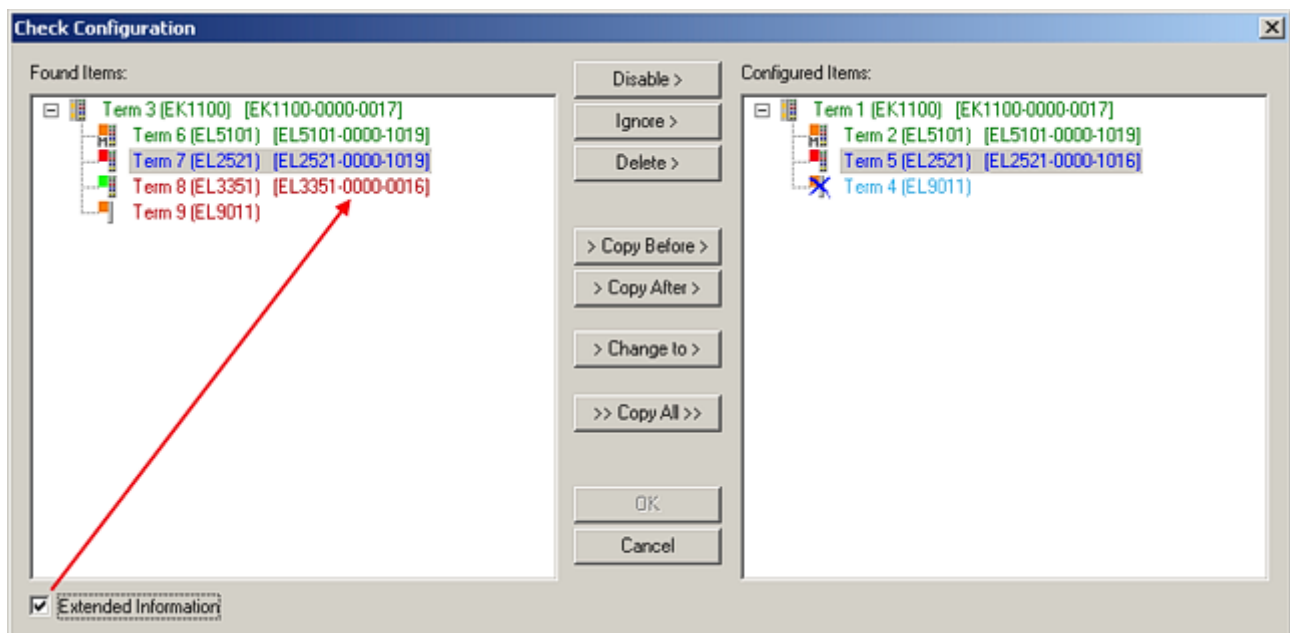
Abb. 127: Korrekturdialog
