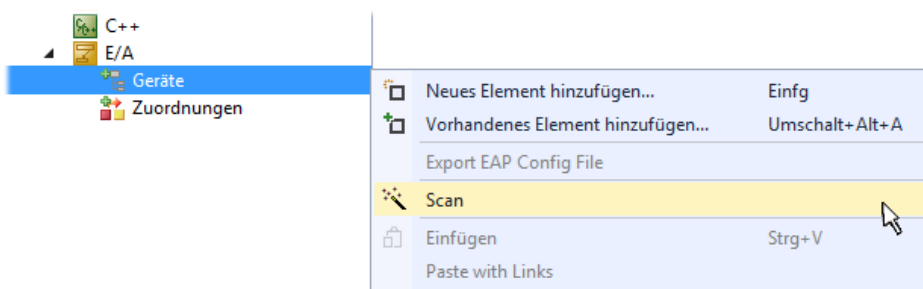
Abb. 66: Auswahl „Scan“
