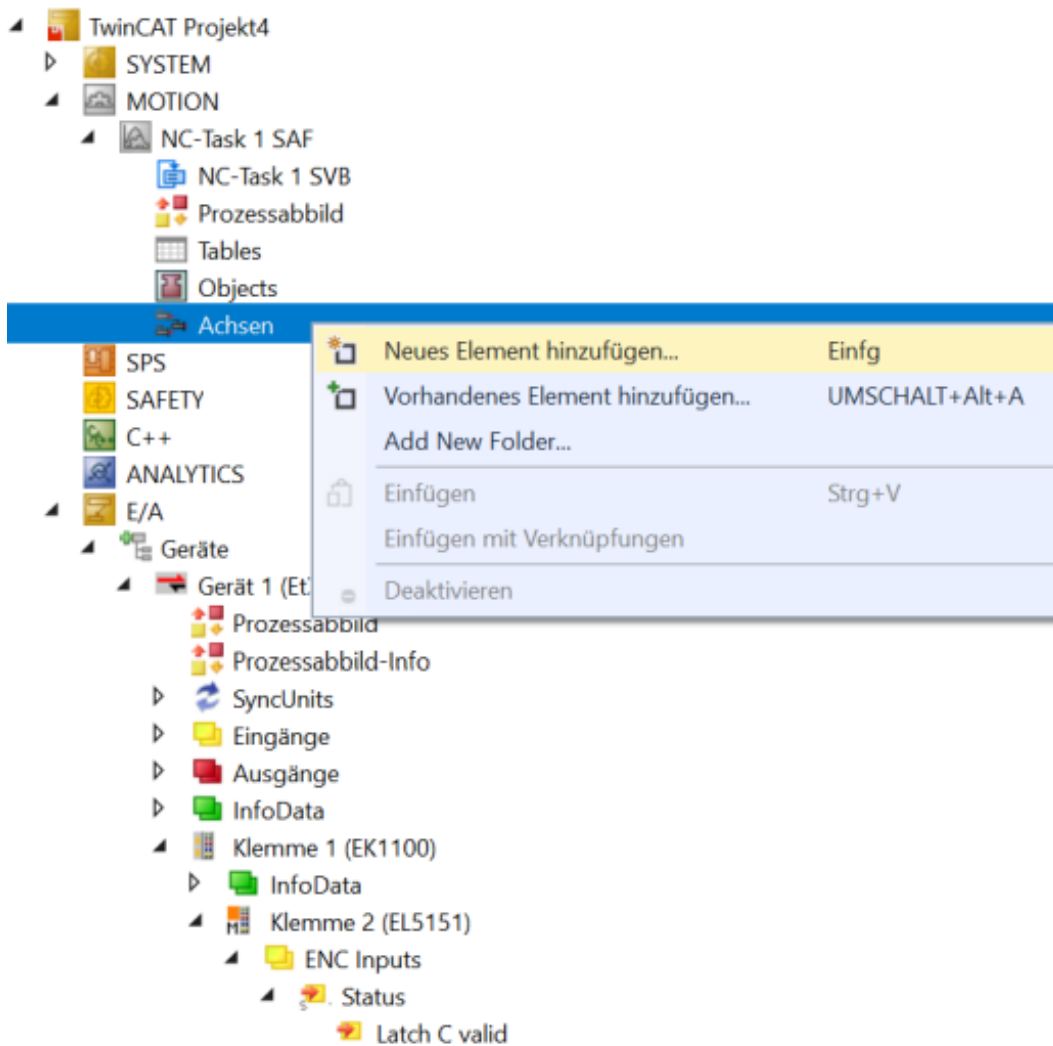
Abb. 144: Achse einfügen
