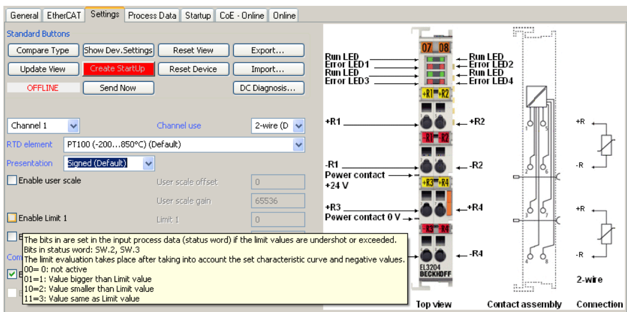
Abb. 152: Beispiel Inbetriebnahmehilfe für eine EL3204
