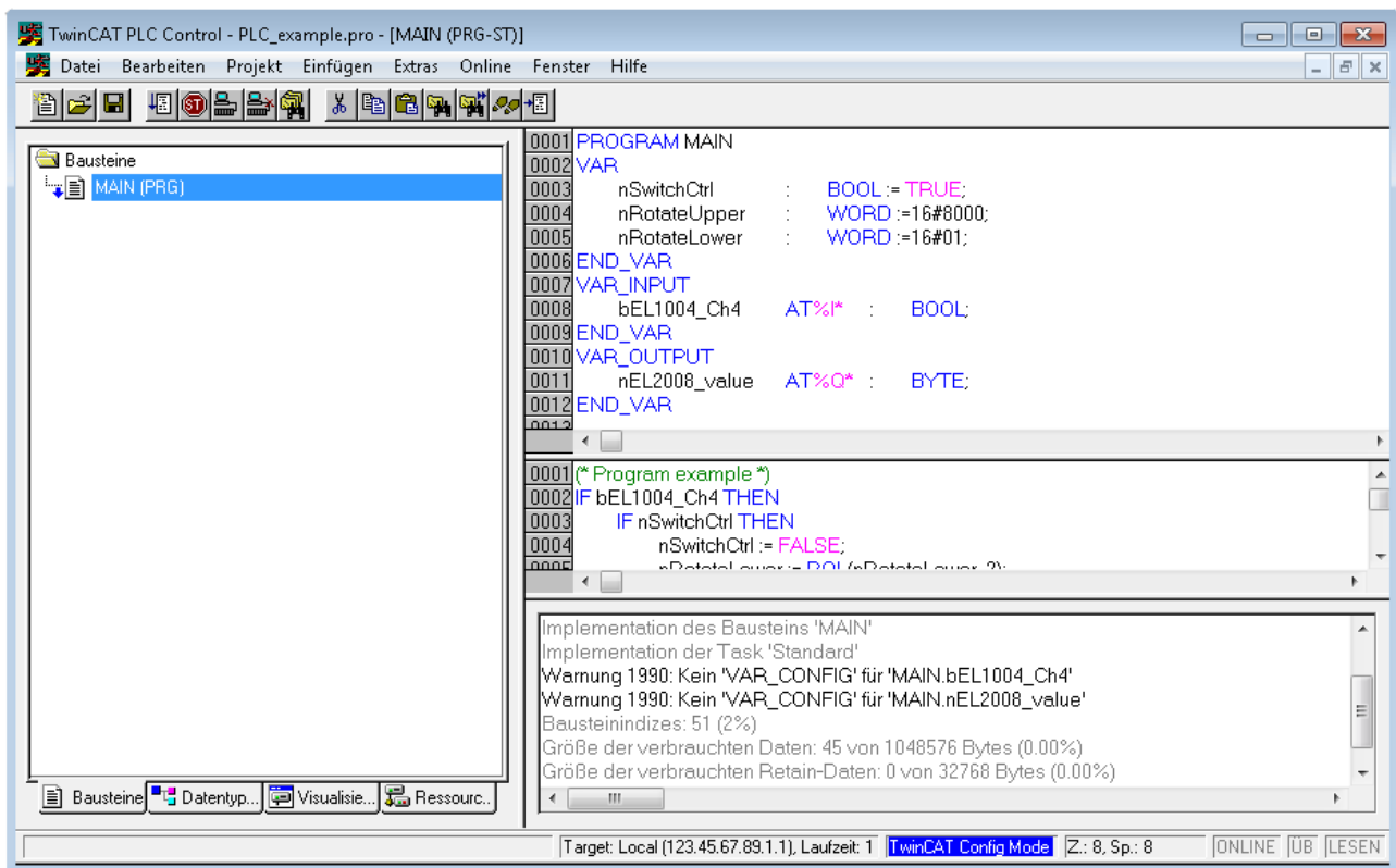
Abb. 52: Beispielprogramm mit Variablen nach einem Kompiliervorgang (ohne Variablenanbindung)
