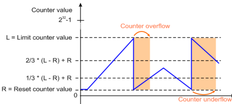
Abb. 176: Über- und Unterschreiten der Zählergrenzen mit festgelegtem Wertebereich
