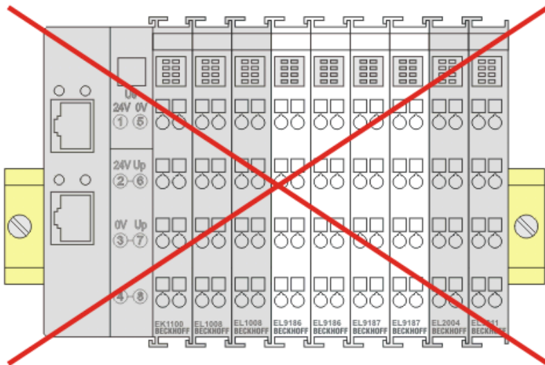
Abb. 26: Inkorrekte Positionierung
