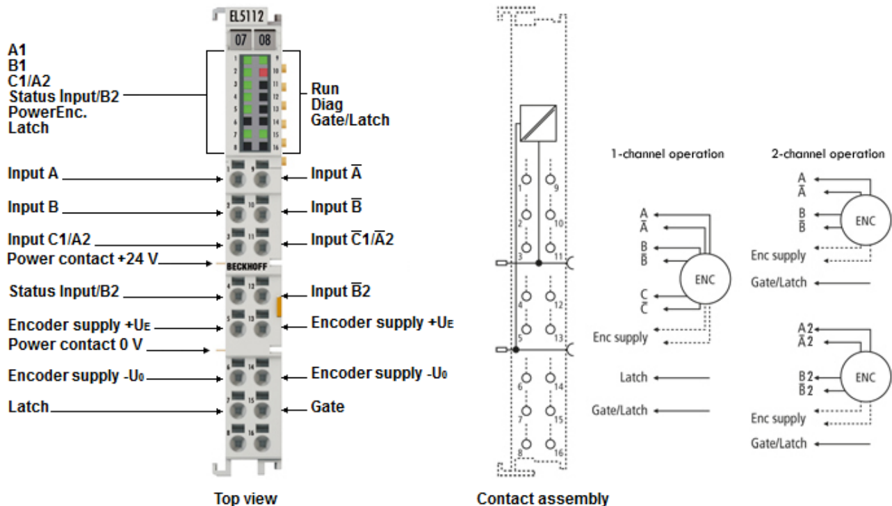
Abb. 27: EL5112 - Anschlussbelegung
