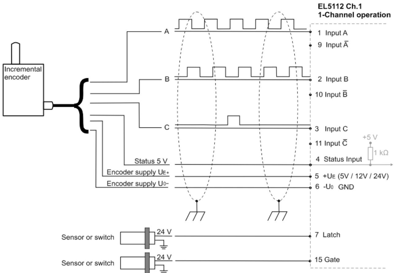
Abb. 30: Anschluss Encoder TTL - Mode mit Nullimpuls im 1-Kanal-Betrieb
