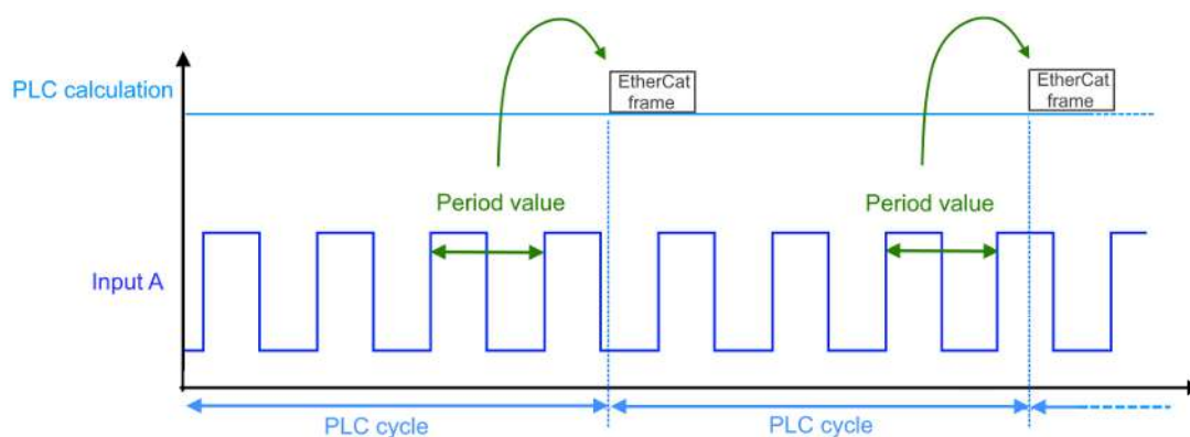
Abb. 181: Periodendauermessung
