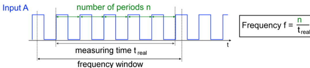
Abb. 179: Frequenzmessung - „Frequency value“
