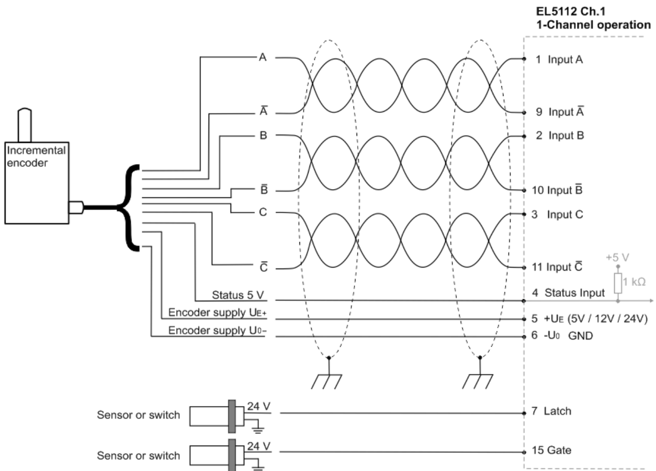
Abb. 28: Anschluss Encoder RS422 - Mode mit Nullimpuls im 1-Kanal-Betrieb
