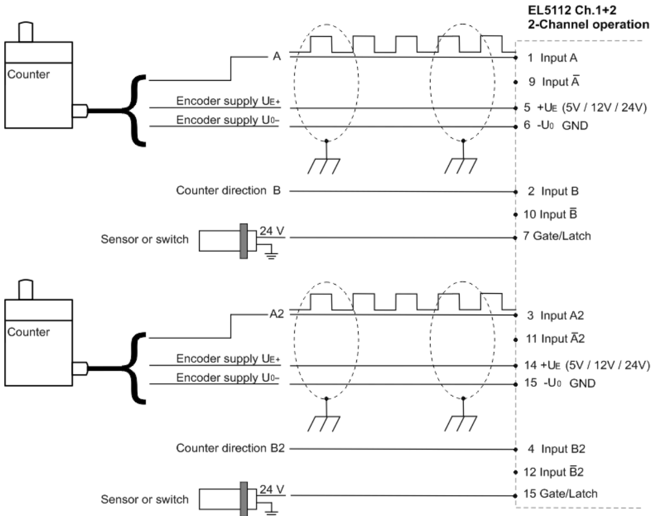
Abb. 37: Anschluss Zähler / Impulsgeber TTL - Mode ohne Nullimpuls im 2-Kanal Betrieb
