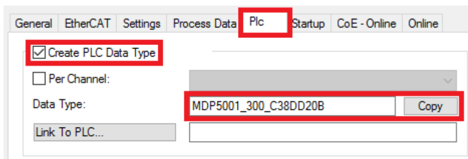
Abb. 79: Erzeugen eines SPS Datentyps
