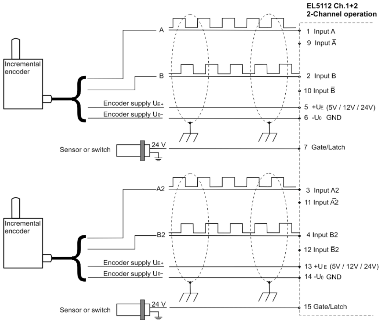
Abb. 36: Anschluss Encoder TTL - Mode ohne Nullimpuls im 2-Kanal Betrieb
