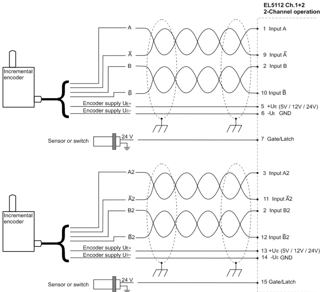
Abb. 34: Anschluss Encoder RS422 - Mode ohne Nullimpuls im 2-Kanal-Betrieb
