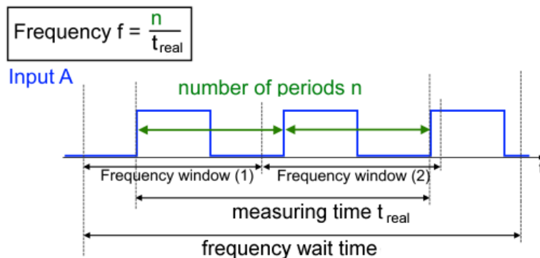
Abb. 168: Frequenzmessung außerhalb des Frequenzfensters mit Wartezeit
