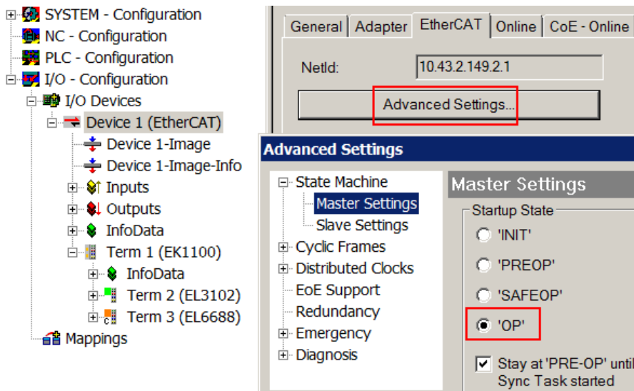
Abb. 153: Default Verhalten System Manager
