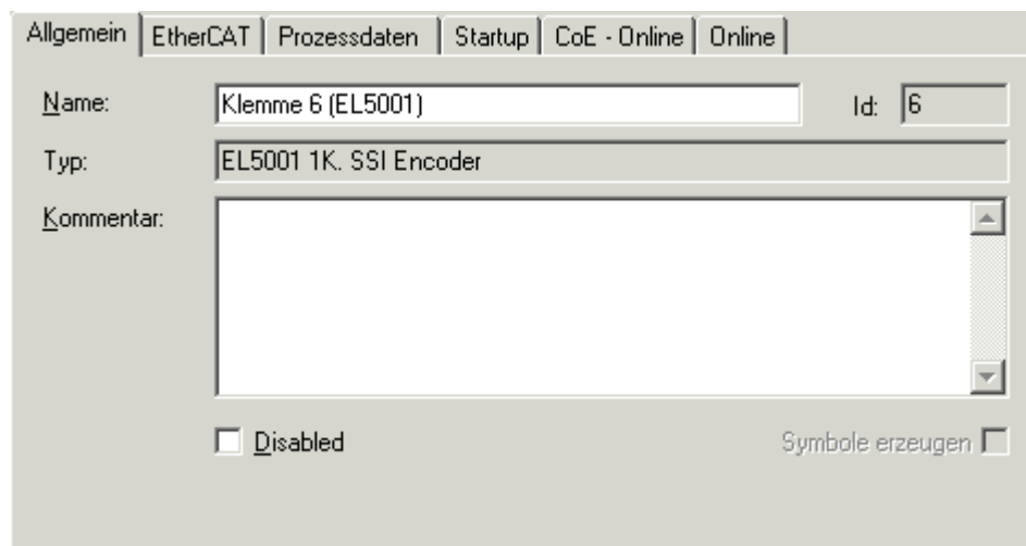
Abb. 133: Karteireiter „Allgemein“
