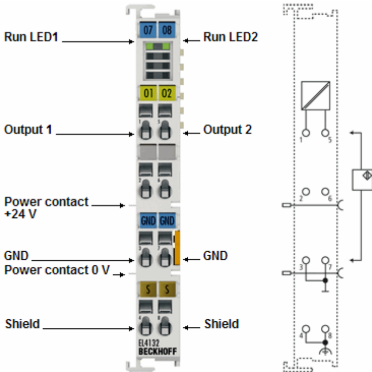
Abb. 16: EL4132
