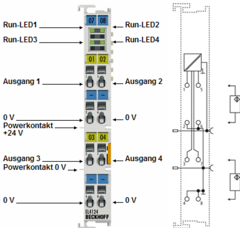
Abb. 15: LED und Anschlussbelegung EL4124
