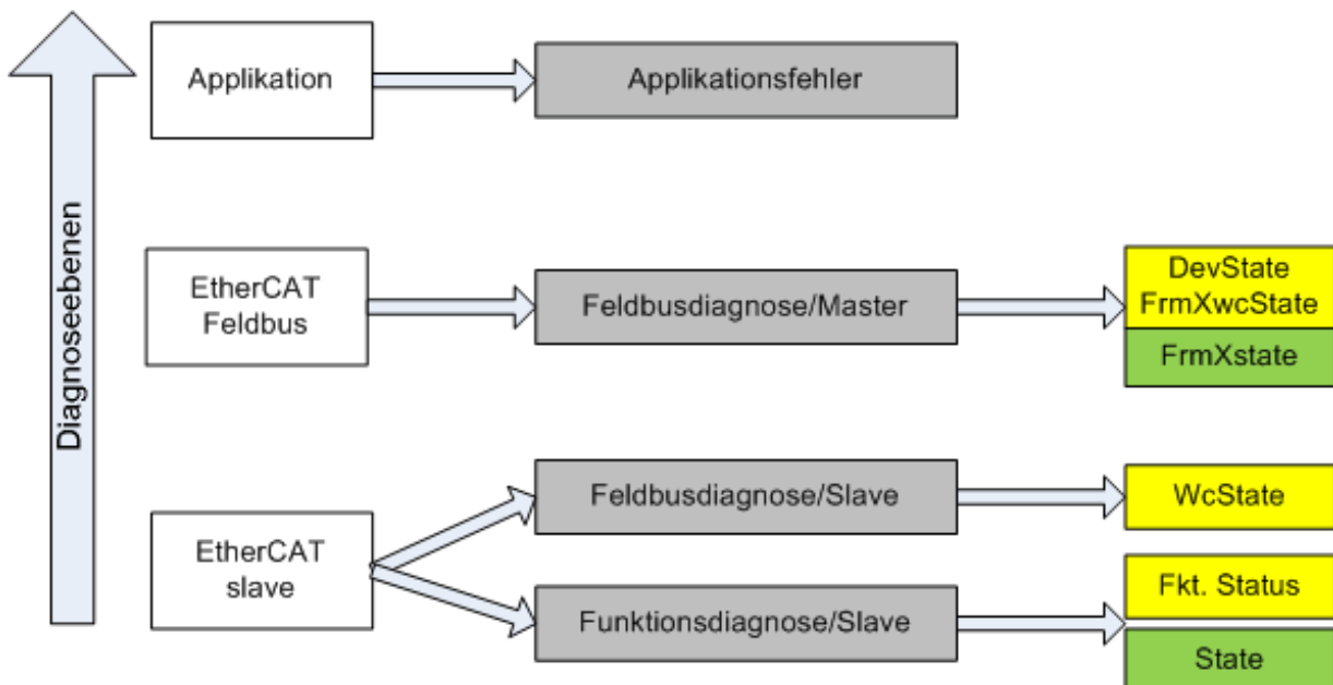
Abb. 140: Auswahl an Diagnoseinformationen eines EtherCAT Slave
