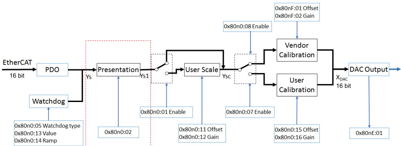
Abb. 154: Blockschaltbild zur Bestimmung der Ausgabewerte mit Default-Einstellungen (Funktion Darstellung)
