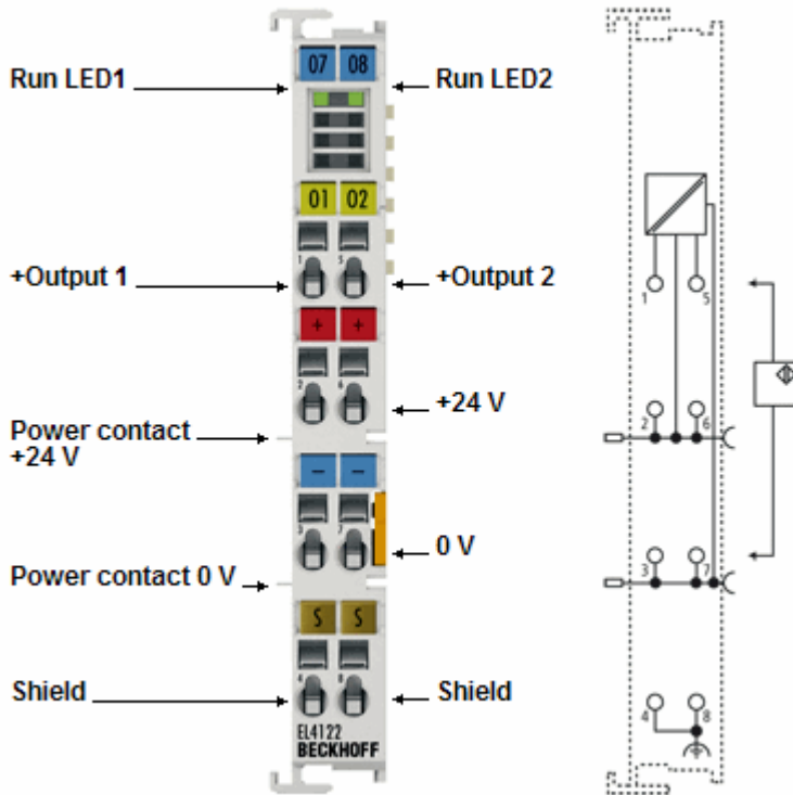
Abb. 13: LED und Anschlussbelegung EL4122
