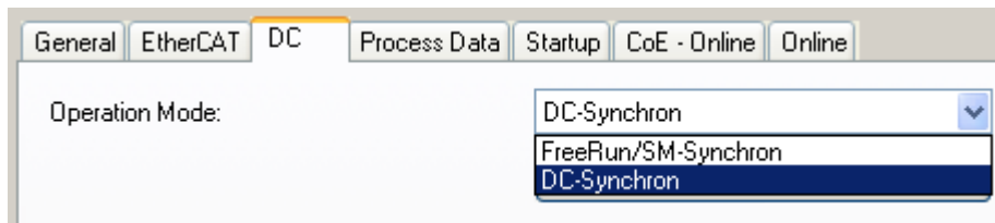
Abb. 158: Umstellung EL41x4 auf DC-Betrieb
