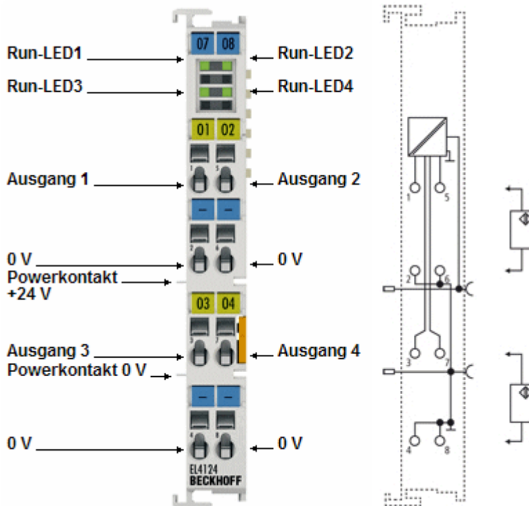
Abb. 14: EL4124
