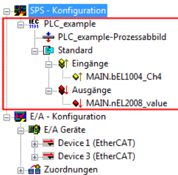
Abb. 52: Eingebundenes PLC-Projekt in der SPS-Konfiguration des System Managers
