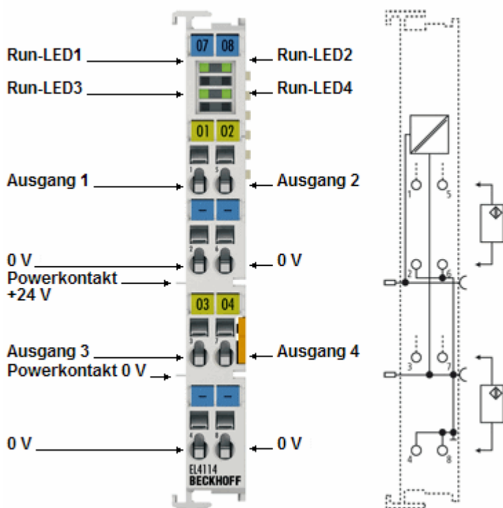
Abb. 11: LED und Anschlussbelegung EL4114-xxxx
