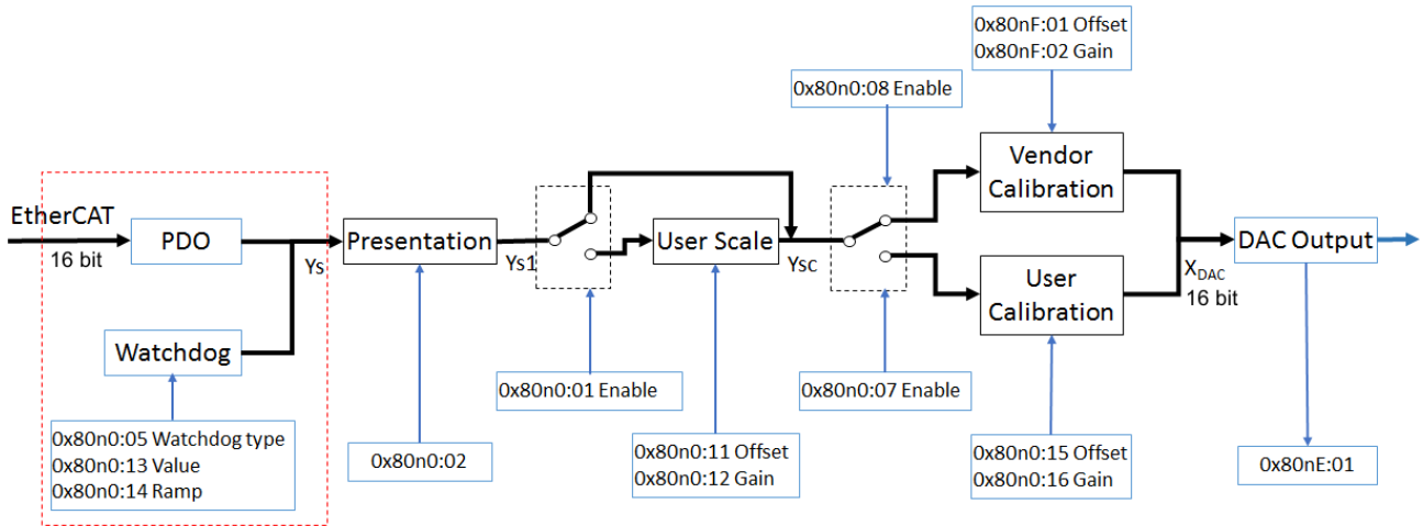
Abb. 152: Blockschaltbild zur Bestimmung der Ausgabewerte in Default-Einstellung (Funktion Watchdog)
