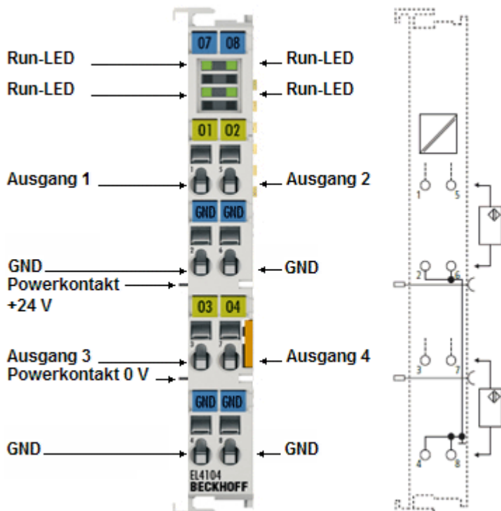
Abb. 7: LED und Anschlussbelegung EL4104
