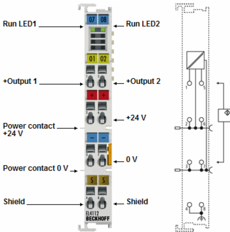
Abb. 9: LED und Anschlussbelegung EL4112-00xx
