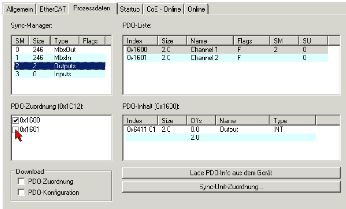
Abb. 163: Ausgangskanal ein- und ausschalten
