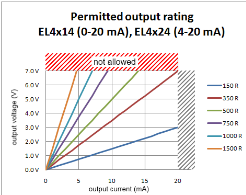
Abb. 160: Zulässiger Betriebsbereich für EL4xx4 Stromausgänge
