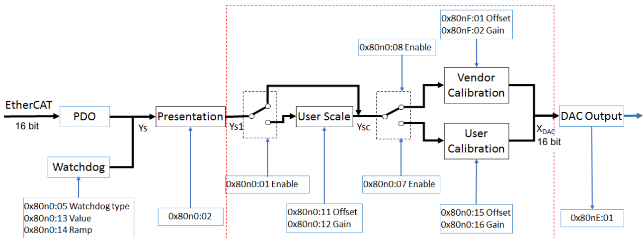
Abb. 155: Blockschaltbild zur Bestimmung der Ausgabewerte in Default-Einstellung (Funktion Gain/Offset)
