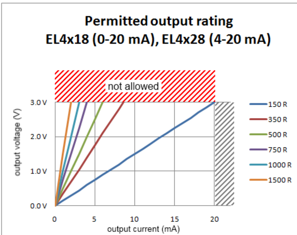
Abb. 161: Zulässiger Betriebsbereich für EL4xx8 Stromausgänge
