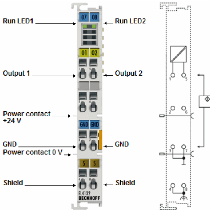
Abb. 17: LED und Anschlussbelegung EL4132
