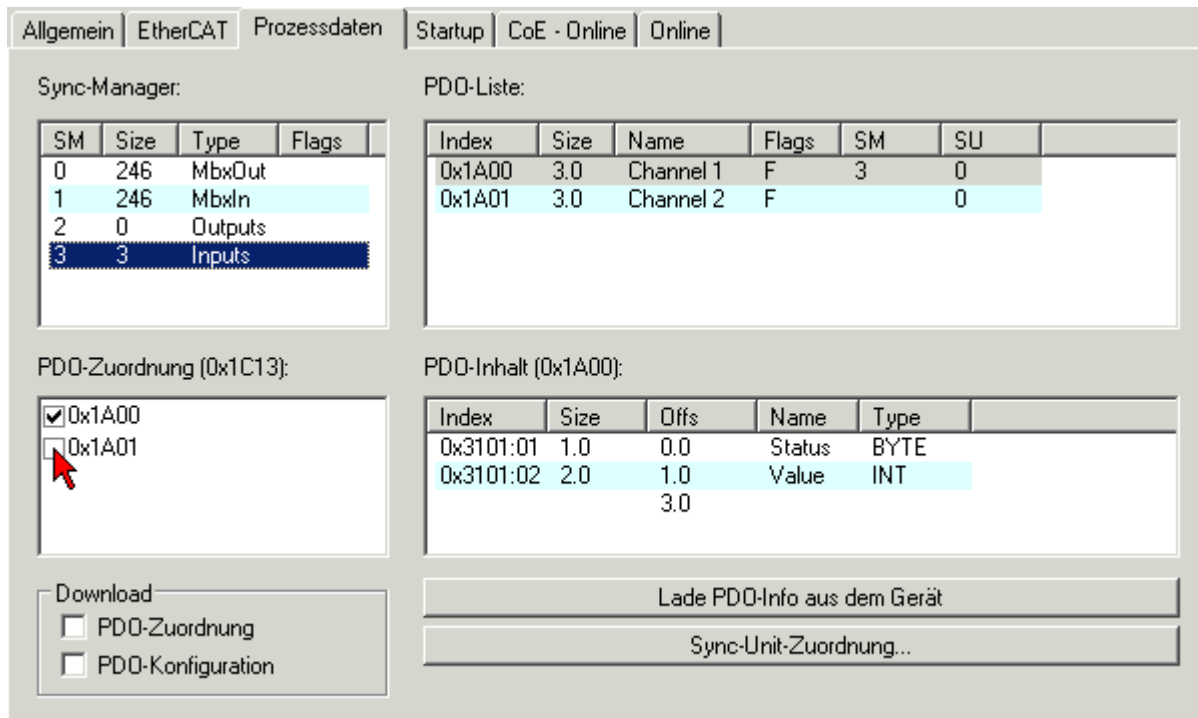
Abb. 162: Eingangskanal ein- und ausschalten
