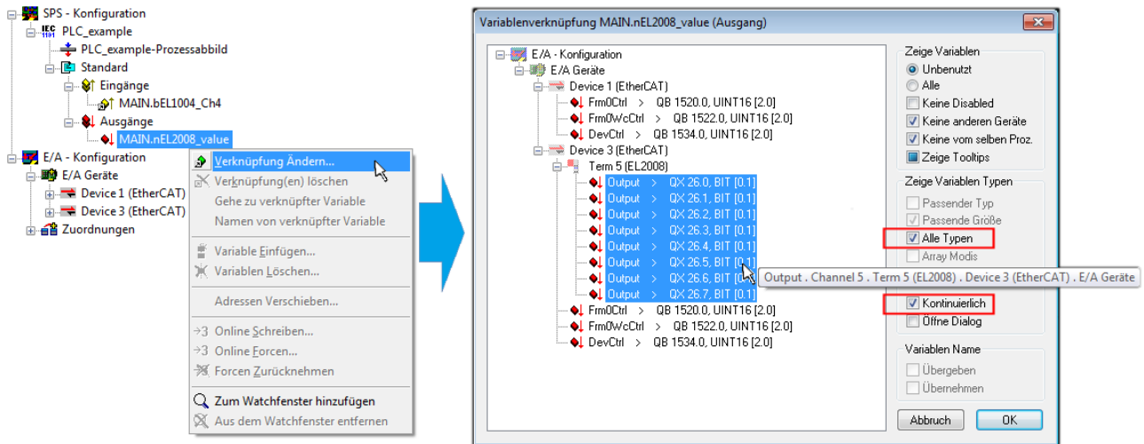
Abb. 55: Auswahl von mehreren PDO gleichzeitig: Aktivierung von „Kontinuierlich“ und „Alle Typen“
