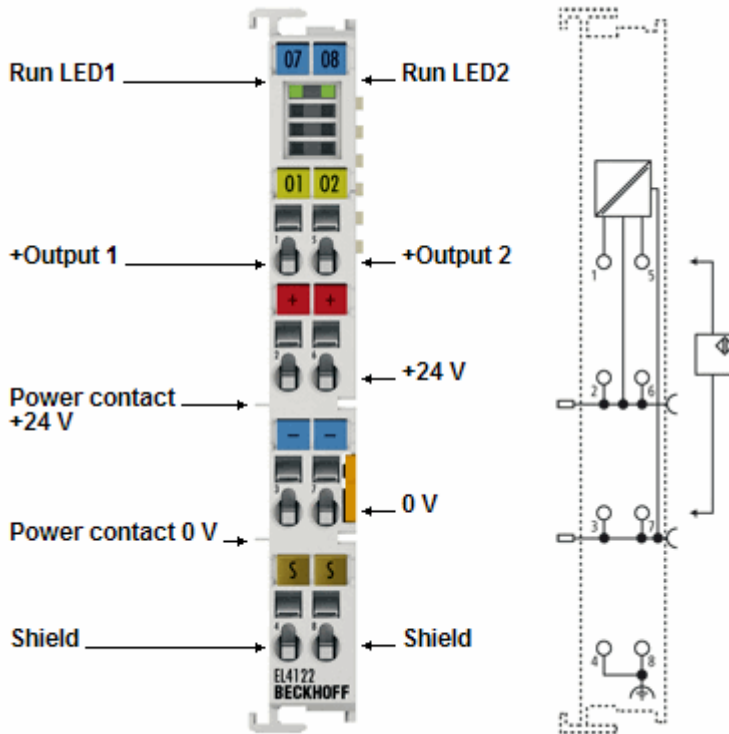
Abb. 12: EL4122
