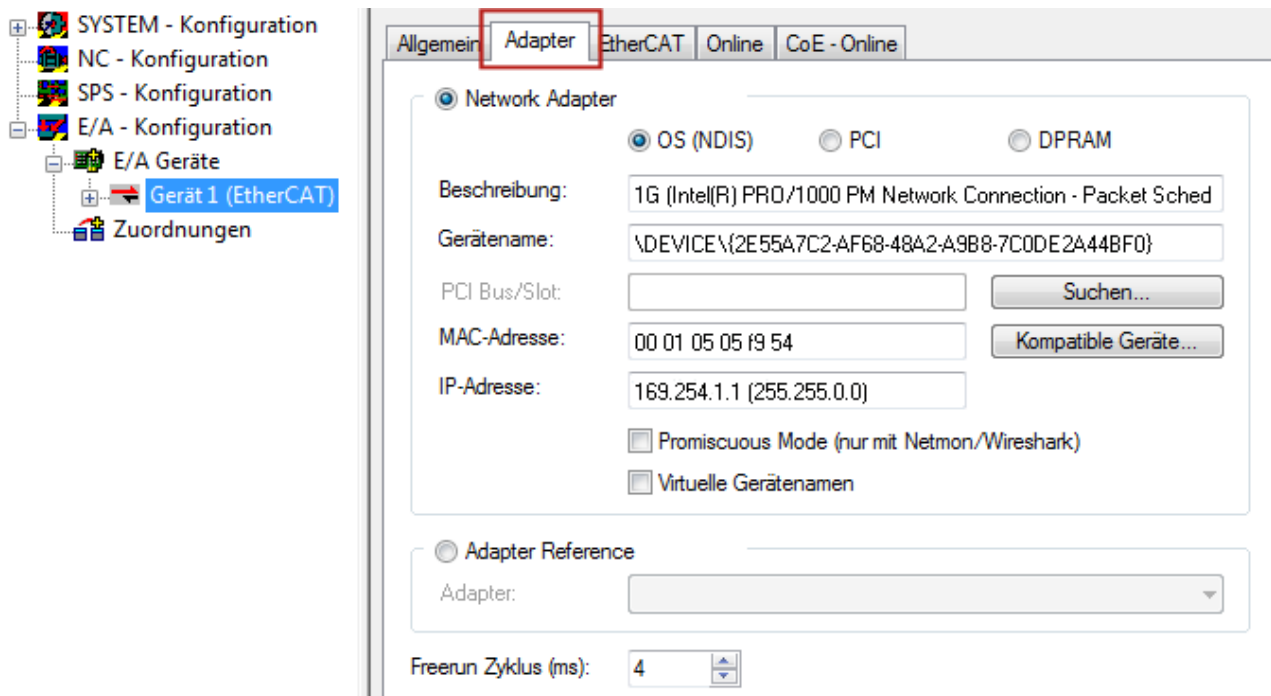
Abb. 102: Eigenschaften EtherCAT-Gerät (TwinCAT 2)
