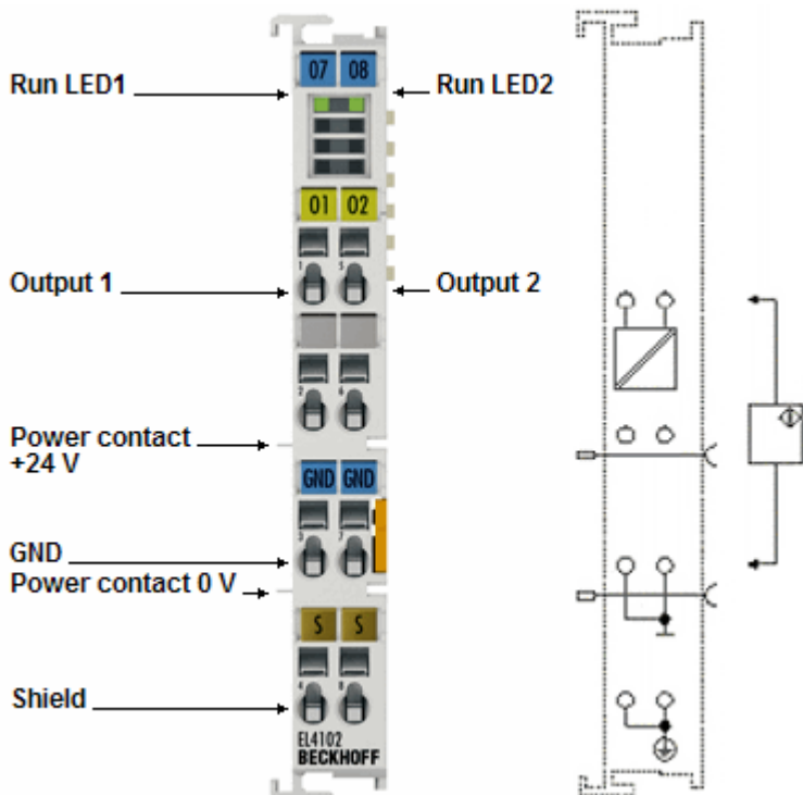
Abb. 5: LED und Anschlussbelegung EL4102
