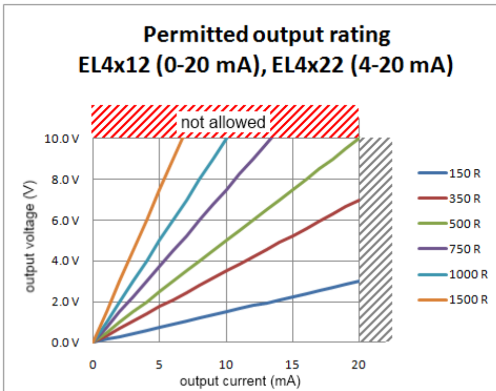
Abb. 159: Zulässiger Betriebsbereich für EL4xx2 Stromausgänge
