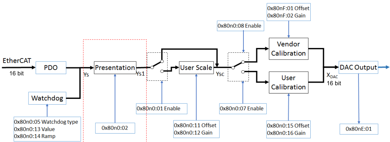
Abb. 150: Blockschaltbild zur Bestimmung der Ausgabewerte mit Default-Einstellungen (Funktion Darstellung)
