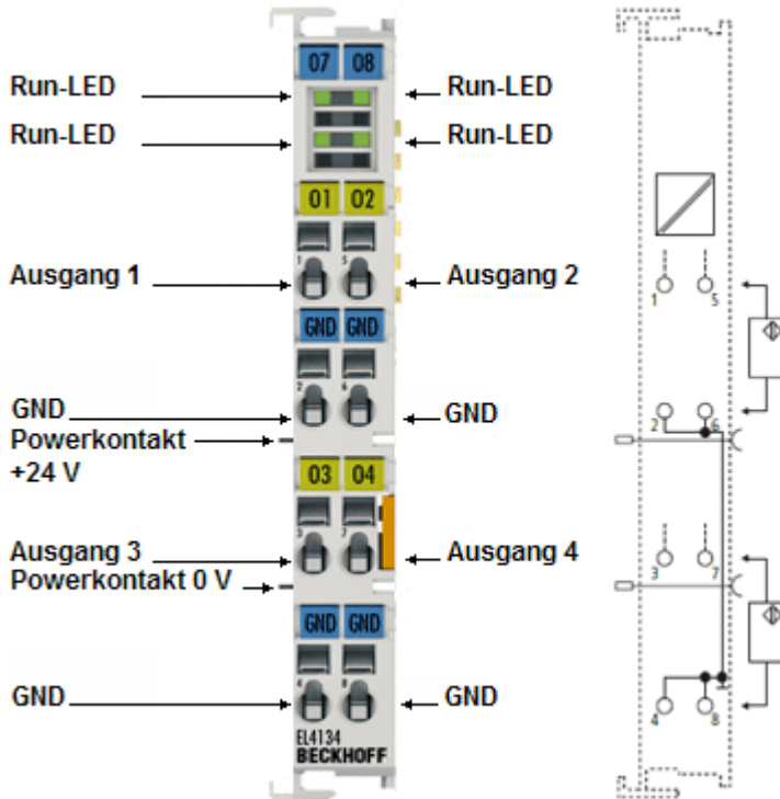
Abb. 19: LED und Anschlussbelegung EL4134-00xx
