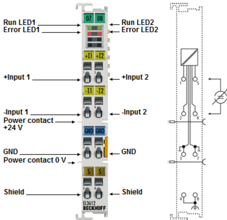
Abb. 5: EL3612
