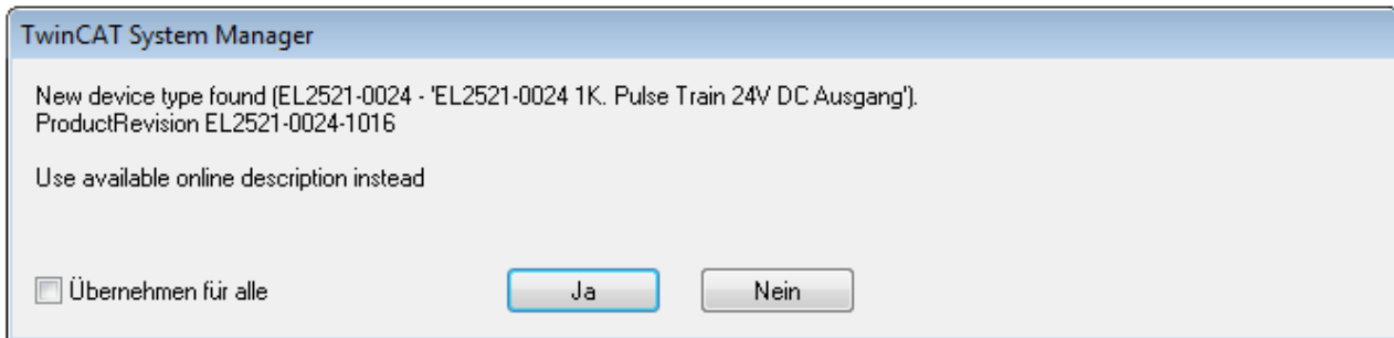
Abb. 90: Hinweisfenster OnlineDescription (TwinCAT 2)
