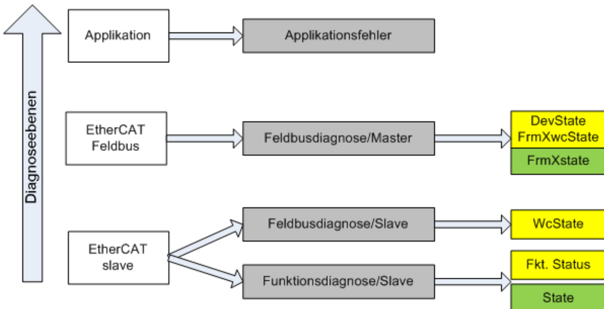
Abb. 138: Auswahl an Diagnoseinformationen eines EtherCAT Slave
