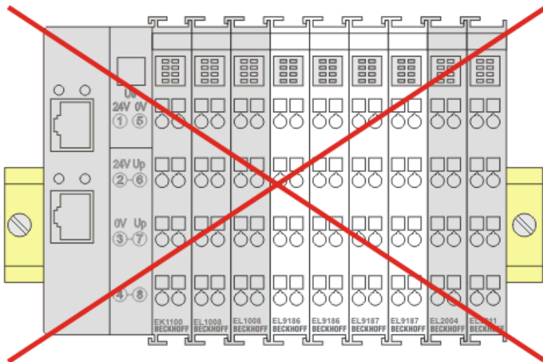
Abb. 26: Inkorrekte Positionierung
