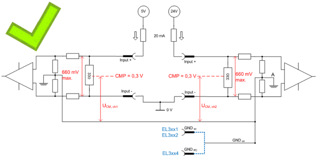
Abb. 34: Beispiel 1: LowSide-Messung
