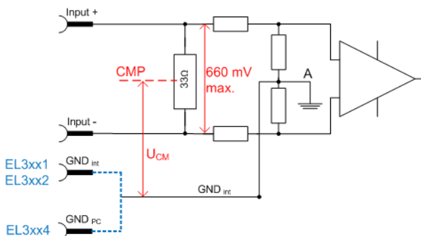
Abb. 32: Interne Anschlussschaltung 0/4...20 mA Eingänge
