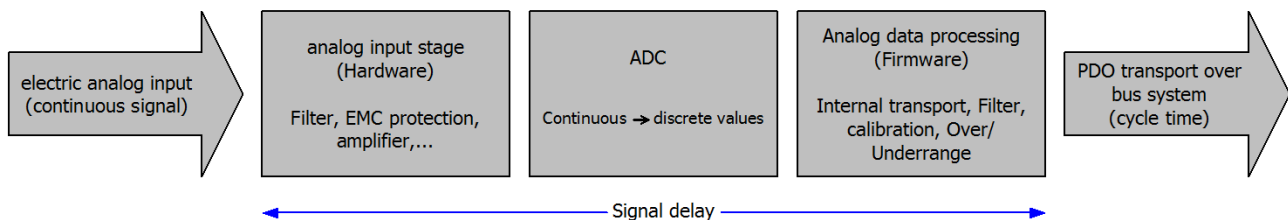
Abb. 155: Signalverarbeitung Analogeingang
