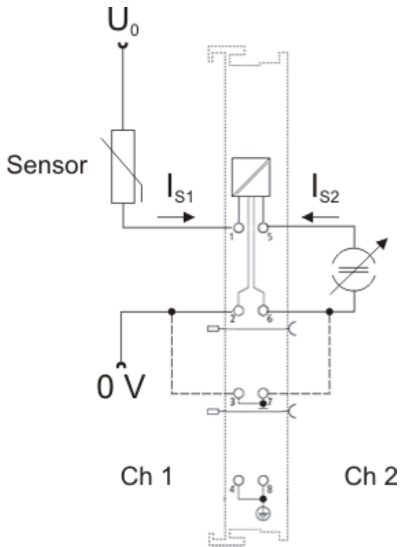
Abb. 31: Variable Stromquelle (Ersatzschaltbild Kanal 2)
