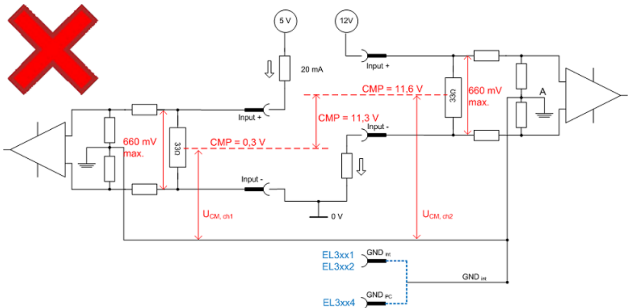
Abb. 36: Beispiel 2, High-Side-/Low-Side-Messung
