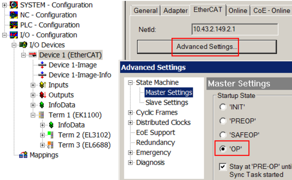
Abb. 142: Default Verhalten System Manager
