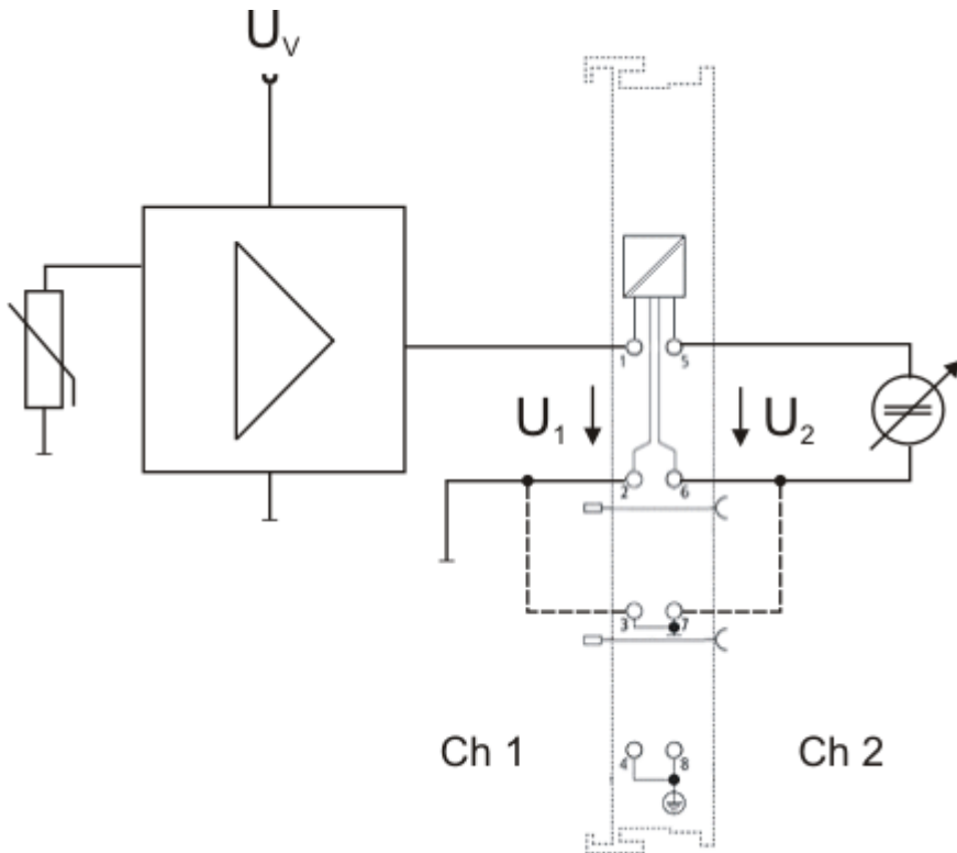
Abb. 30: Variable Spannungsquelle (Ersatzschaltbild Kanal 2)
