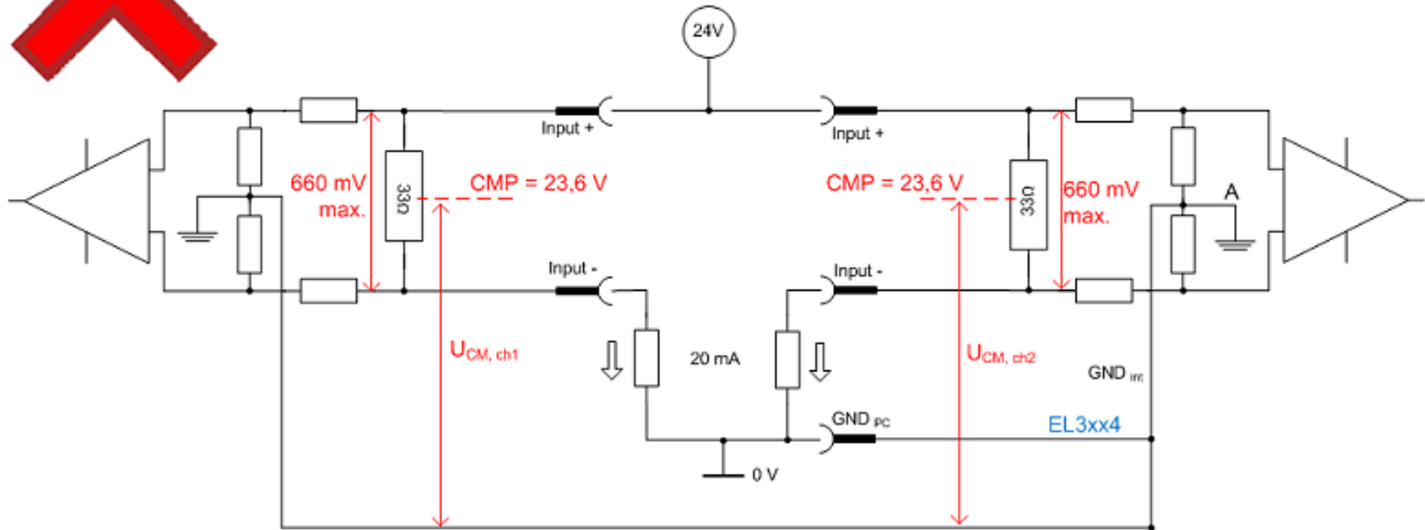
Abb. 37: Unzulässige EL3xx4-Beschaltung
