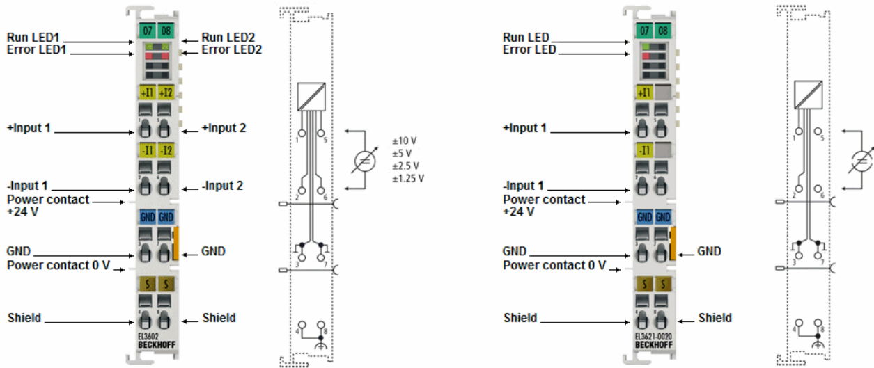
Abb. 28: Anschlussbelegung am Beispiel EL3602 (2 Kanal)/ EL3621-0020 (1 Kanal)
