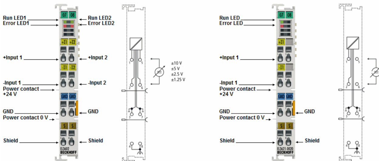
Abb. 27: LEDs am Beispiel EL3602 (2 Kanal)/ EL3621-0020 (1 Kanal)
