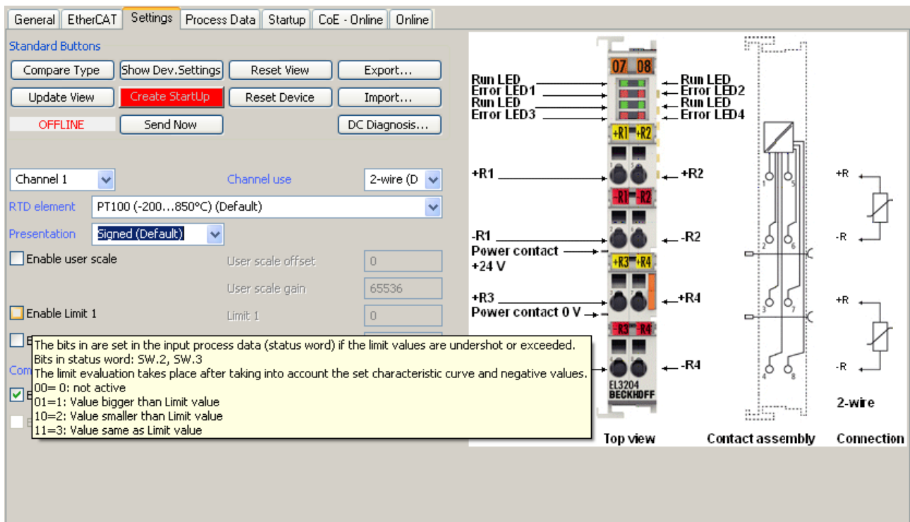
Abb. 141: Beispiel Inbetriebnahmehilfe für eine EL3204
