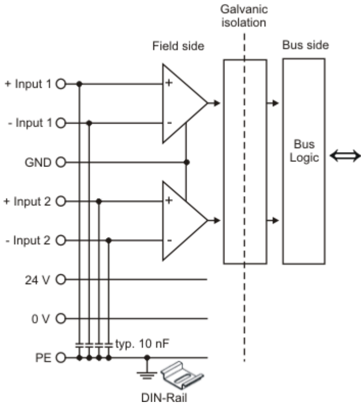
Abb. 29: Galvanische Isolierung der Eingänge
