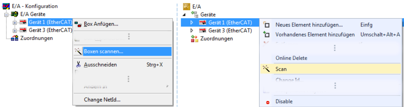
Abb. 115: Manuelles Auslösen des Teilnehmer-Scans auf festgelegtem EtherCAT Device (links: TwinCAT 2; rechts TwinCAT 3)
