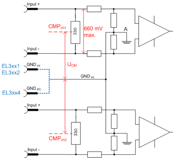
Abb. 33: Interne Anschlussschaltung 0/4...20 mA Eingänge einer EL3xx2
