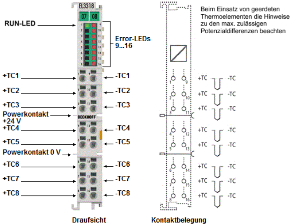
Abb. 77: EL3318
