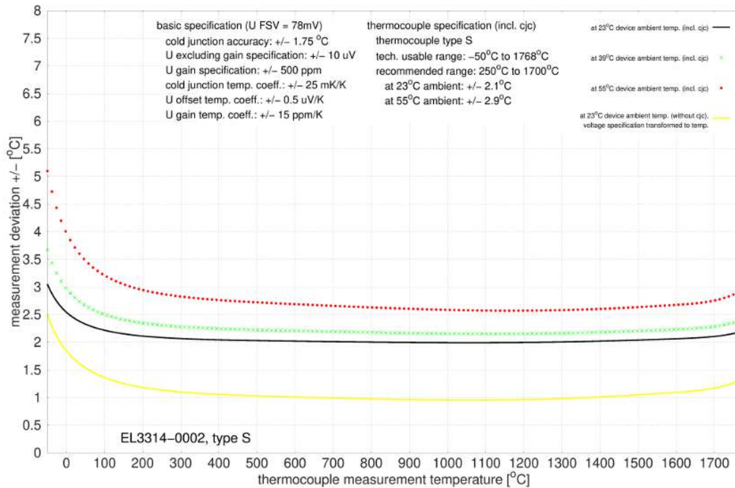
Abb. 73: EL3314-0002 und EL3314-0092 (entspricht EL3314-0002), Typ S
