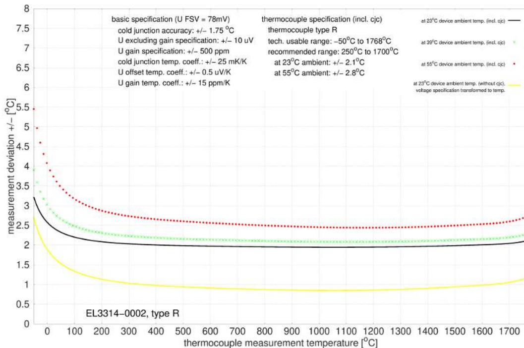
Abb. 18: EL3314-0002 und EL3314-0092 (entspricht EL3314-0002), Typ R
