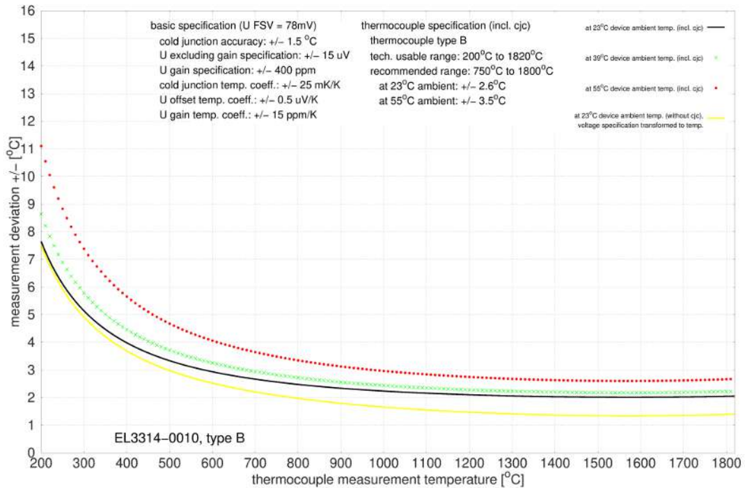
Abb. 37: EL3314-0010, EL3314-0020 und EL3314-0030 (entsprechen EL3314-0010), Typ B
