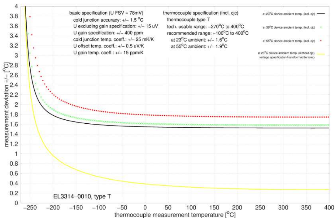
Abb. 59: EL3314-0010, EL3314-0020 und EL3314-0030 (entsprechen EL3314-0010), Typ T
