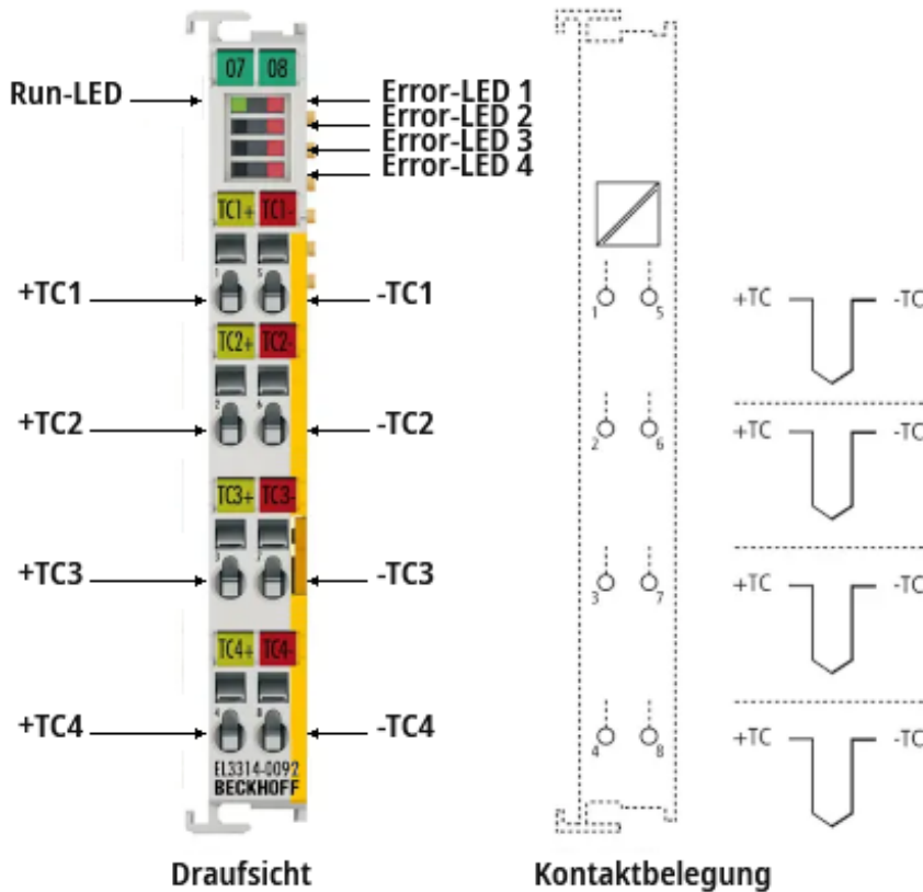
Abb. 64: EL3314-0092
