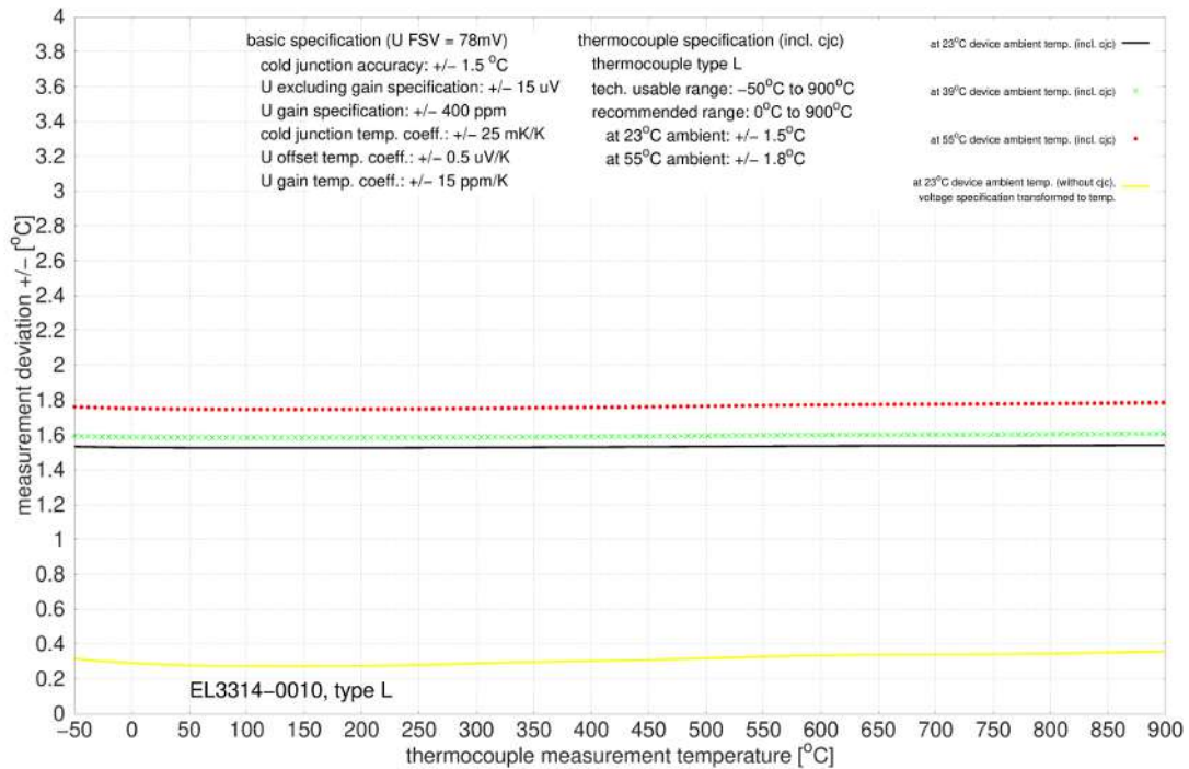
Abb. 29: EL3314-0010, EL3314-0020 und EL3314-0030 (entsprechen EL3314-0010), Typ L
