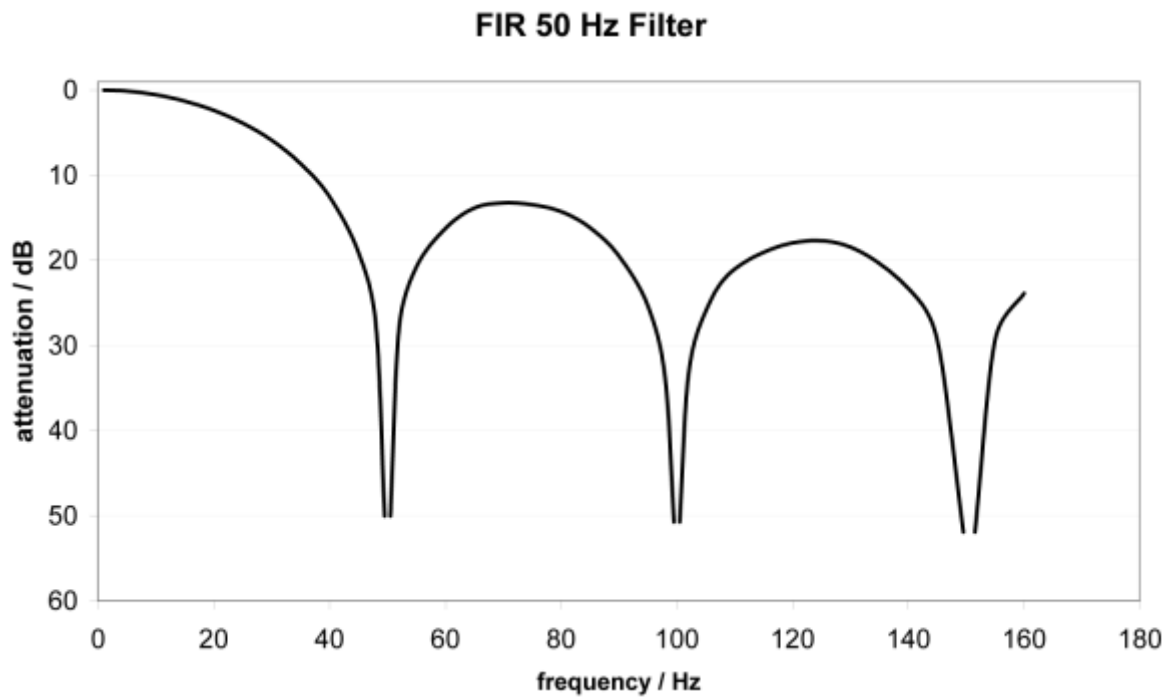
Abb. 225: Beispiel Notchfilter/Kerbfilter
