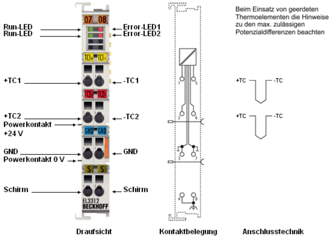
Abb. 7: EL3312
