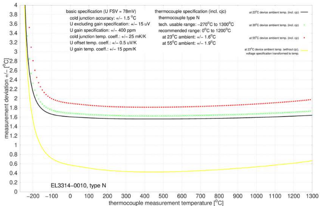
Abb. 43: EL3314-0010, EL3314-0020 und EL3314-0030 (entsprechen EL3314-0010), Typ N
