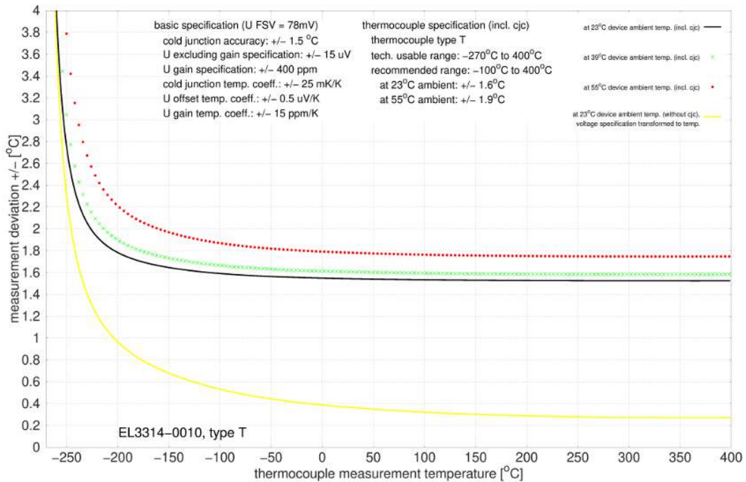
Abb. 33: EL3314-0010, EL3314-0020 und EL3314-0030 (entsprechen EL3314-0010), Typ T
