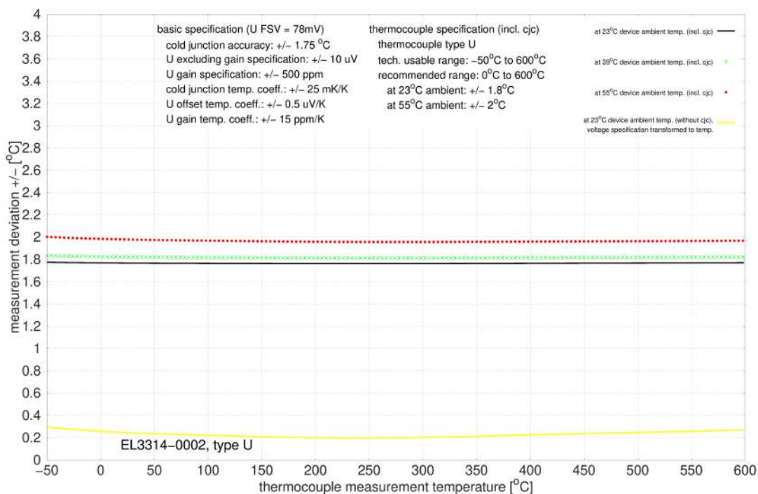
Abb. 75: EL3314-0002 und EL3314-0092 (entspricht EL3314-0002), Typ U
