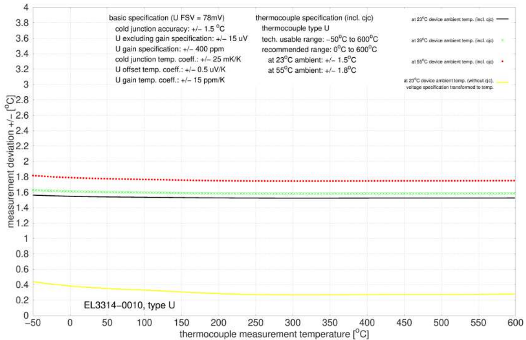
Abb. 47: EL3314-0010, EL3314-0020 und EL3314-0030 (entsprechen EL3314-0010), Typ U
