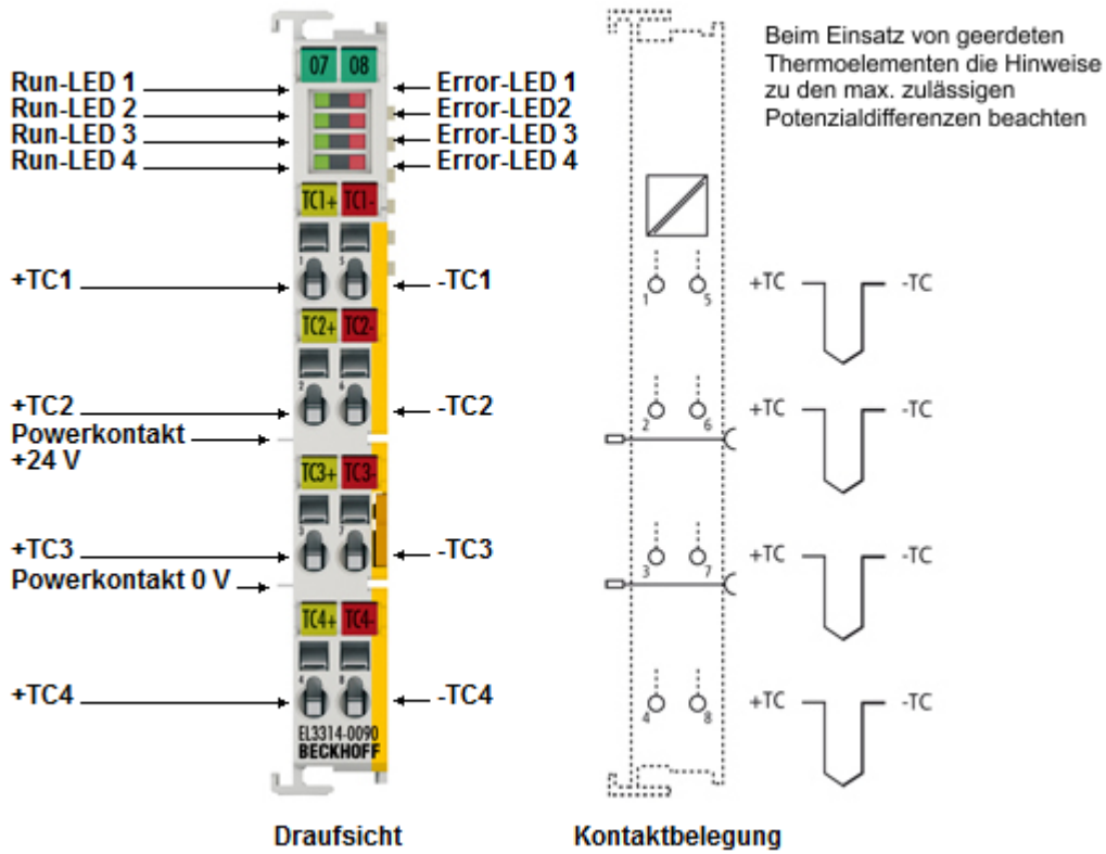
Abb. 63: EL3314-0090
