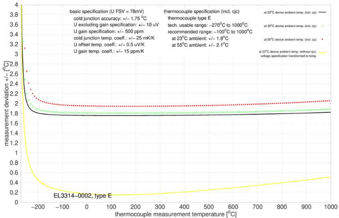
Abb. 13: EL3314-0002 und EL3314-0092 (entspricht EL3314-0002), Typ E
