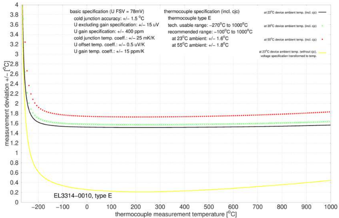
Abb. 39: EL3314-0010, EL3314-0020 und EL3314-0030 (entsprechen EL3314-0010), Typ E
