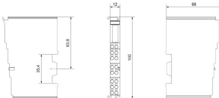
Abb. 78: Technische Zeichnung | Gehäuse EL-12-16pin
