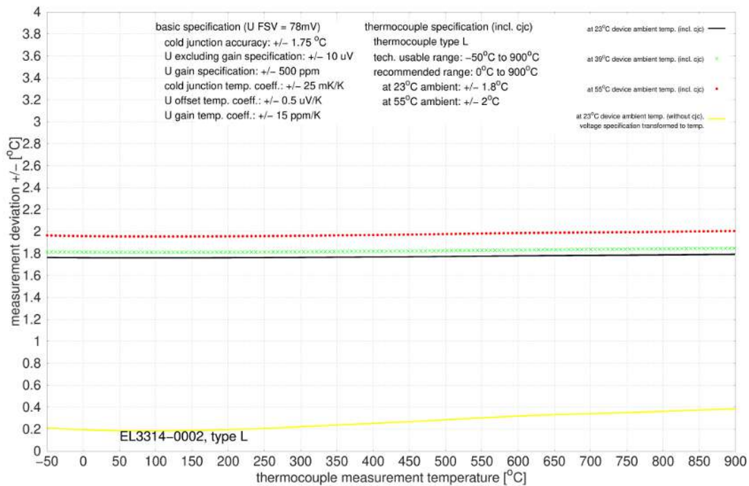
Abb. 70: EL3314-0002 und EL3314-0092 (entspricht EL3314-0002), Typ L
