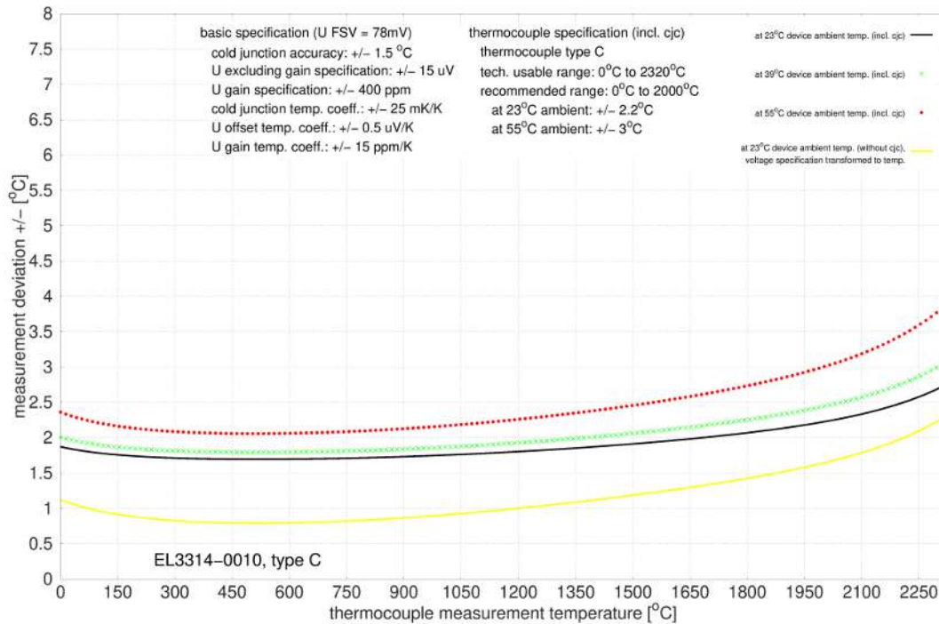
Abb. 51: EL3314-0010, EL3314-0020 und EL3314-0030 (entsprechen EL3314-0010), Typ C
