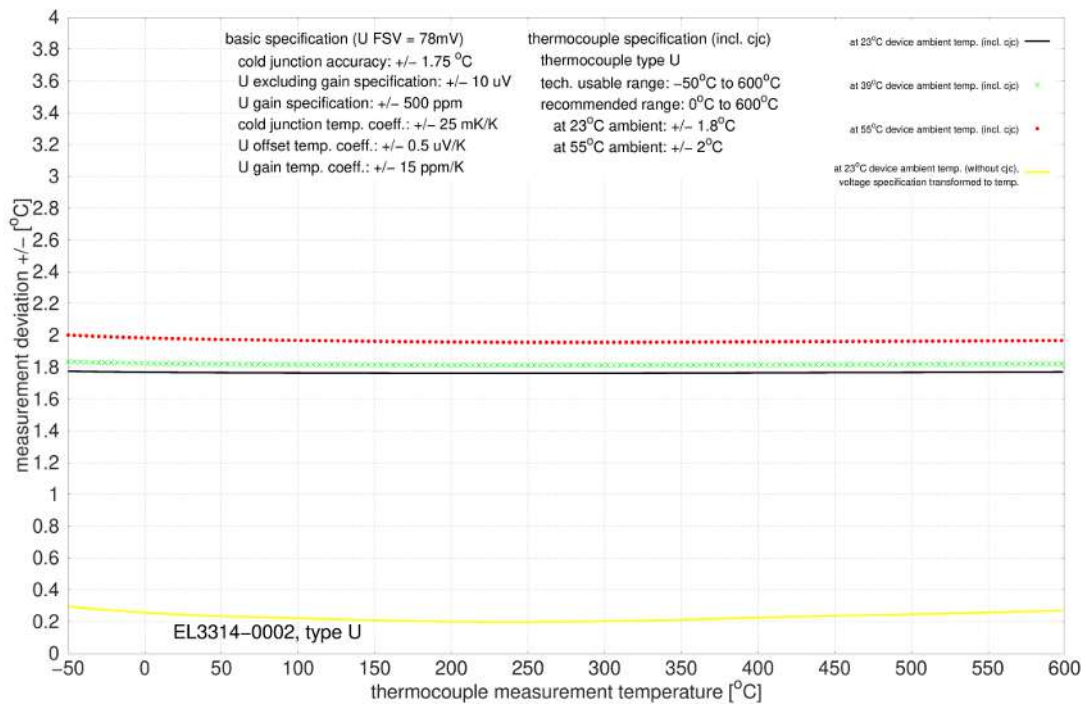
Abb. 21: EL3314-0002 und EL3314-0092 (entspricht EL3314-0002), Typ U
