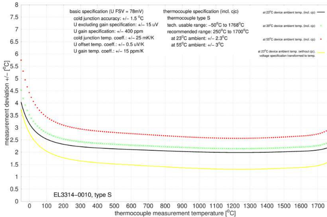
Abb. 45: EL3314-0010, EL3314-0020 und EL3314-0030 (entsprechen EL3314-0010), Typ S
