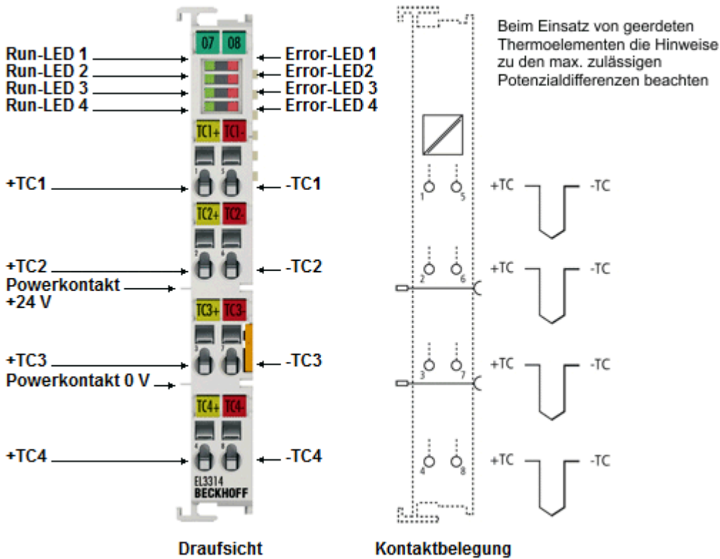
Abb. 9: EL3314
