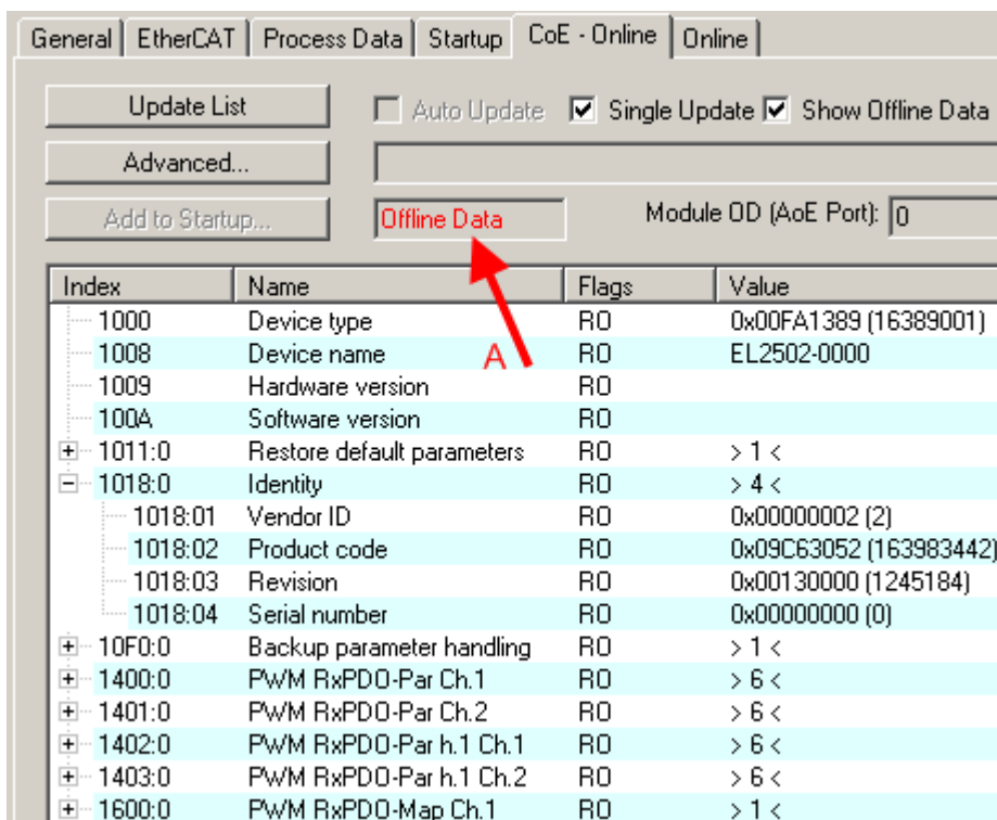
Abb. 87: Offline-Verzeichnis
