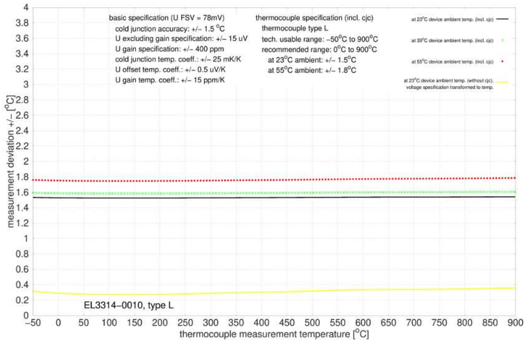
Abb. 42: EL3314-0010, EL3314-0020 und EL3314-0030 (entsprechen EL3314-0010), Typ L
