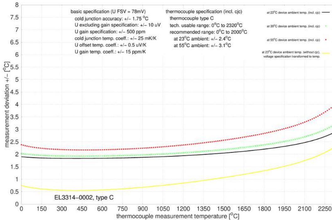
Abb. 12: EL3314-0002 und EL3314-0092 (entspricht EL3314-0002), Typ C
