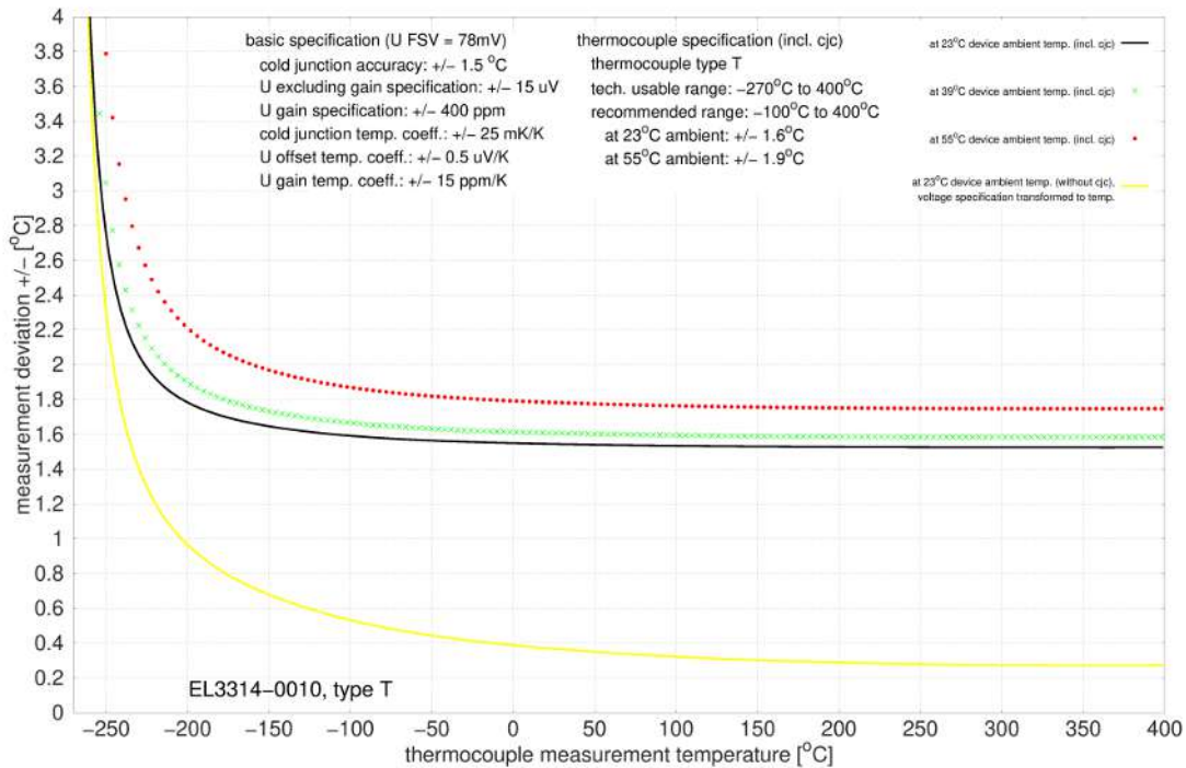
Abb. 46: EL3314-0010, EL3314-0020 und EL3314-0030 (entsprechen EL3314-0010), Typ T
