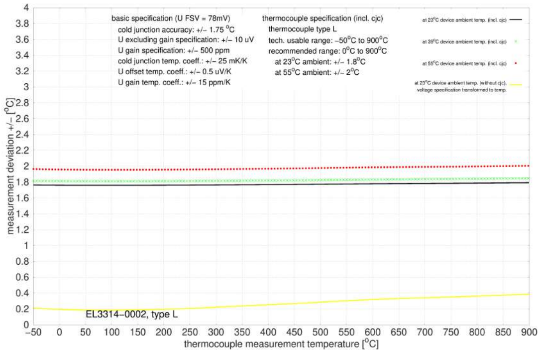
Abb. 16: EL3314-0002 und EL3314-0092 (entspricht EL3314-0002), Typ L
