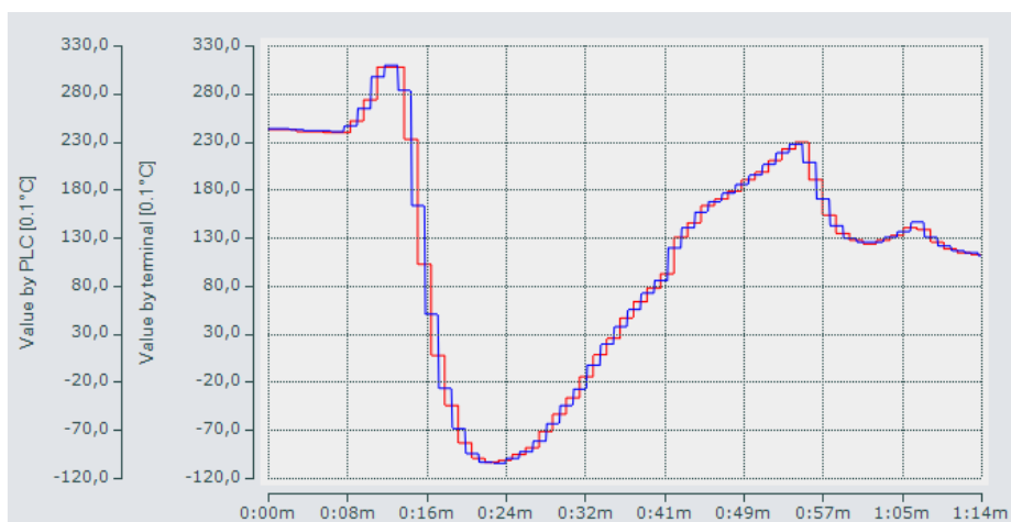
Abb. 240: Blau: Temperaturwerte aus der PLC-Berechnung; Rot: PDO-Werte im Temperaturmessbereich
