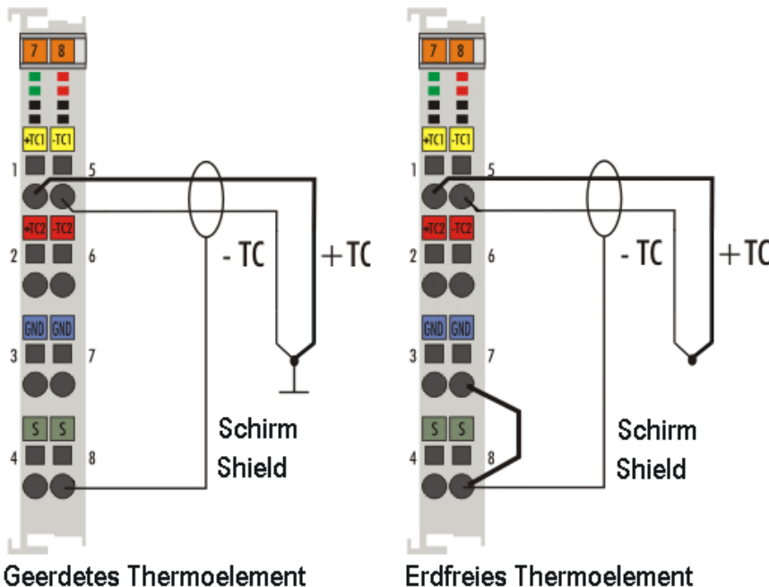
Abb. 97: Anschlussstechniken geerdetes - und erdfreies Thermoelement
