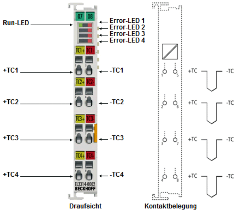
Abb. 22: EL3314-0002
