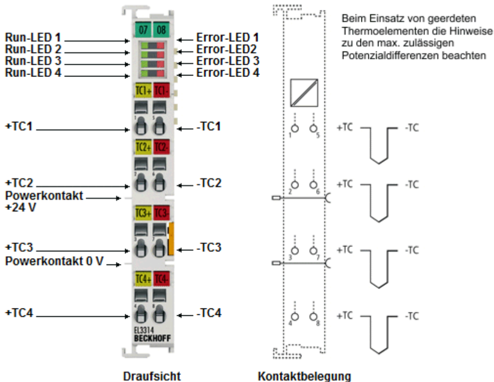
Abb. 8: EL3314
