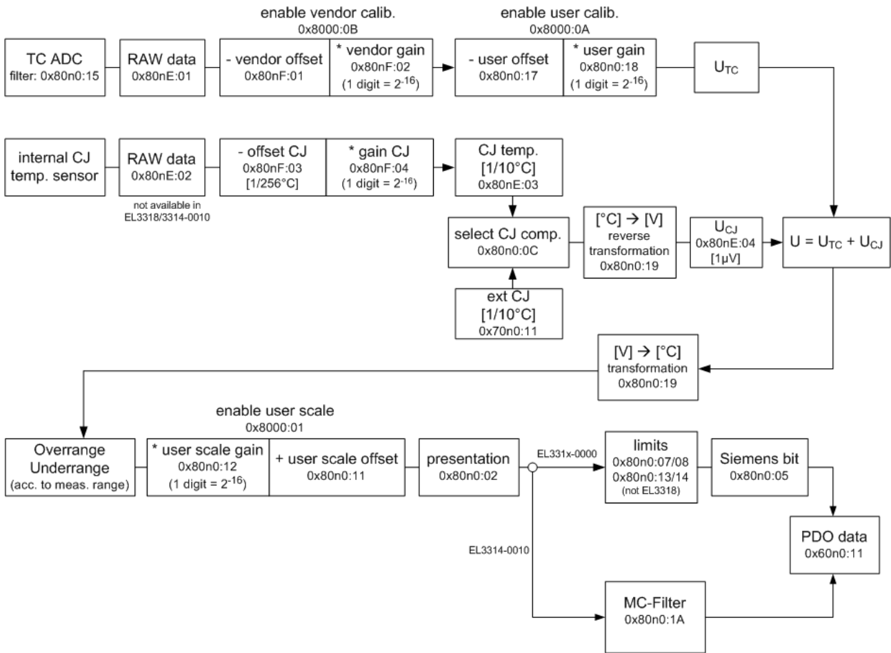
Abb. 214: EL33xx Dataflow
