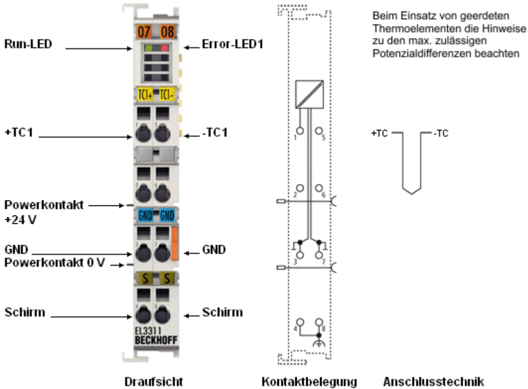
Abb. 5: EL3311
