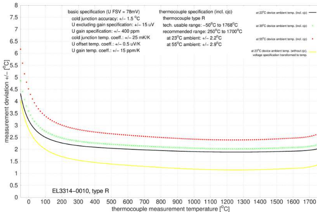
Abb. 31: EL3314-0010, EL3314-0020 und EL3314-0030 (entsprechen EL3314-0010), Typ R
