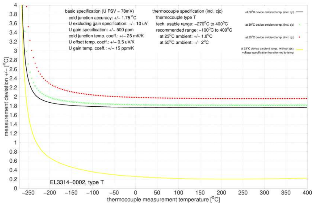
Abb. 20: EL3314-0002 und EL3314-0092 (entspricht EL3314-0002), Typ T
