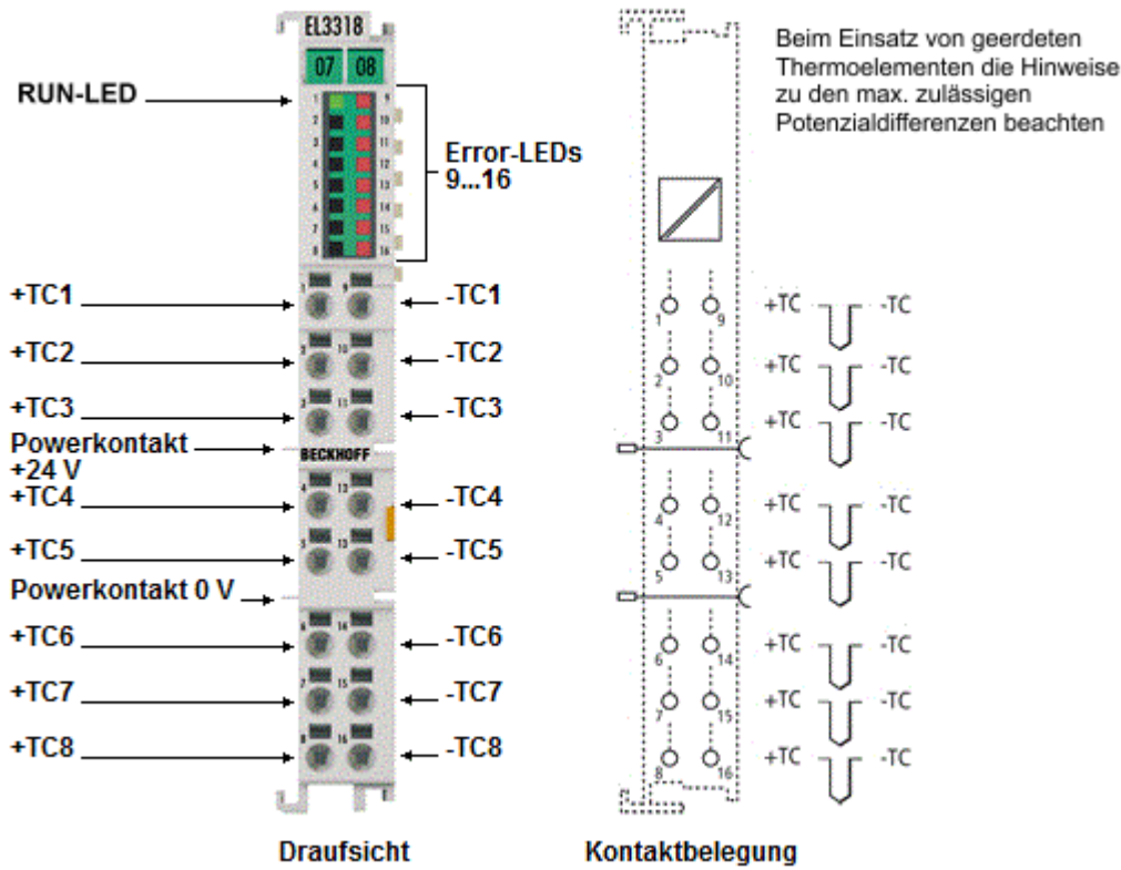
Abb. 79: EL3318
