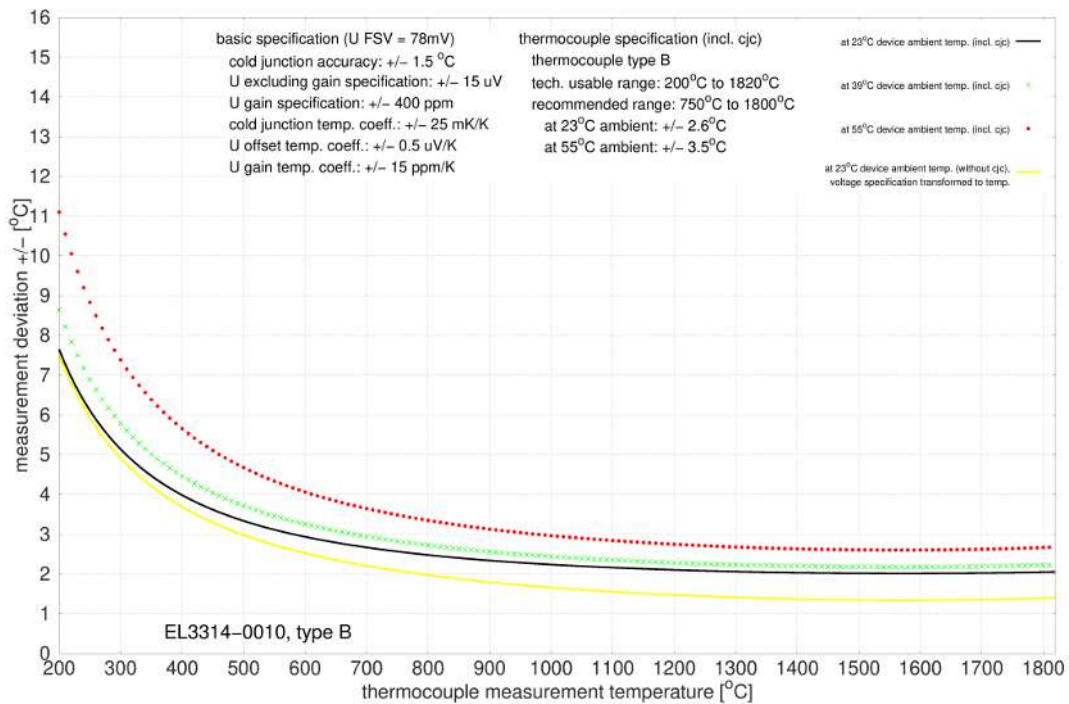
Abb. 50: EL3314-0010, EL3314-0020 und EL3314-0030 (entsprechen EL3314-0010), Typ B
