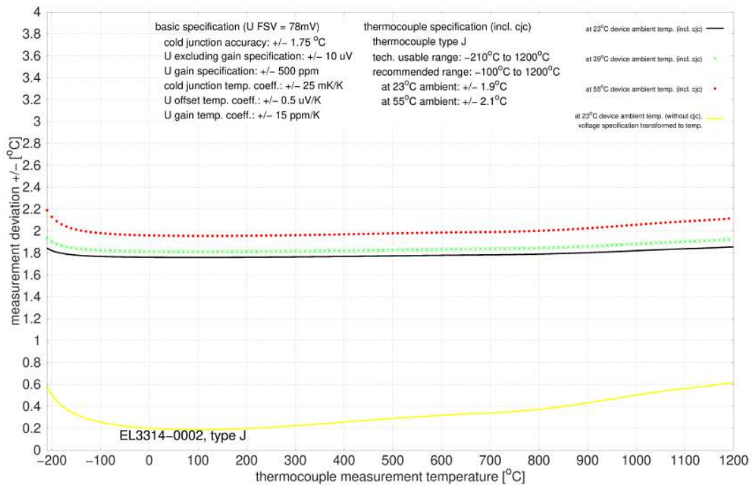
Abb. 14: EL3314-0002 und EL3314-0092 (entspricht EL3314-0002), Typ J
