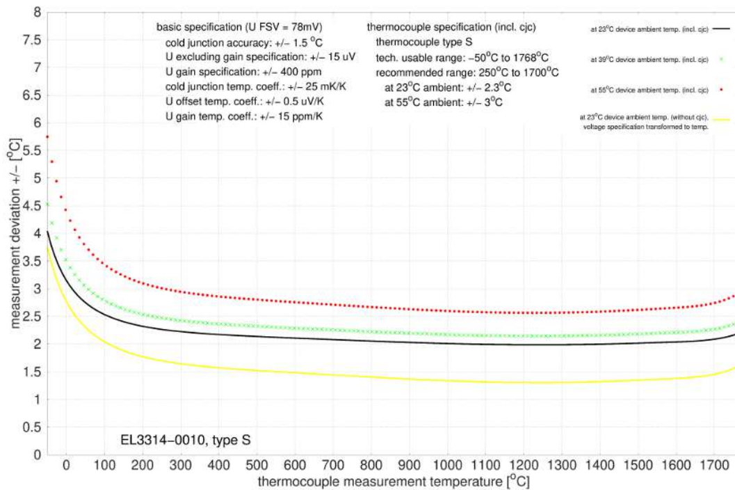
Abb. 58: EL3314-0010, EL3314-0020 und EL3314-0030 (entsprechen EL3314-0010), Typ S
