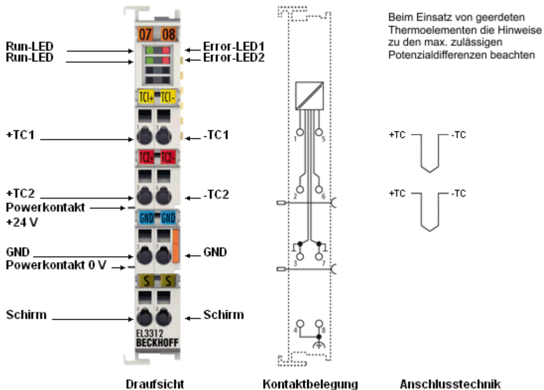
Abb. 6: EL3312
