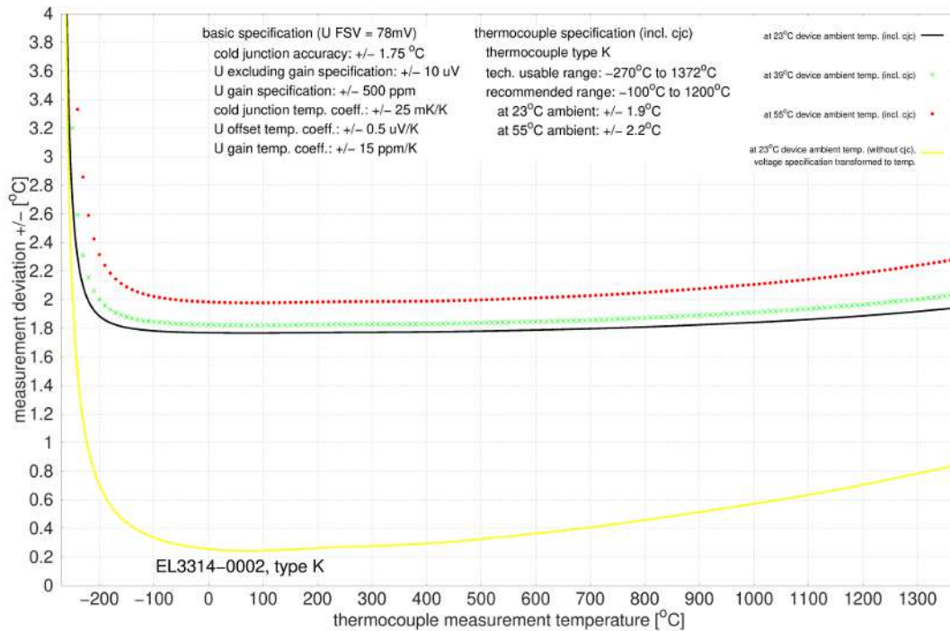
Abb. 69: EL3314-0002 und EL3314-0092 (entspricht EL3314-0002), Typ K
