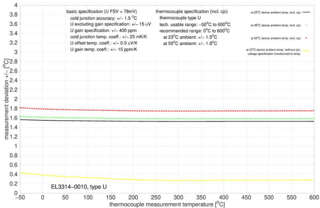
Abb. 34: EL3314-0010, EL3314-0020 und EL3314-0030 (entsprechen EL3314-0010), Typ U
