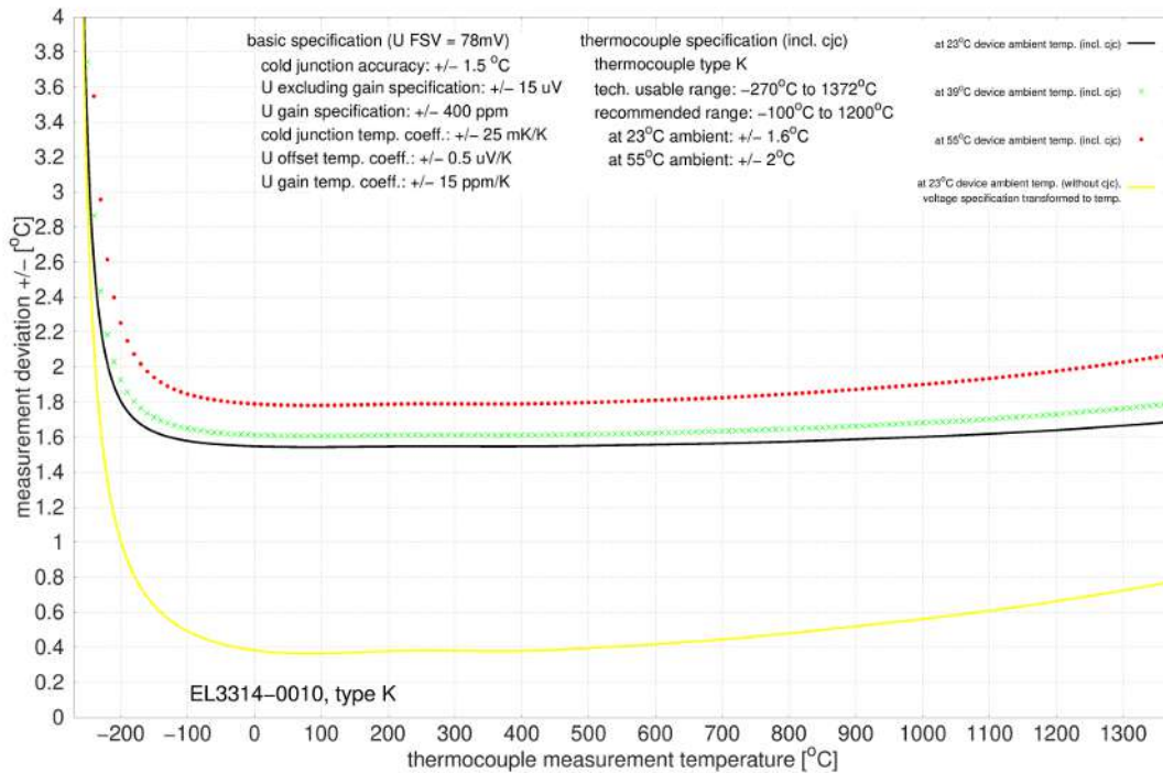
Abb. 54: EL3314-0010, EL3314-0020 und EL3314-0030 (entsprechen EL3314-0010), Typ K
