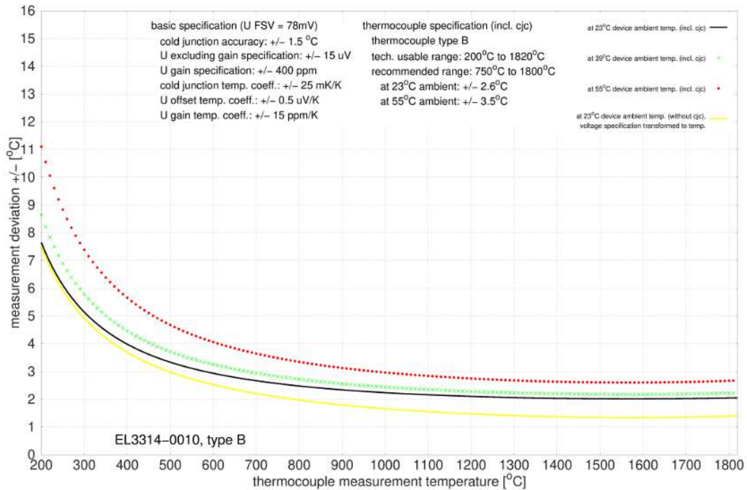
Abb. 24: EL3314-0010, EL3314-0020 und EL3314-0030 (entsprechen EL3314-0010), Typ B
