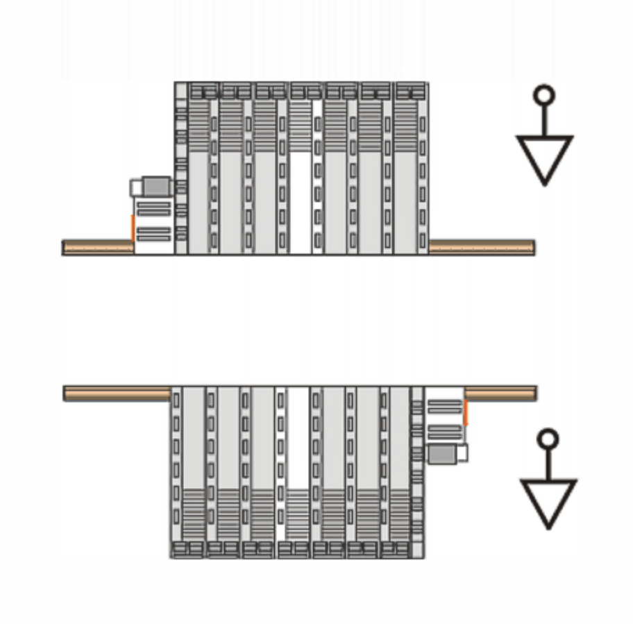
Abb. 101: Weitere Einbaulagen
