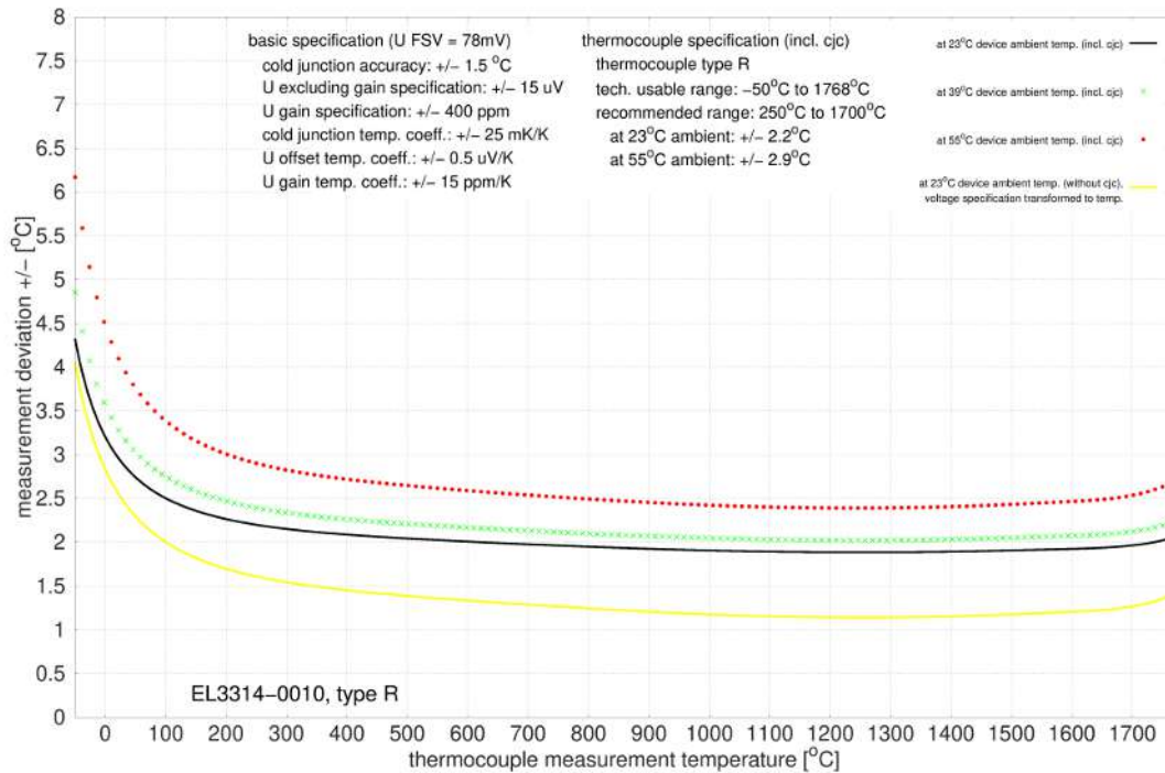
Abb. 57: EL3314-0010, EL3314-0020 und EL3314-0030 (entsprechen EL3314-0010), Typ R
