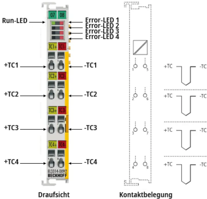
Abb. 76: EL3314-0092
