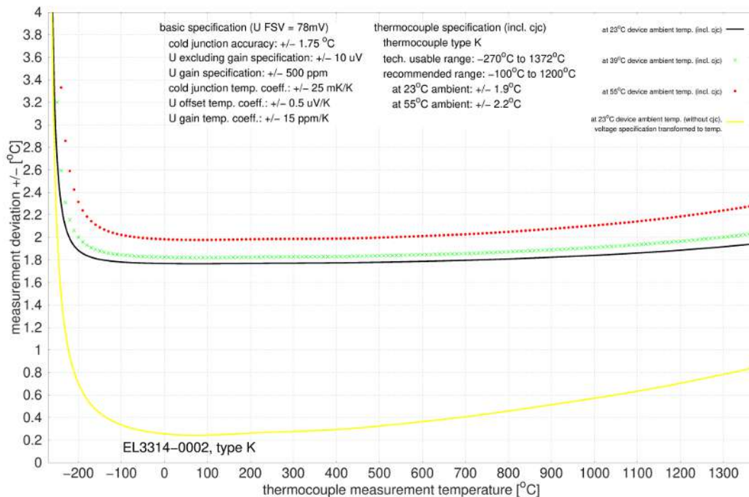
Abb. 15: EL3314-0002 und EL3314-0092 (entspricht EL3314-0002), Typ K
