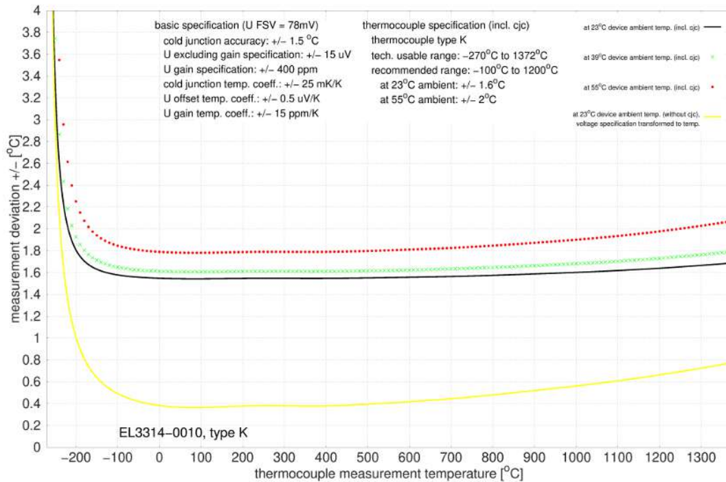
Abb. 41: EL3314-0010, EL3314-0020 und EL3314-0030 (entsprechen EL3314-0010), Typ K
