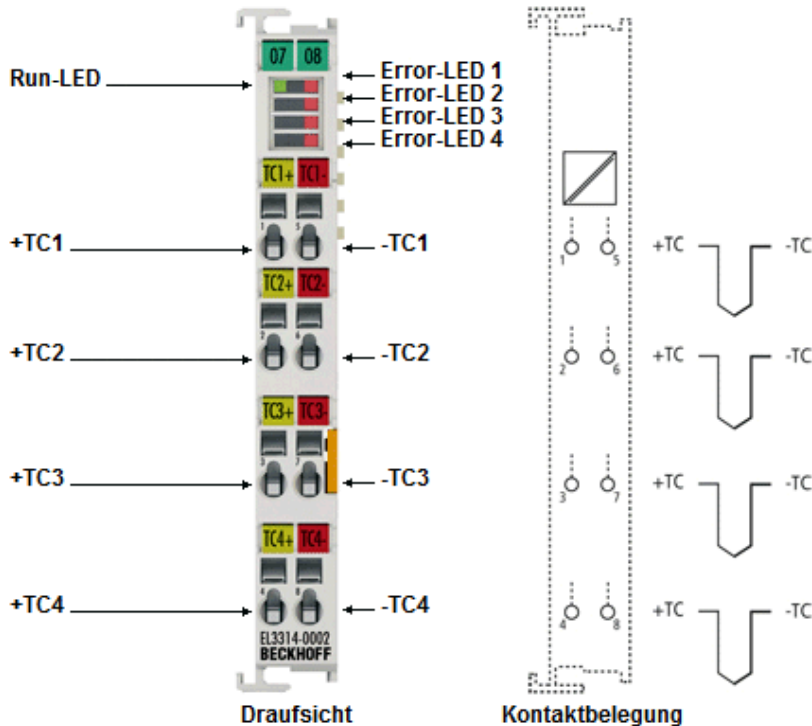
Abb. 10: EL3314-0002
