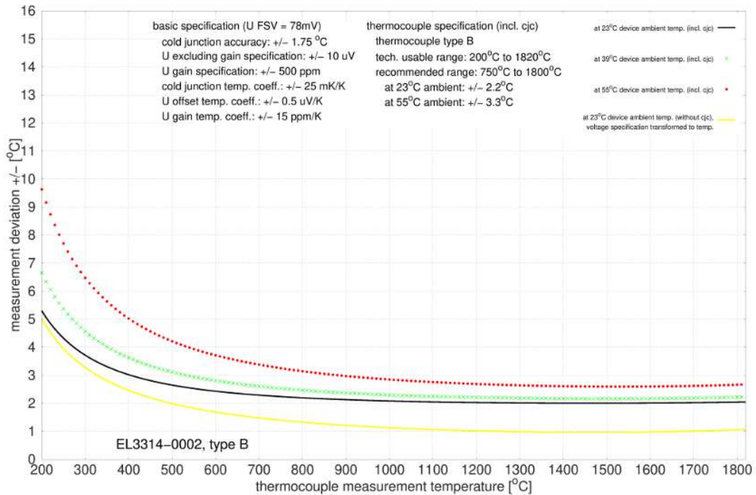
Abb. 65: EL3314-0002 und EL3314-0092 (entspricht EL3314-0002), Typ B
