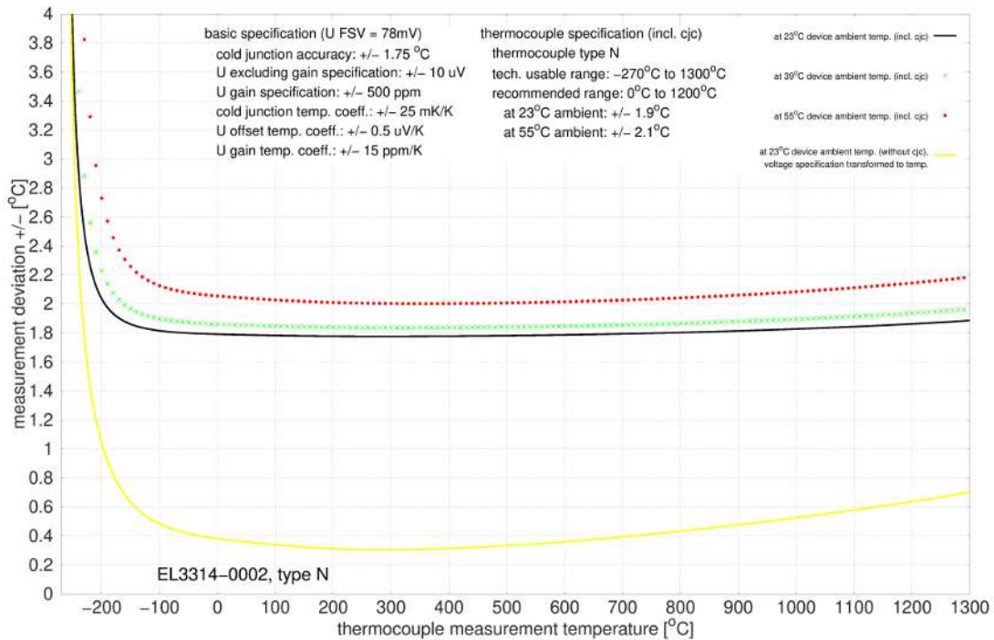
Abb. 71: EL3314-0002 und EL3314-0092 (entspricht EL3314-0002), Typ N
