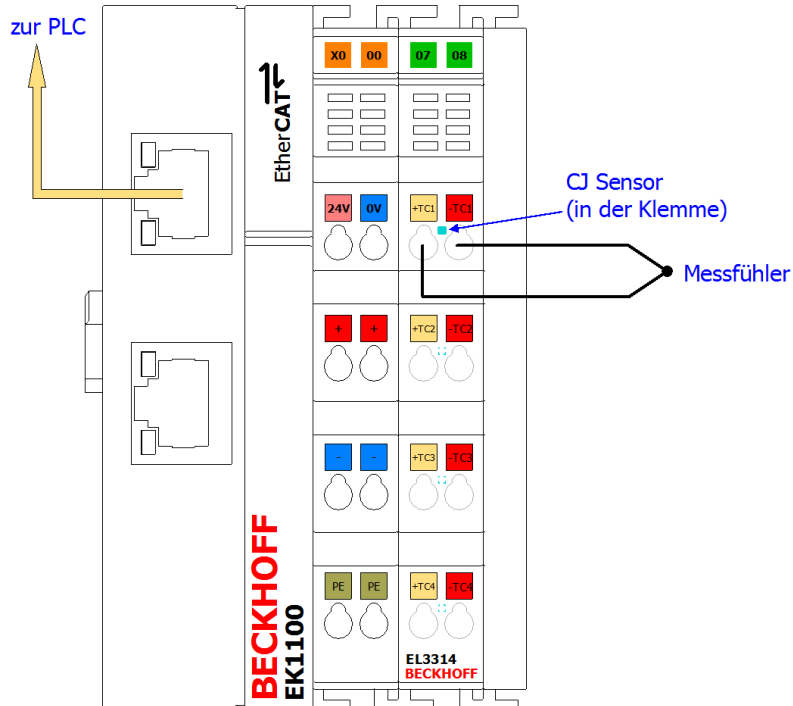
Abb. 241: Aufbau zum Beispielprogramm zur „separaten Temperaturberechnung mit CJC in der PLC“
