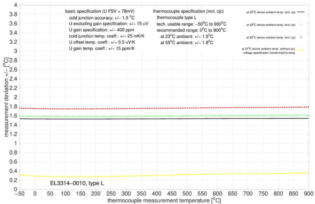
Abb. 55: EL3314-0010, EL3314-0020 und EL3314-0030 (entsprechen EL3314-0010), Typ L
