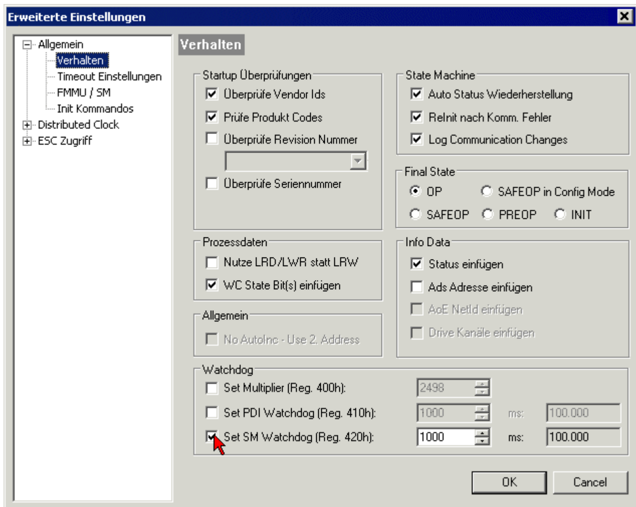
Abb. 83: Karteireiter EtherCAT -> Erweiterte Einstellungen -> Verhalten -> Watchdog
