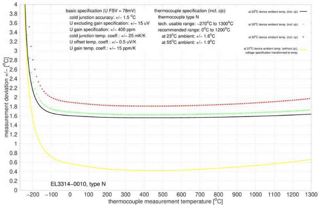
Abb. 56: EL3314-0010, EL3314-0020 und EL3314-0030 (entsprechen EL3314-0010), Typ N
