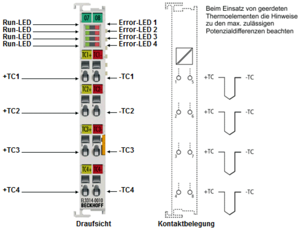
Abb. 48: EL3314-0020 (entspricht EL3314-0010)
