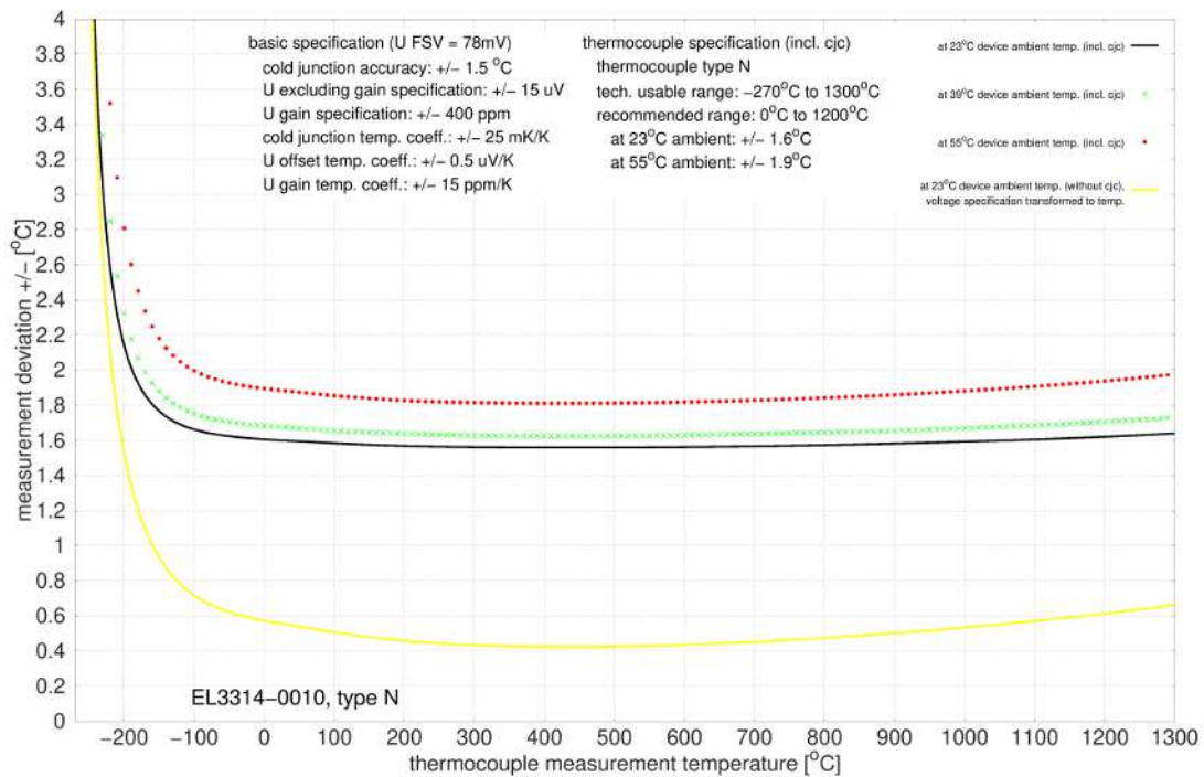
Abb. 30: EL3314-0010, EL3314-0020 und EL3314-0030 (entsprechen EL3314-0010), Typ N
