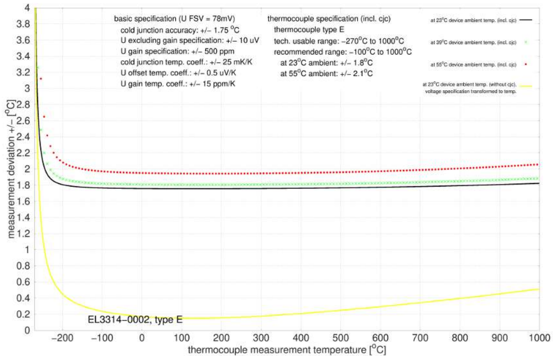
Abb. 67: EL3314-0002 und EL3314-0092 (entspricht EL3314-0002), Typ E
