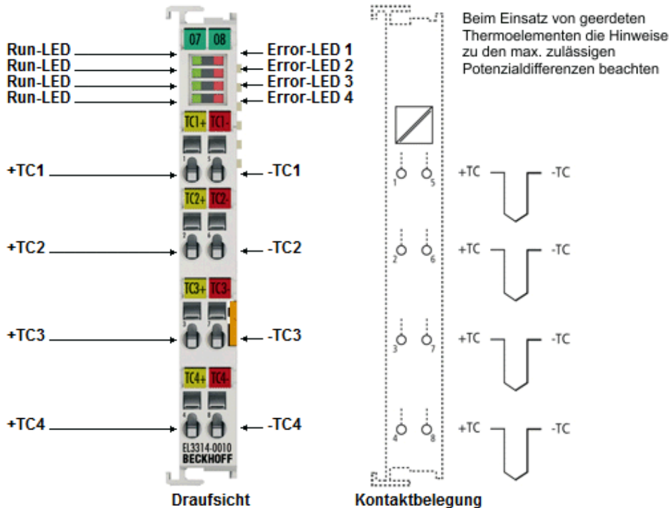
Abb. 36: EL3314-0020 (entspricht EL3314-0010)
