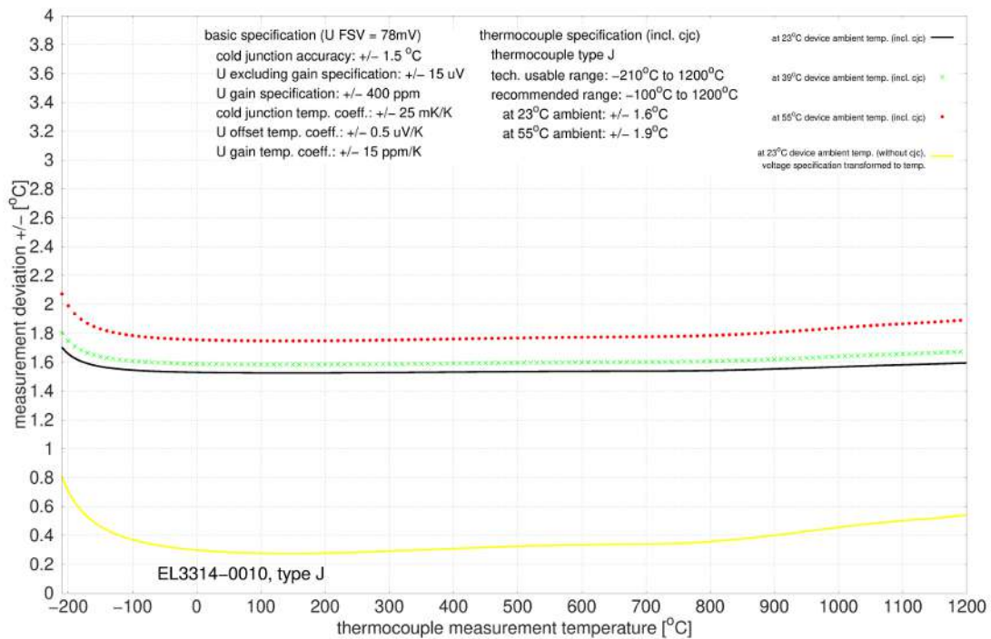
Abb. 40: EL3314-0010, EL3314-0020 und EL3314-0030 (entsprechen EL3314-0010), Typ J
