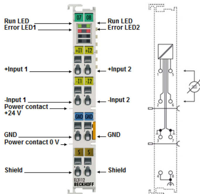
附图 12: EL3112
