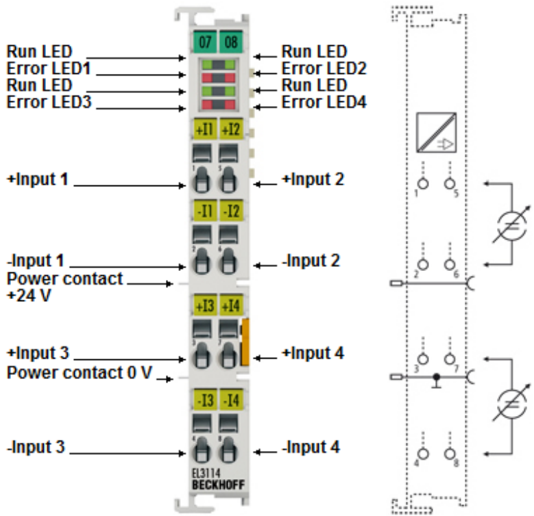
附图 17: EL3114 - LED 和连接
