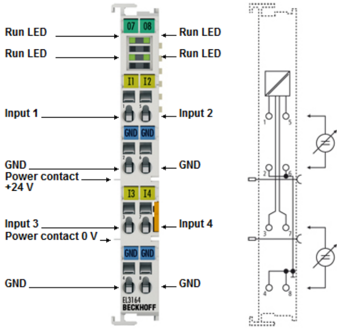
附图 45: EL3164 - LED 和连接
