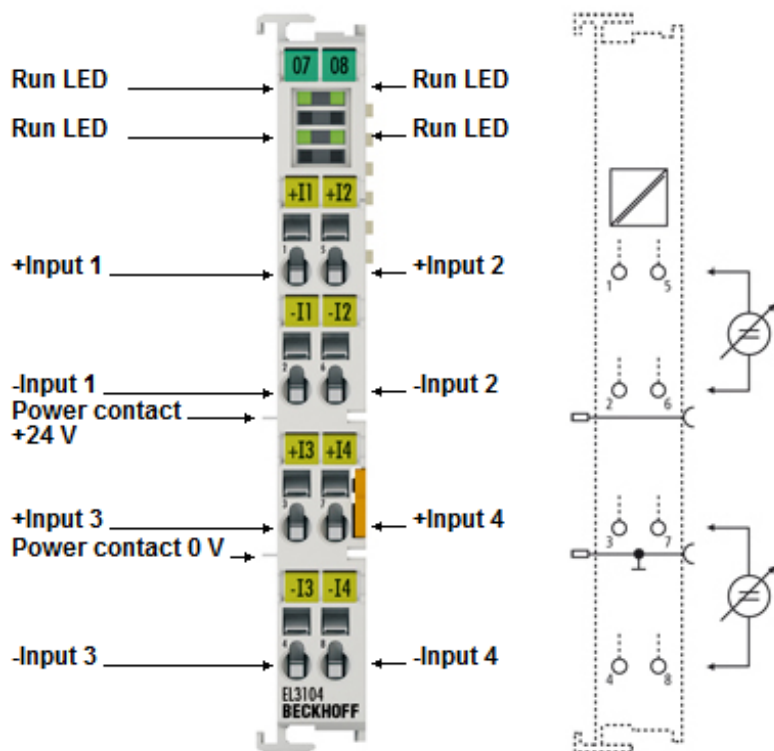
附图 8: EL3104
