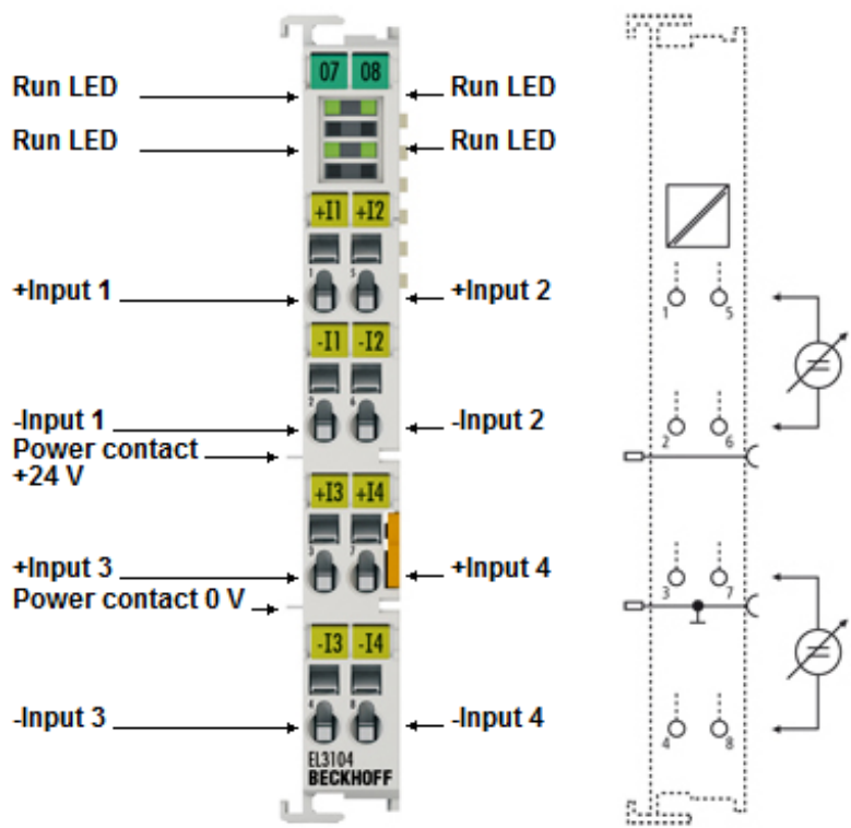
附图 9: EL3104 - LED 和连接
