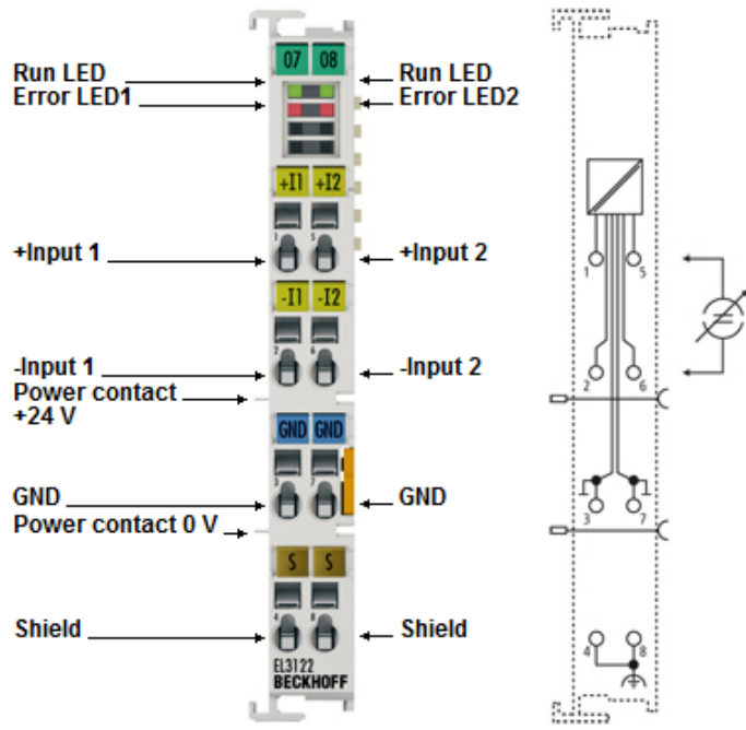
附图 21: EL3122 - LED 和连接
