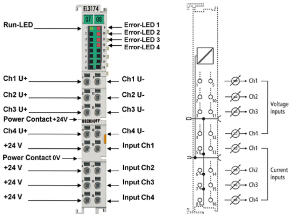
附图 48: EL3174
