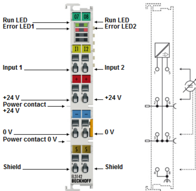
附图 28: EL3142
