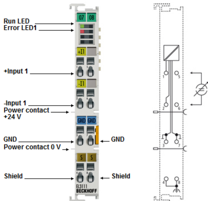
附图 10: EL3111
