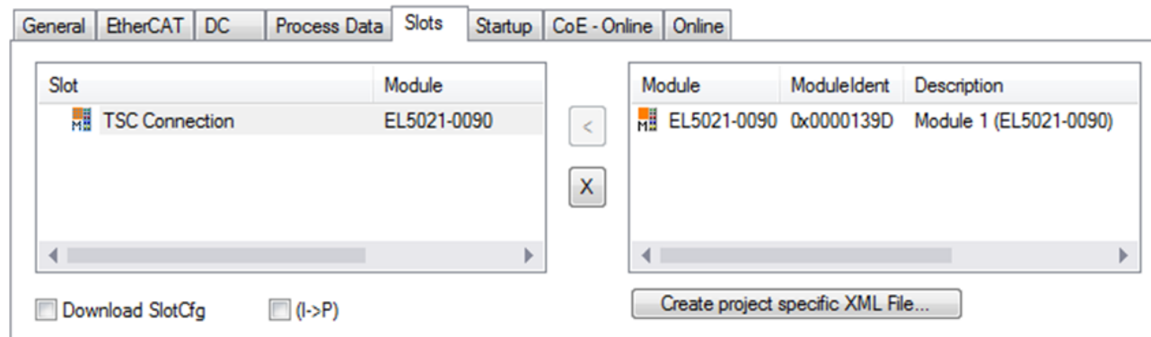
附图 221: 在组件下添加TwinSAFE SC过程数据，如EL5021-0090
