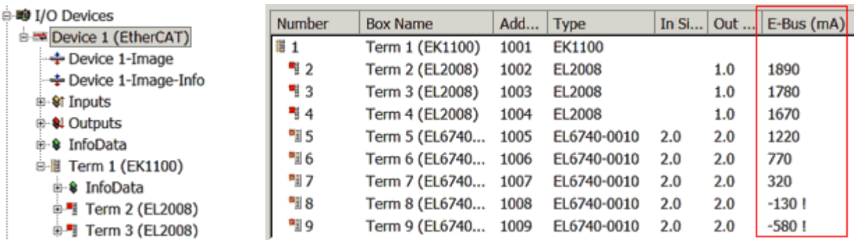
附图 61: System Manager中的电流计算
