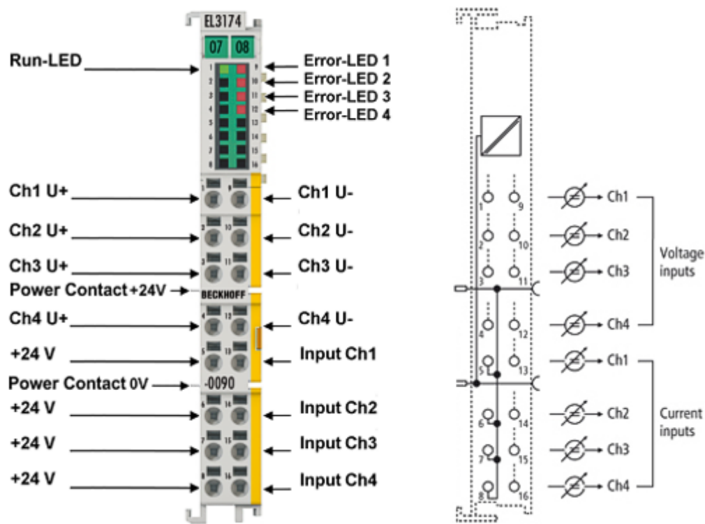
附图 60: EL3174-0090 - LED 和连接
