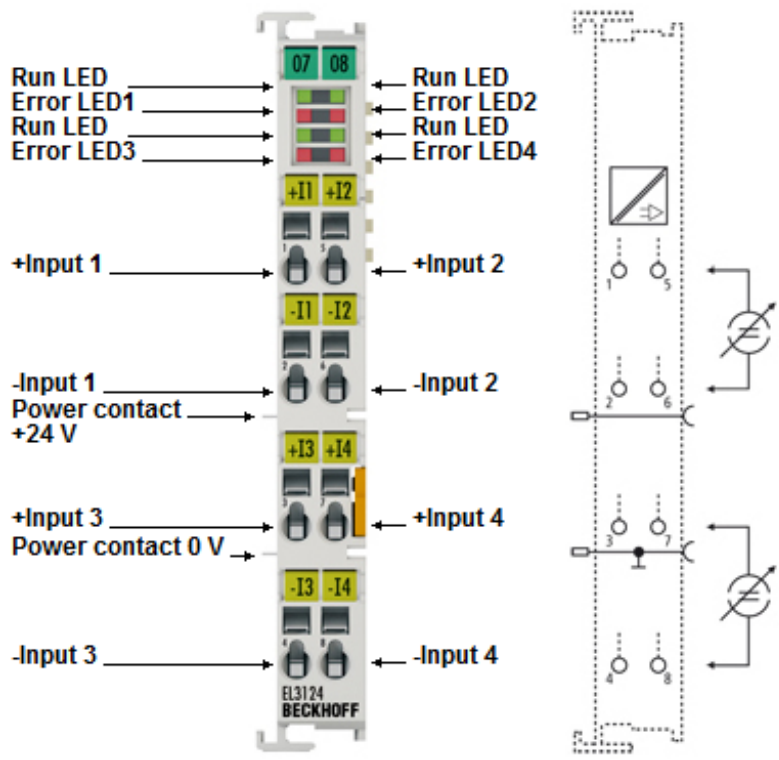
附图 23: EL3124 - LED 和连接
