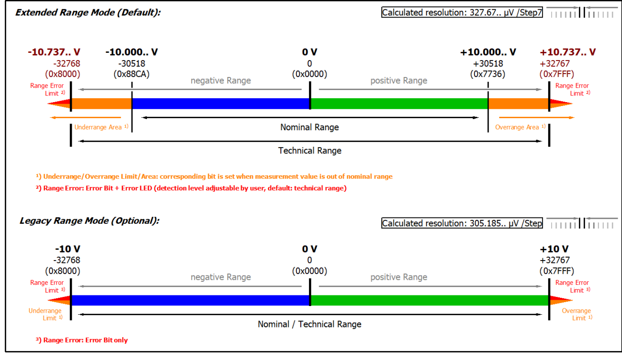
附图 209: EL3172、EL3174、EL3174-0002、EL3174-0090：量程 -10…+10 V
