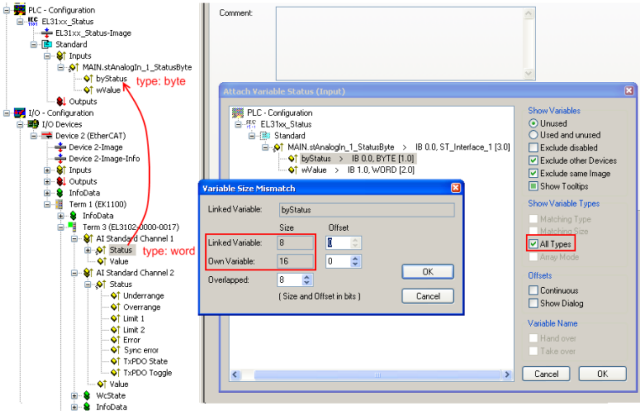
附图 201: 将 EL31xx 的 4 字节接口连接到项目中已有的 3 字节接口
