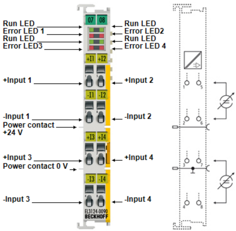
附图 25: EL3124-0090 - LED 和连接
