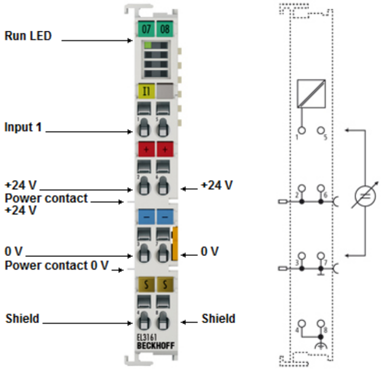
附图 41: EL3161 - LED 和连接
