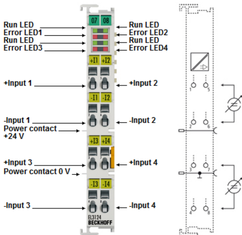
附图 22: EL3124
