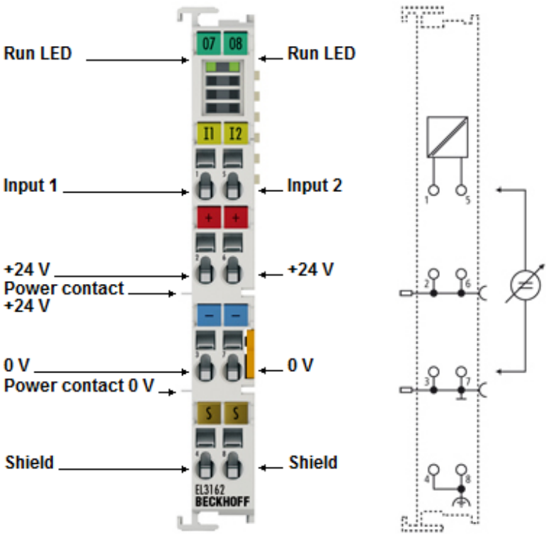
附图 43: EL3162 - LED 和连接
