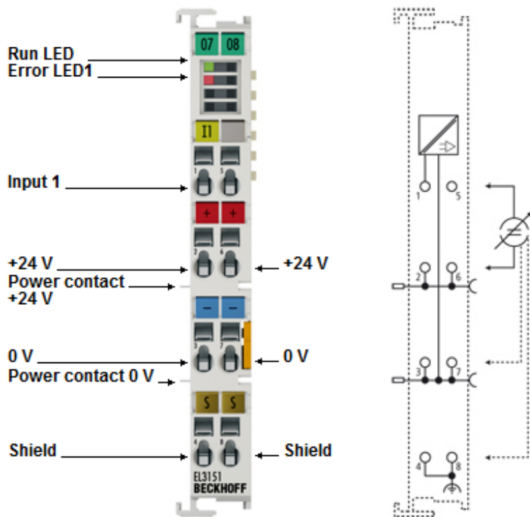
附图 34: EL3151
