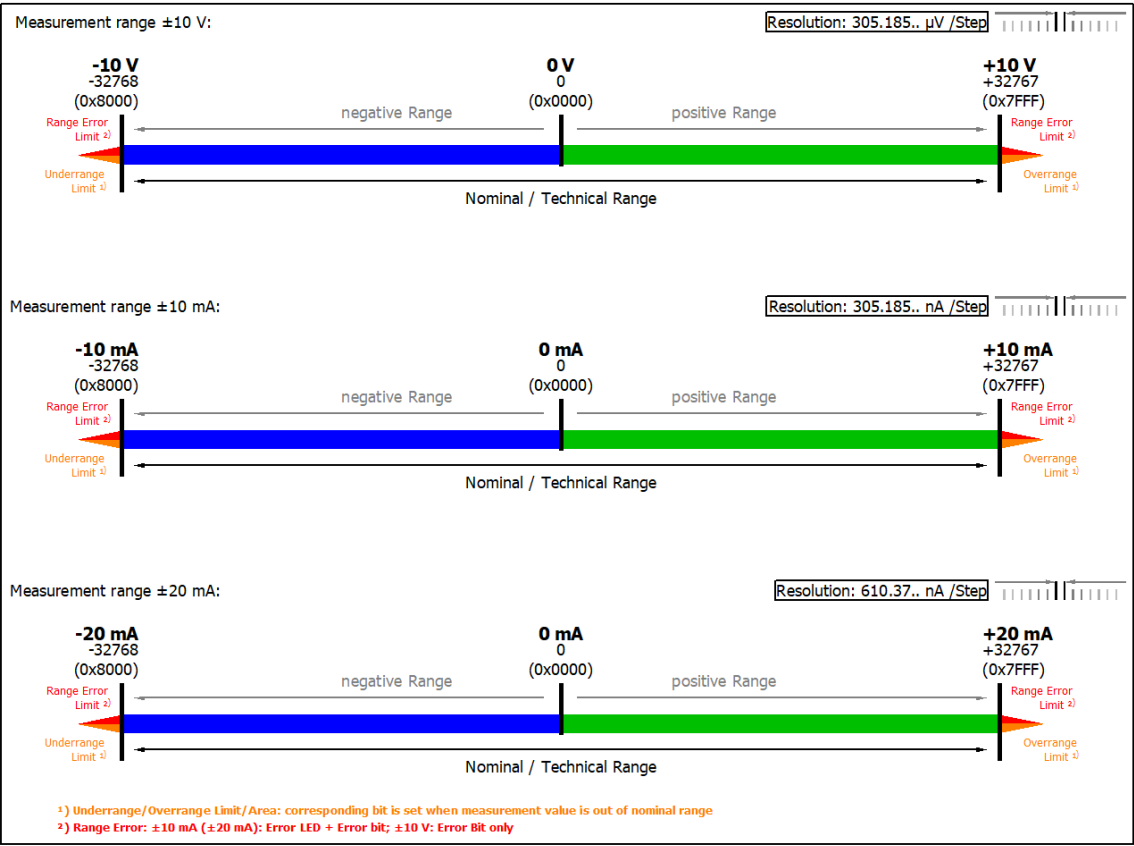
附图 205: 量程 \pm 10\text{ V} 、 \pm 10\text{ mA} 和 \pm 20\text{ mA} (下表中“X”表示适用范围)
