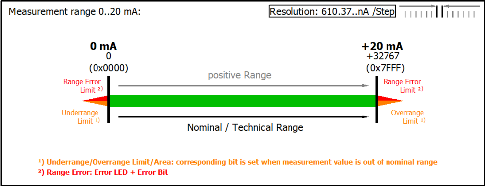
附图 206: 量程 0...20 mA
