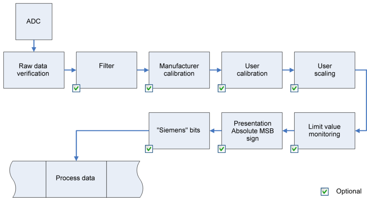
附图 204: EL31xx 的数据流示意图
