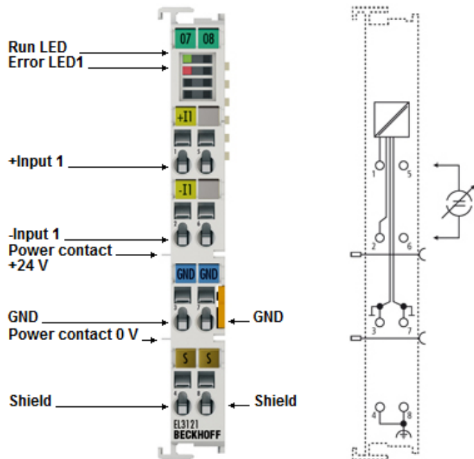
附图 18: EL3121
