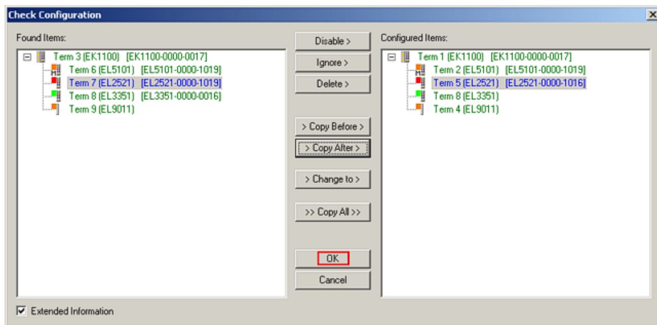
附图 168: 更正对话框，有修改项
