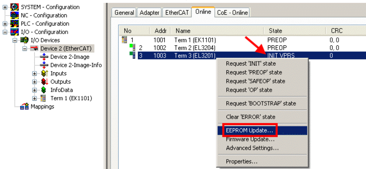
附图 235: EEPROM 更新
