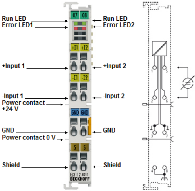
附图 15: EL3112-0011 – LED 和连接
