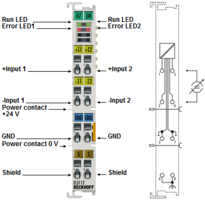
附图 13: EL3112 - LED 和连接
