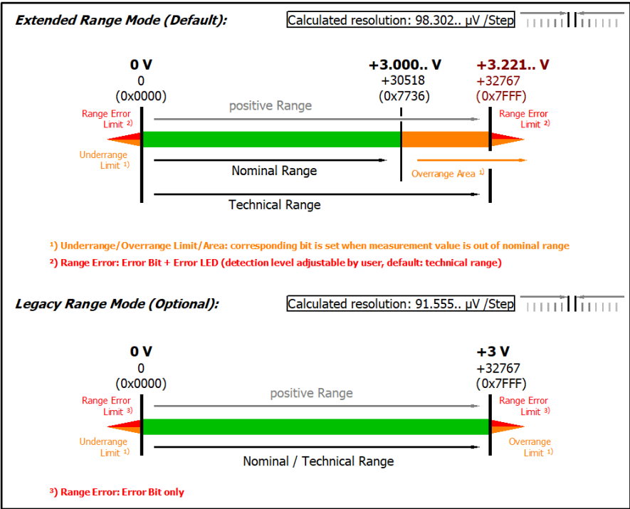
附图 214: EL3174-0032：量程 0…3 V
