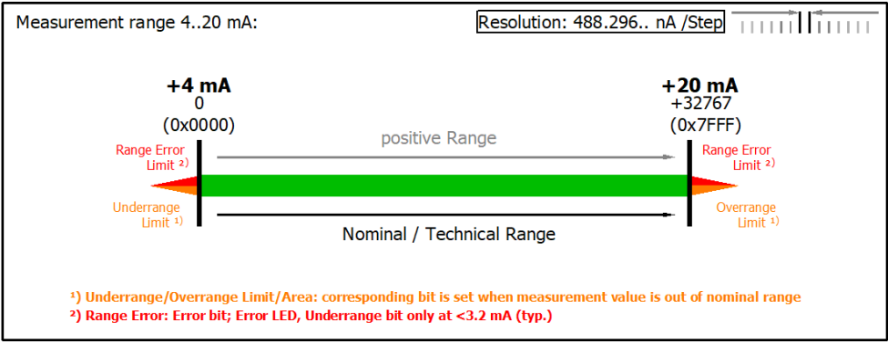
附图 207: 量程 4...20 mA
