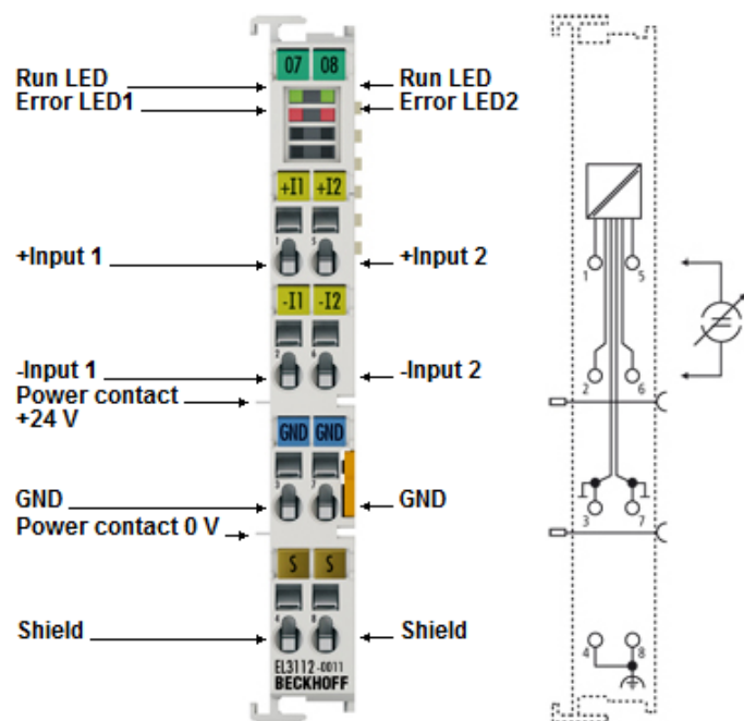
附图 14: EL3112-0011
