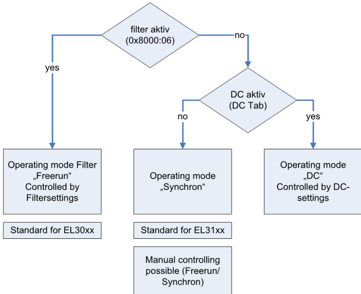
附图 193: 运行模式的关系
