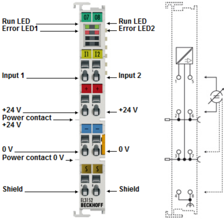
附图 37: EL3152 - LED 和连接
