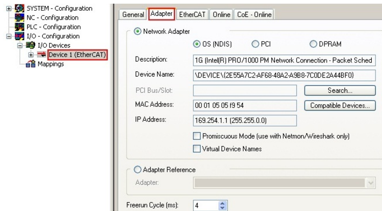
附图 143: EtherCAT 设备属性（TwinCAT 2）
