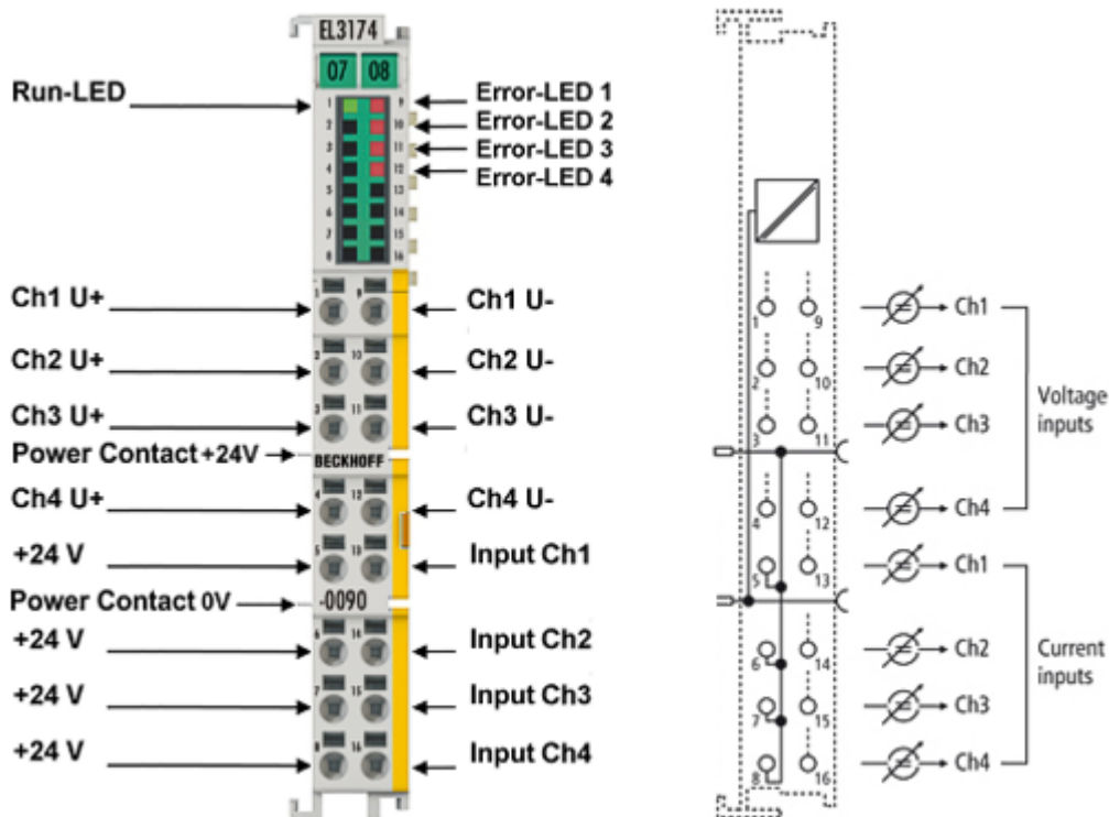
附图 59: EL3174-0090
