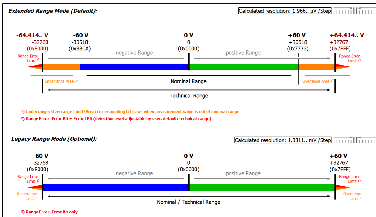
附图 212: EL3174-0042: 量程 -60\cdots+60\text{ V}
