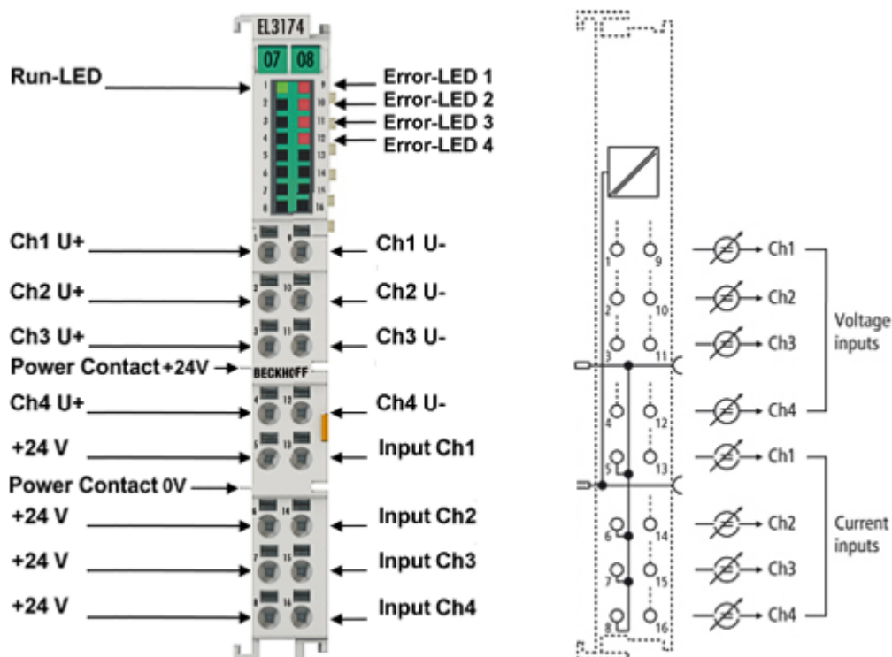
附图 52: EL3174-0030
