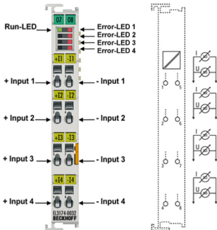
附图 55: EL3174-0032
