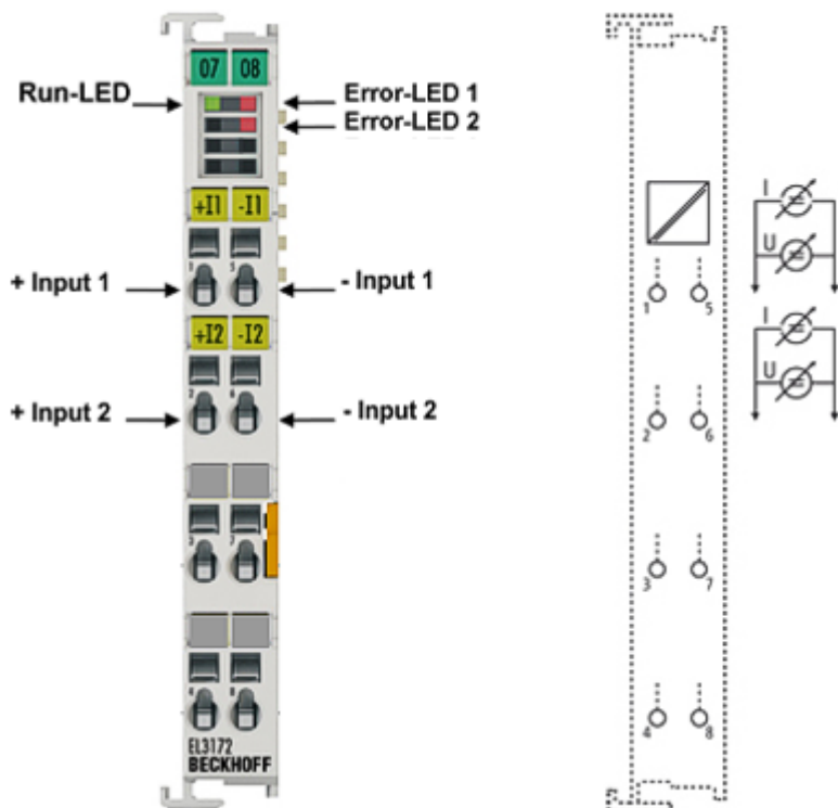
附图 46: EL3172
