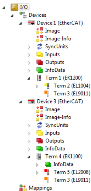
附图 106: 在集成于 VS shell 的TwinCAT 3 环境中配置映射
