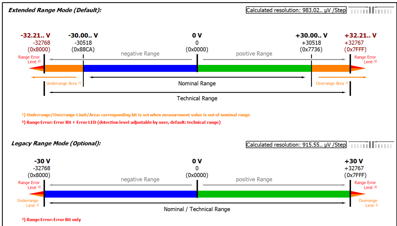
附图 211: EL3174-0042: 量程 -30\cdots+30\text{ V}
