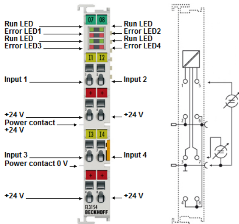
附图 38: EL3154
