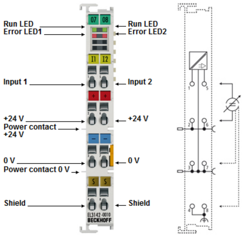
附图 31: EL3142-0010 - LED 和连接
