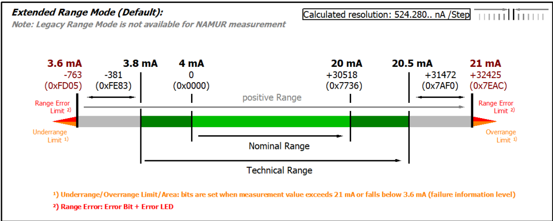
附图 218: EL3172, EL3174, EL3174-00xx: 量程 4...20 mA (NAMUR NE43)
