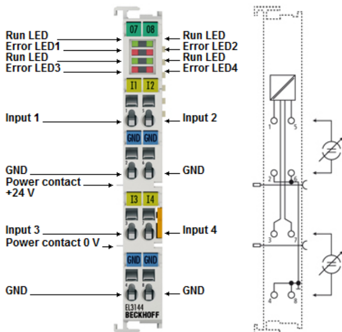
附图 32: EL3144
