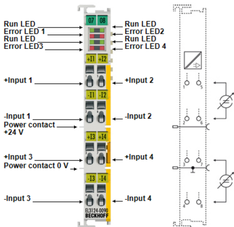
附图 24: EL3124-0090
