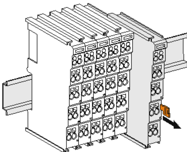
附图 71: 端子模块的拆卸
