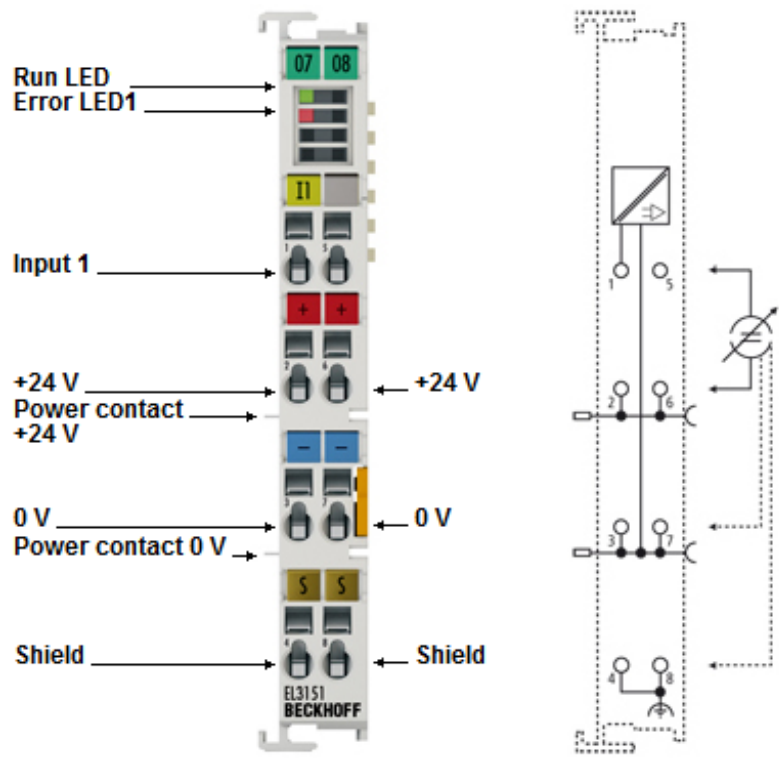
附图 35: EL3151 - LED 和连接
