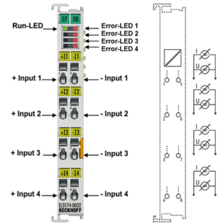
附图 56: EL3174-0032 - LED 和连接
