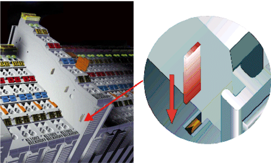
附图 70: 左侧的电源触点
