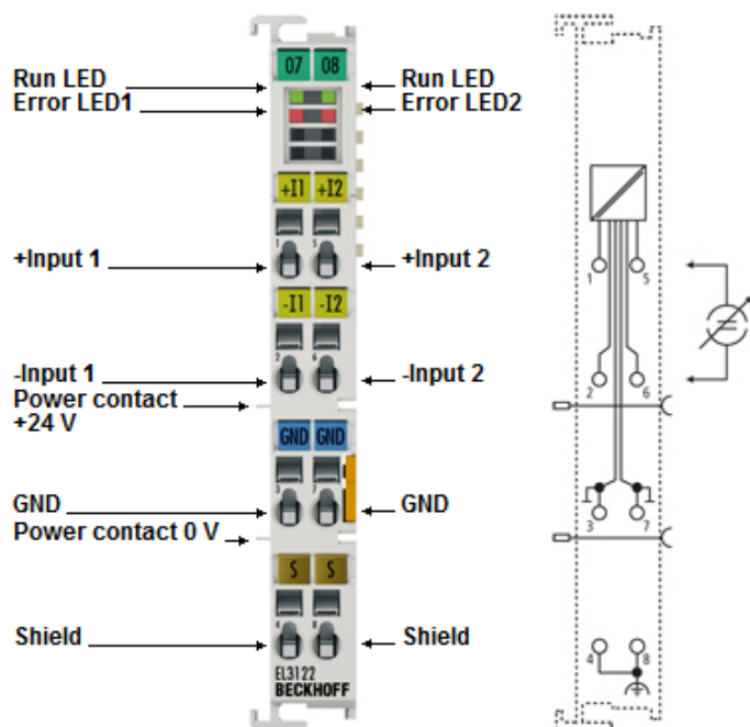
附图 20: EL3122
