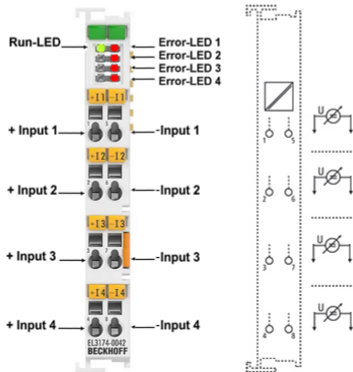
附图 58: EL3174-0042 - LED 和连接
