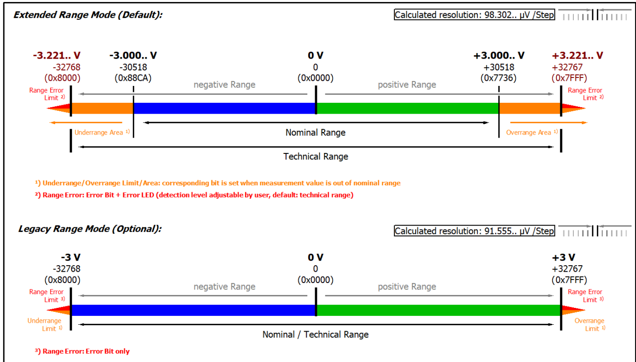
附图 210: EL3174-0032: 量程 -3\cdots+3\text{ V}
