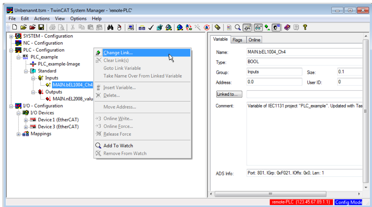
附图 93: 在 PLC 变量和过程对象之间建立链接
