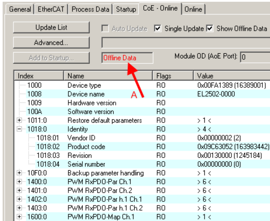
附图 66: 离线列表
