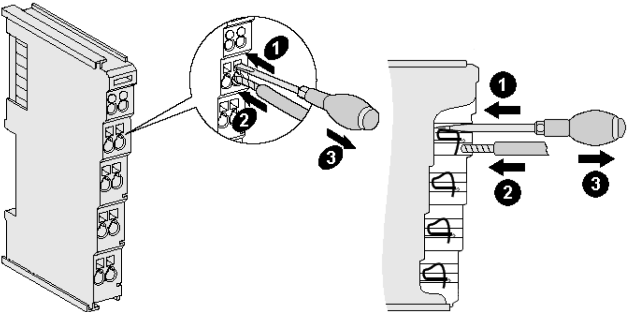
附图 75: 在一个接线点上连接线缆
