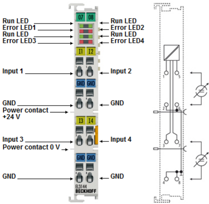
附图 33: EL3144 - LED 和连接
