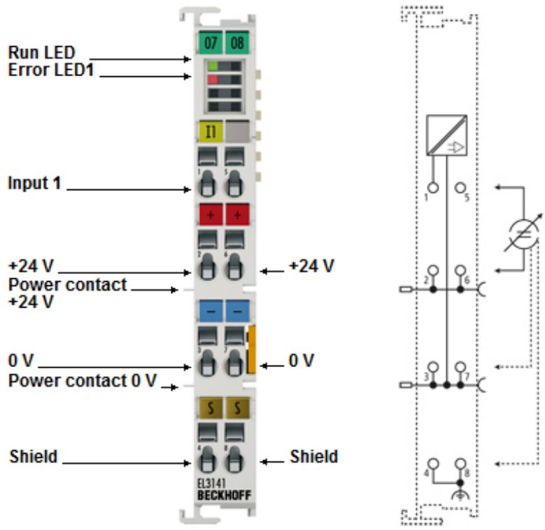
附图 27: EL3141 - LED 和连接
