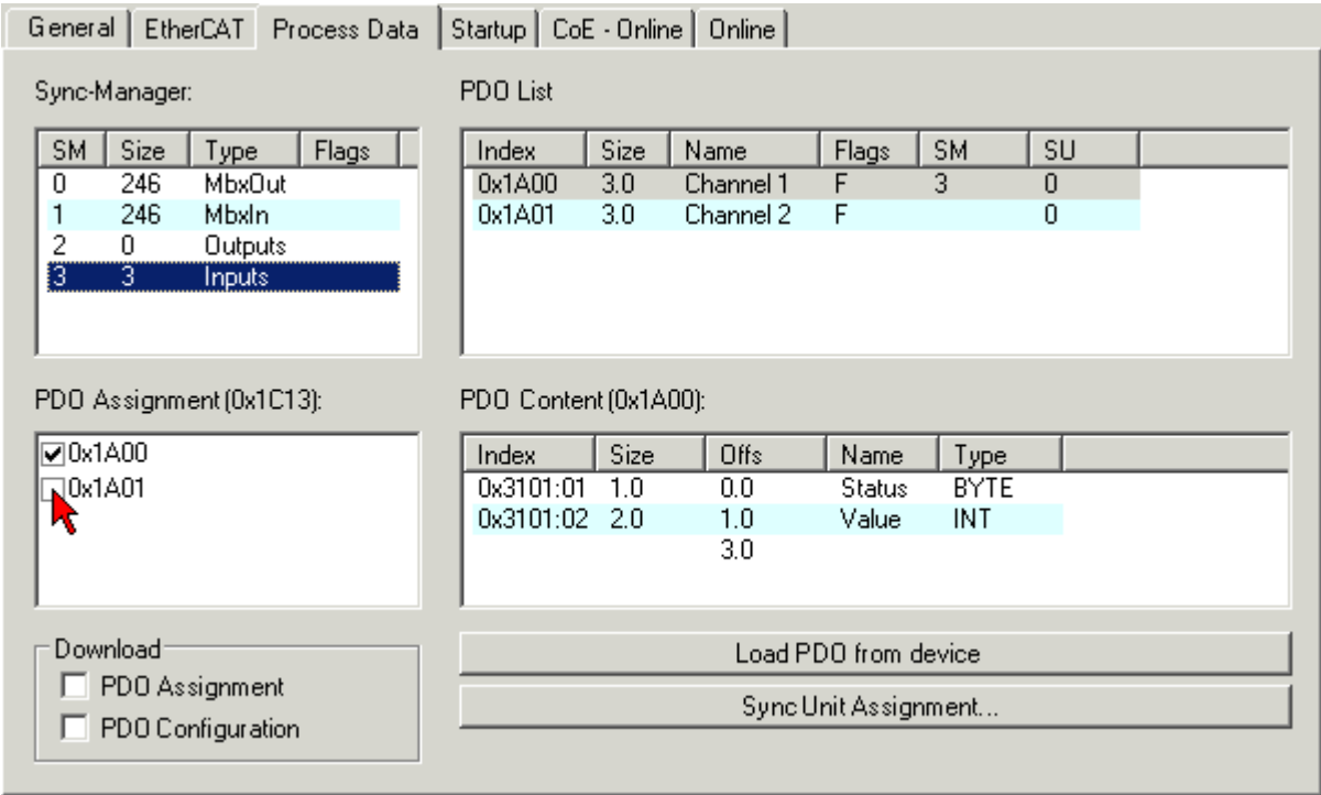
附图 219: 打开和关闭输入通道
