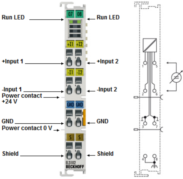
附图 7: EL3102 - LED 和连接
