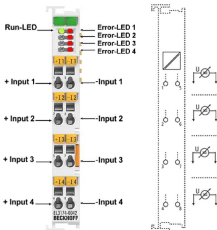
附图 57: EL3174-0042
