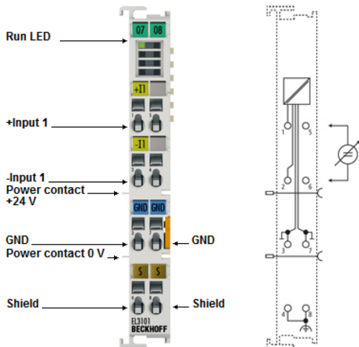
附图 4: EL3101
