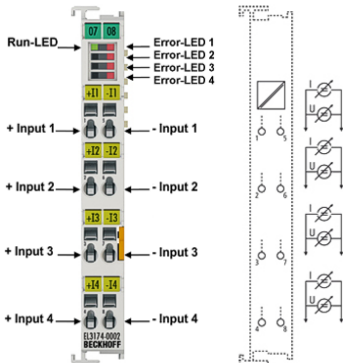
附图 50: EL3174-0002
