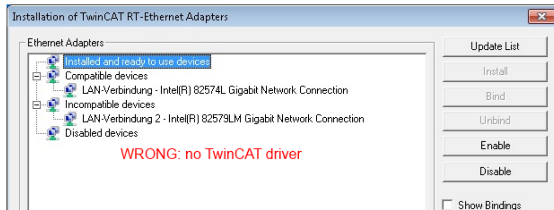
附图 129: 以太网端口驱动程序的错误设置
