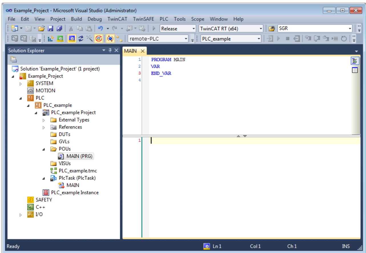
附图 110: 标准 PLC 项目的初始程序“Main”
