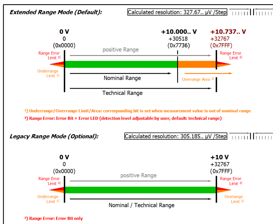
附图 213: EL3172、EL3174、EL3174-0002、EL3174-0090: 量程 0\cdots10\text{ V}
