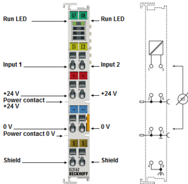
附图 42: EL3162
