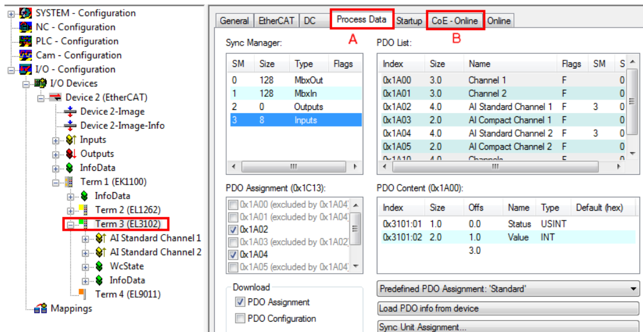
附图 190: EL31xx 参数化
