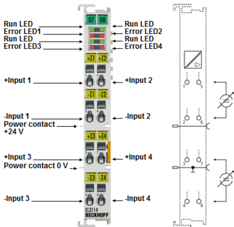
附图 16: EL3114
