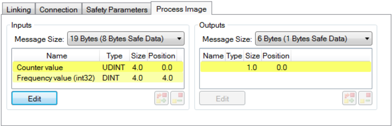
附图 226: 选择过程数据大小和过程数据
