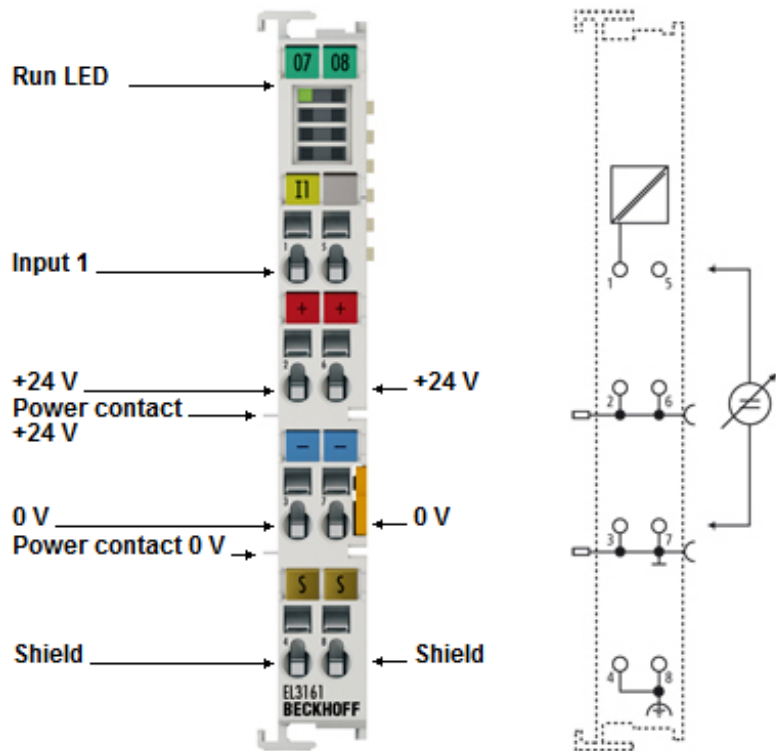
附图 40: EL3161
