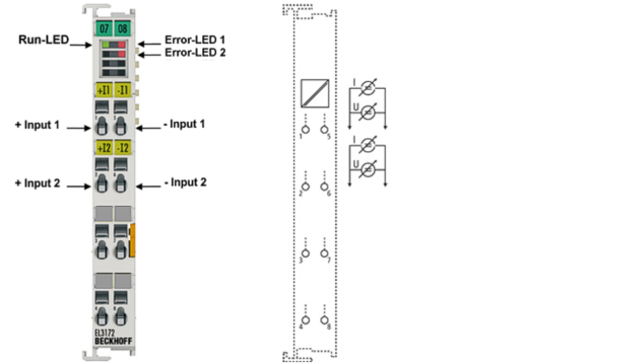
附图 47: EL3172 - LED 和连接
