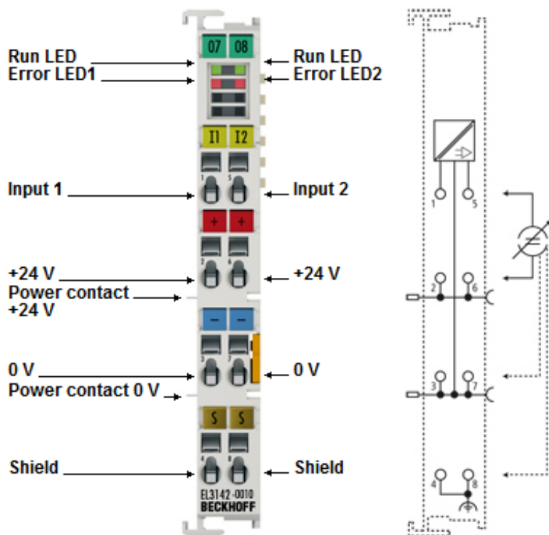
附图 30: EL3142-0010
