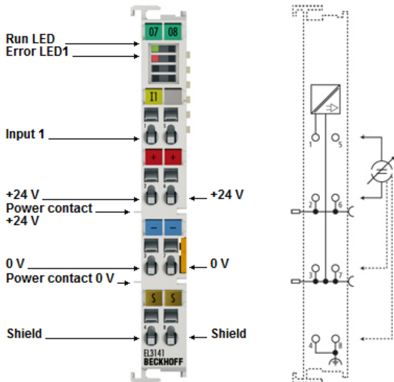
附图 26: EL3141
