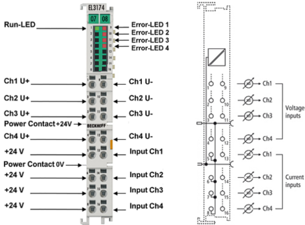
附图 53: EL3174-0030 - LED 和连接
