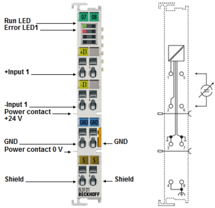
附图 19: EL3121 - LED 和连接
