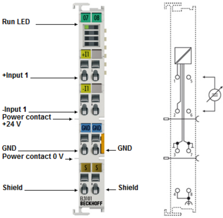
附图 5: EL3101 - LED 和连接
