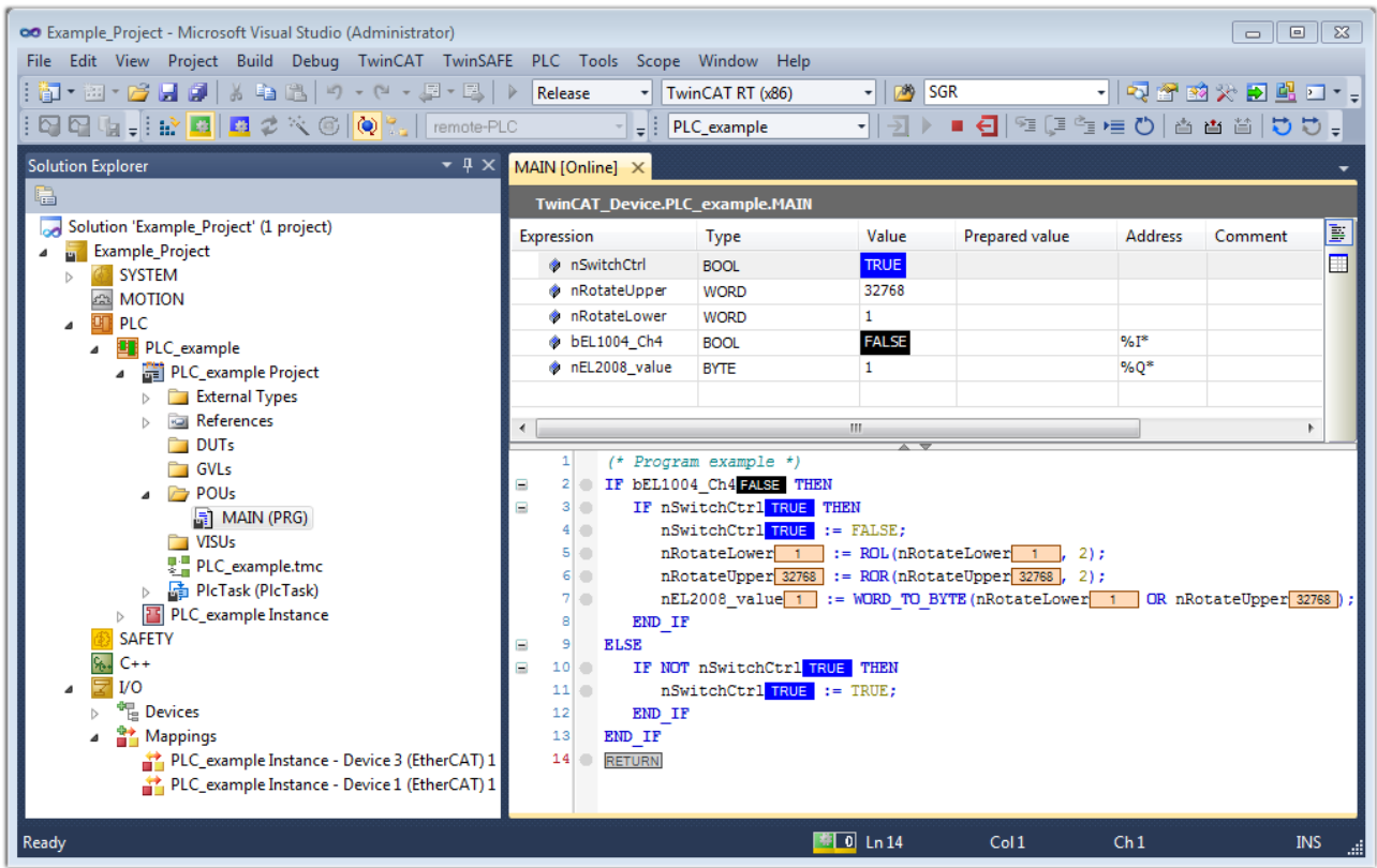
附图 121: TwinCAT 3 开发环境（VS shell）：Login 后，程序已运行
