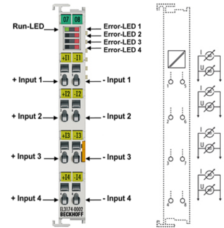
附图 51: EL3174-0002 - LED 和连接
