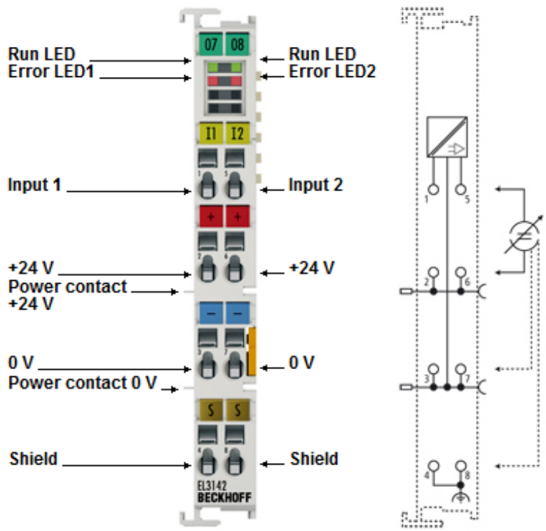
附图 29: EL3142 - LED 和连接
