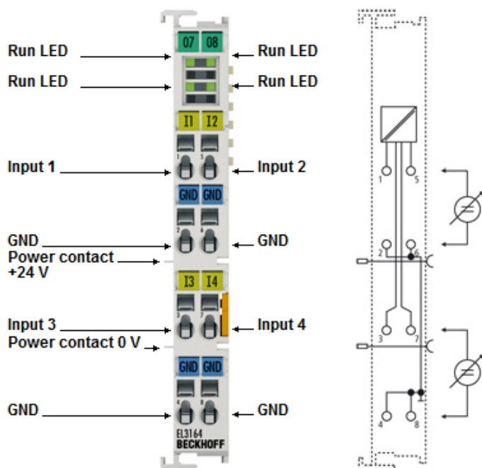
附图 44: EL3164
