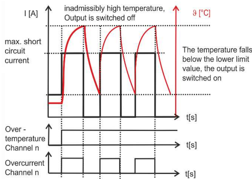
附图 9: 过载情况下的过热关断示意图
