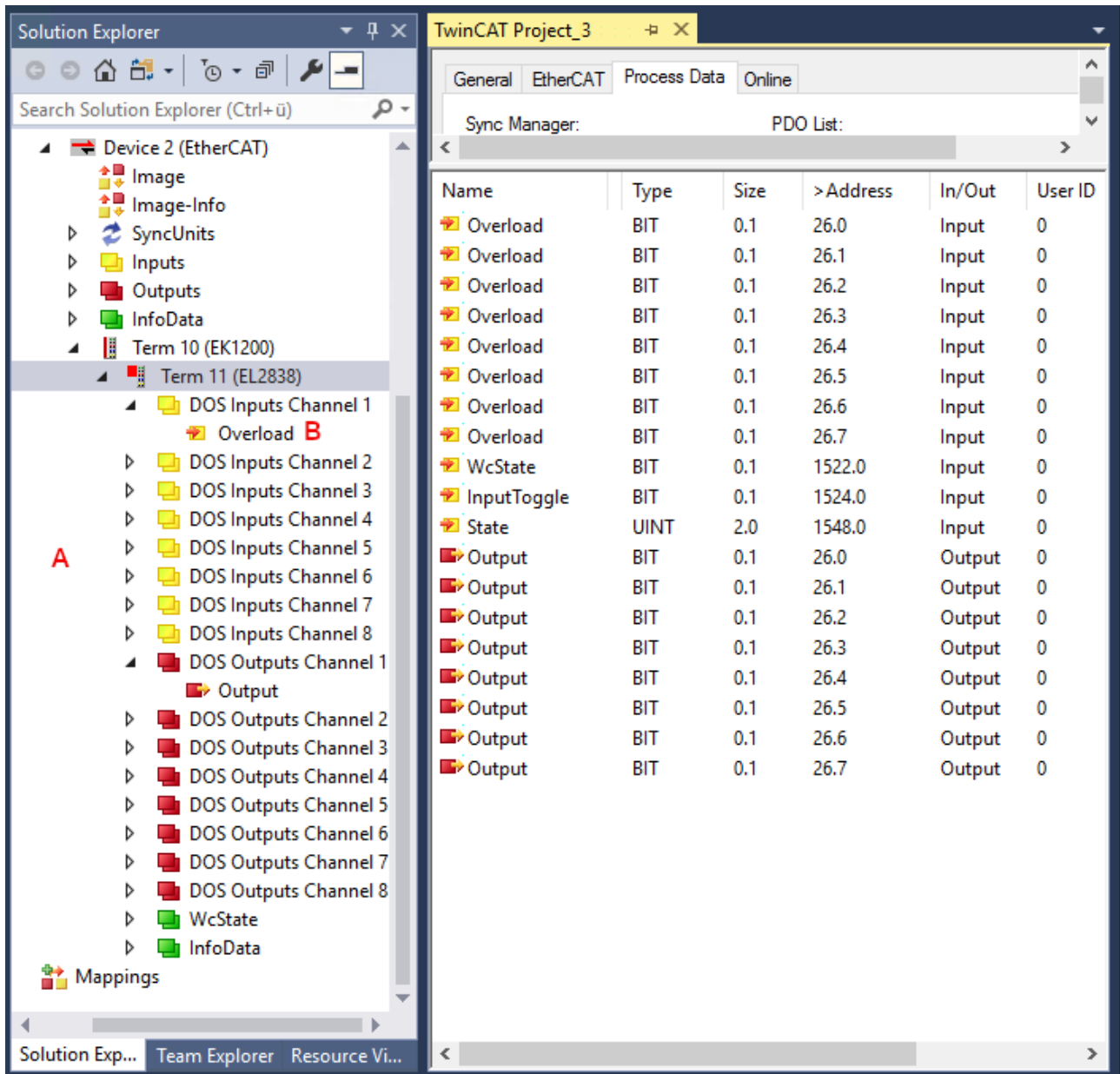
附图 12: 系统管理器中的过程数据和结构内容的 EL2838 在线说明
