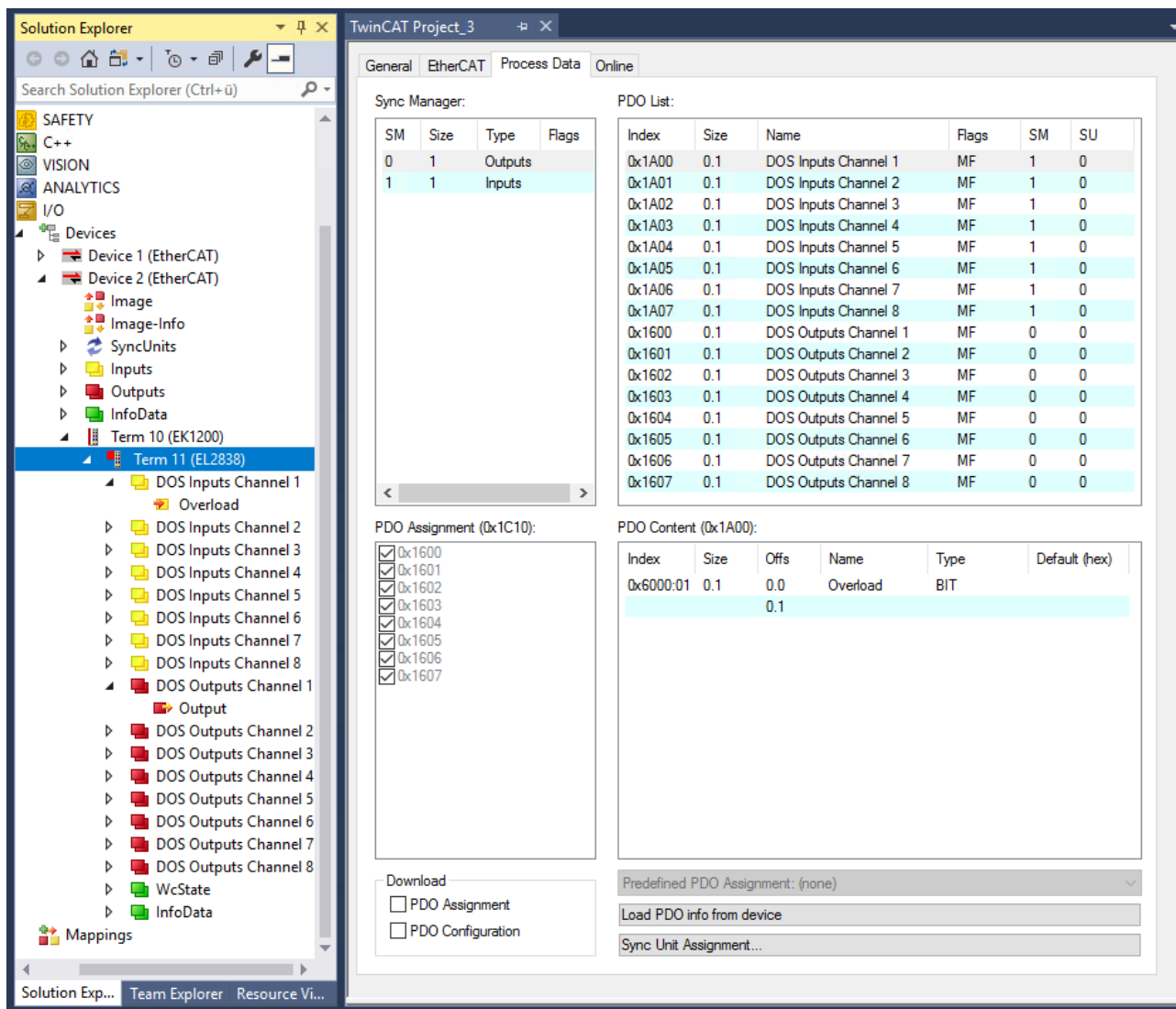
附图 11: EL2838 “过程数据”选项卡
