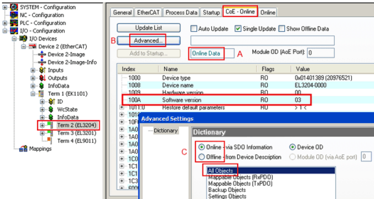
附图 145: EL3204 固件版本的显示
