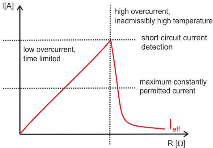
附图 8: 过载电流限制
