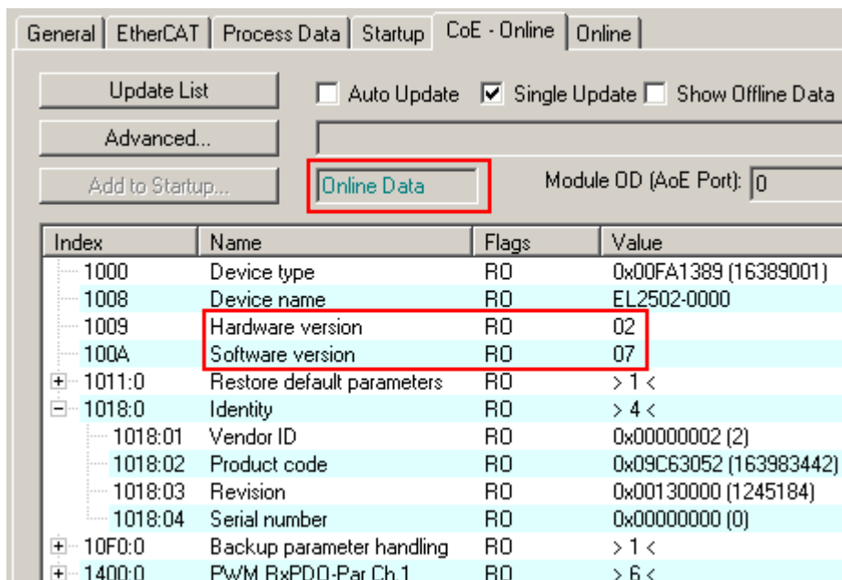
附图 19: 在线列表
