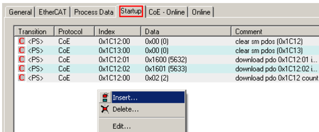
附图 17: TwinCAT System Manager 中的 Startup List
