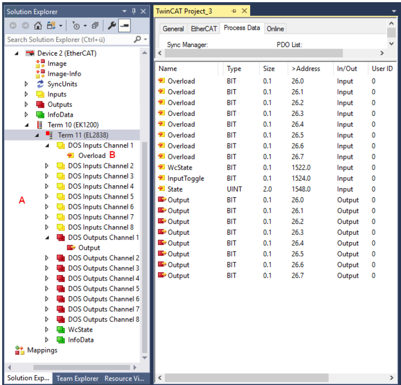
Abb. 12: EL2838 Online - Darstellung der Prozessdaten und Strukturinhalte im System Manager
