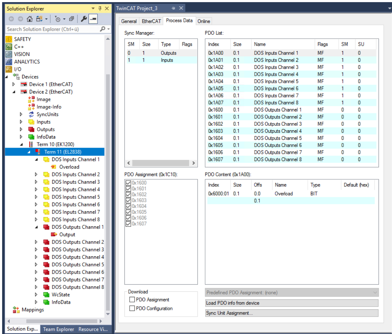
Abb. 11: EL2838 Reiter „Prozessdaten“
