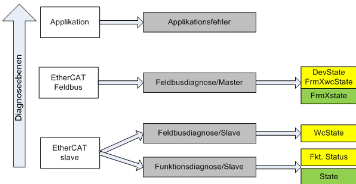
Abb. 130: Auswahl an Diagnoseinformationen eines EtherCAT-Slaves
