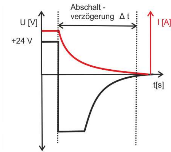
Abb. 10: Abschalten induktiver Lasten
