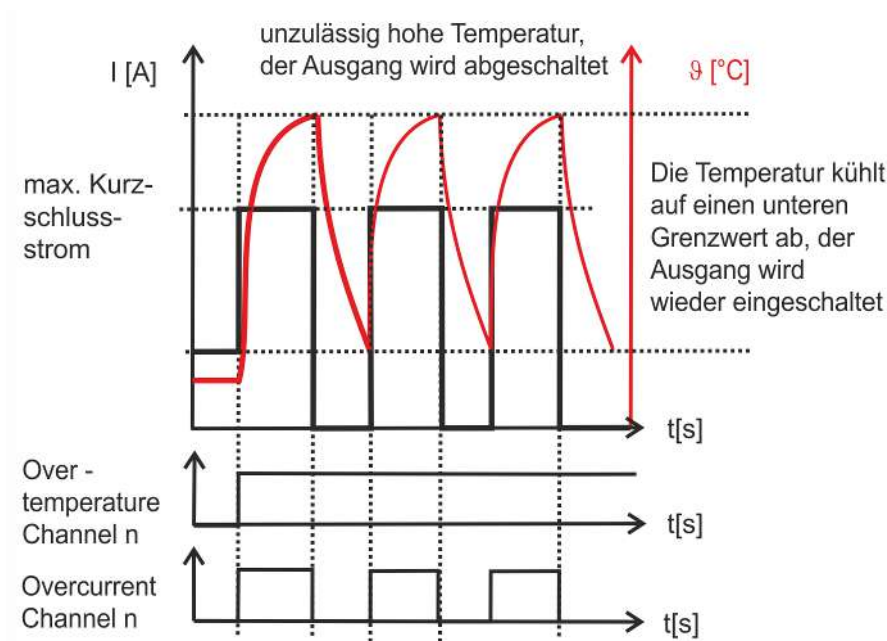
Abb. 9: Schematische Darstellung der thermischen Abschaltung bei Überlast
