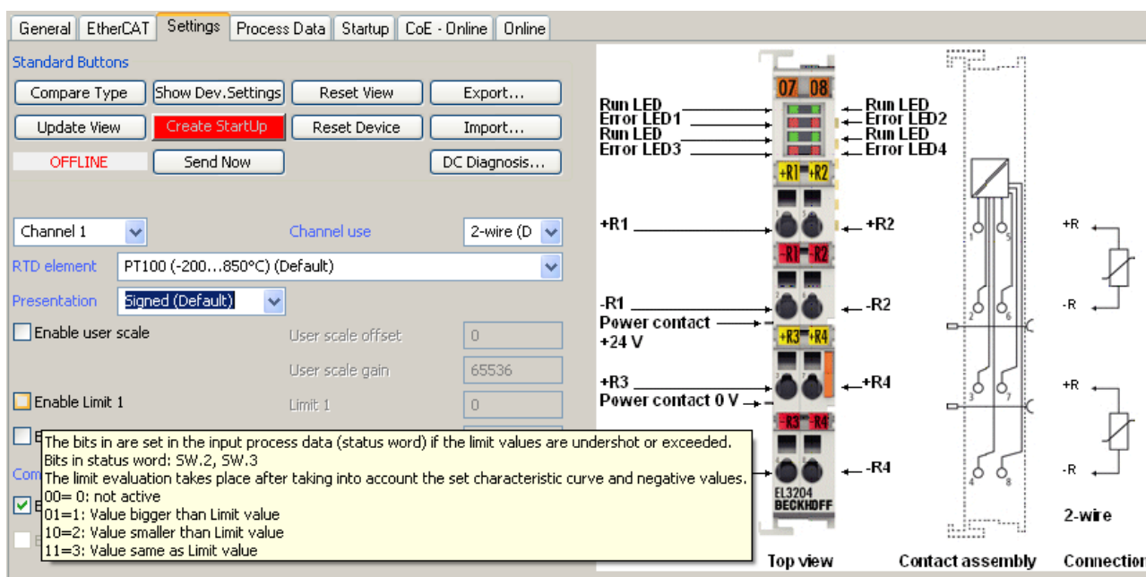
Abb. 133: Beispiel Inbetriebnahmehilfe für eine EL3204
