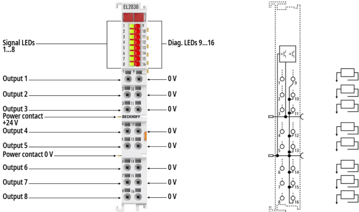
Abb. 7: EL2838
