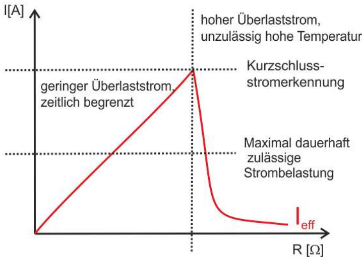
Abb. 8: Strombegrenzung bei Überlast
