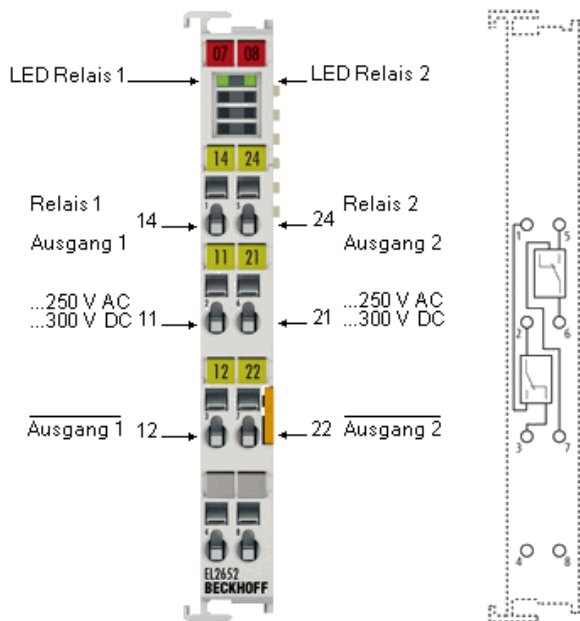
Abb. 13: EL2652
