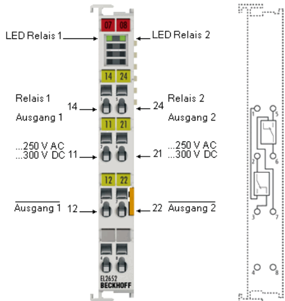
Abb. 12: EL2652
