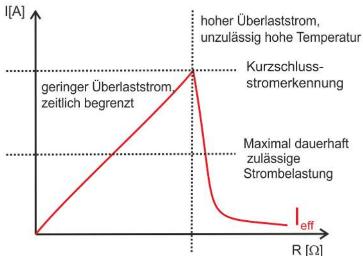
Abb. 9: Strombegrenzung bei Überlast
