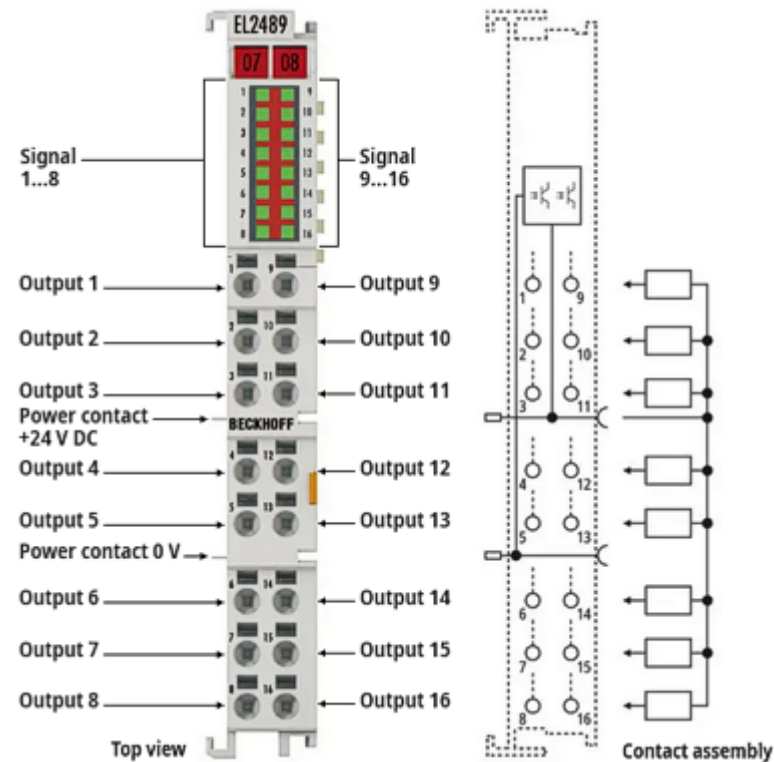
Abb. 8: EL2489
