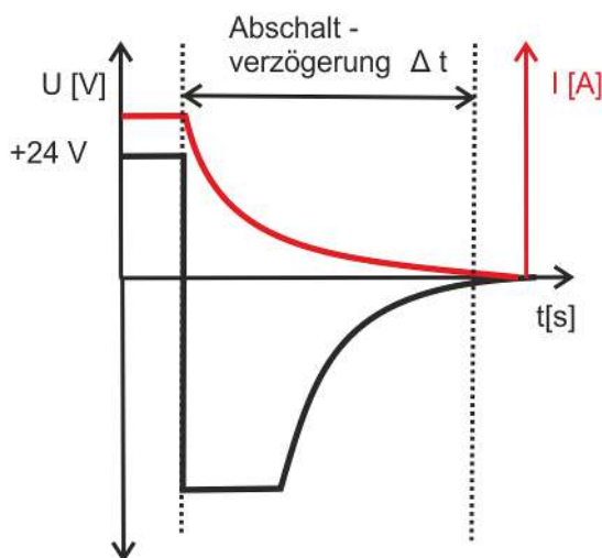
Abb. 10: Abschalten induktiver Lasten
