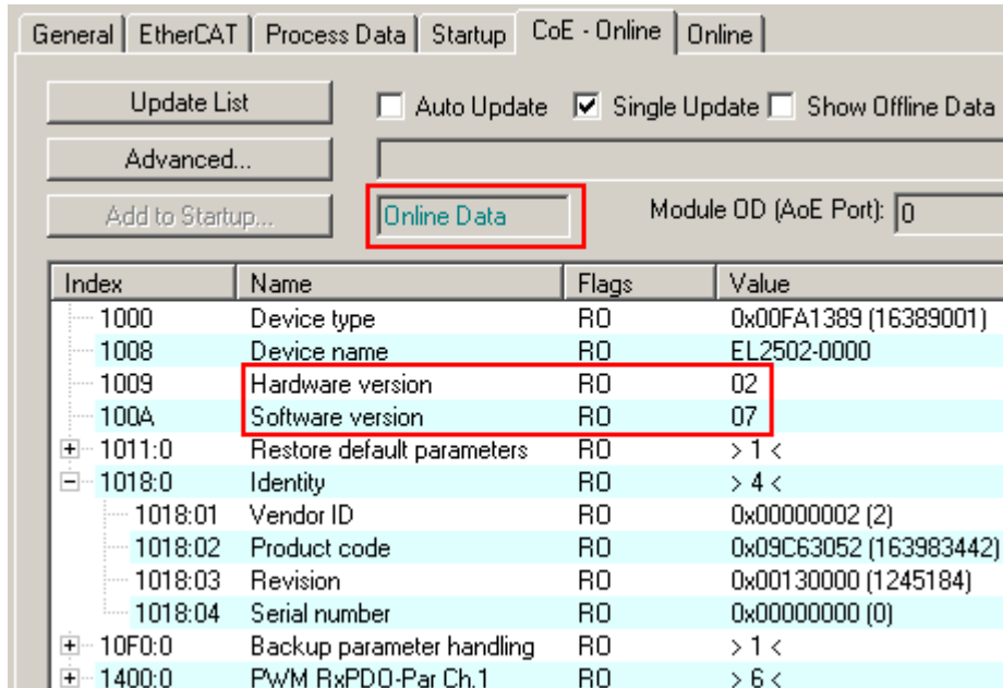
Abb. 17: Online-Verzeichnis
