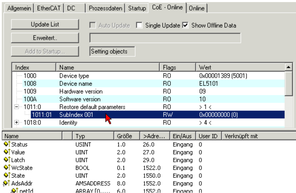
Abb. 154: Auswahl des PDO Restore default parameters
