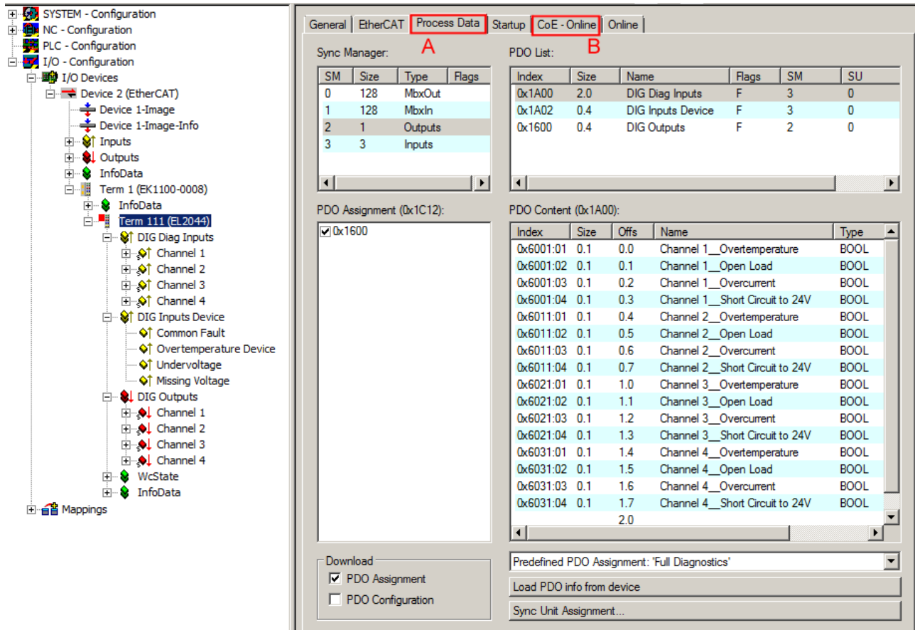
Abb. 9: EL2044 - Reiter „Prozessdaten“
