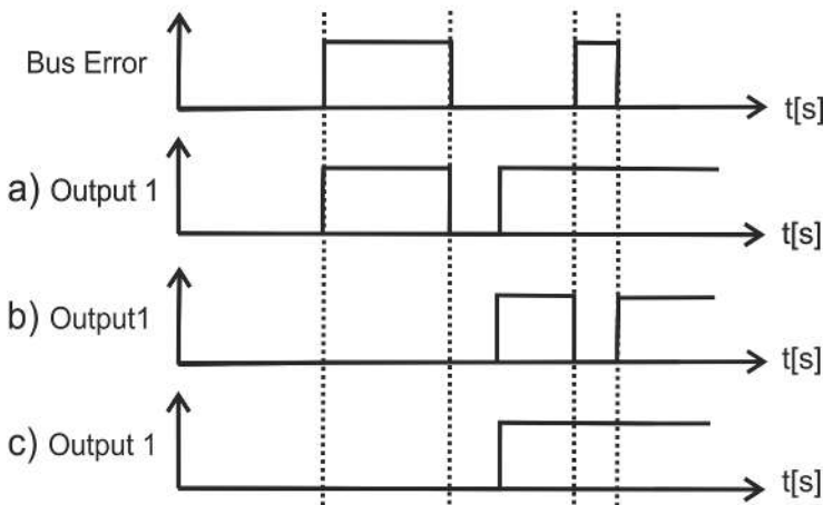
Abb. 14: graphische Darstellung des Kanalzustands bei Busstörung
