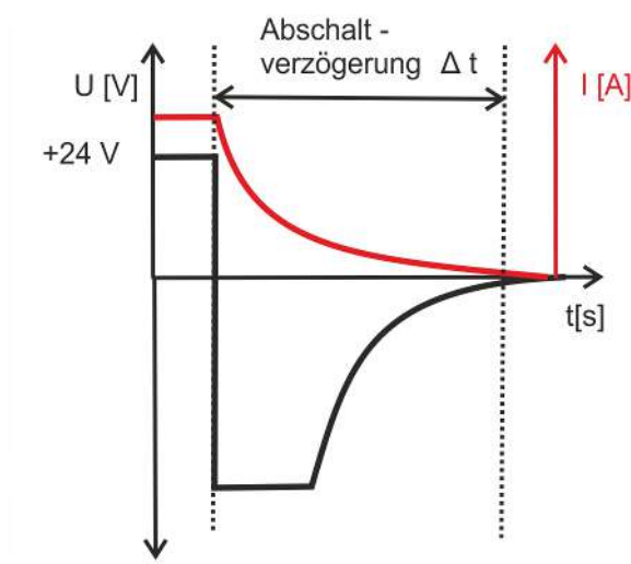
Abb. 8: Abschalten induktiver Lasten
