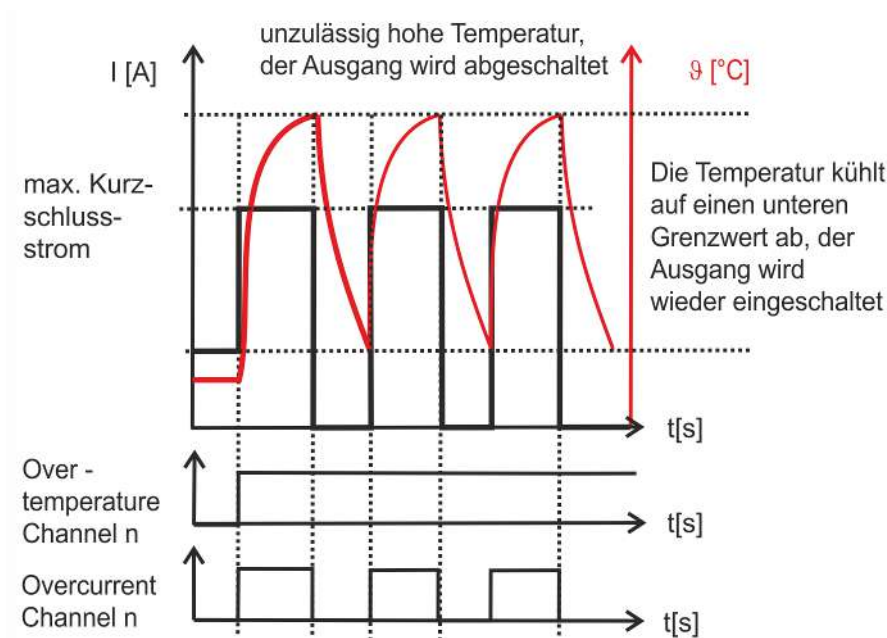
Abb. 7: Schematische Darstellung der thermischen Abschaltung bei Überlast
