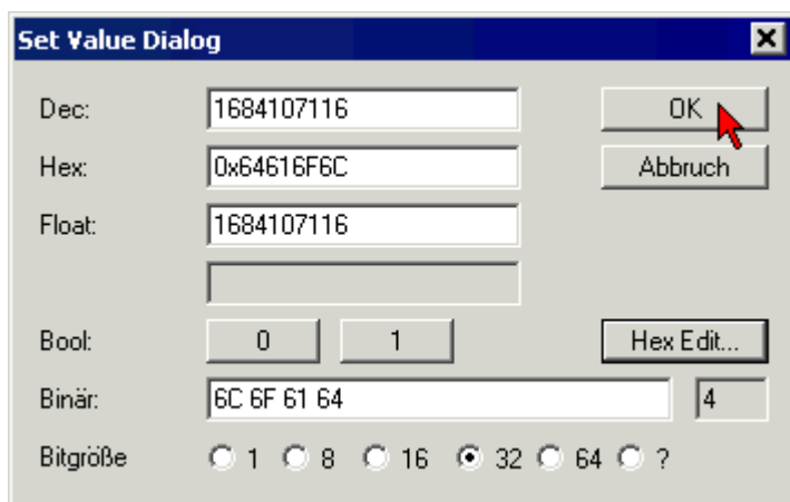
Abb. 155: Eingabe des Restore-Wertes im Set Value Dialog
