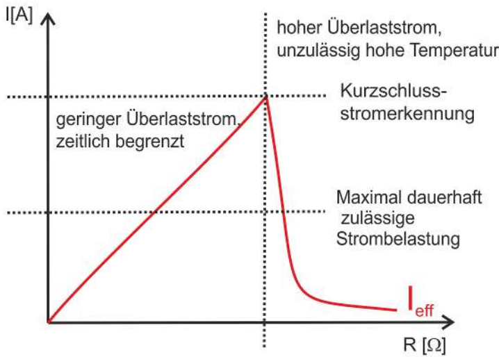
Abb. 6: Strombegrenzung bei Überlast
