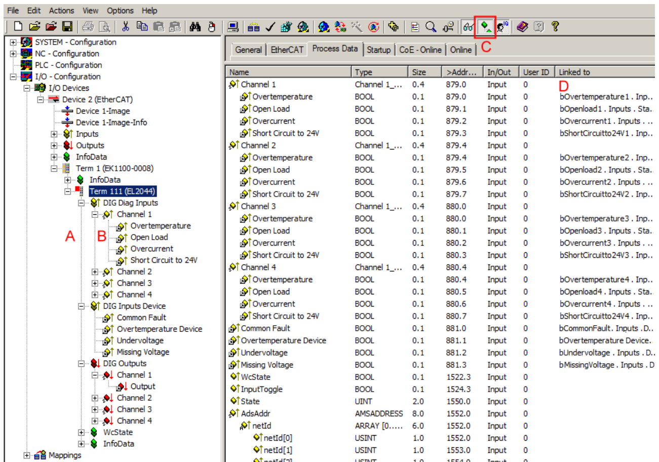
Abb. 10: EL2044 Online - Darstellung der Prozessdaten und Strukturinhalte im System Manager
