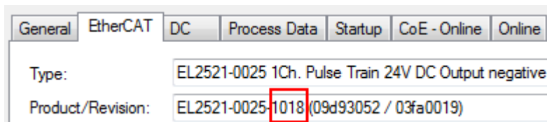
Abb. 107: Einbau EtherCAT-Klemme mit Revision -1018
