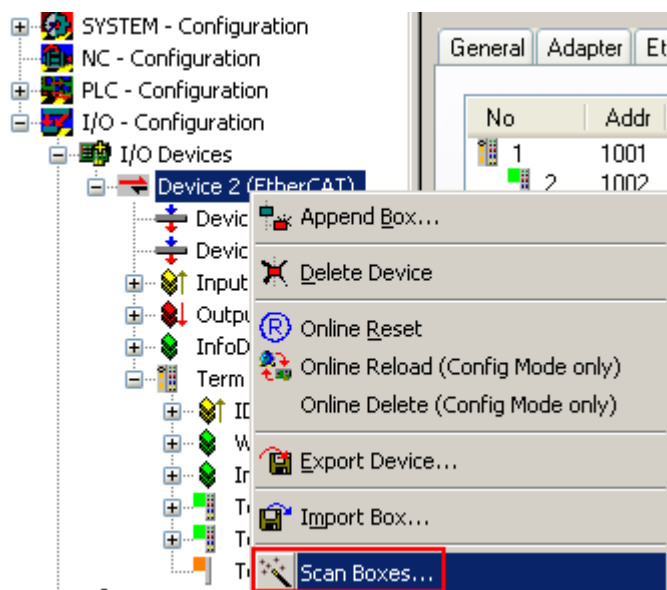
附图 138: 右键单击 EtherCAT Device 扫描下级从站
