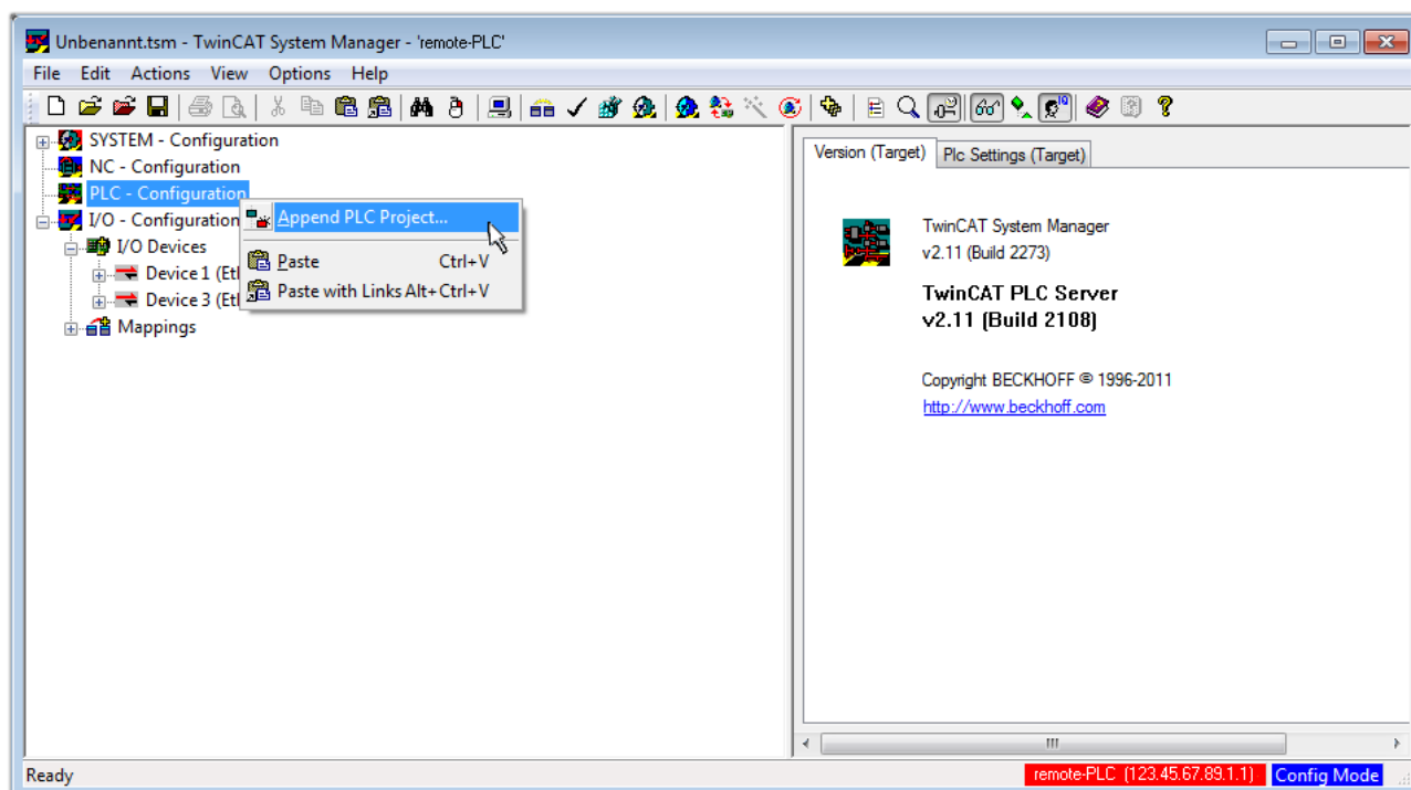
附图 38: 添加 TwinCAT PLC Control 项目
