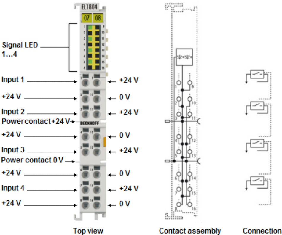
附图 4: EL1804, EL1814
