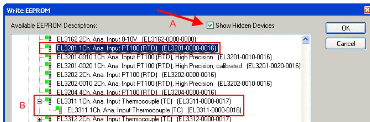
附图 142: 选择新的 ESI
