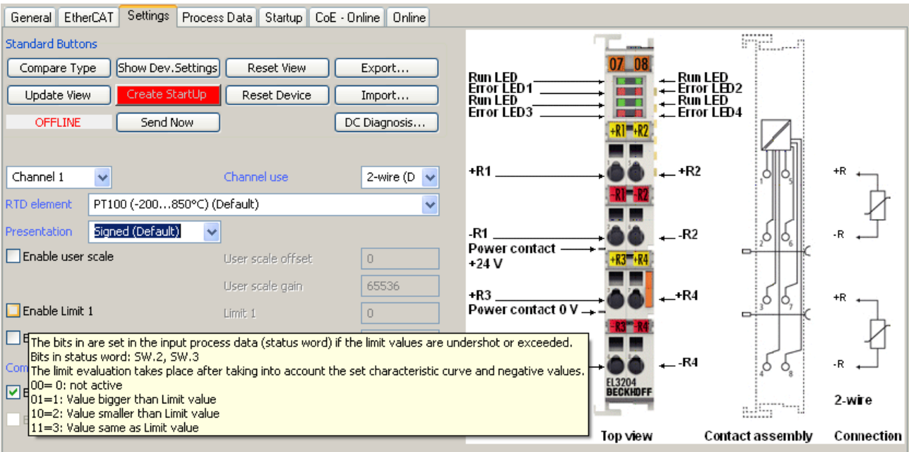
附图 131: EL3204 调试助手示例
