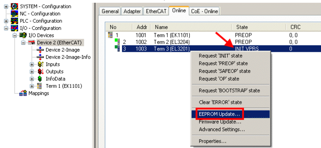
附图 141: EEPROM 更新
