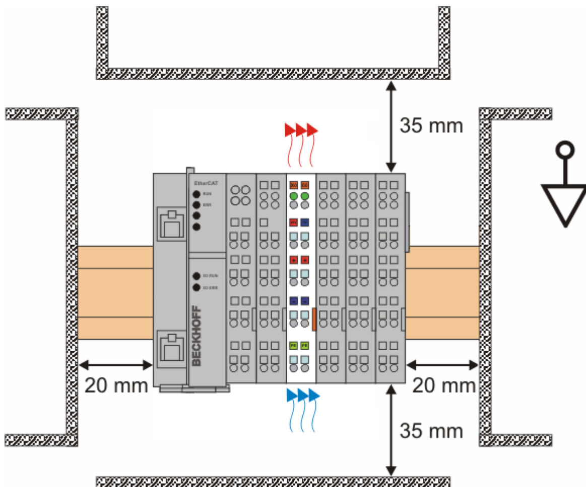
附图 19: 标准安装位置的推荐距离
