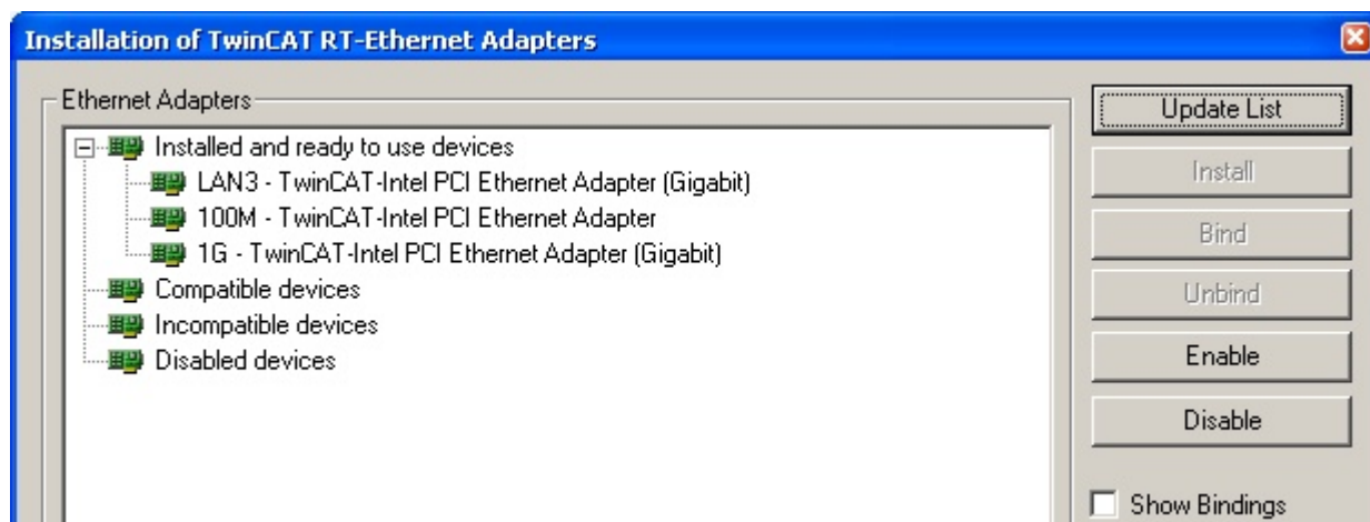
附图 72: 网络接口概览
