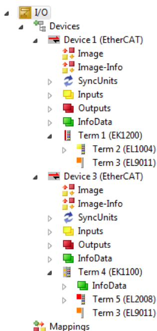
附图 53: 在集成于 VS shell 的TwinCAT 3 环境中配置映射
