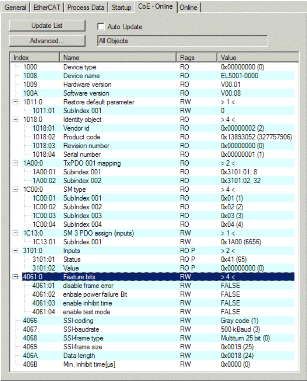
附图 124: “CoE - Online” 选项卡
