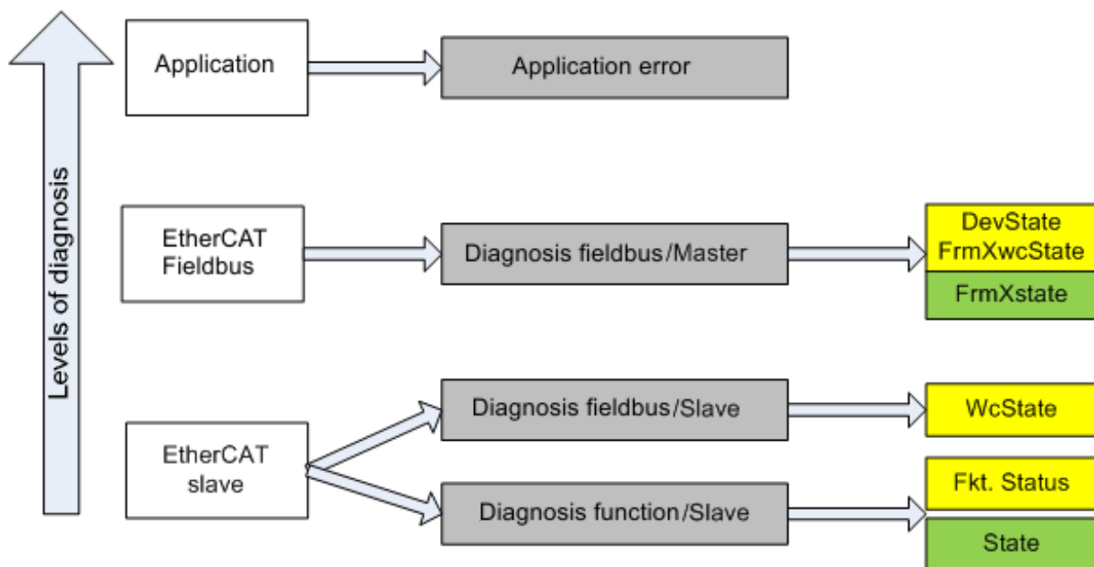
附图 128: 选择 EtherCAT 从站的诊断信息
