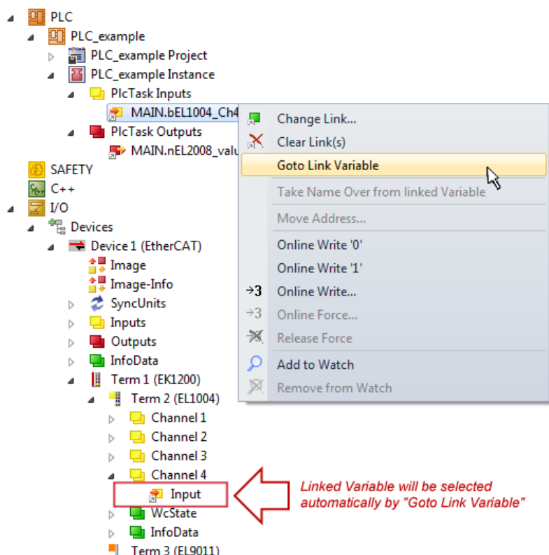
附图 63: “Goto Link Variable” 的应用, 以 “MAIN.bEL1004_Ch4” 为例
