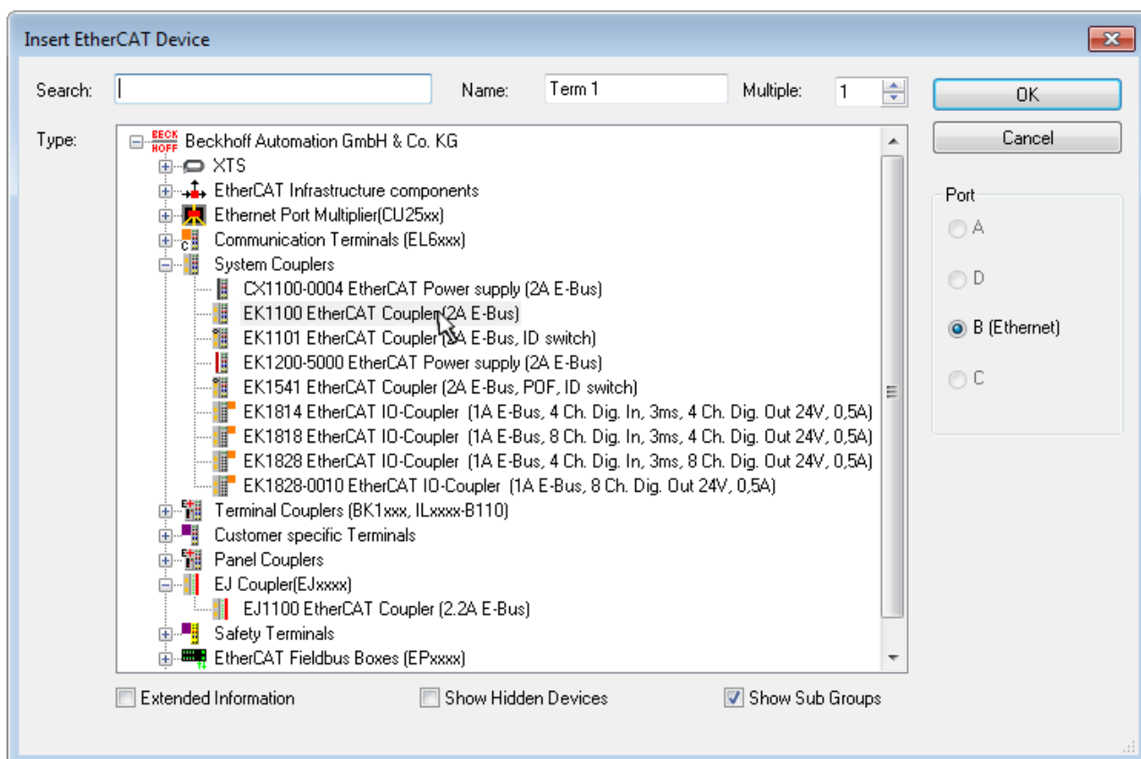
附图 92: 新增 EtherCAT 设备的选择对话框
