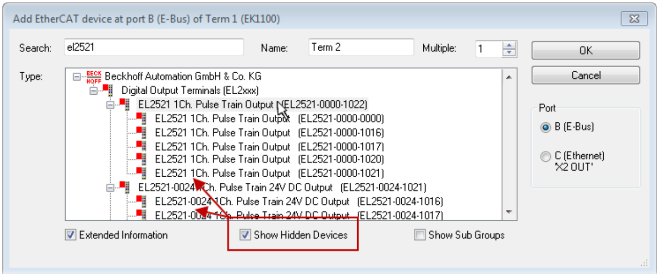
附图 94: 显示以前的版本
