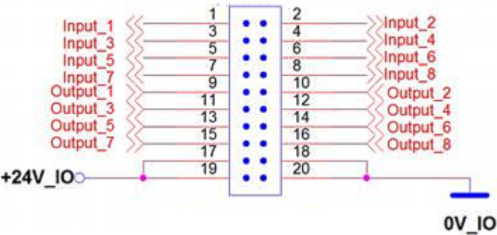
附图 8: 连接器引脚分配
