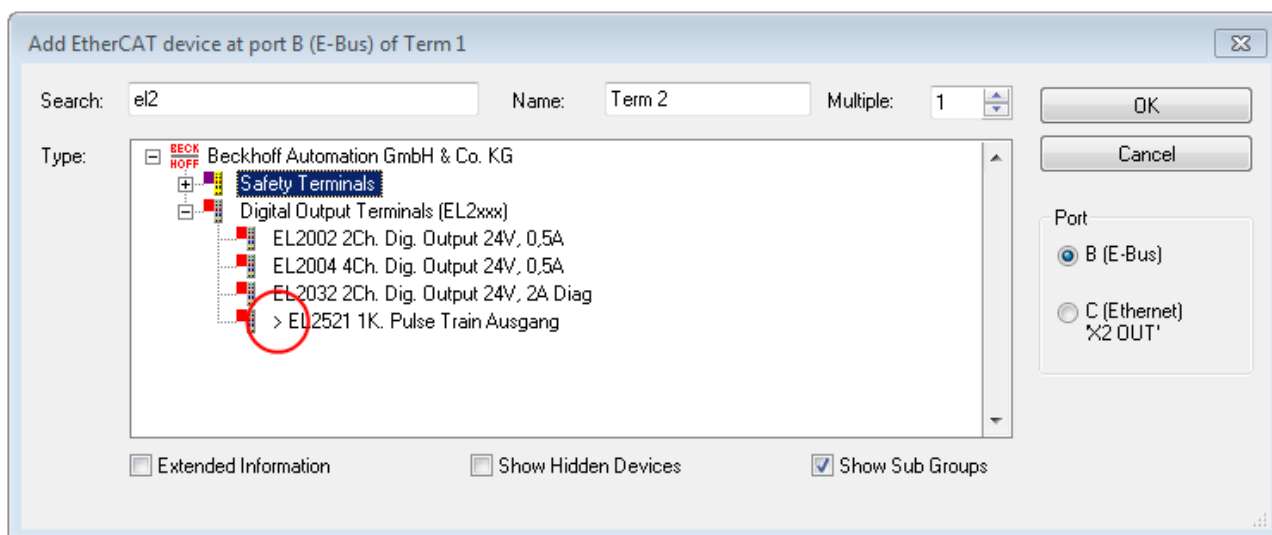
附图 82: 以EL2521为例说明用在线 ESI 文件创建的从站
