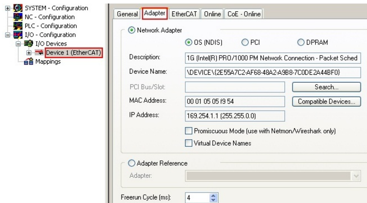
附图 90: EtherCAT 设备属性（TwinCAT 2）
