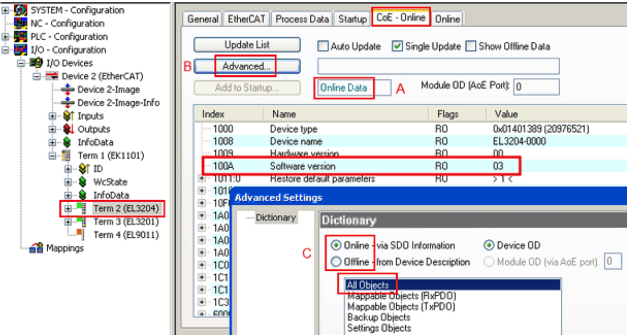
附图 143: EL3204 固件版本的显示
