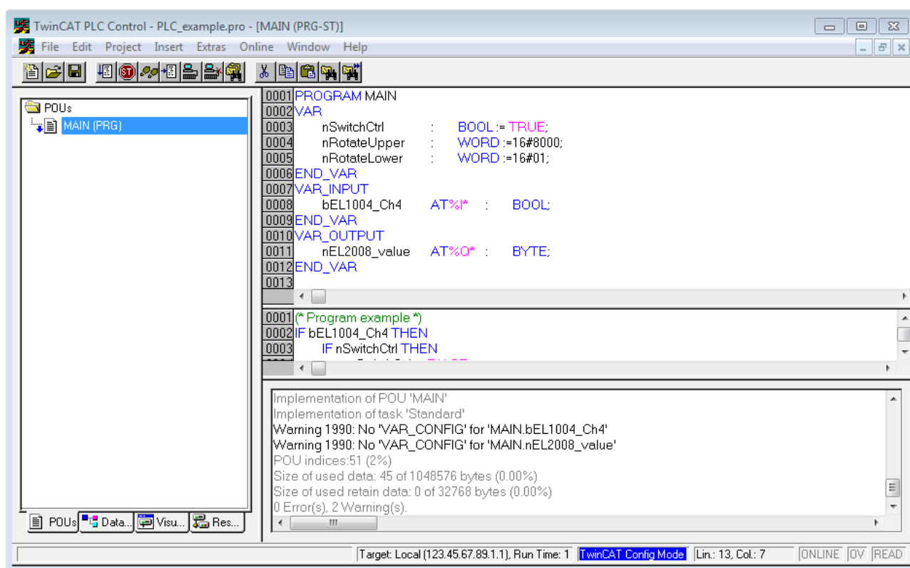
附图 37: 示例程序编译后，包含未分配地址的变量
