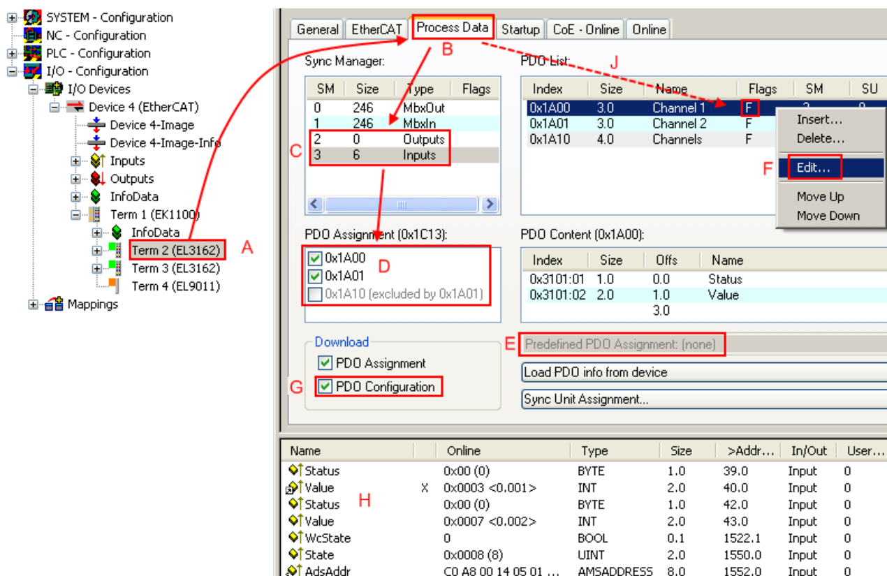
附图 122: 配置过程数据
