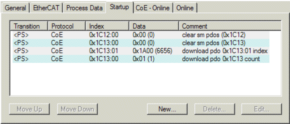
附图 123: “Startup (启动)” 选项卡
