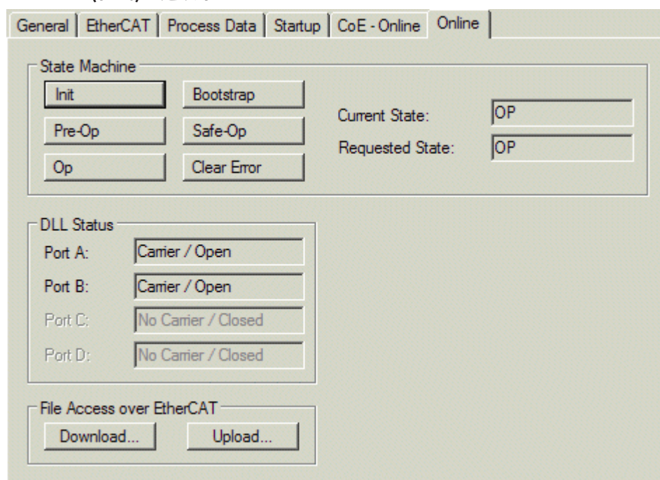
附图 126: “Online (在线)” 选项卡
