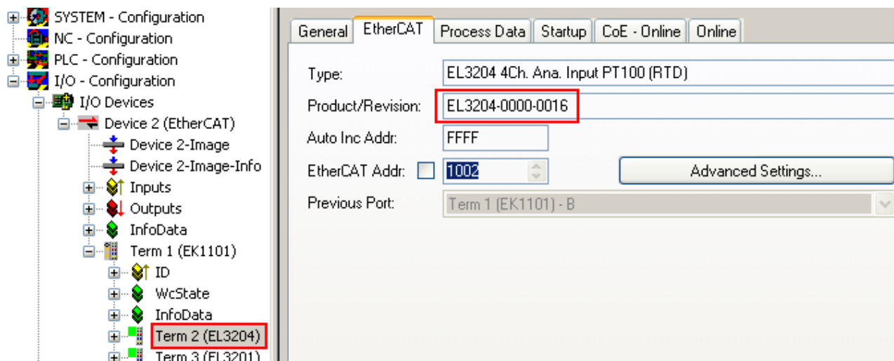
附图 137: 由名称 EL3204-0000 和修订版本号 0016 组成的设备标识符
