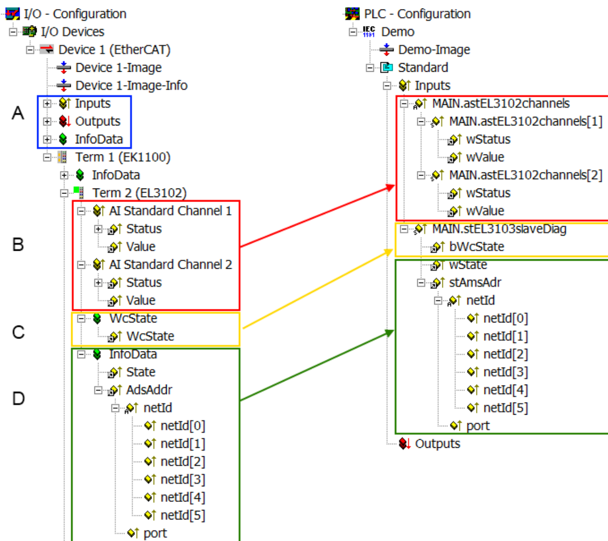
附图 129: PLC 中的 EtherCAT 从站基本诊断
