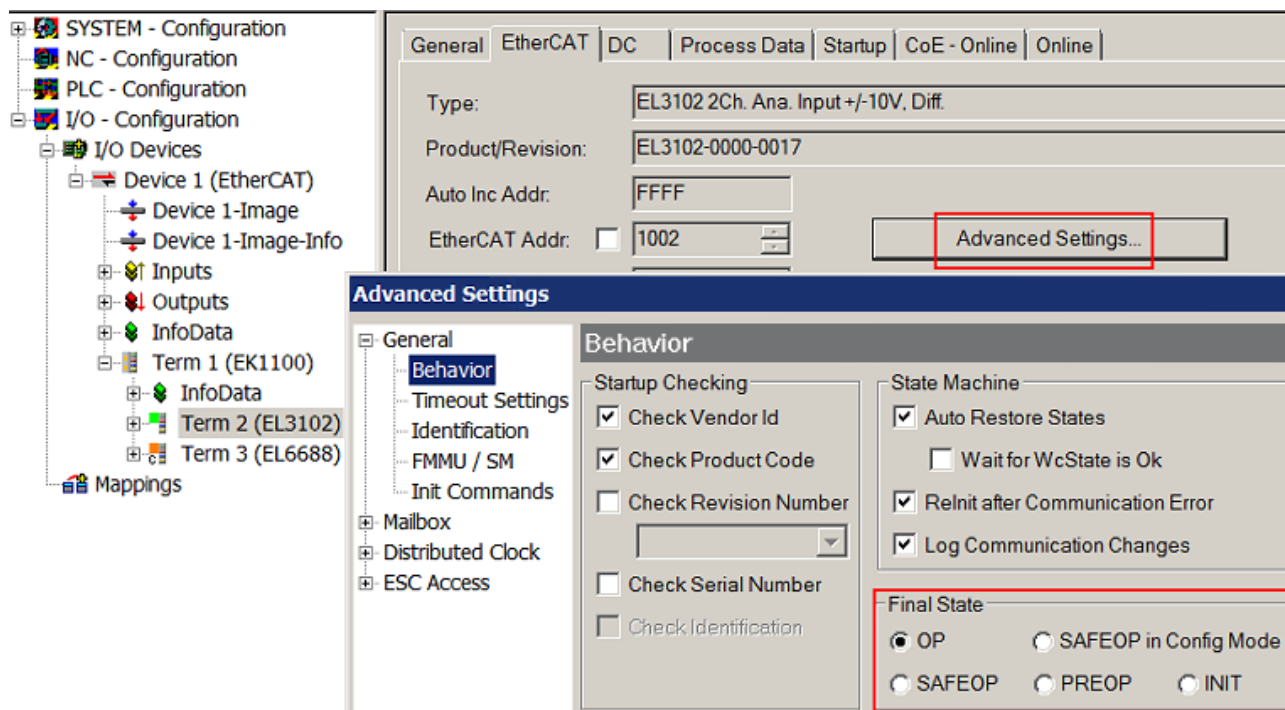
附图 133: 从站的默认目标状态
