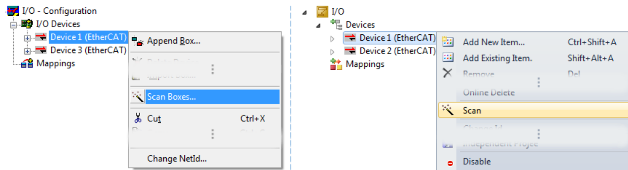
附图 105: 手动扫描特定 EtherCAT 主站上的设备（左：TwinCAT 2；右：TwinCAT 3）
