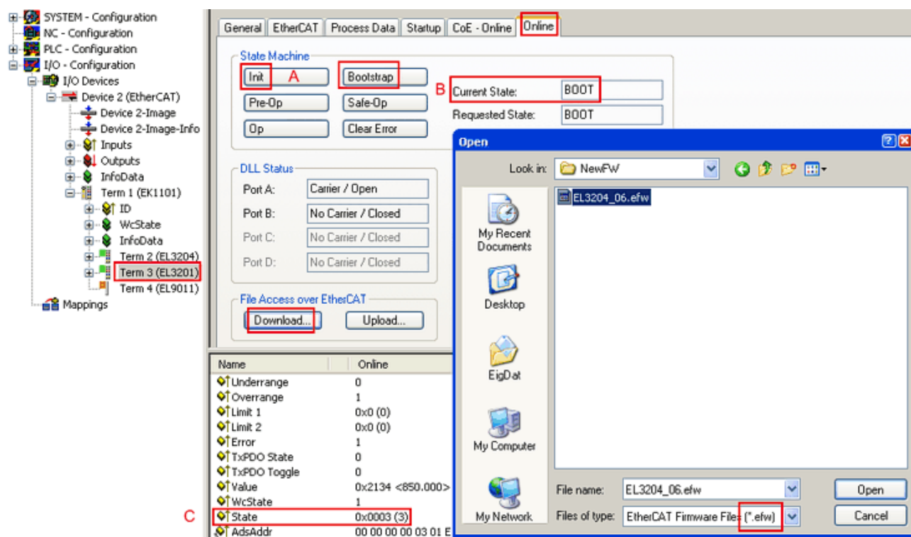
附图 144: 固件更新
