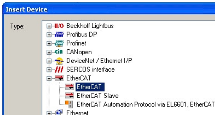
附图 88: 选择 EtherCAT 连接（TwinCAT 2.11, TwinCAT 3）
