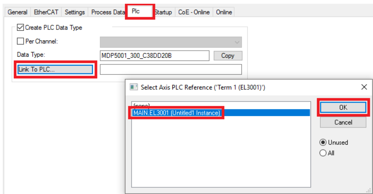
附图 66: 结构体的链接
