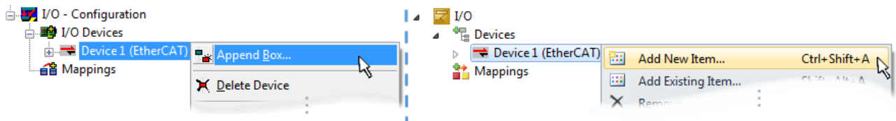
附图 84: 添加 EtherCAT 设备 (左: TwinCAT 2; 右: TwinCAT 3)
