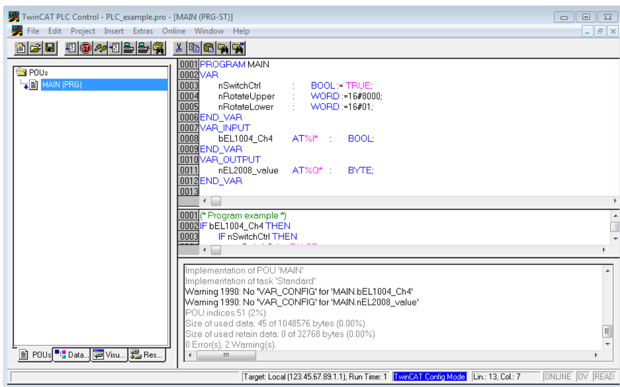
附图 31: 示例程序编译后，包含未分配地址的变量
