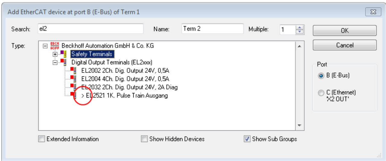
附图 76: 以EL2521为例说明用在线 ESI 文件创建的从站
