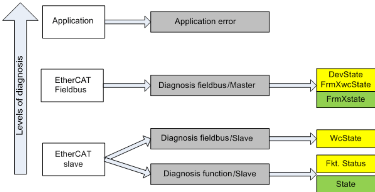
附图 121: 选择 EtherCAT 从站的诊断信息
