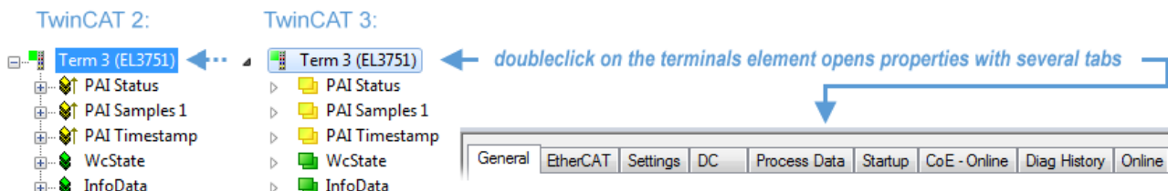
附图 112: 树形结构的分支, 端子模块 EL3751
