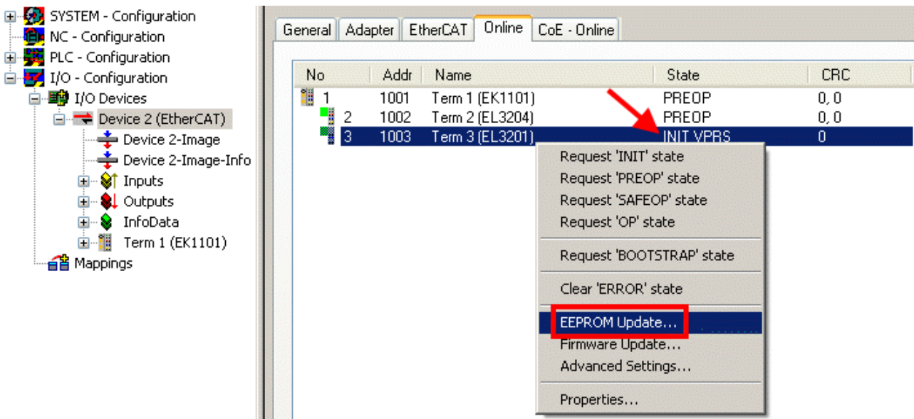
附图 135: EEPROM 更新
