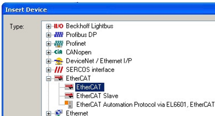
附图 82: 选择 EtherCAT 连接 (TwinCAT 2.11, TwinCAT 3)
