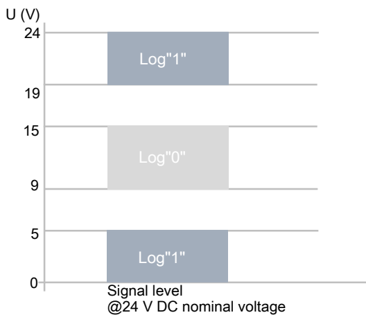
附图 5: 信号电压 “0” 和 “1” 的开关特性:
