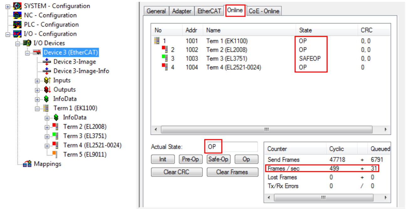
附图 104: 在线显示示例
