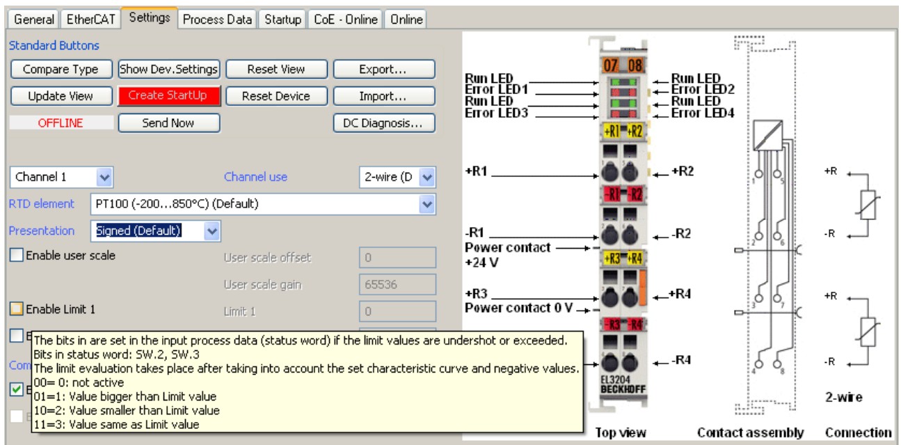
附图 125: EL3204 调试助手示例
