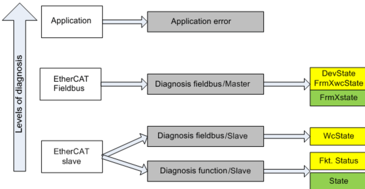
附图 122: 选择 EtherCAT 从站的诊断信息
