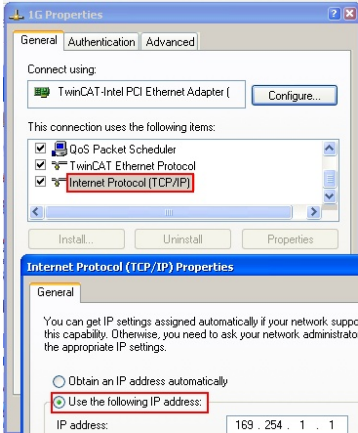
附图 71: 以太网端口的 TCP/IP 设置
