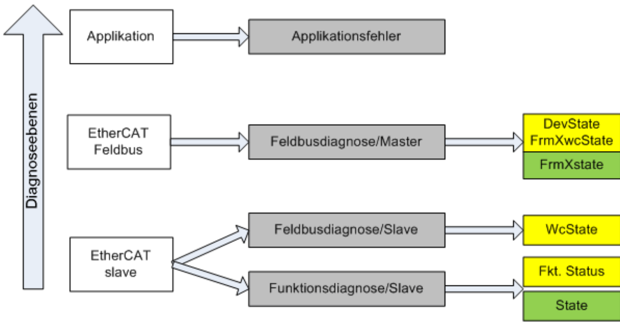
Abb. 122: Auswahl an Diagnoseinformationen eines EtherCAT-Slaves
