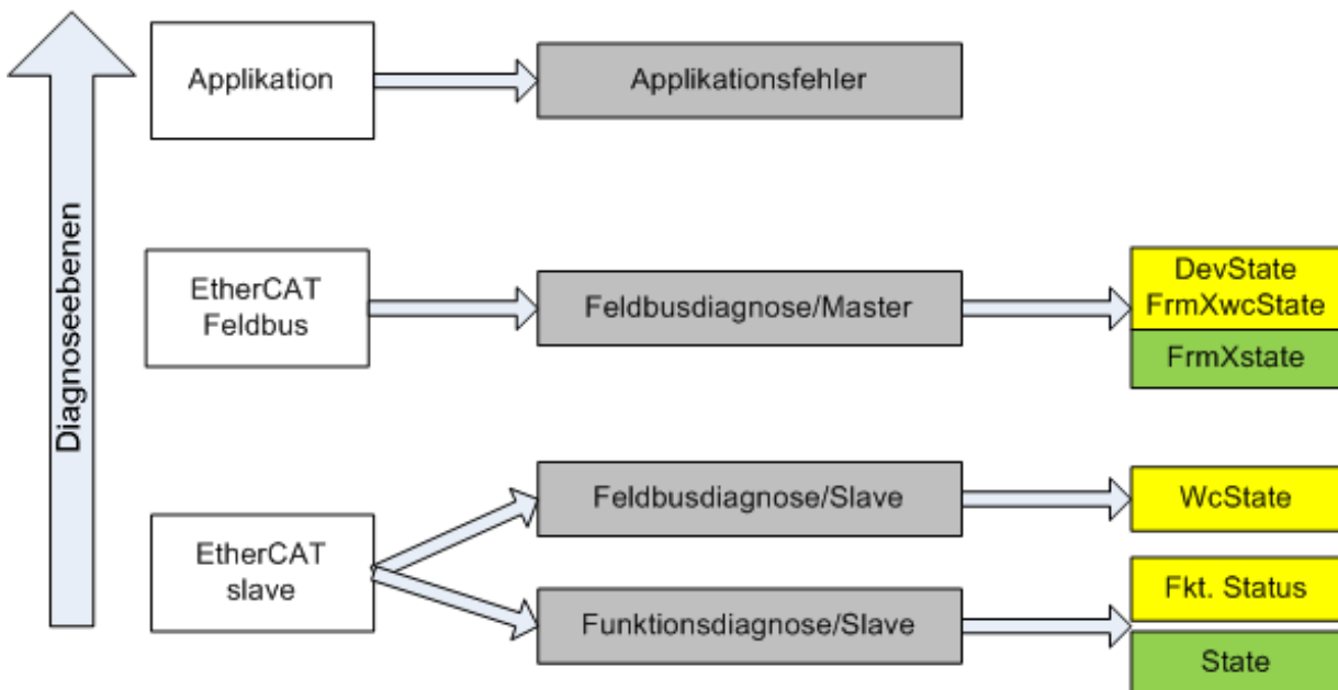
Abb. 125: Auswahl an Diagnoseinformationen eines EtherCAT-Slaves
