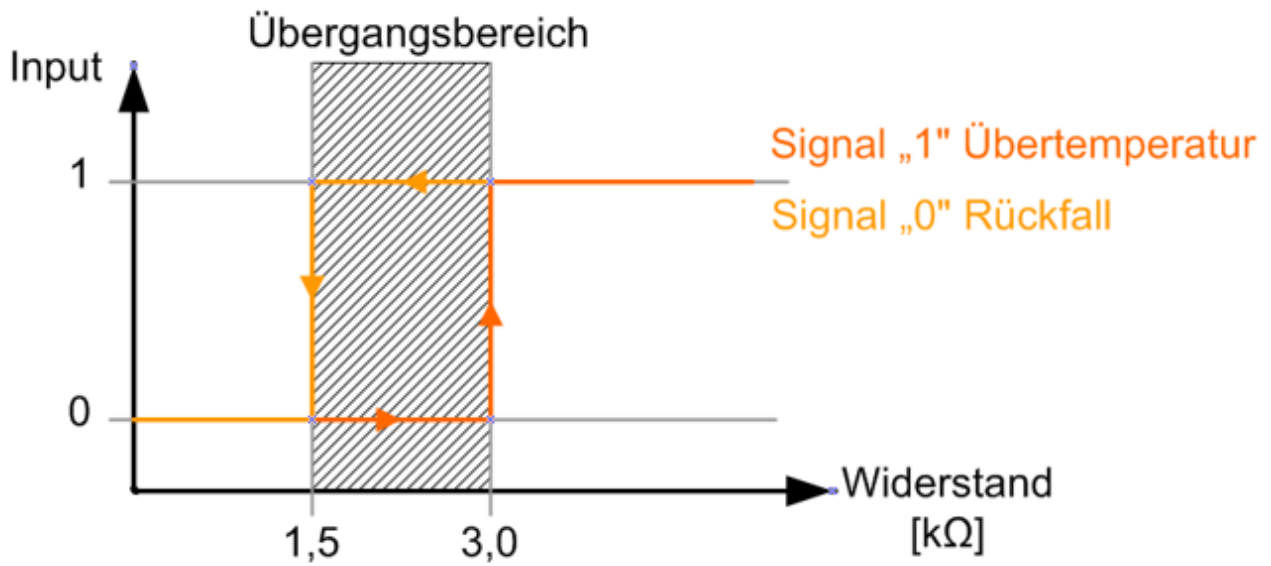
Abb. 135: Schaltverhalten
