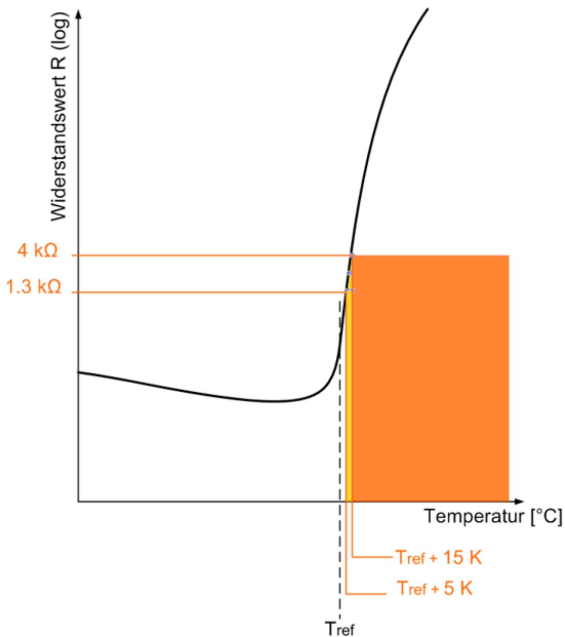
Abb. 134: Schematische Darstellung der Widerstandskennlinie von Thermistorsensoren
