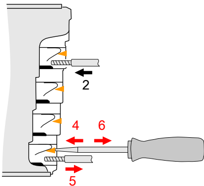
Abb. 20: Anschließen und Lösen der Leiter
