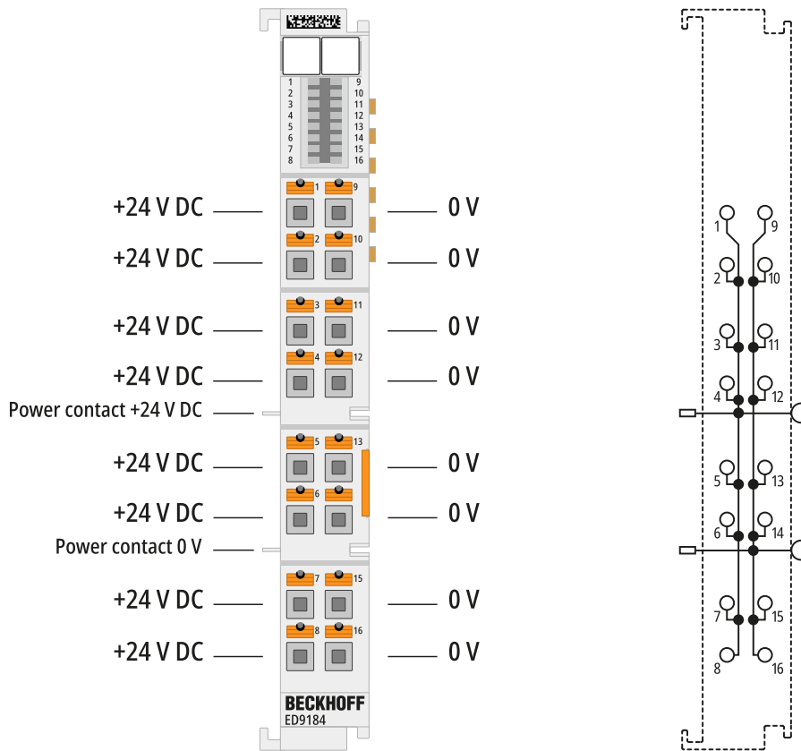
Abb. 5: ED9184
