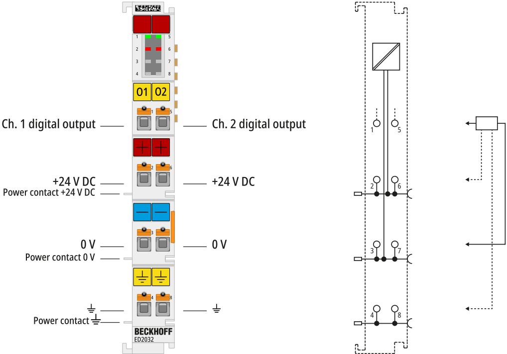
Abb. 4: ED2032 - Anschlussbelegung
