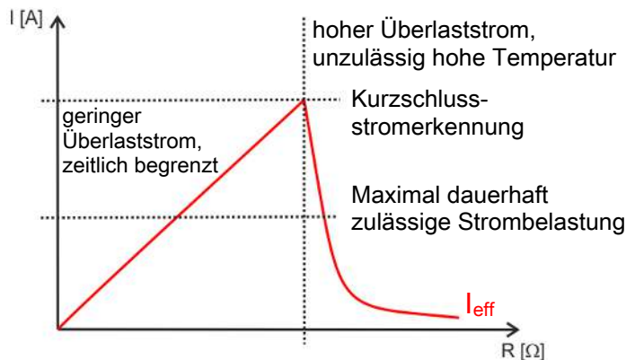
Abb. 20: Strombegrenzung bei Überlast
