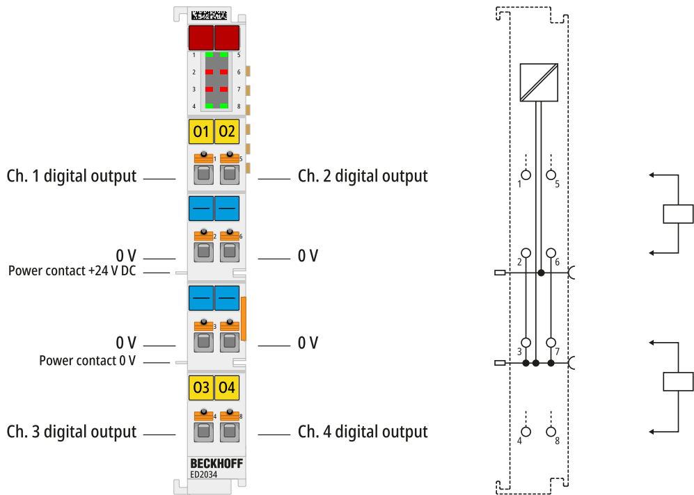
Abb. 5: ED2034 - Anschlussbelegung
