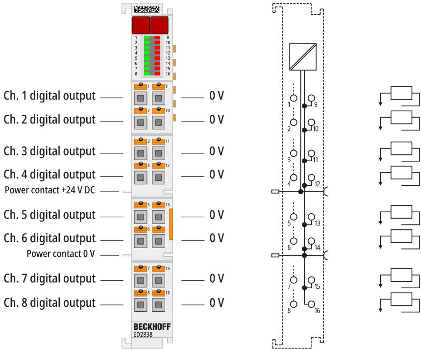
Abb. 6: ED2838 - Anschlussbelegung
