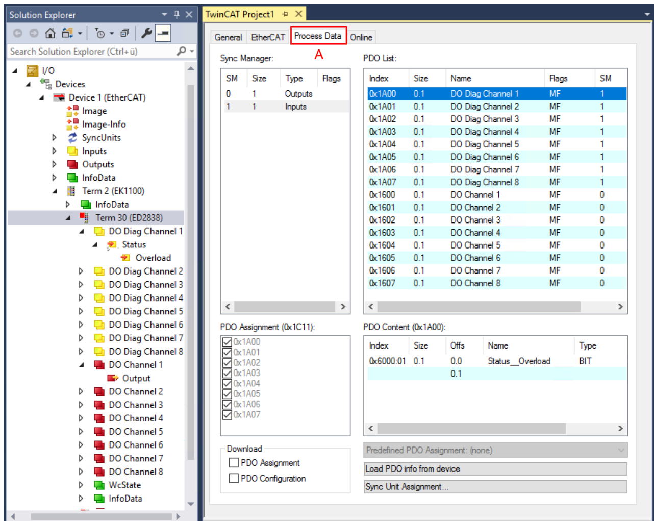
Abb. 23: Reiter „Process data“ am Beispiel ED2838
