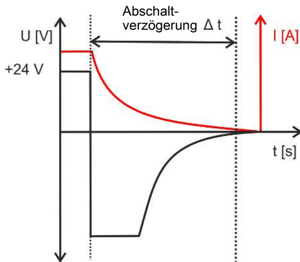
Abb. 22: Abschalten induktiver Lasten
