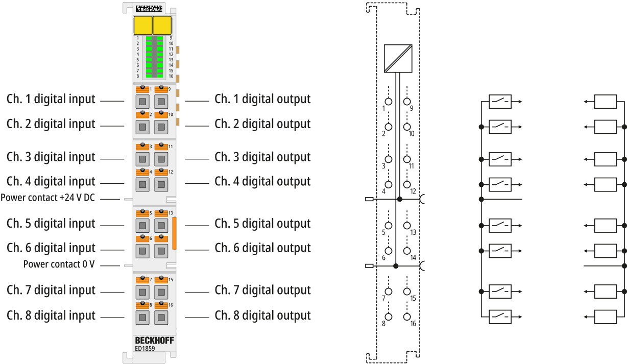
Abb. 4: ED1859 - Anschlussbelegung
