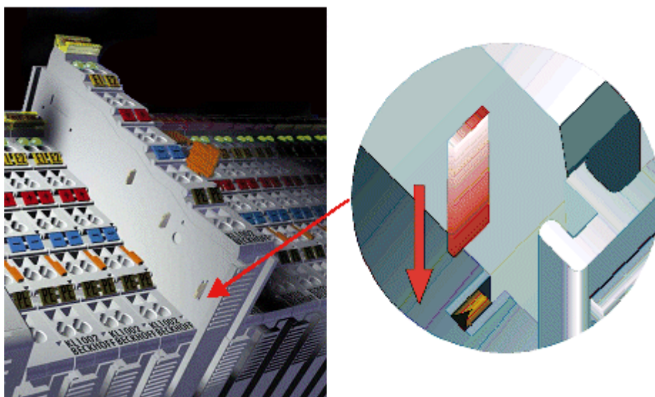
Abb. 8: Linksseitiger Powerkontakt
