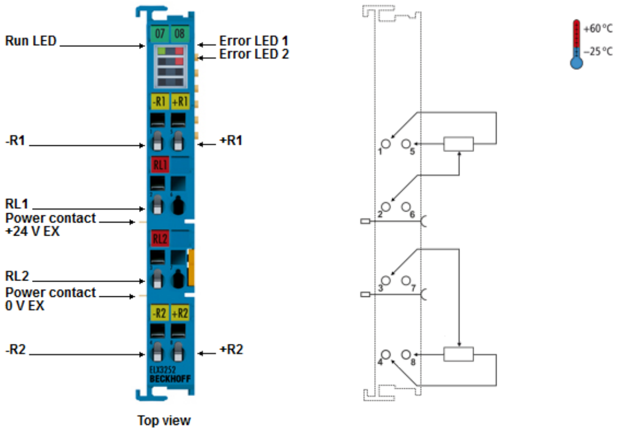
附图 20: ELX3252 - 触点分配
