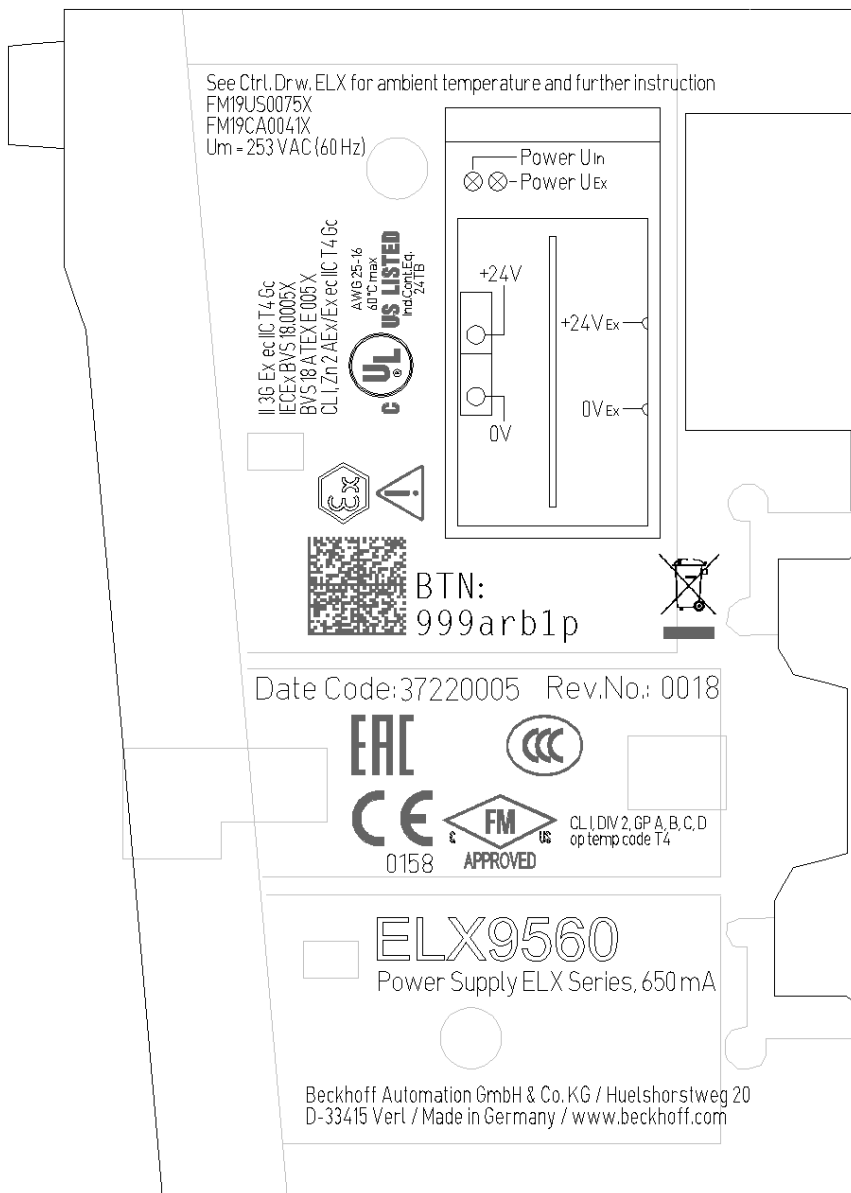
附图 2: ELX9560-0000, 日期代码 37220005, BTN 999arb1p 和防爆标识
