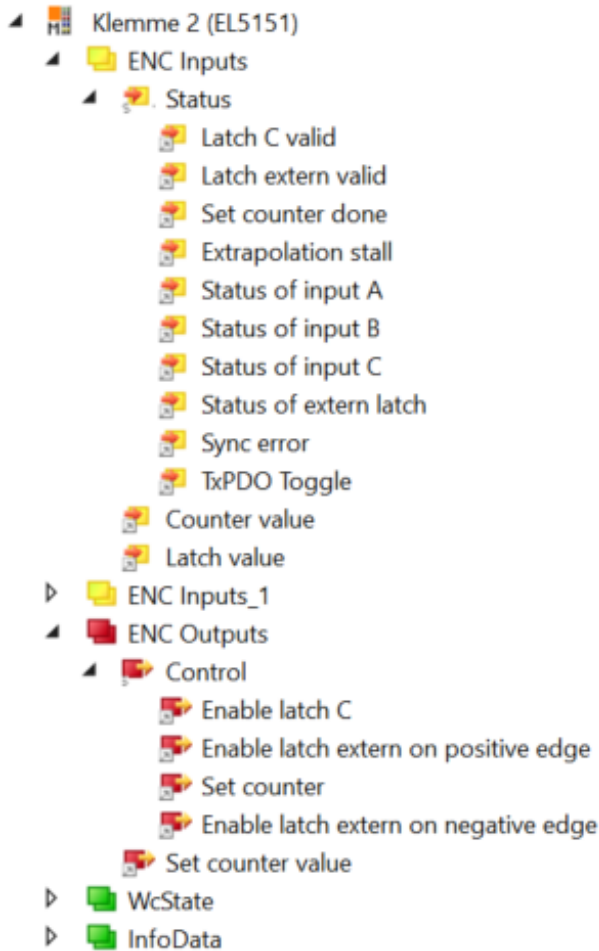
Abb. 141: Verknüpfte Ein- und Ausgänge der EL5151 mit der NC-Task
