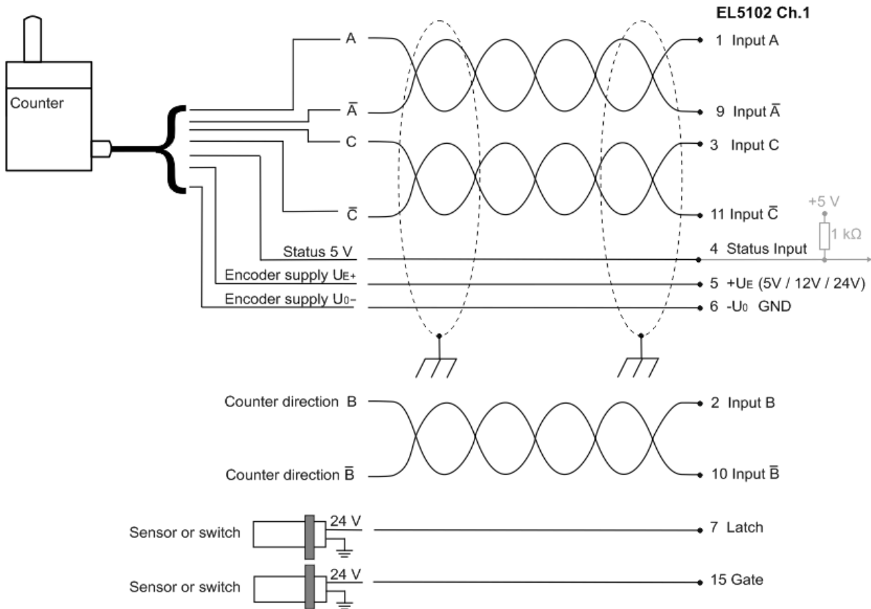
Abb. 29: Anschluss Zähler / Impulsgeber RS422 - Mode mit Nullimpuls
