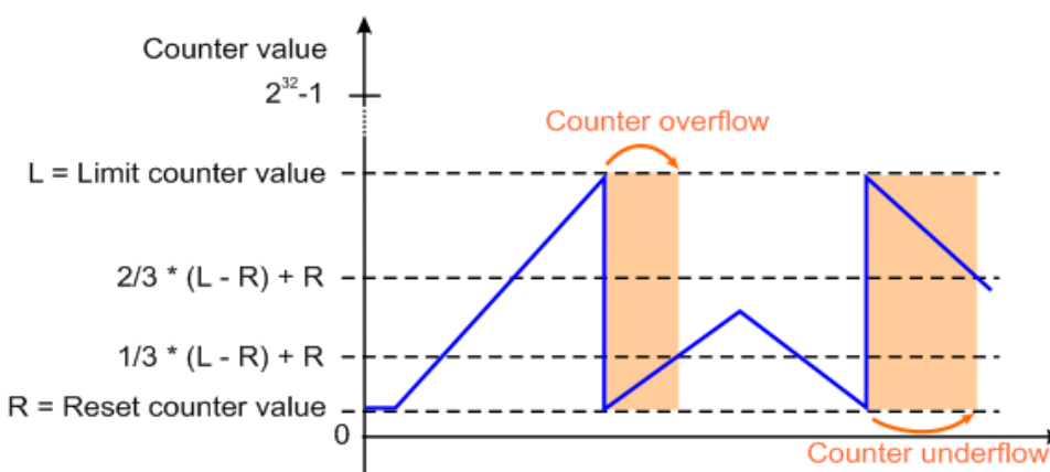
Abb. 154: Über- und Unterschreiten der Zählergrenzen mit festgelegtem Wertebereich
