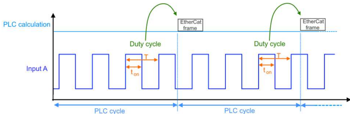
Abb. 164: Duty Cycle Messung
