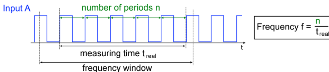
Abb. 160: Frequenzmessung - „Frequency value“
