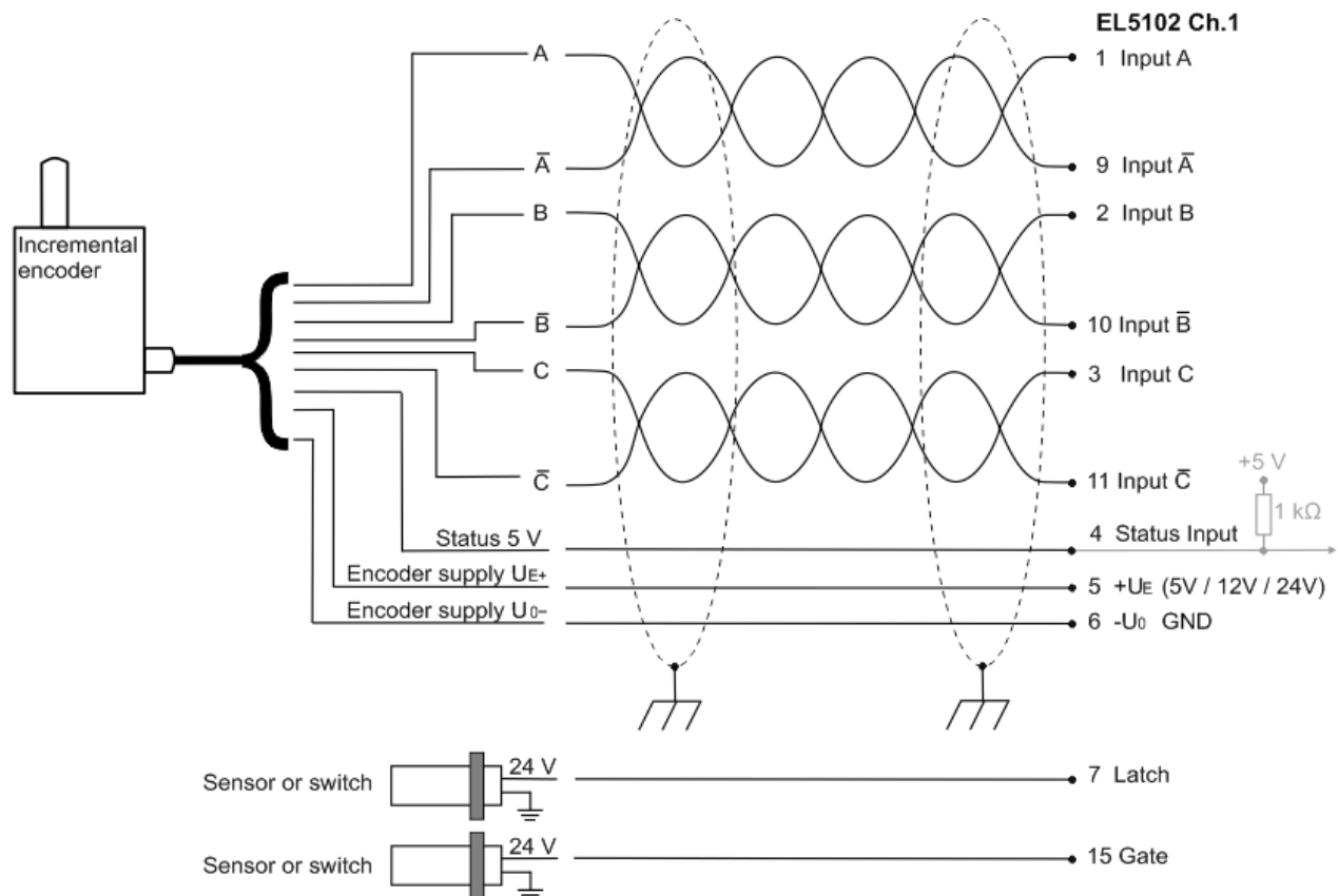
Abb. 28: Anschluss Encoder RS422 - Mode mit Nullimpuls
