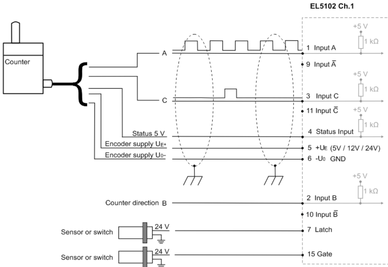
Abb. 33: Anschluss Zähler / Impulsgeber Open Collector - Mode mit Nullimpuls
