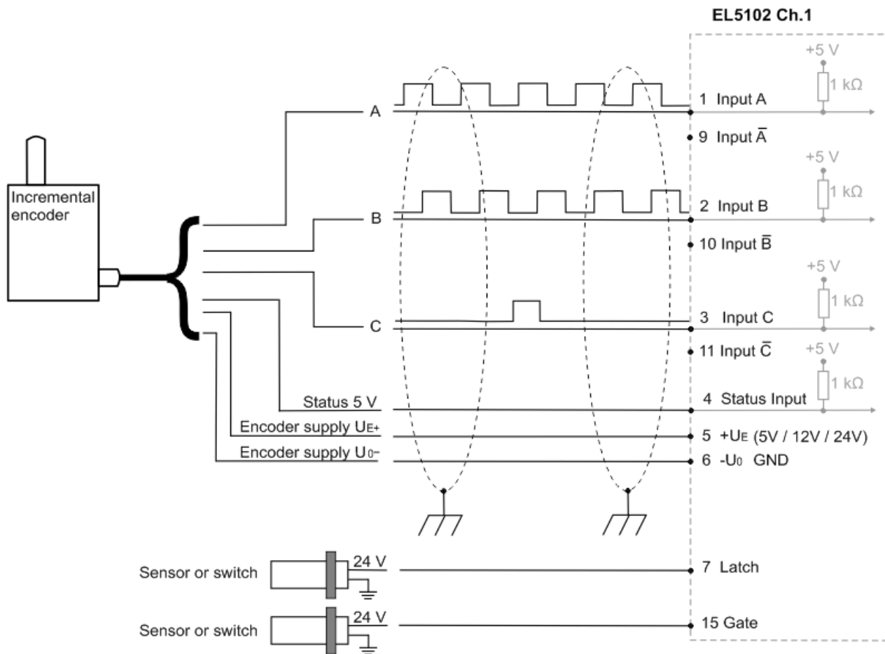
Abb. 32: Anschluss Encoder Open Collector - Mode mit Nullimpuls
