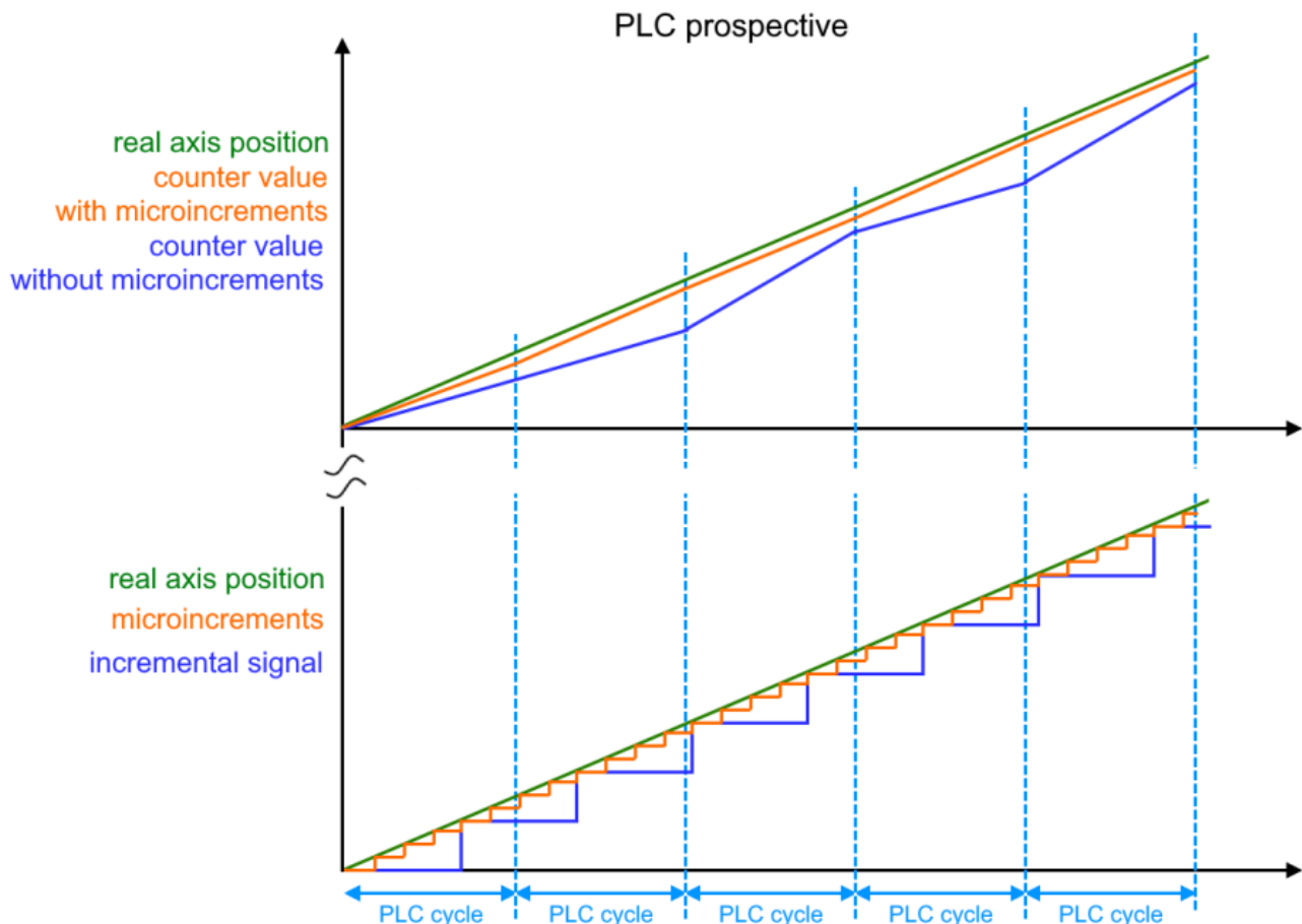
Abb. 165: Funktionsprinzip Mikroinkremente
