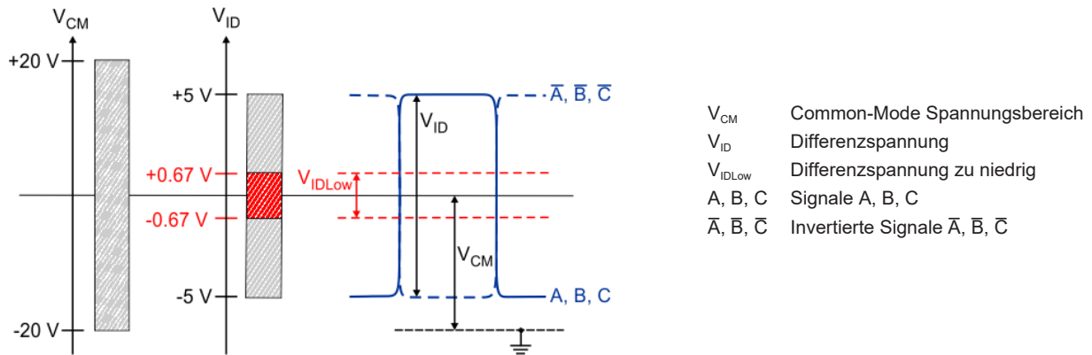
RS422 Signalpegel
