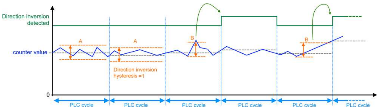
Abb. 159: Stillstandsüberwachung mit Hysterese und Detektion der Zählrichtungsumkehr
