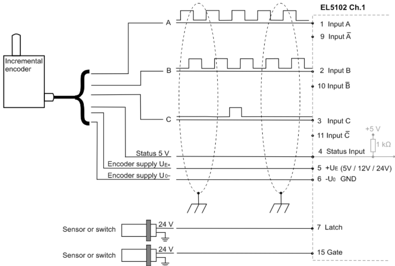
Abb. 30: Anschluss Encoder TTL - Mode mit Nullimpuls
