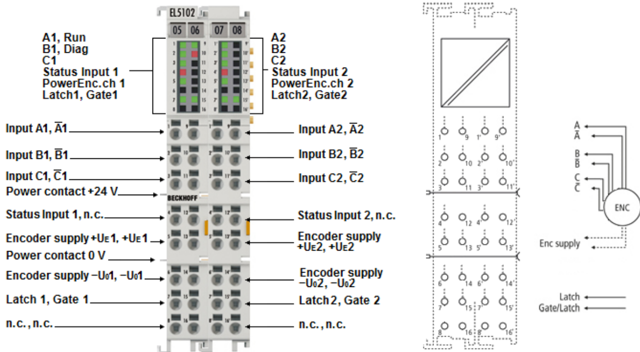
Abb. 27: EL5102 - Anschlussbelegung
