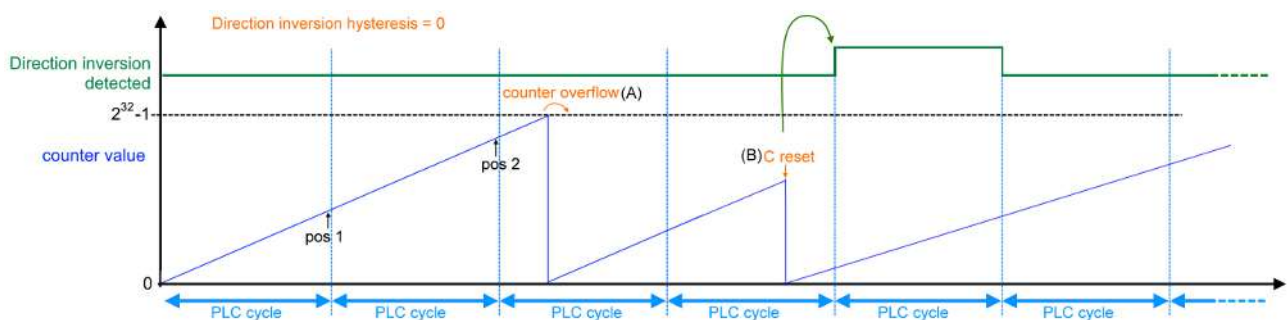
Abb. 157: Detektion der Zählrichtung
