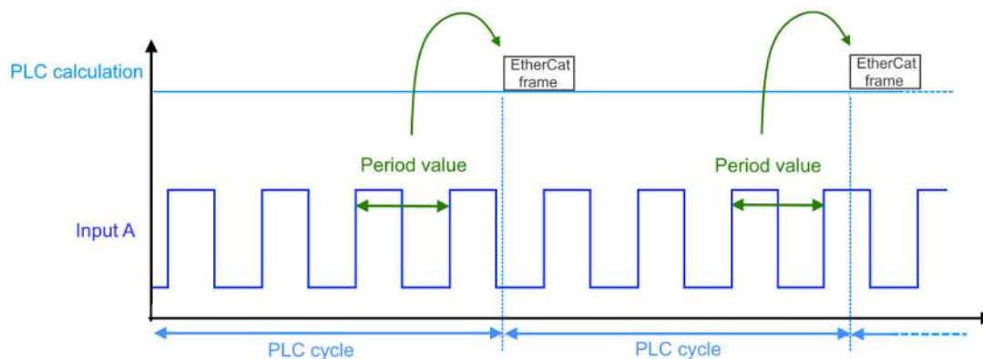
Abb. 162: Periodendauermessung
