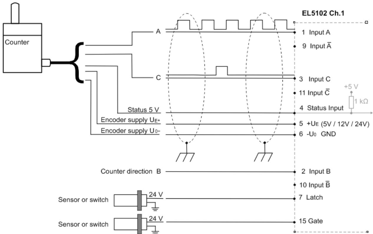
Abb. 31: Anschluss Zähler / Impulsgeber TTL - Mode mit Nullimpuls
