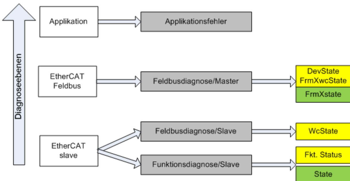
Abb. 127: Auswahl an Diagnoseinformationen eines EtherCAT-Slaves
