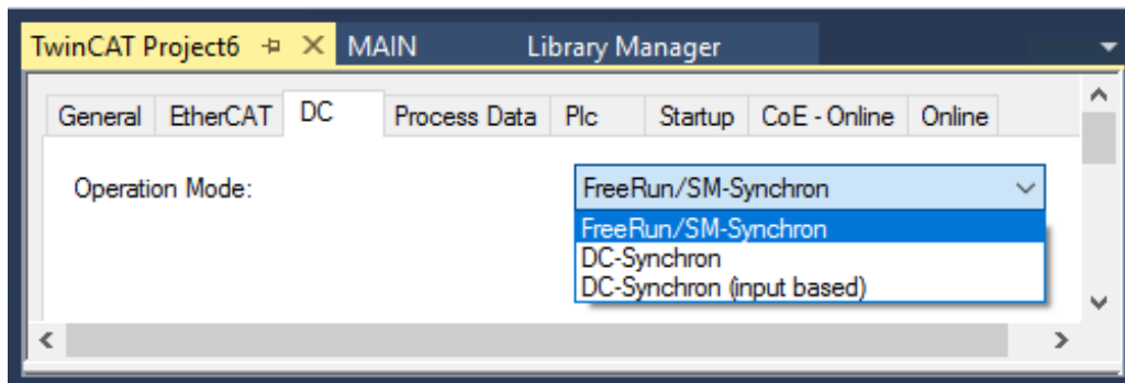
Abb. 137: Reiter "DC", Auswahlliste „Operation Mode“ Betriebsart (Trigger Modus)
