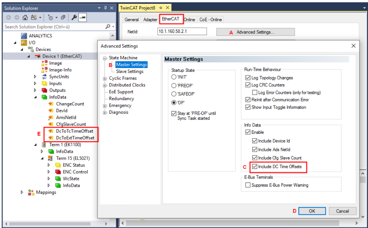
Abb. 140: Erweiterte Einstellungen des EtherCAT-Masters im TwinCAT System Manager
