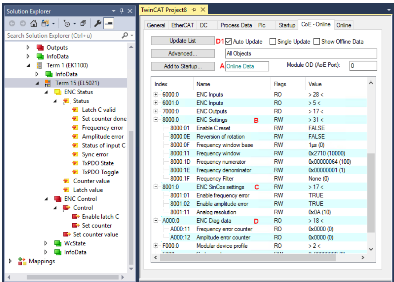
Abb. 143: CoE-Verzeichnis am Beispiel der EL5021
