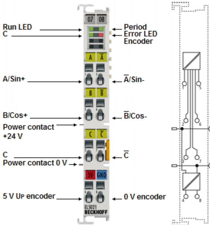
Abb. 4: EL5021
