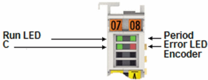
Abb. 26: EL5021-00x0 Diagnose LEDs
