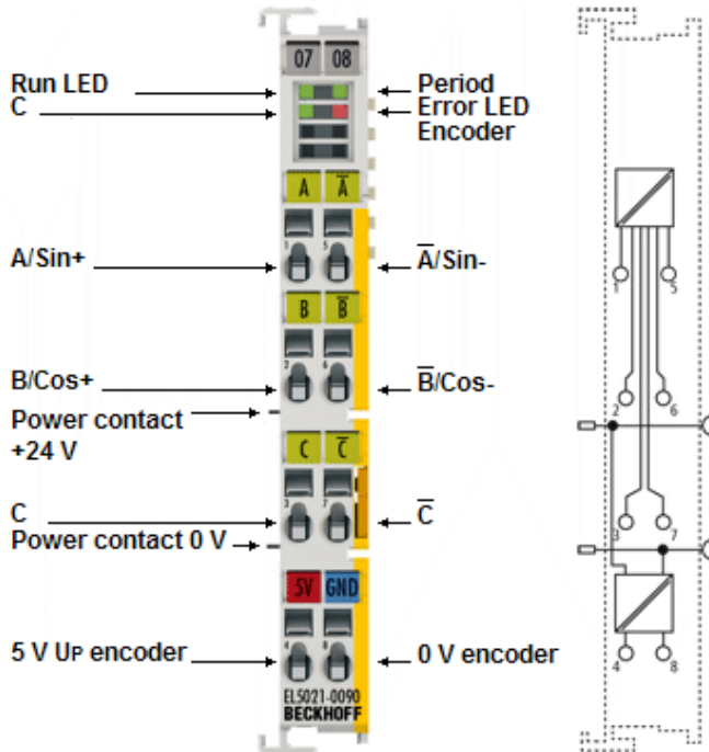
Abb. 5: EL5021-0090
