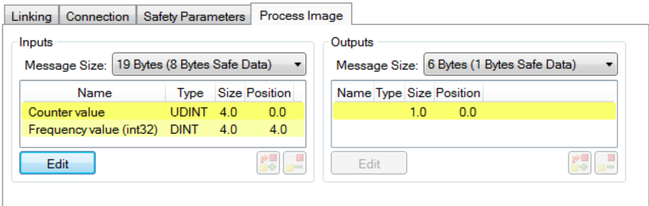
Abb. 154: Auswahl der Prozessdatengröße bzw. der Prozessdaten
