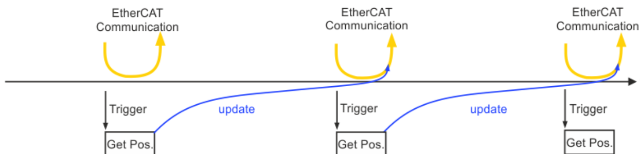
Abb. 138: frame-getriggerte EtherCAT Kommunikation
