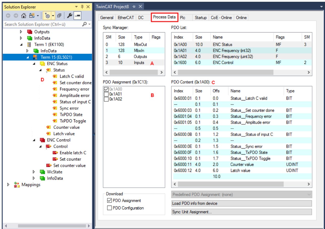
Abb. 141: EL5021 - Prozessdaten (default)
