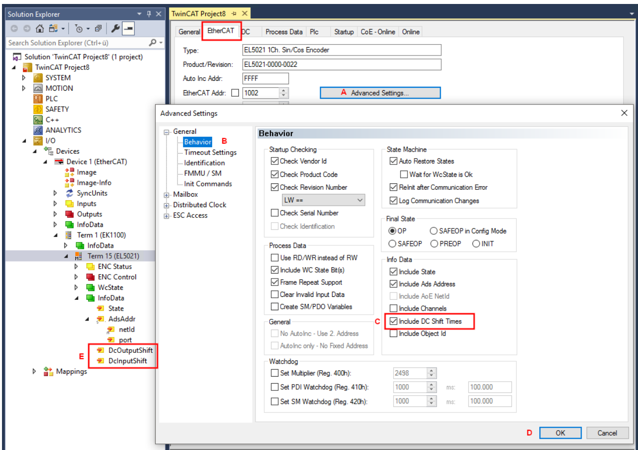
Abb. 139: Erweiterte Einstellungen der Klemme im TwinCAT System Manager
