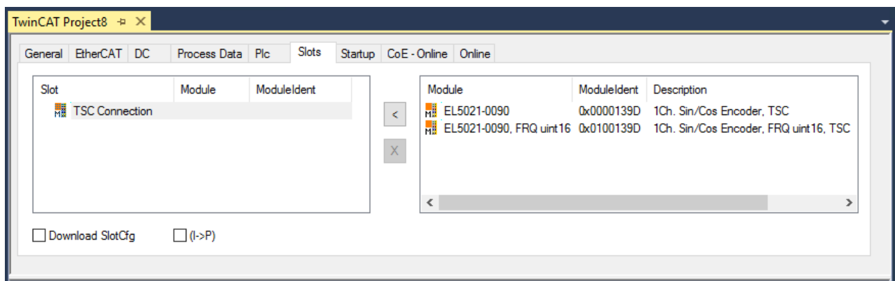
Abb. 142: EL5021-0090 – Slot-Module Zuordnung im Reiter Slots
