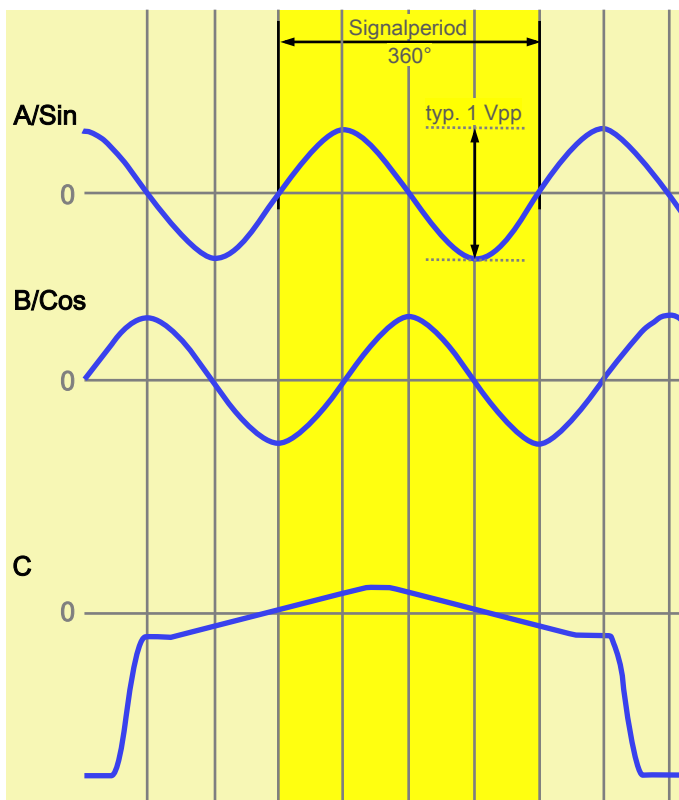
Abb. 136: Signalausgänge des Positionsgebers
