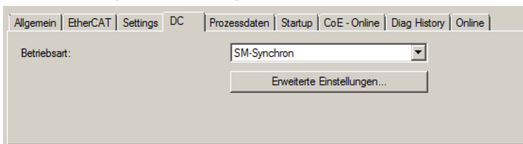
Abb. 126: Karteireiter „DC“ (Distributed Clocks)
