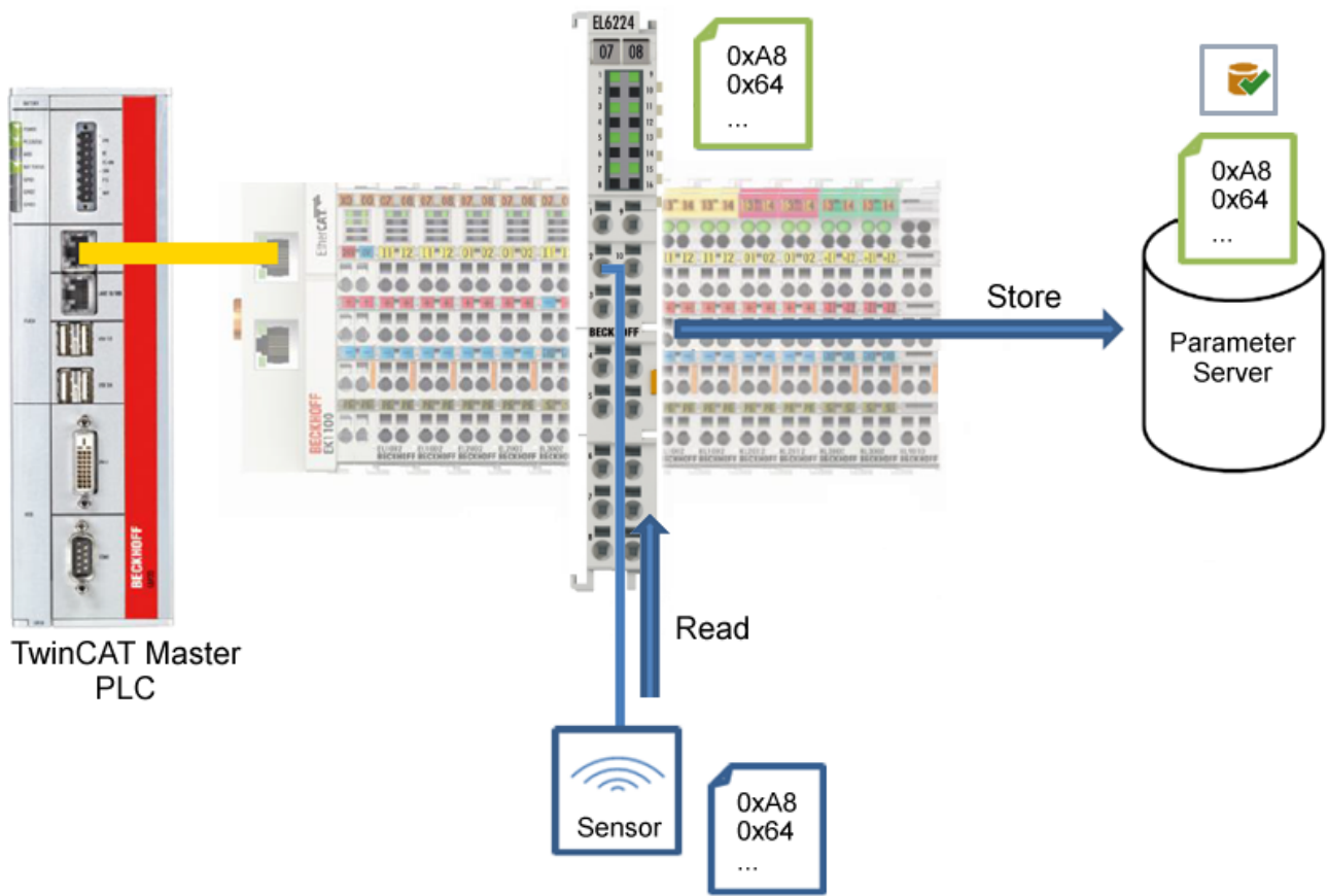
Fig. 33: Store parameters
