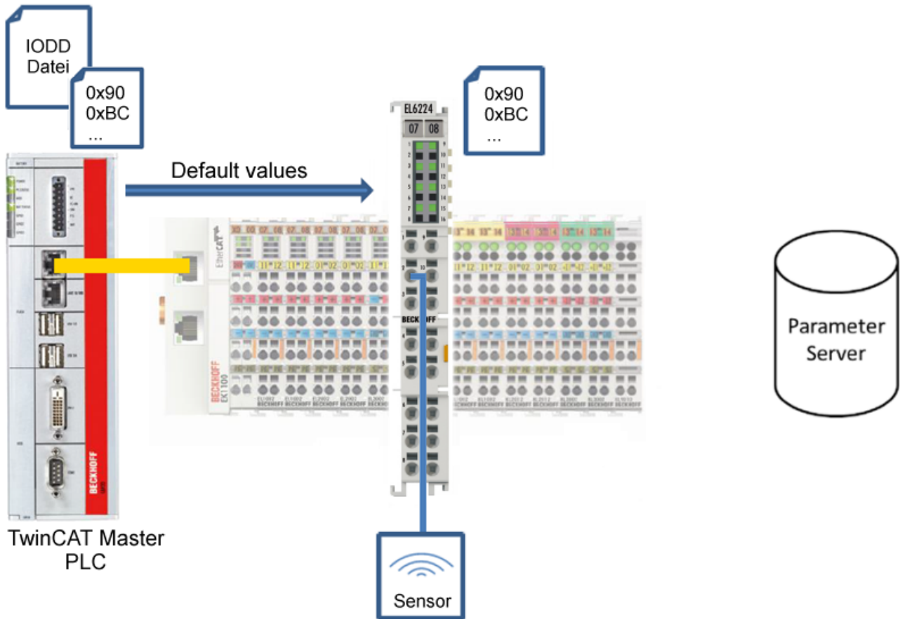
Fig. 28: Reset parameter values to default
