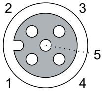
Abb. 16: M12-Buchse
