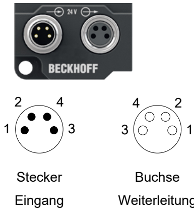
Abb. 4: M8-Steckverbinder
