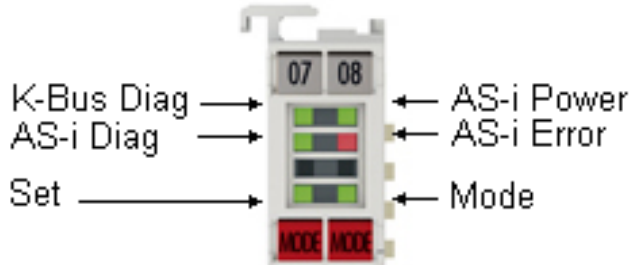
Abb. 37: LEDs
