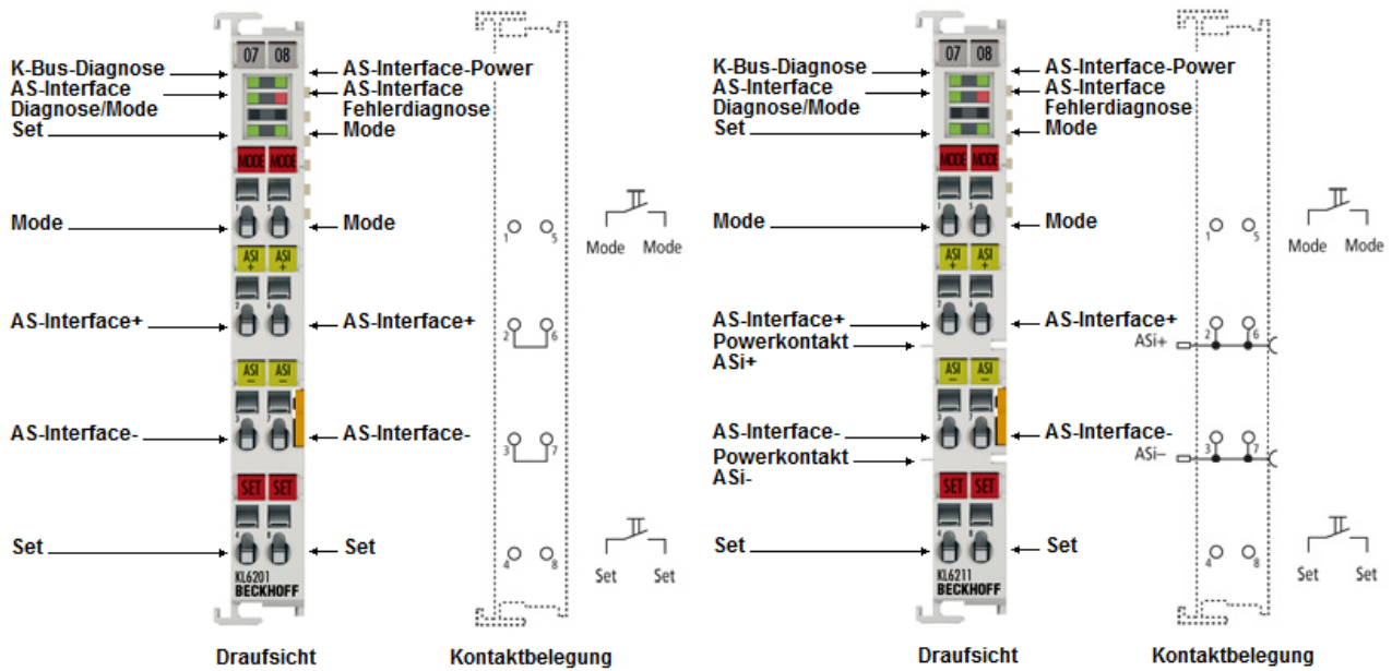
Abb. 1: KL6201, KL6211
