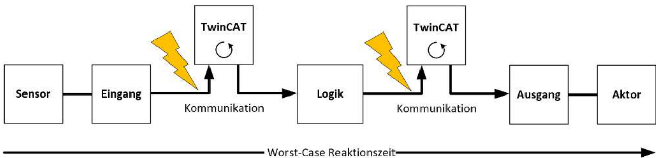
Abb. 150: Worst-Case-Reaktionszeit
