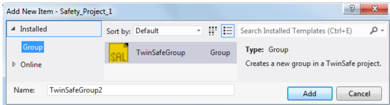
Abb. 37: Anlegen einer TwinSAFE-Gruppe
