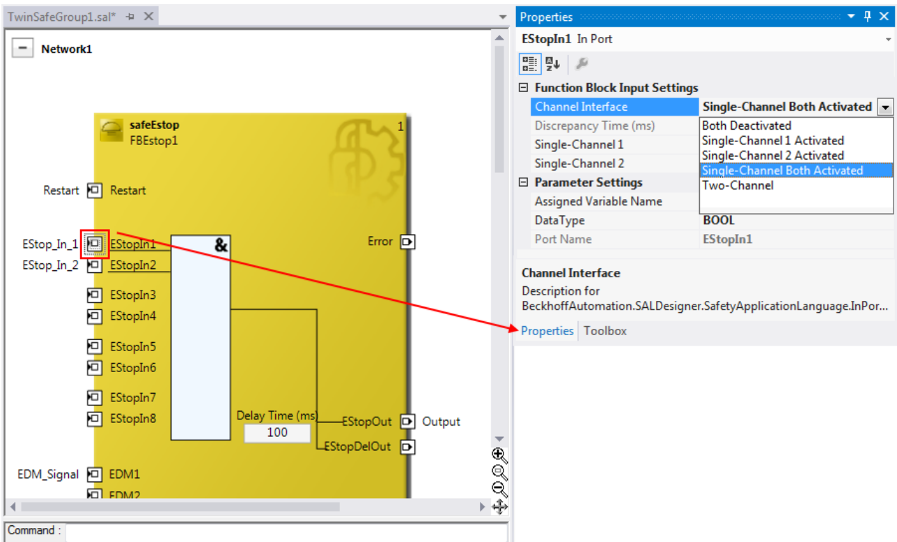
Abb. 46: Properties der FB-Ports
