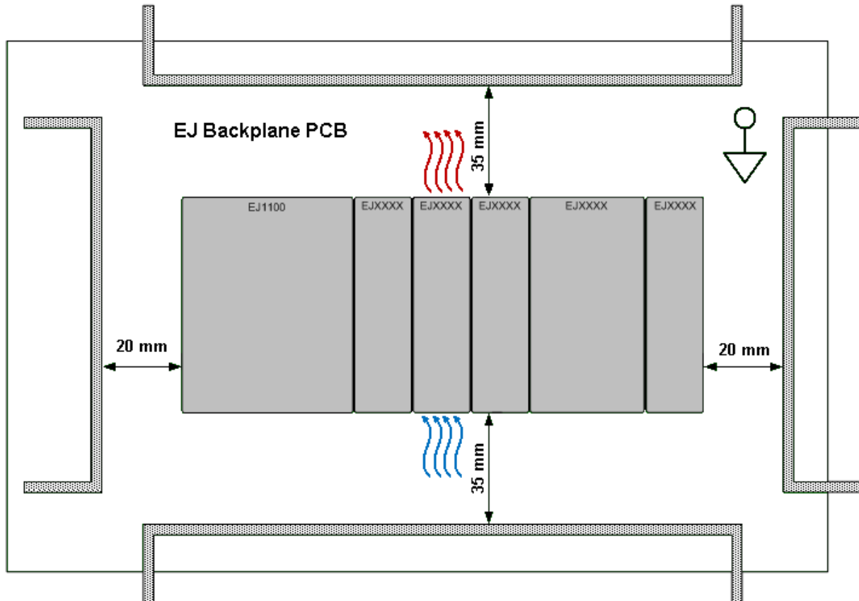
Abb. 4: Einbaulage und Mindestabstände
