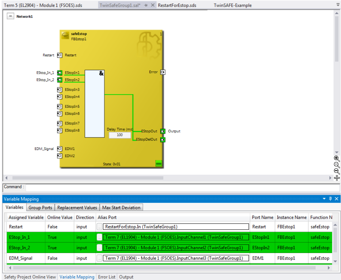
Abb. 61: sal-Arbeitsblattes und Variable Mapping im Online-Modus
