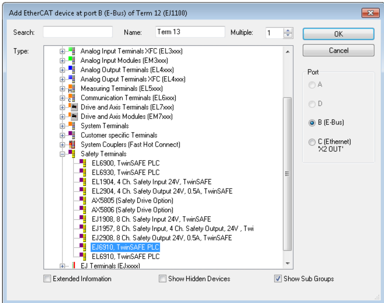
Abb. 5: TwinCAT - Einfügen eines EJ6910
