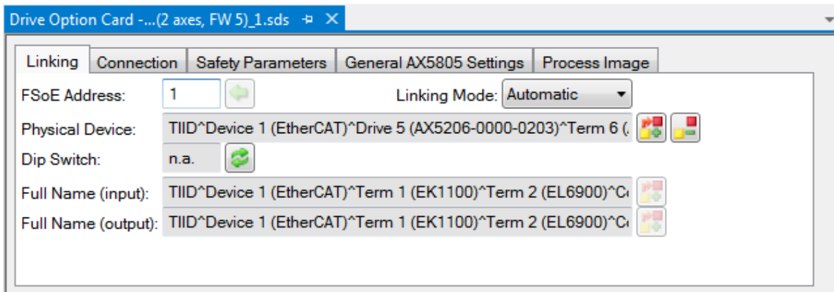
Abb. 19: AX5000-Safety-Antriebsoptionen
