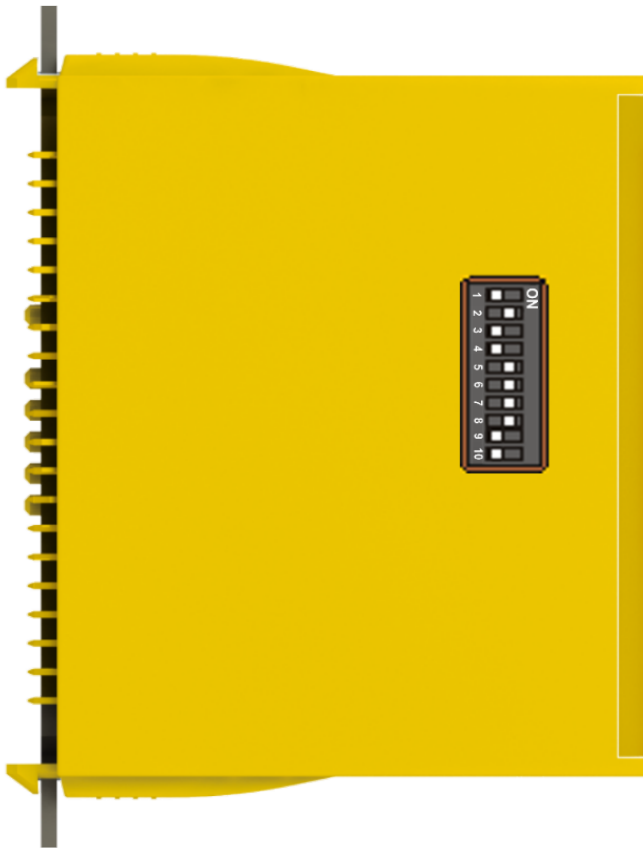
Abb. 6: Adresseinstellung auf TwinSAFE-EJ-Modulen mit 1023 möglichen Adressen
