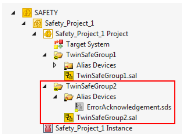
Abb. 38: Bestandteile der TwinSAFE-Gruppe
