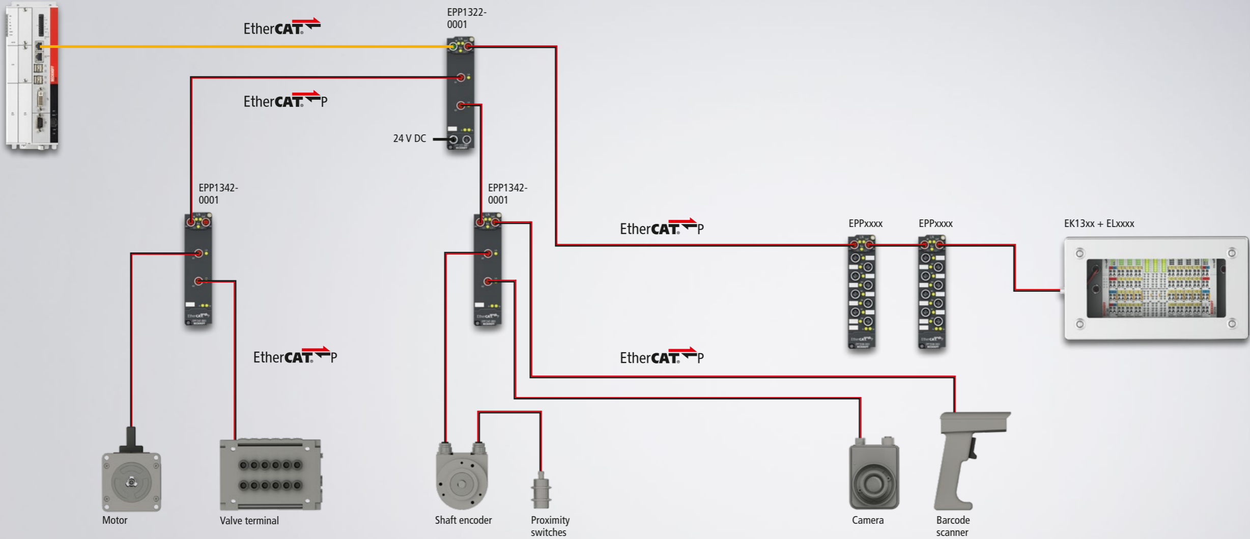
EtherCAT master
