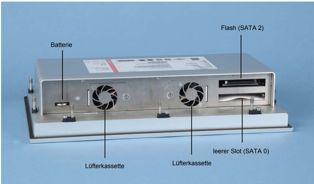
Abb.: CP2216, Ansicht auf Speichermedien, Batterie und Lüfter
