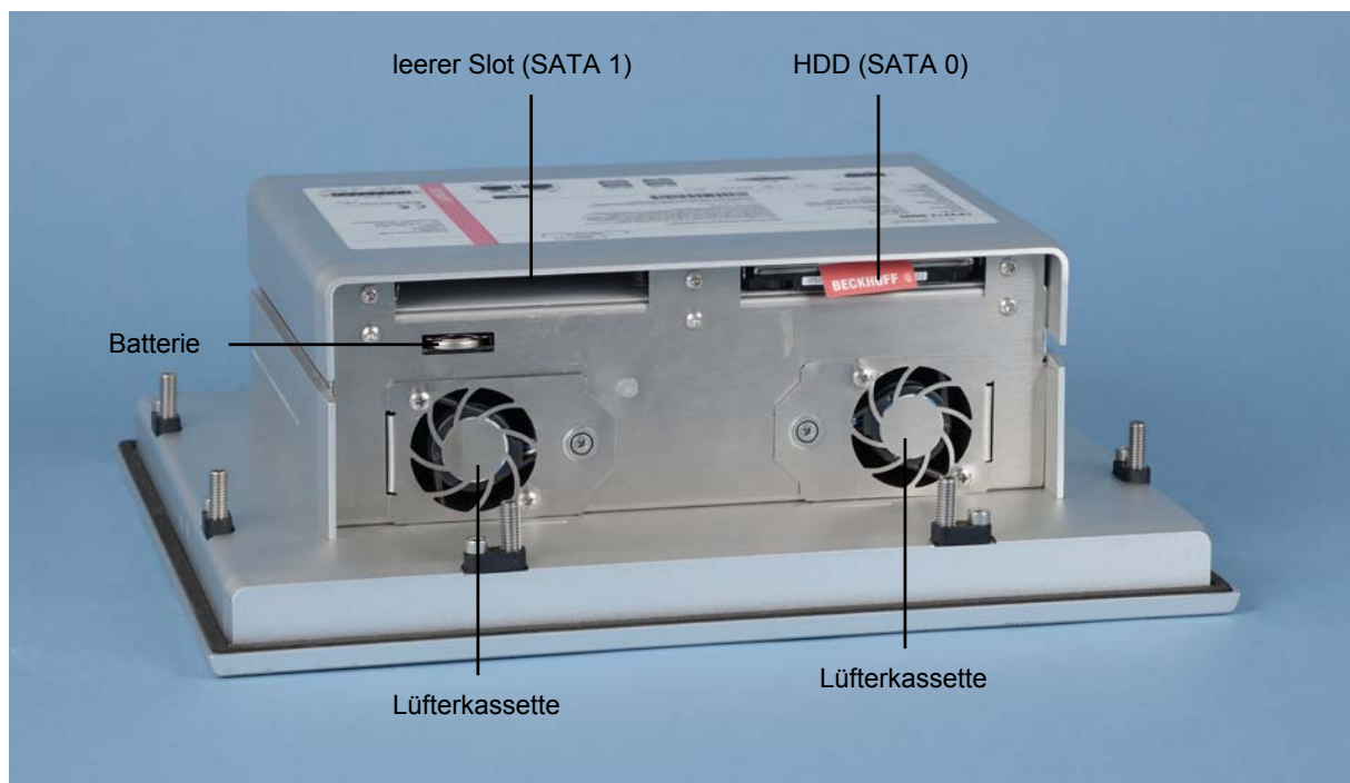
Abb.: CP2212, Ansicht auf Speichermedien, Batterie und Lüfter
