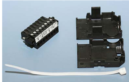
Steckerleiste 8-polig, Zugentlastungsgehäuse mit Kabelbinder
