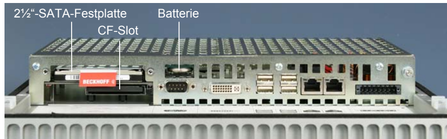
Zugang zur Festplatte, dem CF-Slot und der Batterie
