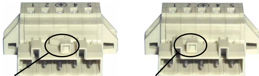
Kodierung bei 100-240 V AC 50-60 Hz Kodierung bei 24 V DC Netzteil
