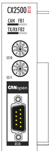
Feldbusmodul
