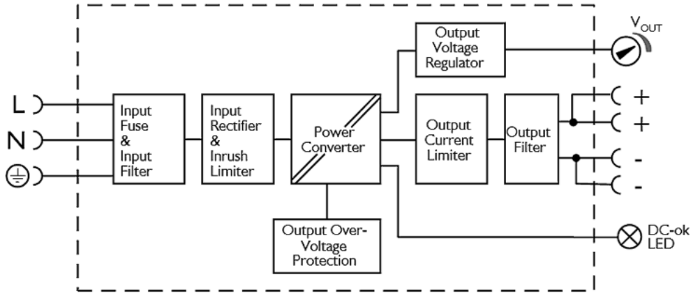
Abb. 9: Funktionsschaltbild
