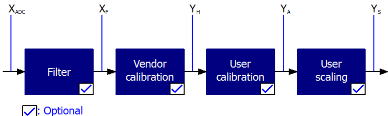
附图 43: 过程数据的计算
