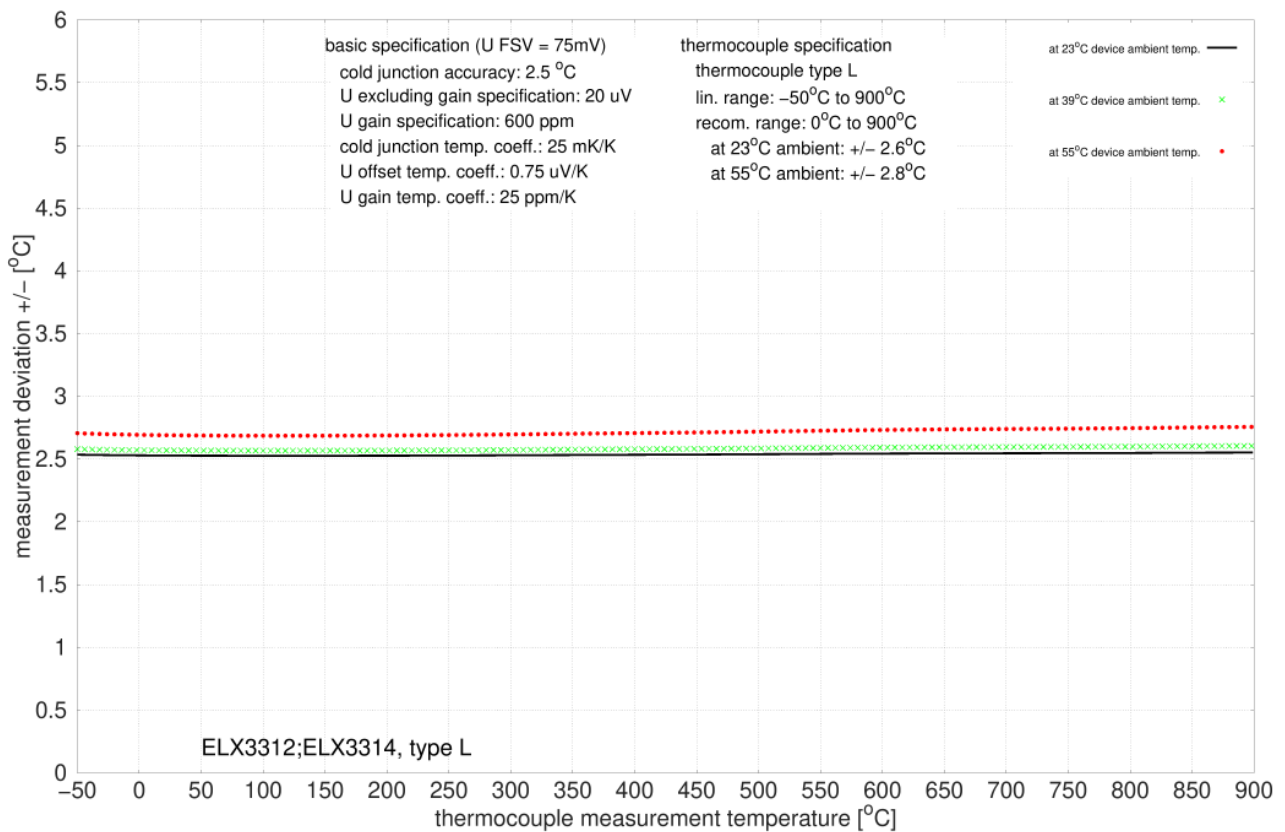
附图 36: L 型热电偶的测量不确定度
