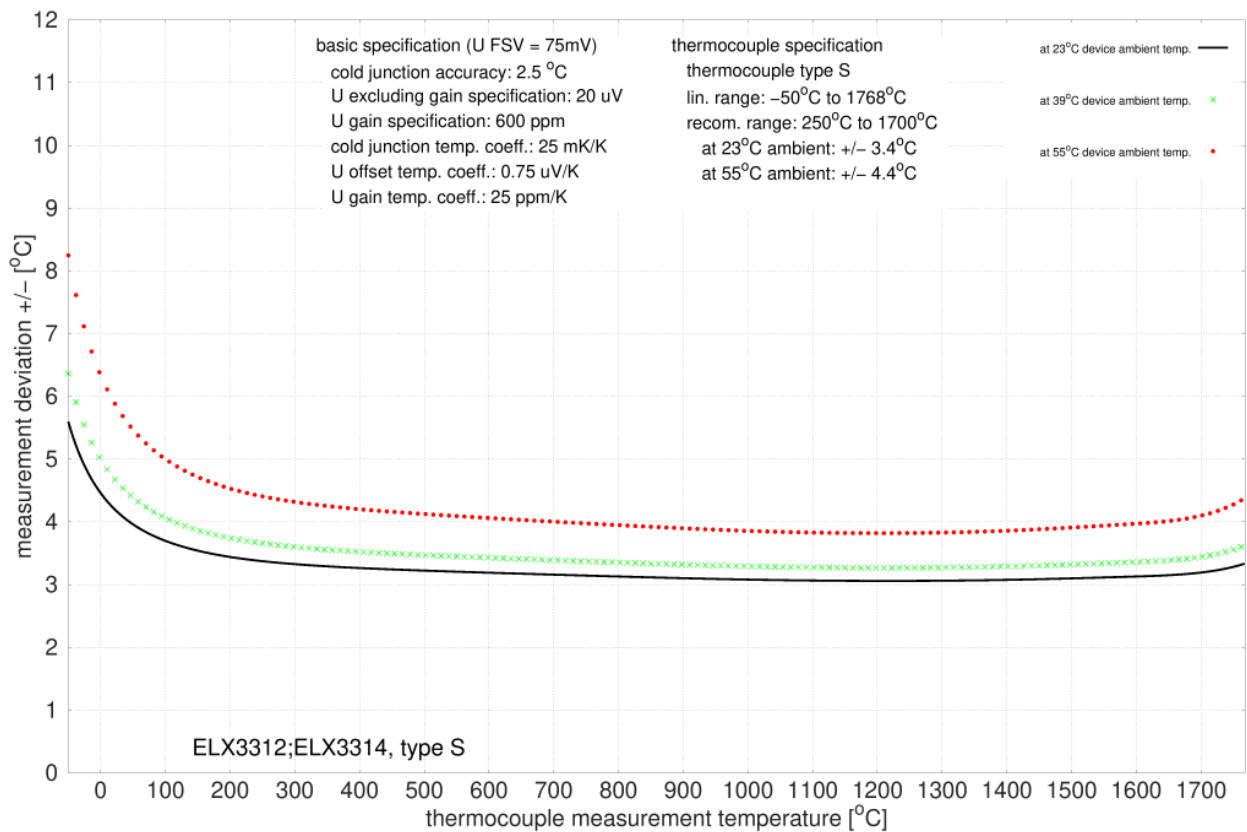
附图 39: S 型热电偶的测量不确定度
