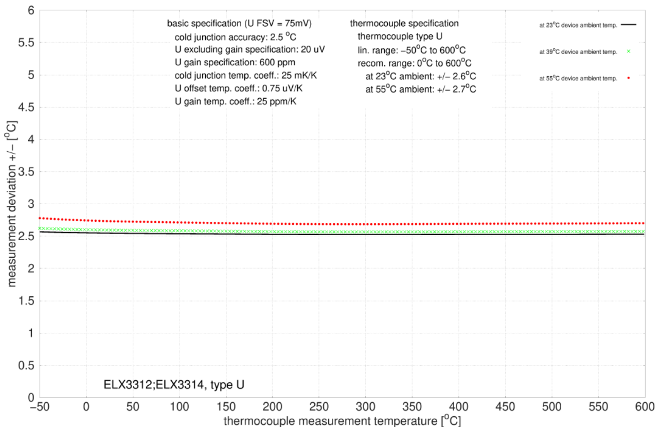
附图 41: U 型热电偶的测量不确定度
