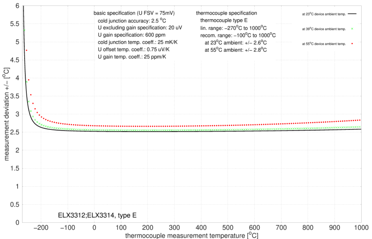
附图 33: E 型热电偶的测量不确定度
