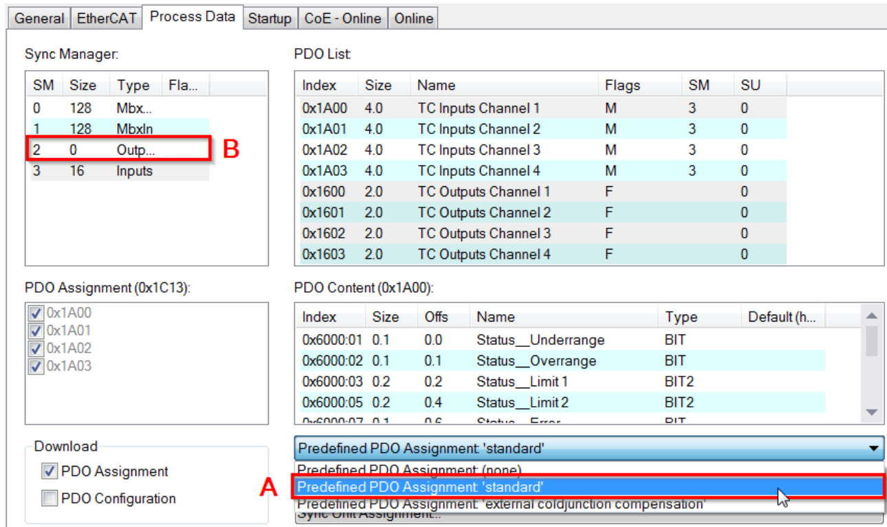
附图 49: TwinCAT 系统管理器，带预定义 PDO 选项标准
