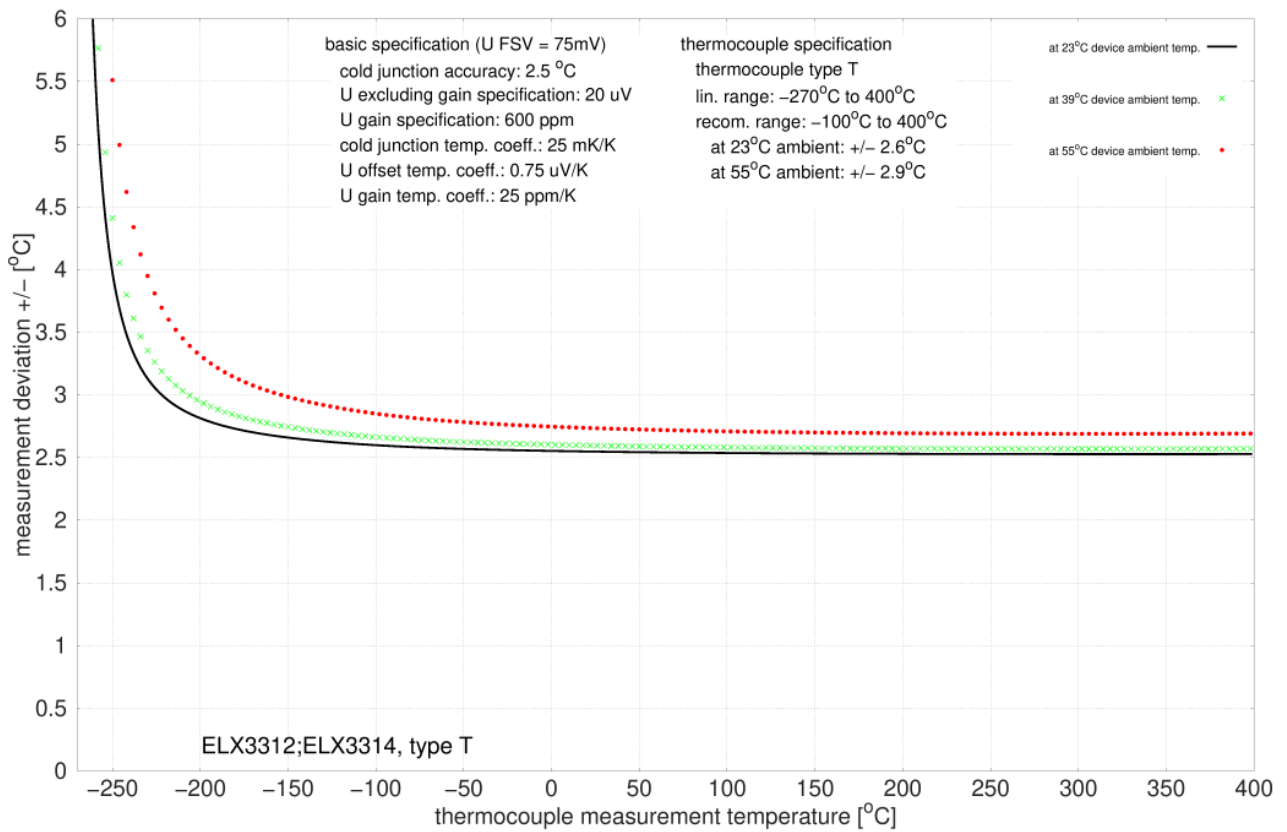
附图 40: T 型热电偶的测量不确定度
