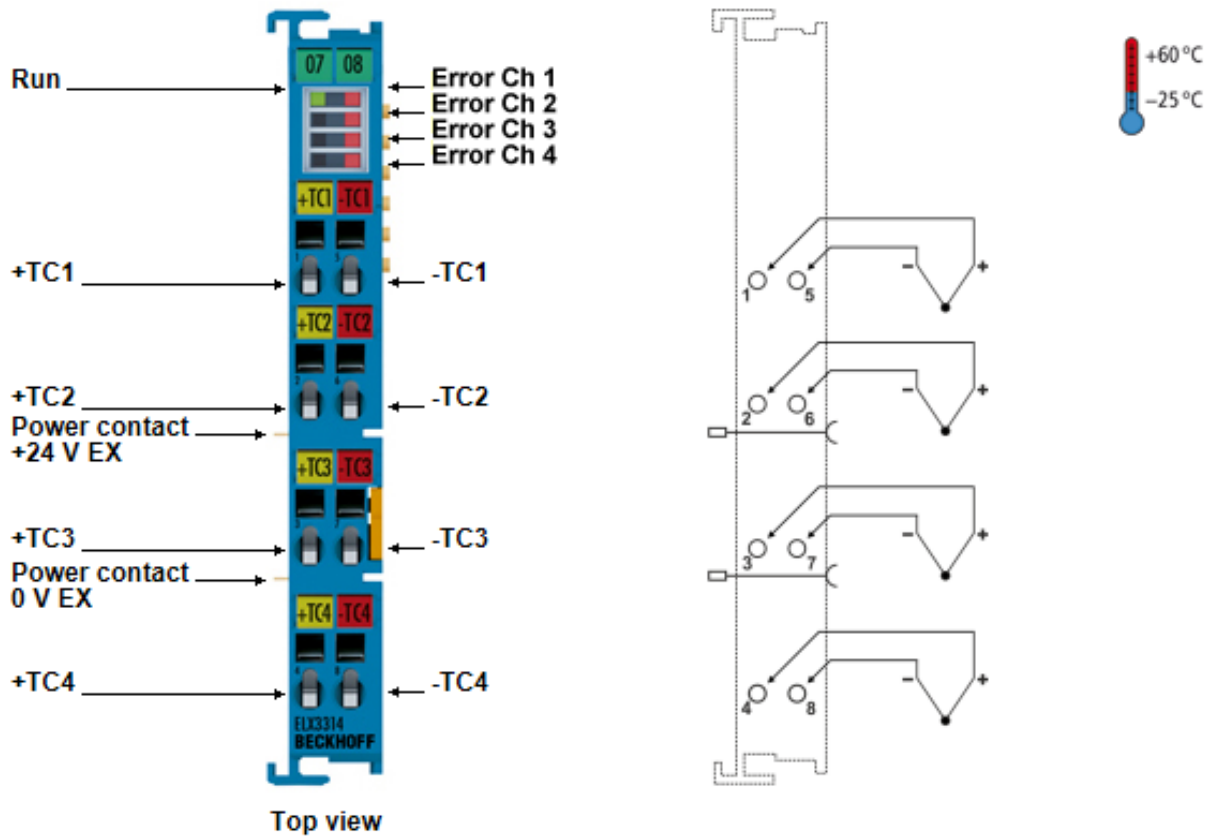
附图 21: ELX3314 - 触点分配
