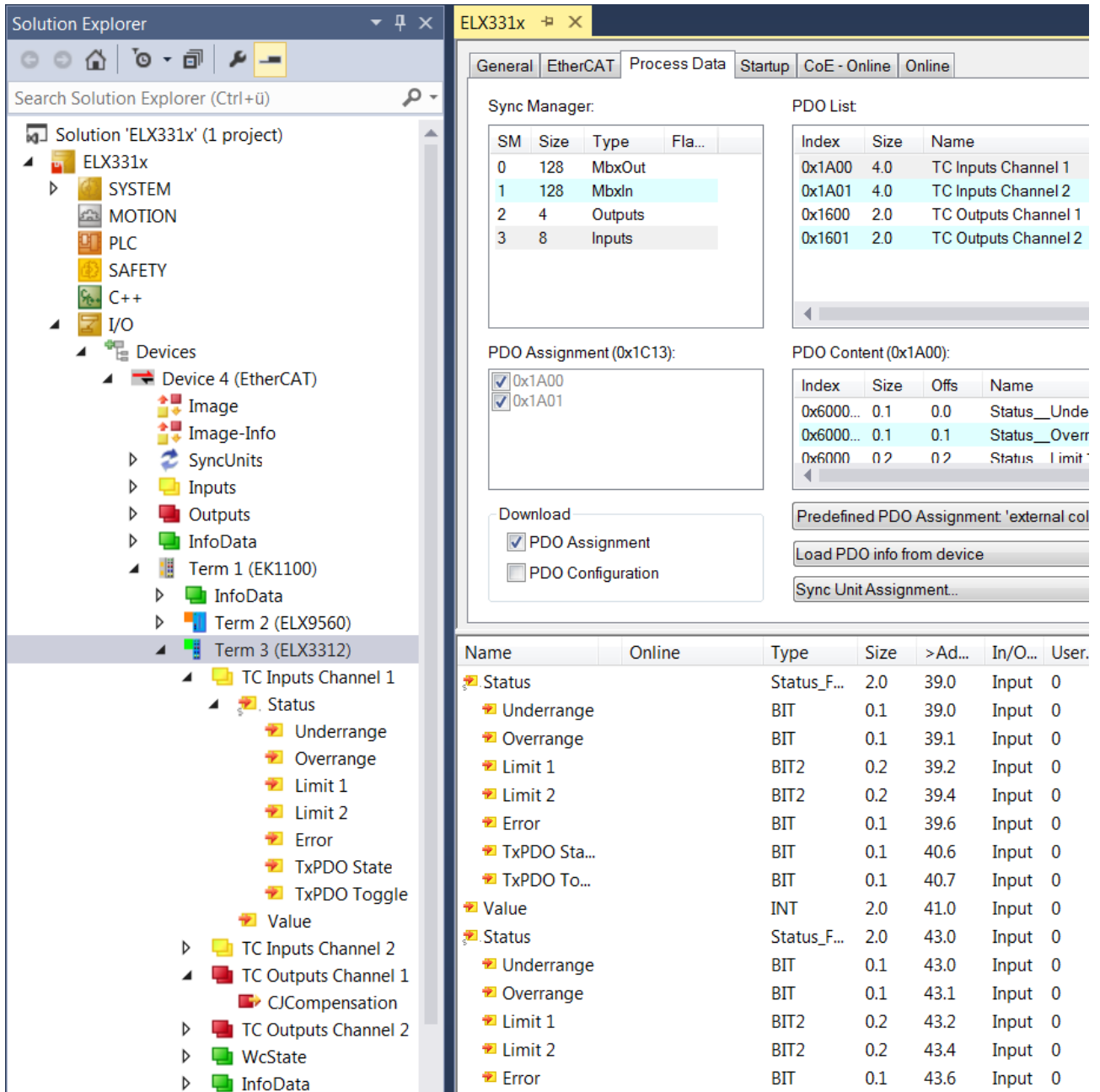
附图 45: ELX3312 - 过程数据
