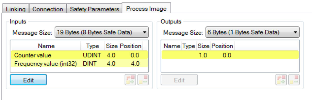
附图 56: 选择过程数据大小和过程数据
