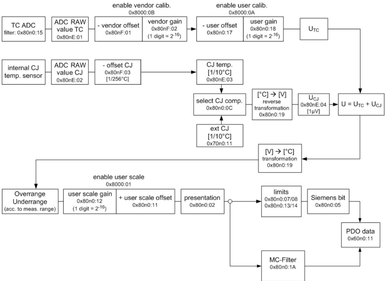
附图 42: ELX331x - 数据流
