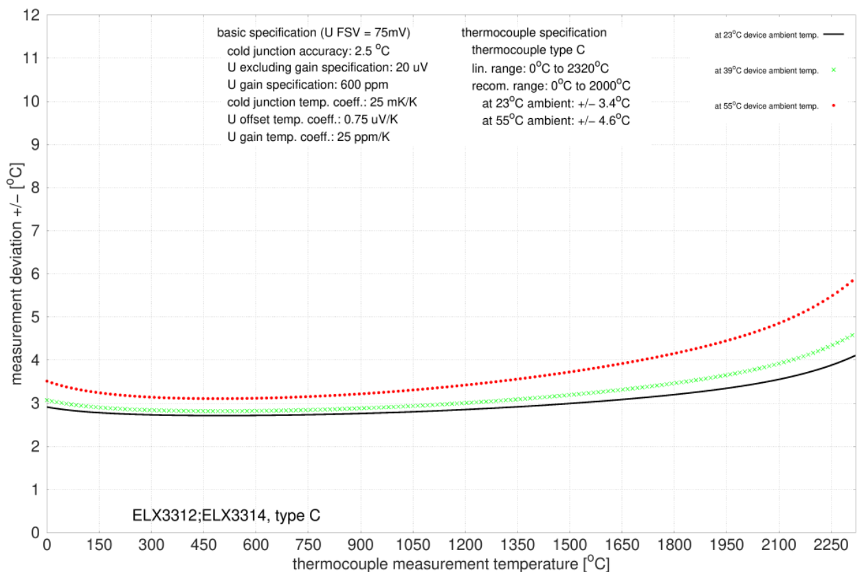
附图 32: C 型热电偶的测量不确定度
