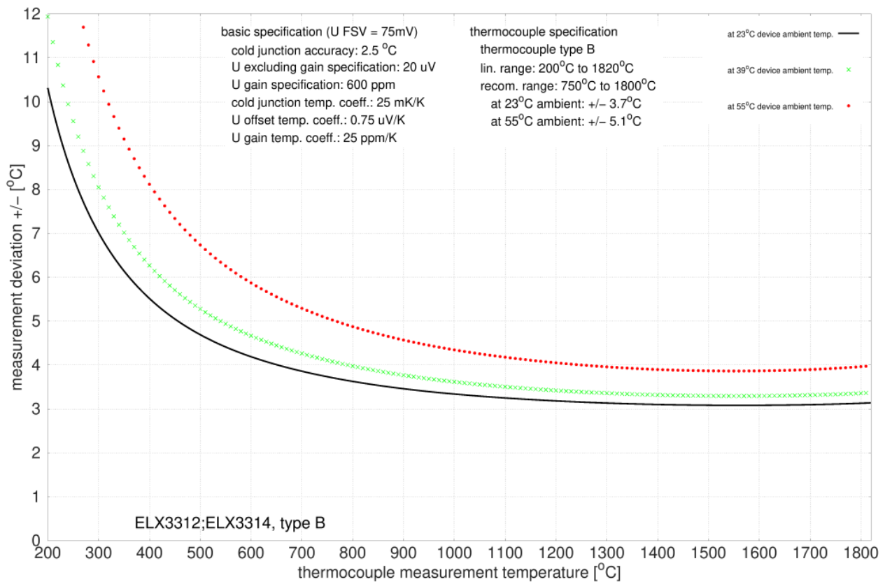
附图 31: B 型热电偶的测量不确定度
