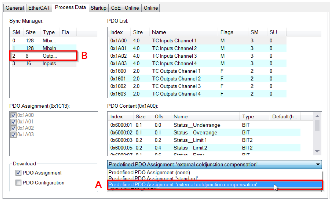
附图 50: 带有预定义 PDO 选择的 TwinCAT 系统管理器外部补偿
