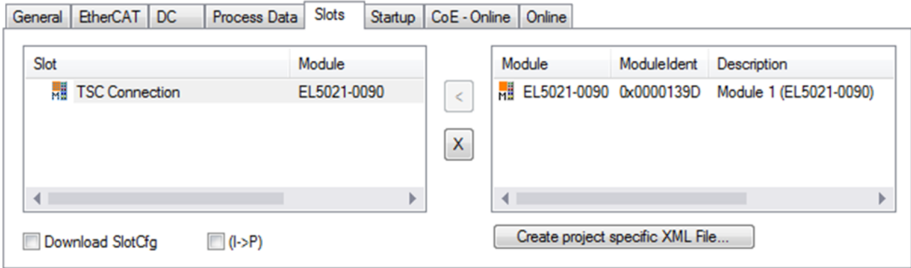
附图 51: 在组件下添加TwinSAFE SC过程数据，如EL5021-0090
