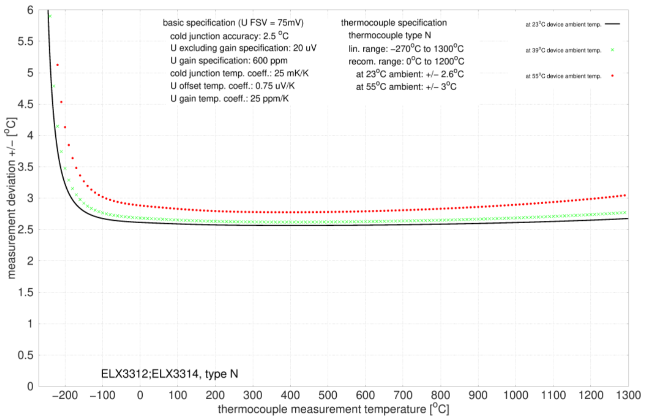
附图 37: N 型热电偶的测量不确定度
