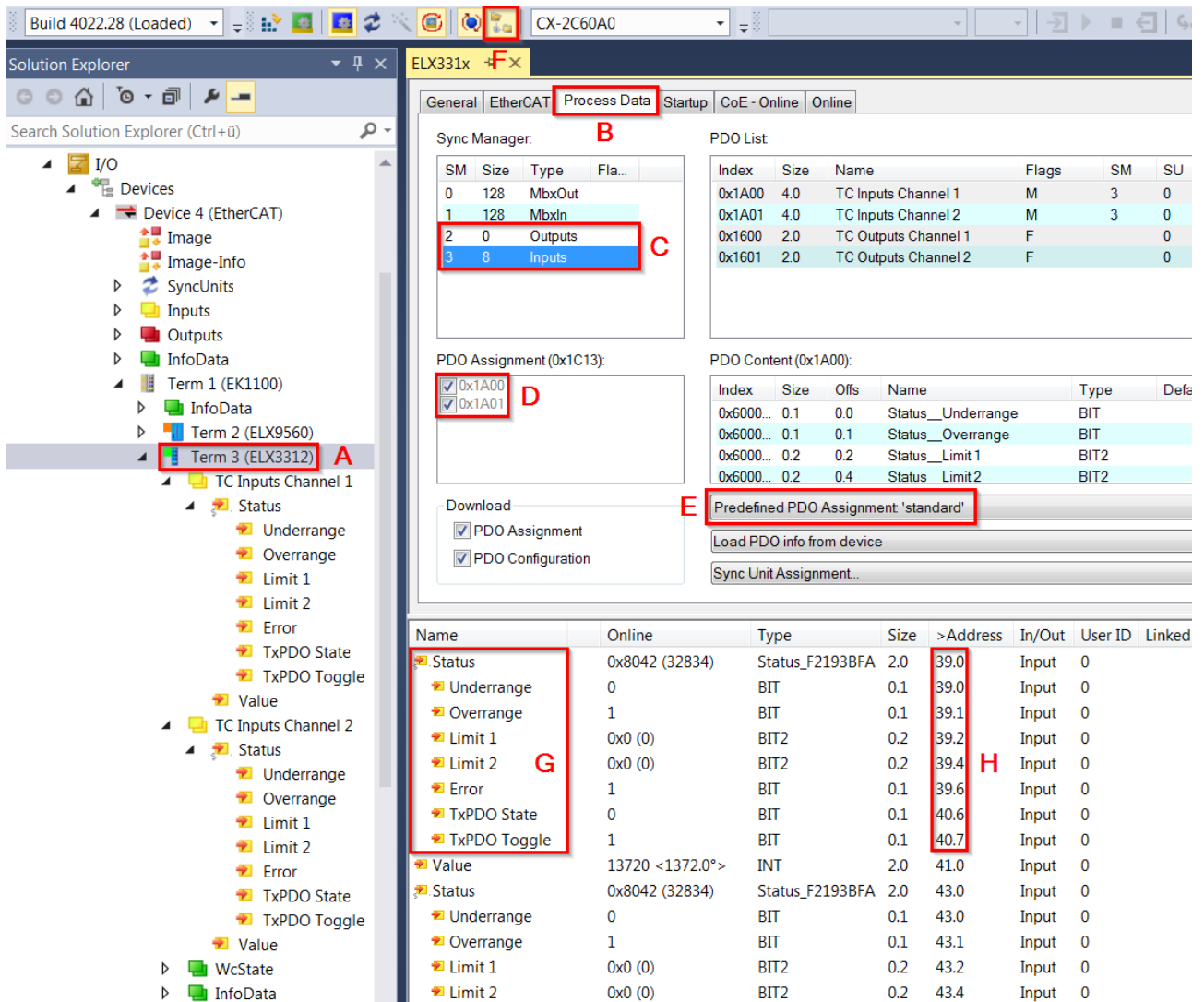
附图 46: ELX3312 - TwinCAT 中的过程数据选择
