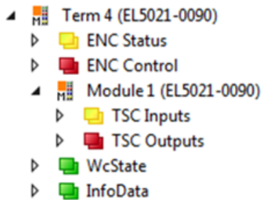
附图 52: TwinSAFE SC组件的过程数据，示例EL5021-0090
