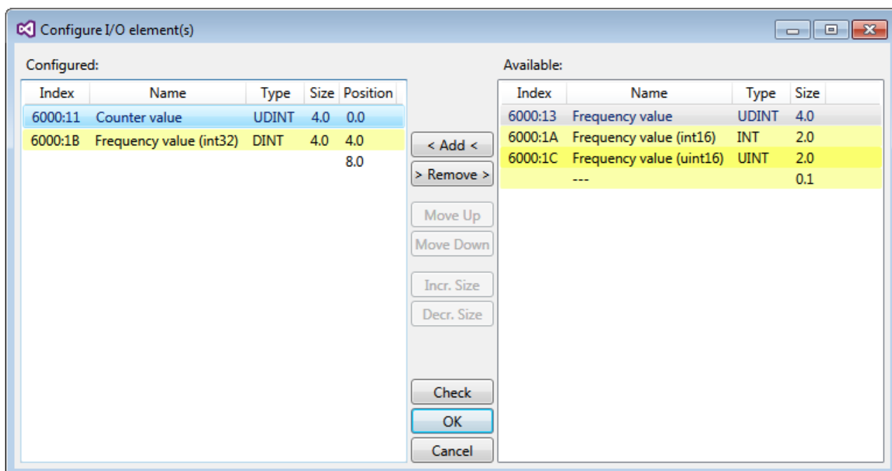
附图 57: 过程数据的选择
