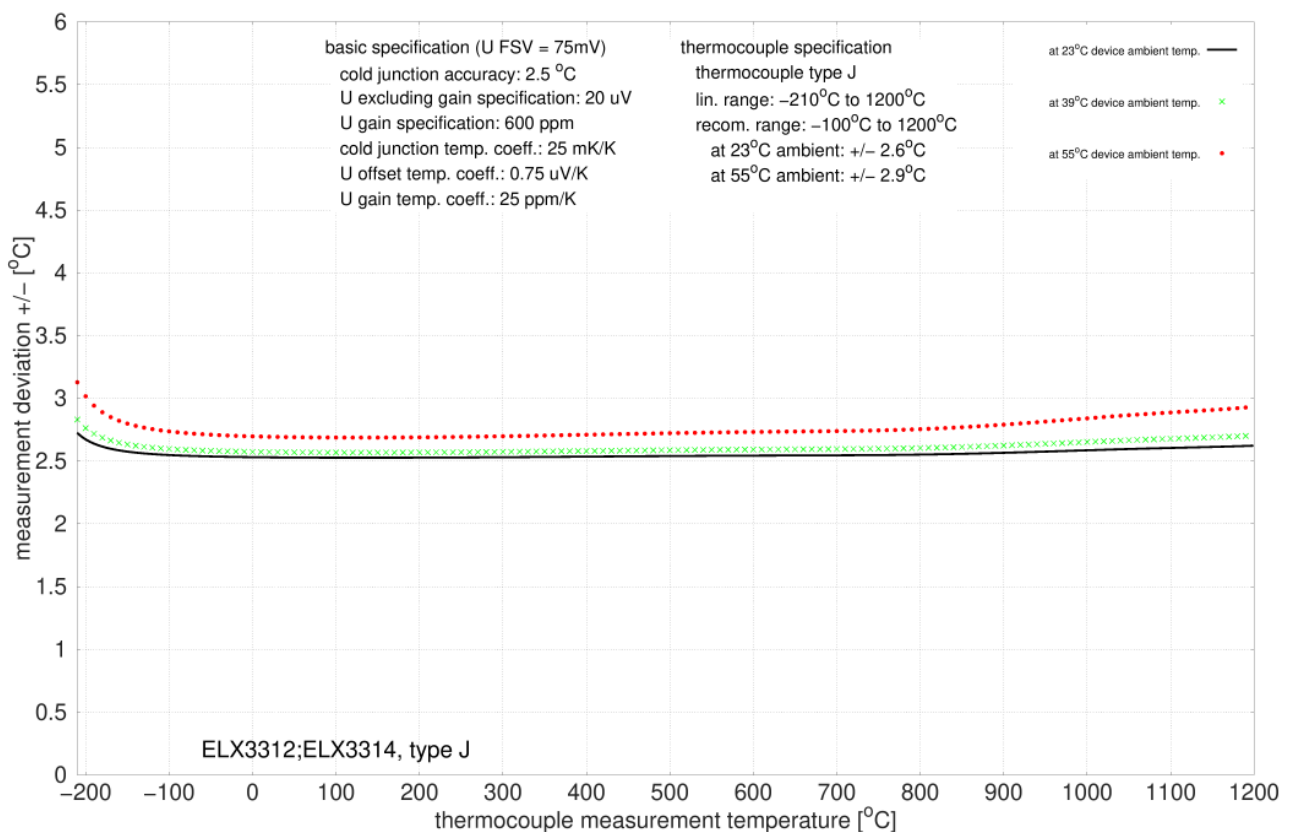
附图 34: J 型热电偶的测量不确定度
