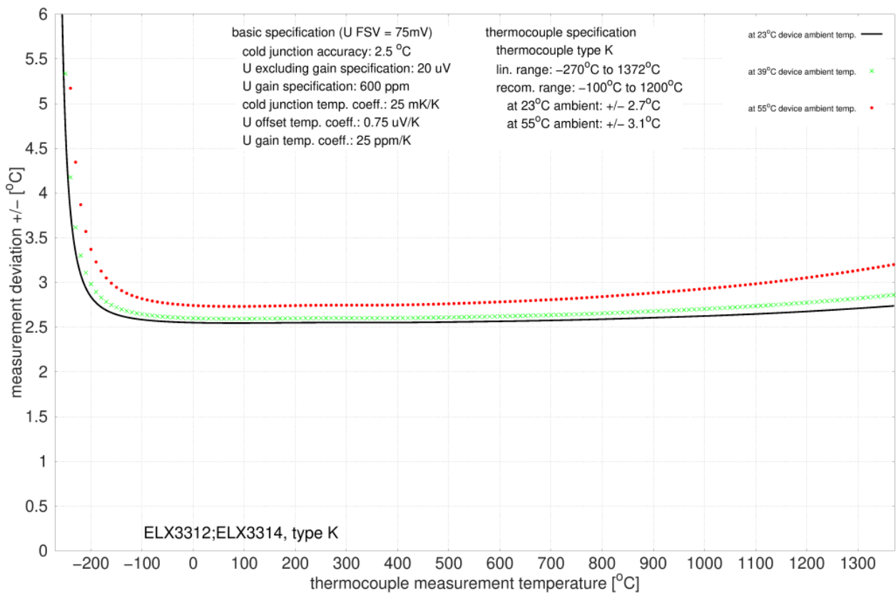
附图 35: K 型热电偶的测量不确定度
