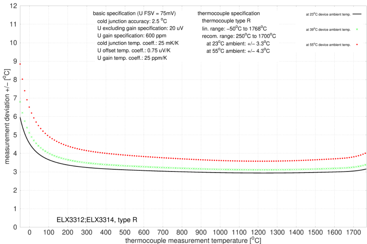
附图 38: R 型热电偶的测量不确定度
