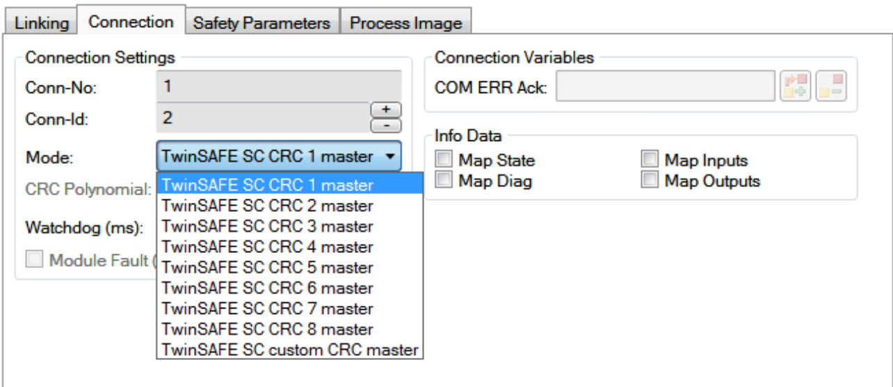
附图 55: 选择一个自由CRC
