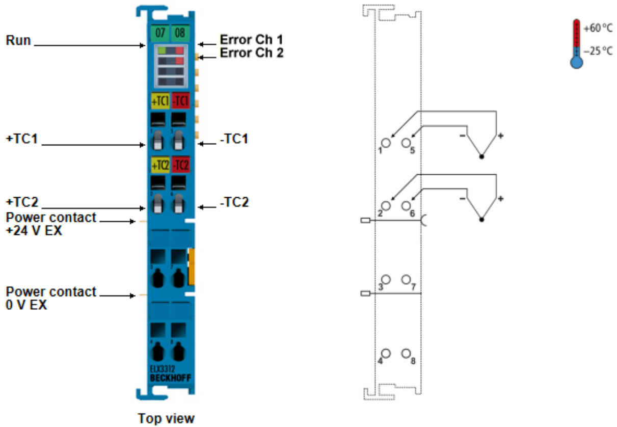
附图 20: ELX3312 - 触点分配
