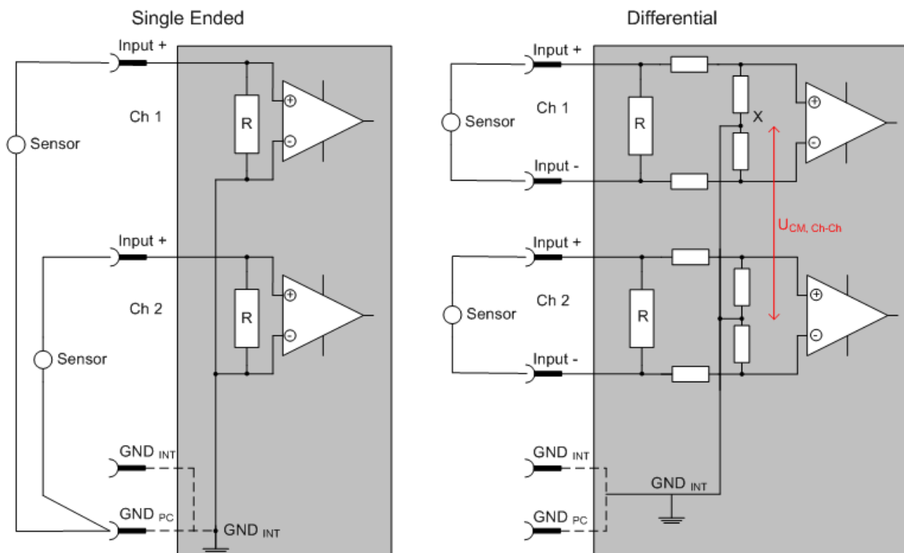
附图 23: SE和DIFF模块为2通道版本
