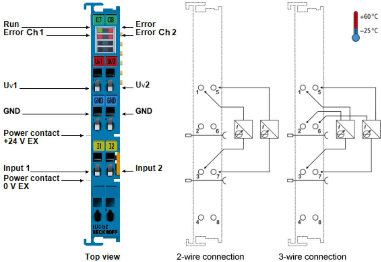
附图 4: ELX3152 - 两通道, 模拟输入终端, 0/4 ... 20 mA, 单端, 16位, Ex i
