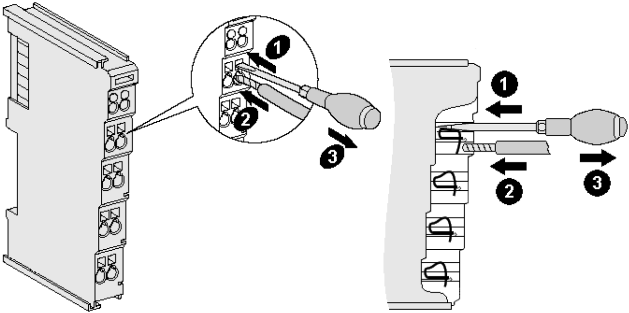
附图 19: 在一个接线点上连接电缆
