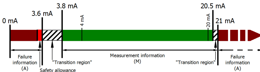
附图 30: NAMUR建议NE43中定义的表述 (2003年2月3日版本)
