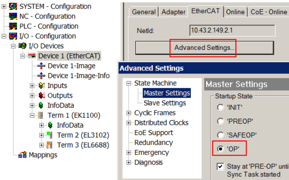
附图 134: 系统管理器的默认行为
