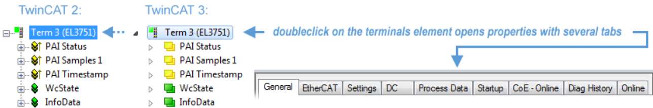
附图 120: 终端EL3751的分支元件
