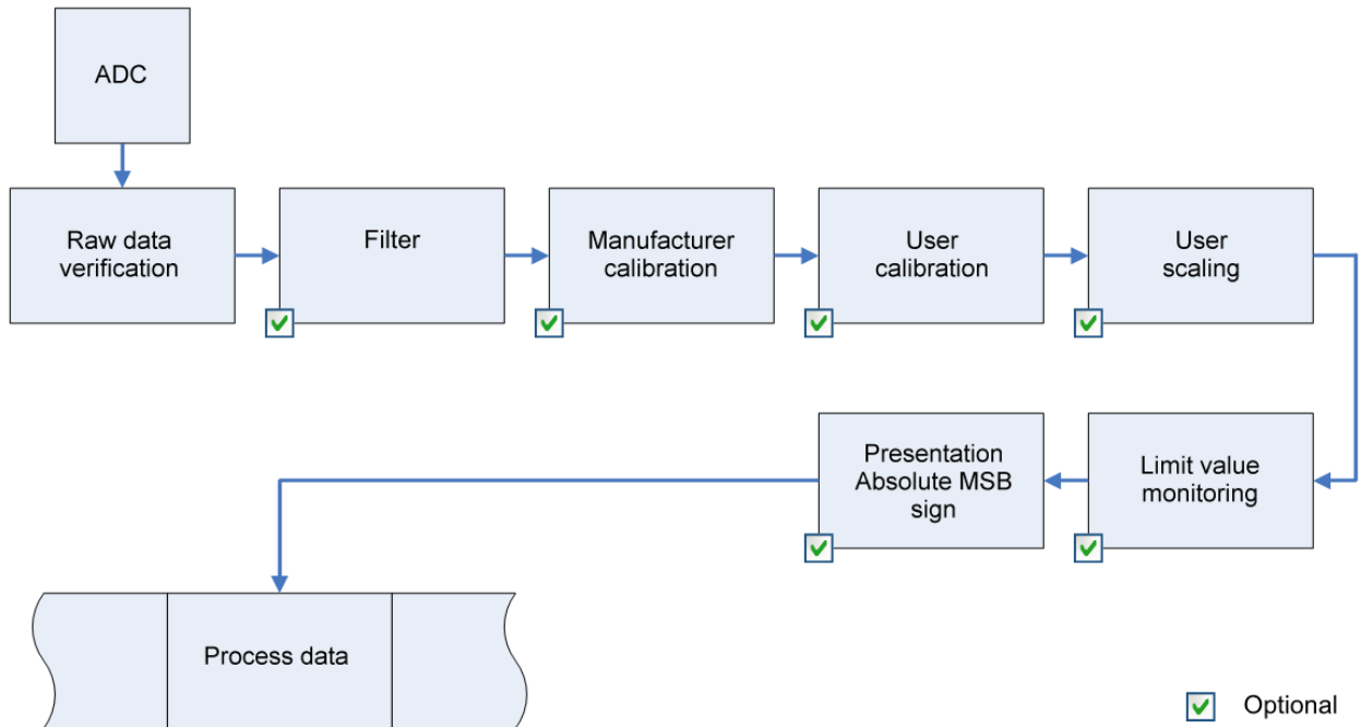
附图 150: ELX31xx的数据流
