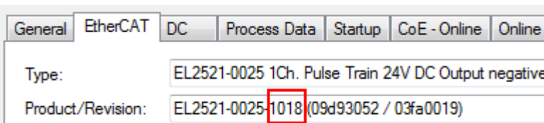
附图 104: 安装EtherCAT终端，修订版本-1018
