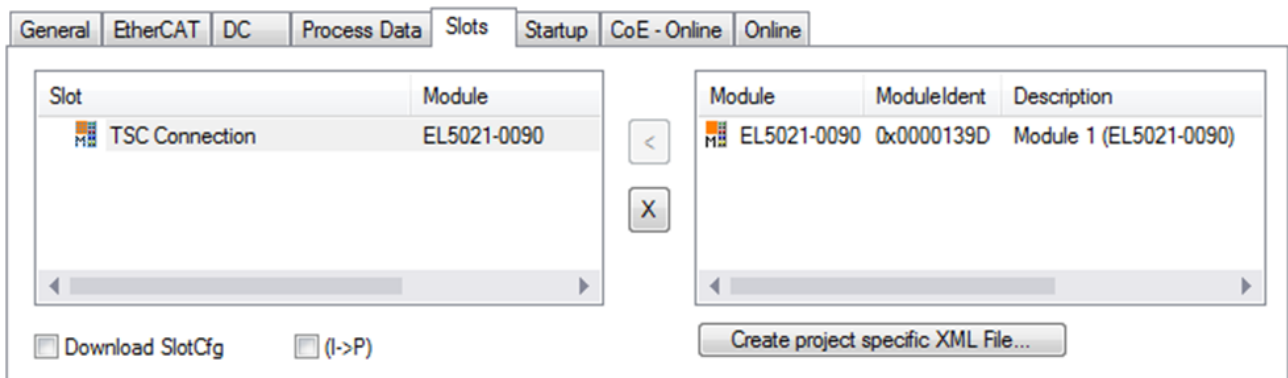
附图 154: 在组件下添加TwinSAFE SC过程数据，如EL5021-0090
