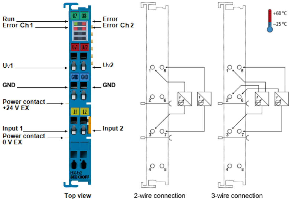
附图 20: ELX3152 - 触点分配
