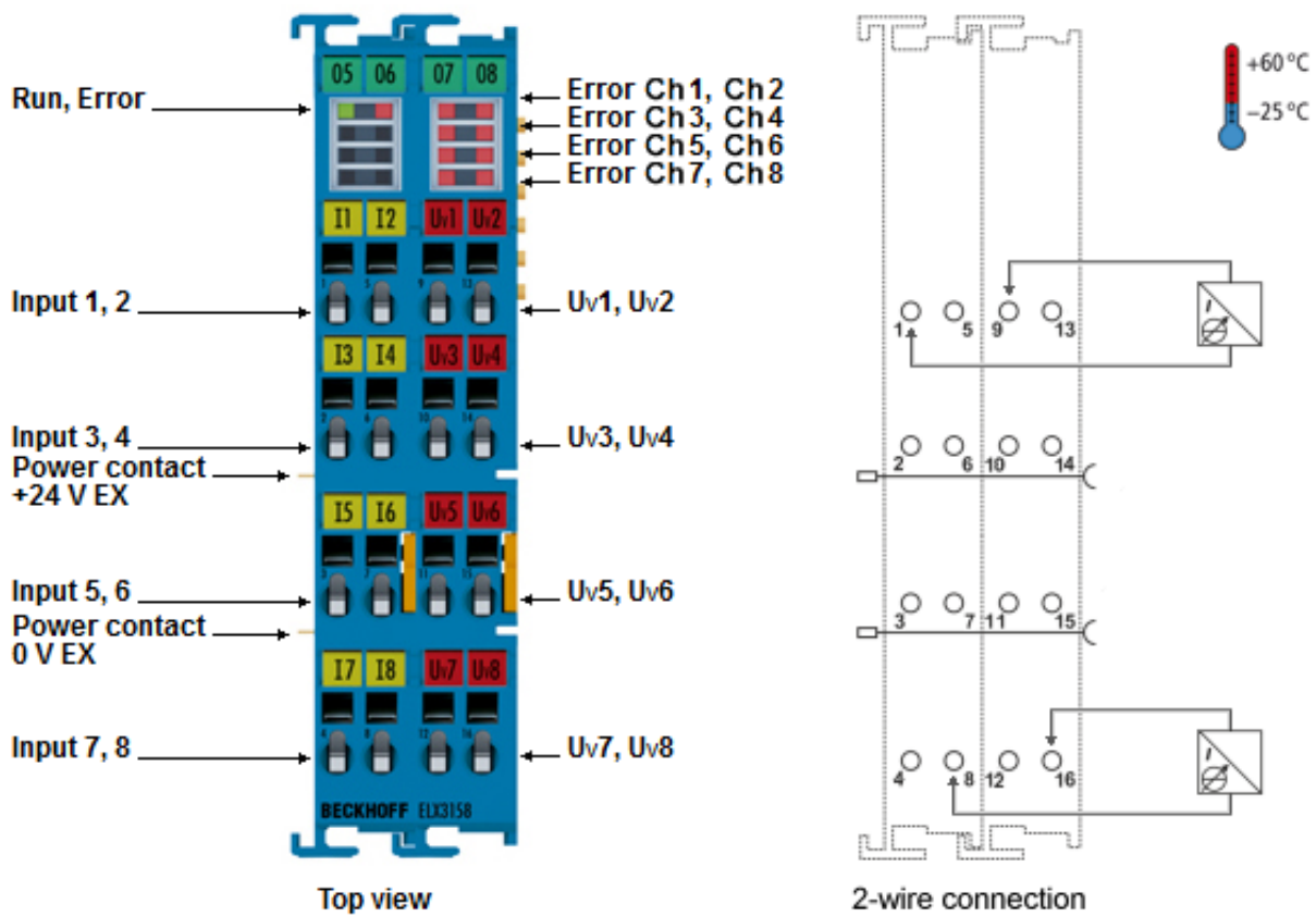
附图 21: ELX3158 - 触点分配
