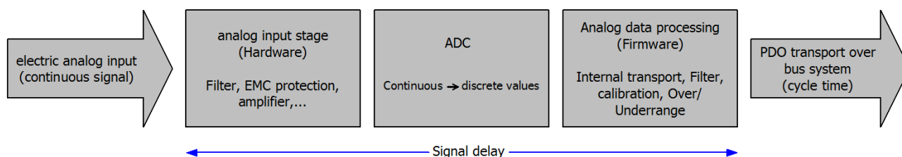
附图 27: 信号处理模拟输入
