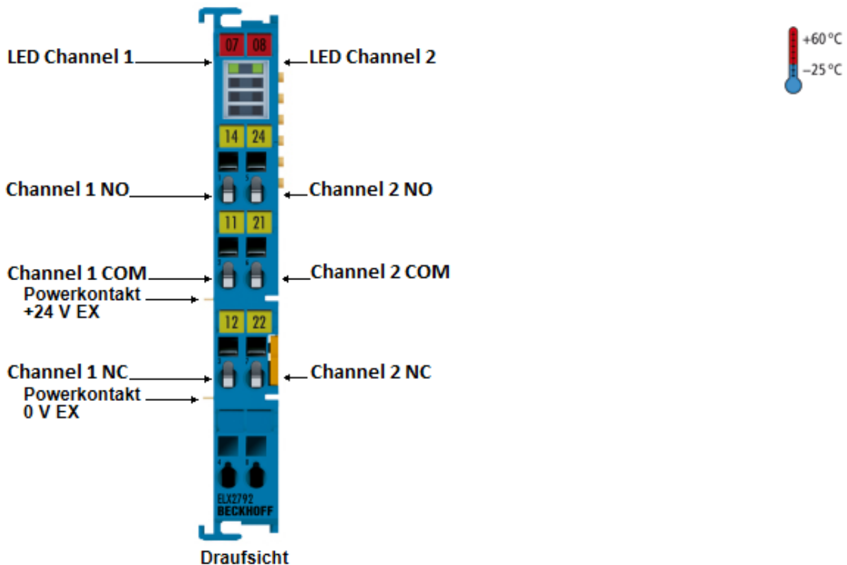
Abb. 19: ELX2792 - Anschlussbelegung und LEDs
