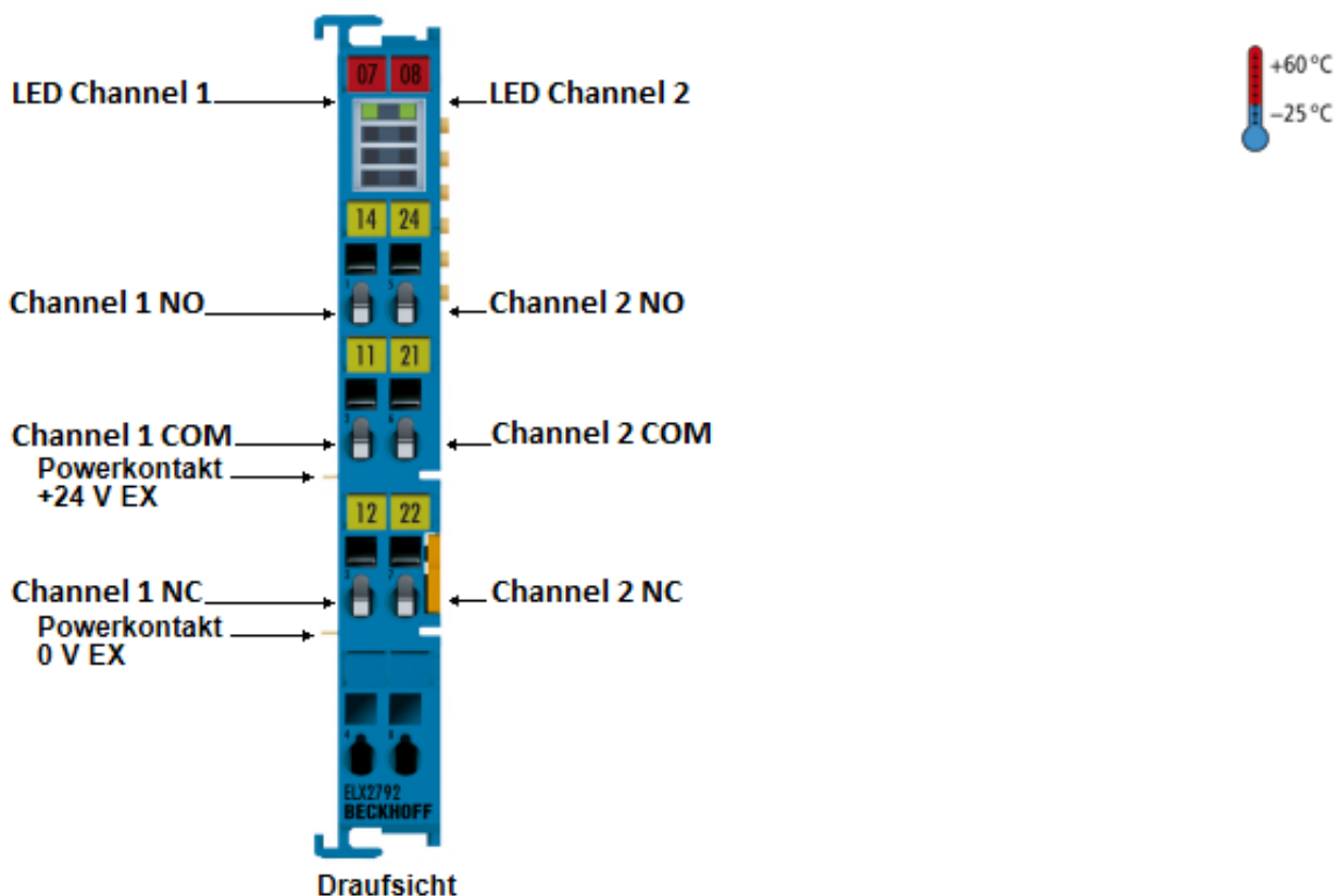
Abb. 4: ELX2792 - Zweikanalige Relais-Ausgangsklemme, Solid State, potenzialfrei, Ex i
