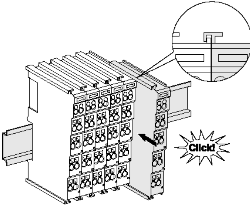
附图 23: 安装在安装轨道上
