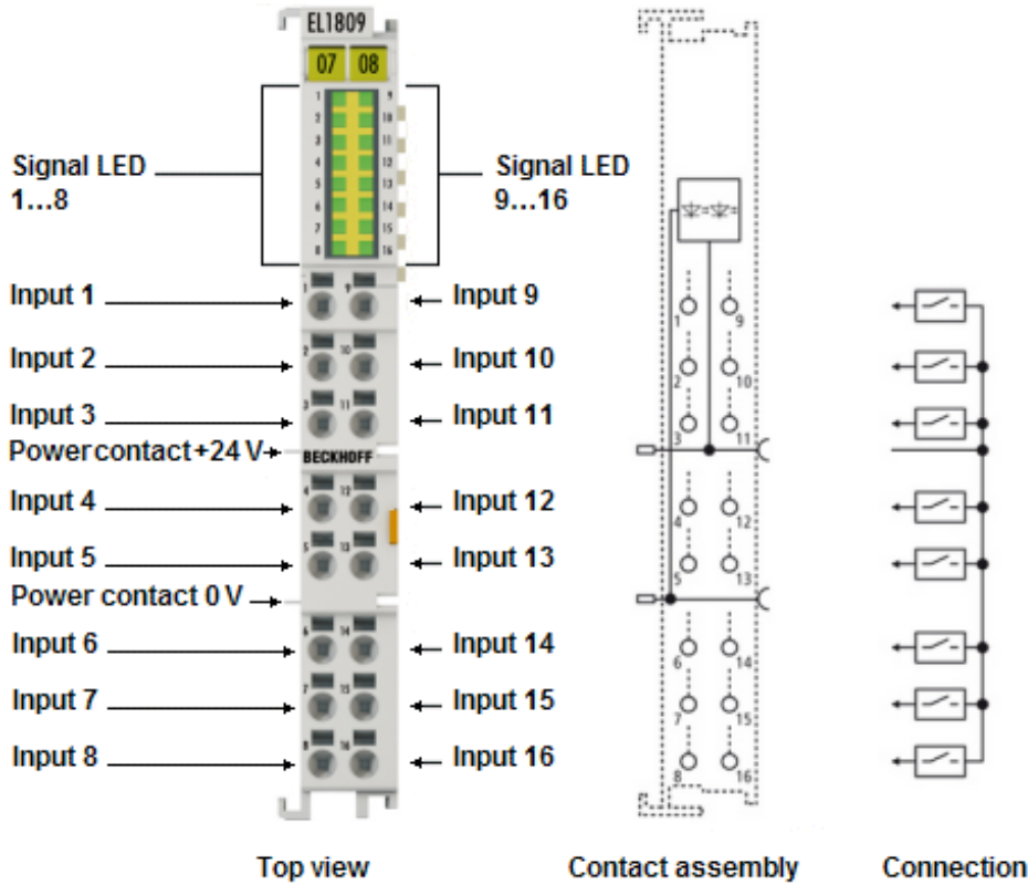
附图 9: EL1809, EL1819
