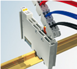
附图 27：可插拔接线
