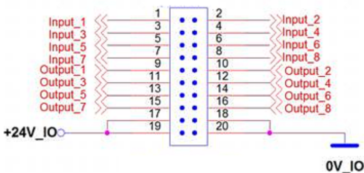
附图 12: 连接器引脚分配
