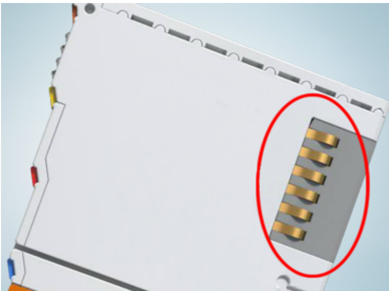
附图 22: 倍福 I/O 组件的弹簧触点
