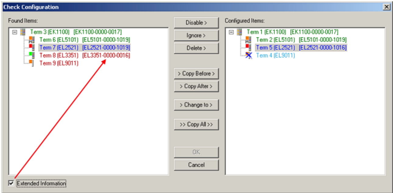
附图 119: 校正对话框
