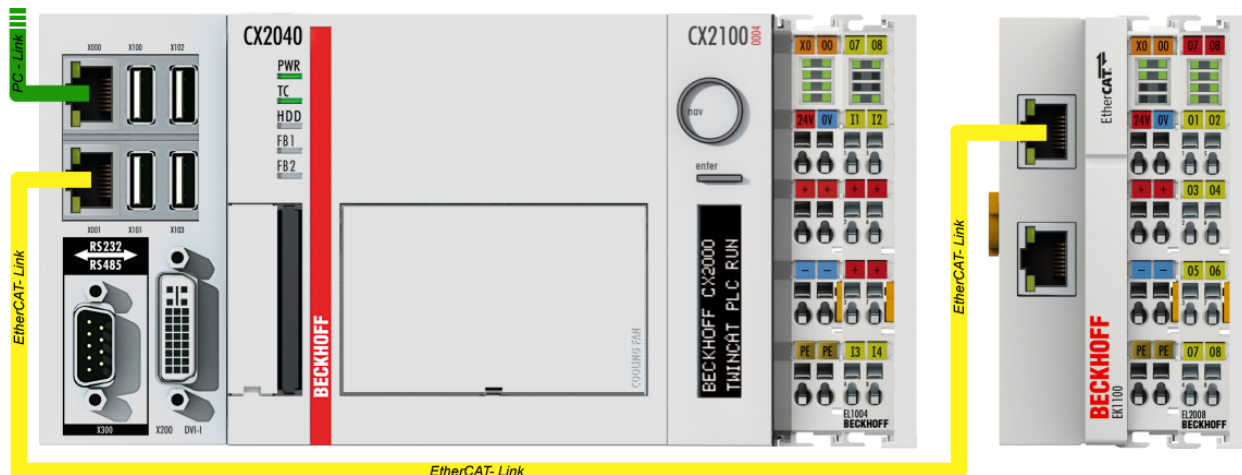
附图 35：控制配置，带嵌入式控制器、输入（EL1004）和输出（EL2008）
