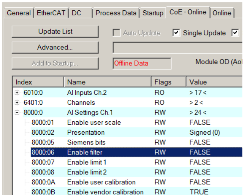
附图 136: EL3102, CoE 目录
