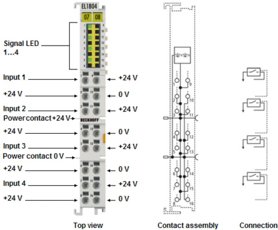
附图 5: EL1804, EL1814
