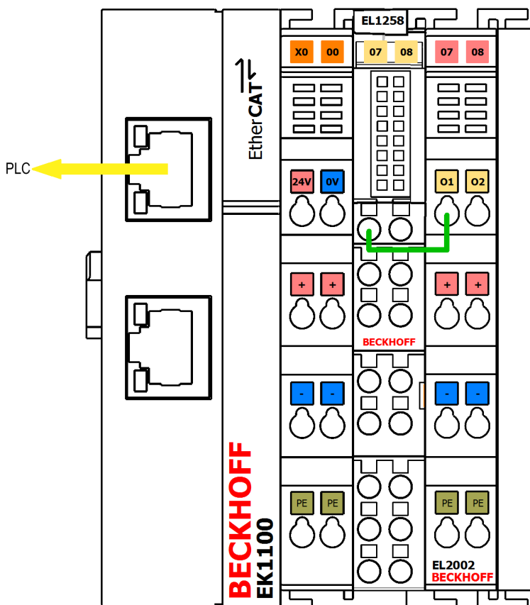
Abb. 179: Empfohlener Aufbau für das Beispielprogramm zur EL1258
