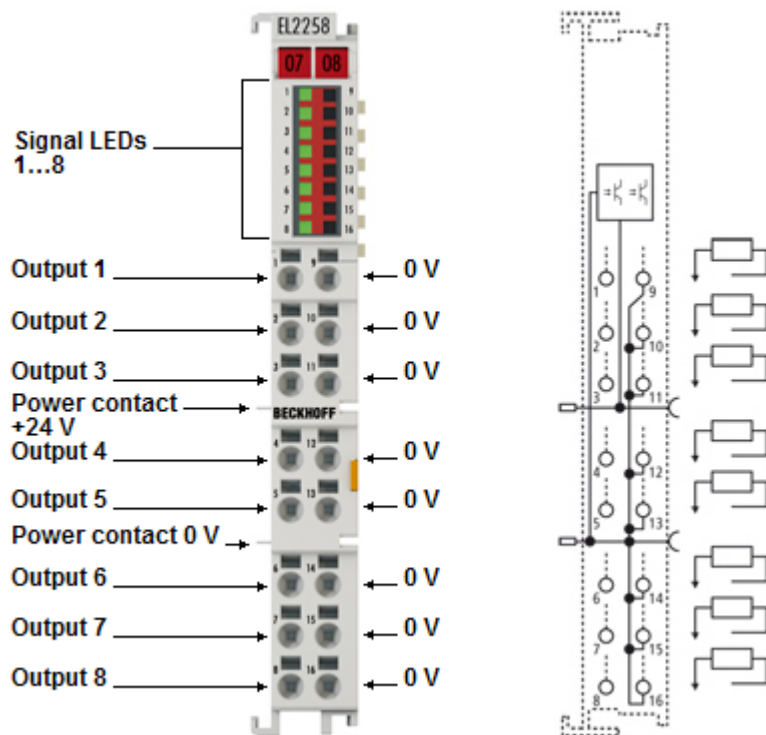
Abb. 10: EL2258
