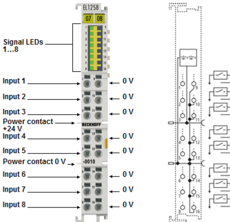
Abb. 20: EL1258-0010
