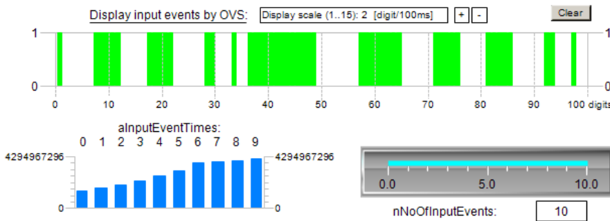
Abb. 182: Beispielprogramm EL1258/ Visualisierung_2: Darstellung eingegangener Ereignisse in zeitlicher Abfolge anhand der Zeitstempel der EL1258
