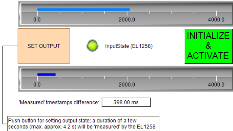
Abb. 181: Beispielprogramm EL1258/ Visualisierung_1: einfache Zeitmessung anhand zweier Zustandswechsel
