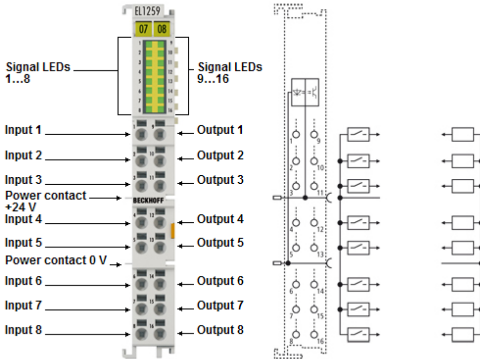
Abb. 21: EL1259
