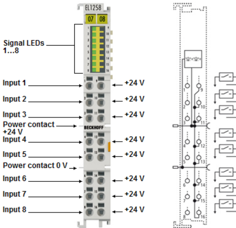
Abb. 19: EL1258
