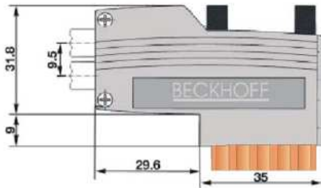
DeviceNet Stecker
