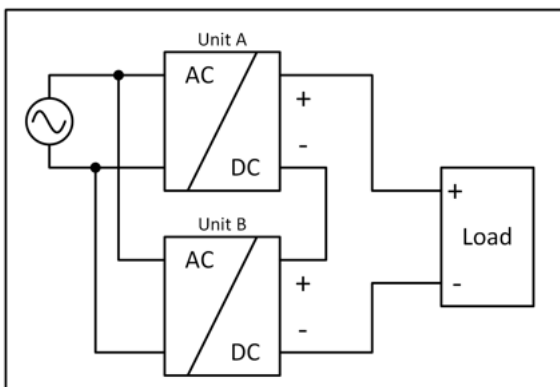
Abb. 14: Serienschaltung
