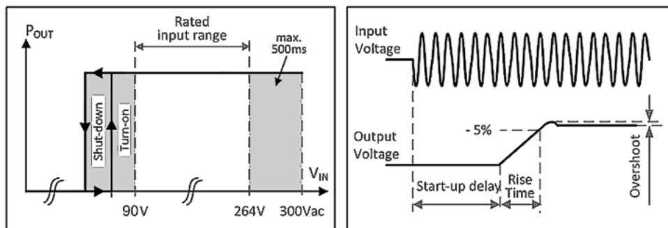
Abb. 1: Eingangsspannungsbereich; Einschaltverhalten-Definitionen
