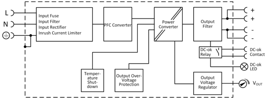
Abb. 10: Funktionsschaltbild
