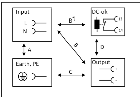
Abb. 13: Spannungsfestigkeit
