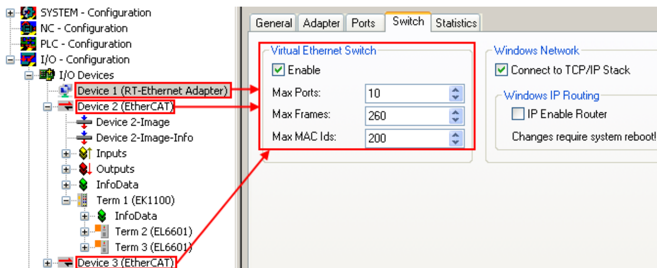
Fig. 40: CU2508 EoE settings
