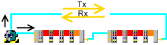
Fig. 41: TwinCAT EtherCAT cable redundancy
